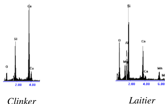
Figure V-16 : Surface polie et spectres EDX d'un grain de laitier de silicomanganèse et d'un grain de clinker
