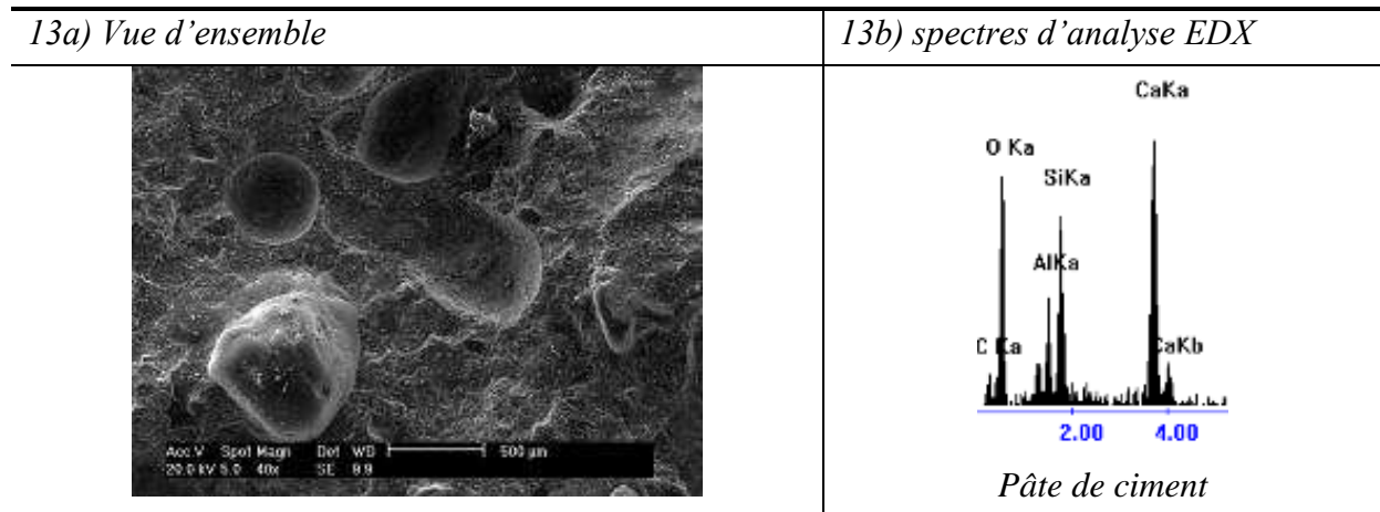
Figure V-13 : Fracture fraîche d'un échantillon de mortier de formule F4 LSiMn à 90 jours observé au MEB et spectre d'analyse EDX de la pâte de ciment
