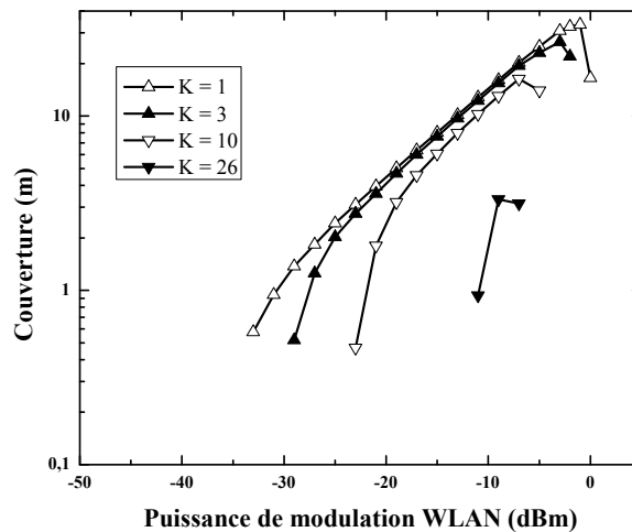
FIGURE 3.25 – Résultats en couverture WLAN en fonction de la puissance de modulation du VCSEL, pour un exposant de pertes de propagation n valant 2 et pour différentes valeurs de K , avec un front-end de gain supérieur de 10 dB par rapport aux résultats de la figure 3.24.
