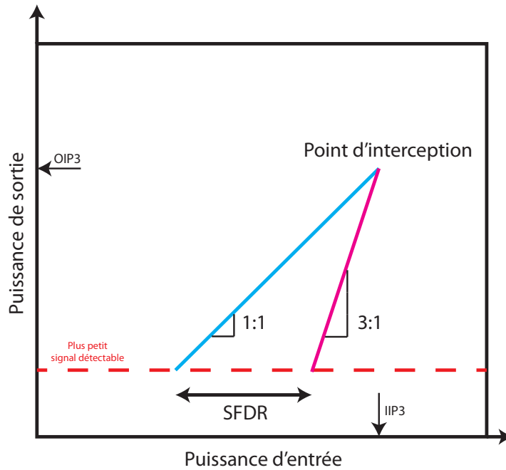
FIGURE 2.12 – Schéma du principe de mesure de SFDR d'un système à partir de mesures de gain AM/AM et d'IIP3.
