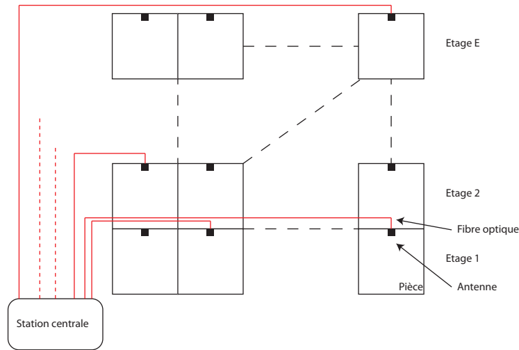
FIGURE 3.7 – Schéma de l'infrastructure lors d'une architecture en étoile est déployée.
