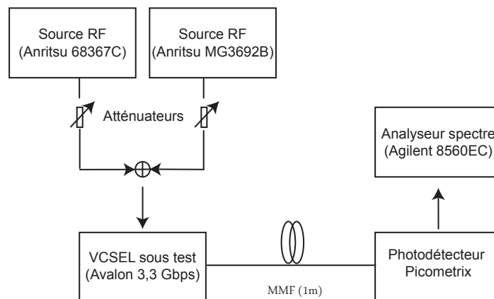
FIGURE 2.10 – Schéma d'expérience de mesures d'IP3.
