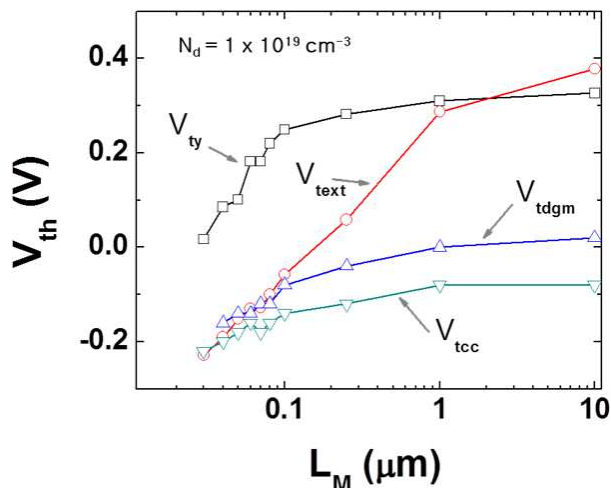
Figure 5. Valeurs de la tension de seuil ( V_{th} ) extraite par différentes techniques en fonction de la longueur de grille. L'extraction a été faite par la méthode Y en inversion ( V_{ty} ), par extrapolation linéaire de la caractéristique de transfert ( V_{text} ), par le maximum de la dérivée de la transconductance ( V_{tdgm} ) et par référence à une densité de courant sous le seuil donnée ( V_{tcc} ).
