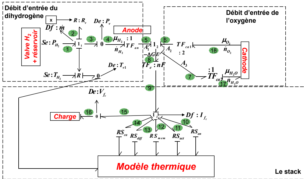
FIGURE 5.4 – Modèle Bond Graph de la pile à combustible
