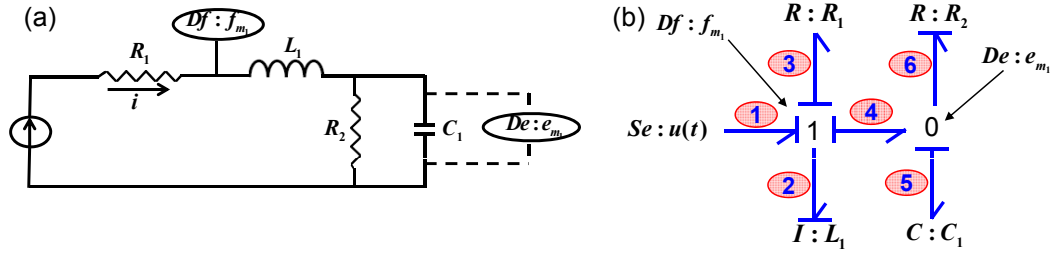
FIGURE 3.4 – Système électrique (a) le modèle bond graph correspondant (b)
