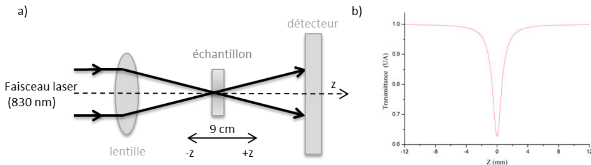
Figure 191. Principe de la technique z-scan en « open aperture »
