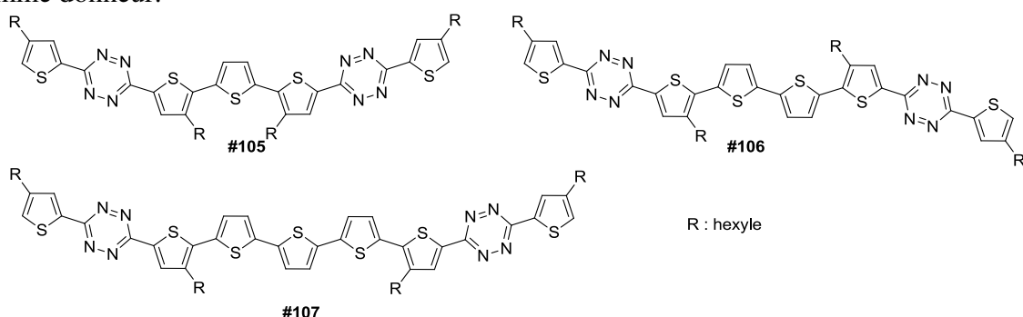
Figure 55. Structures de petites molécules à base de tétrazine utilisées comme donneur dans une cellule photovoltaïque organique
