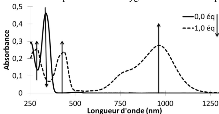
Figure 132. Spectres d'absorption lors de l'oxydation de 39 par \text{Cu}(\text{ClO}_4)_2 dans l'acétonitrile pour [\text{Cu}(\text{II})]/[\text{39}] = 0 et 1 éq, [\text{39}] = 9,3 \cdot 10^{-6} \text{ mol.L}^{-1}
