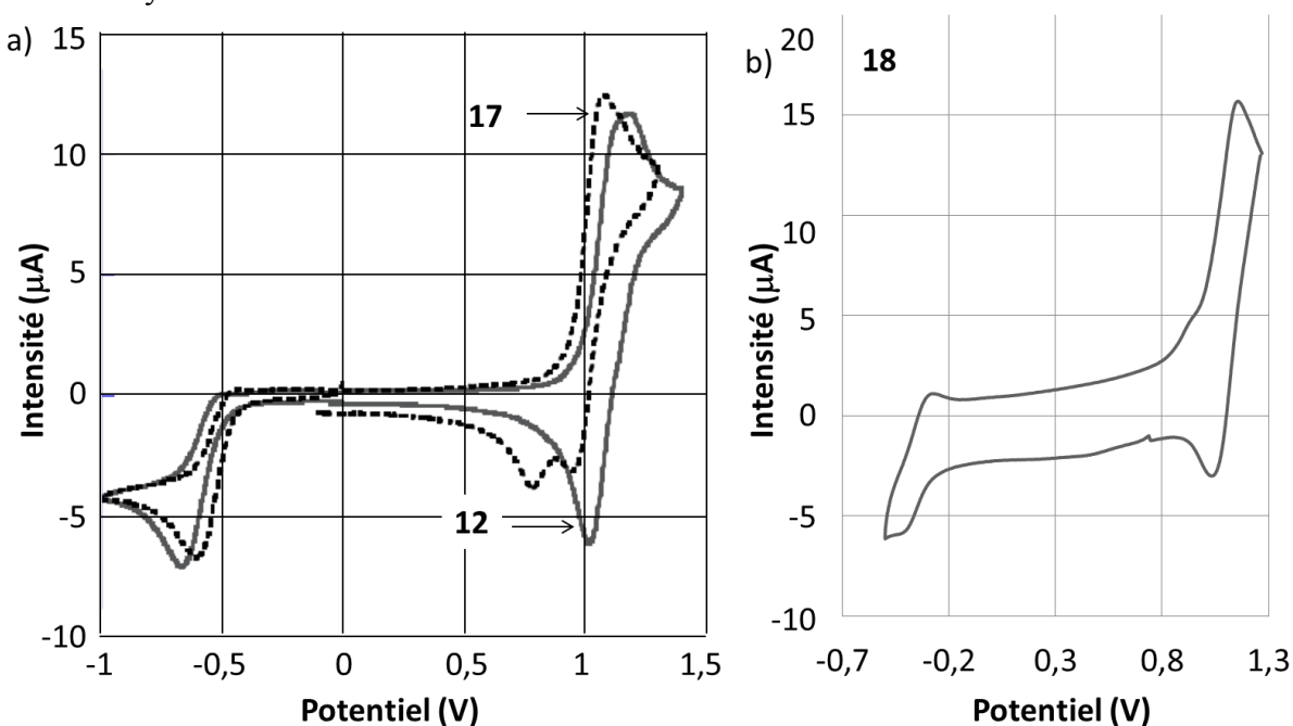
Figure 105. Cyclovoltamogrammes de a) 12 (ligne continue grise) et 17 (ligne pointillée noire) b) 18 . Les potentiels sont référencés par rapport à \text{Ag}^+/\text{Ag} (C, \text{Ag}^+/\text{Ag} , Pt, dichlorométhane, \nu = 0,1 \text{ V}\cdot\text{s}^{-1} ).
