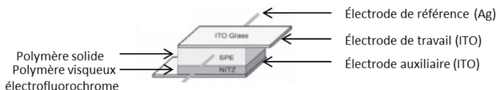
Figure 60. Fenêtre électrofluorescente
