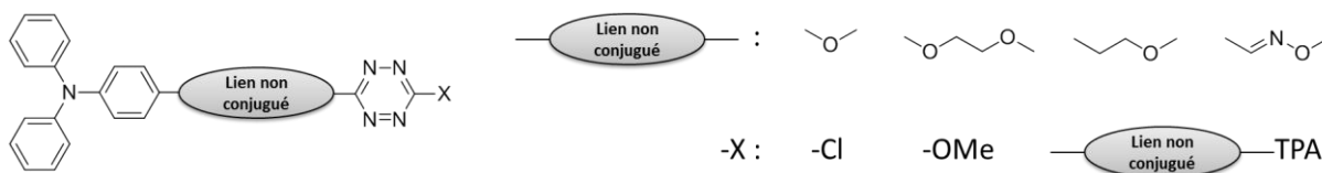
Figure 72. Structures des liens envisagés
