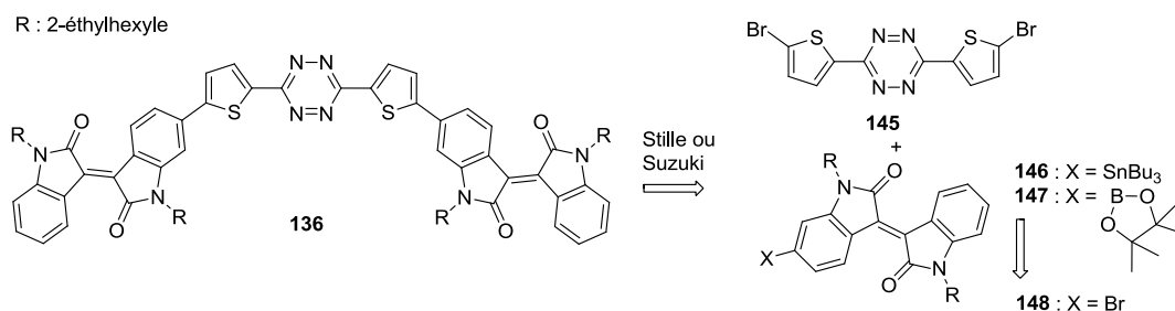
Figure 202. Rétrosynèses de 136
