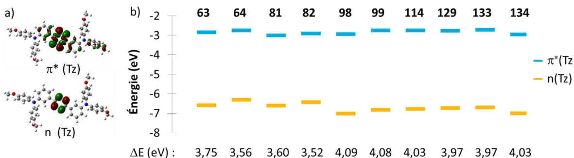
Figure 186. a) Représentation des orbitales n et \pi^* responsables de la bande d'absorption à environ 550 nm de 129 , b) Représentation des énergies des orbitales n et \pi^* pour l'ensemble des composés donneur-attracteur
