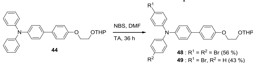
Figure 139. Bromation en positions para de la triphénylamine 44
