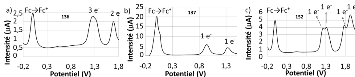
Figure 210. Voltamétrie différentielle pulsée pour a) 136 , b) 137 , c) 152 . Les potentiels sont référencés par rapport au ferrocène (C, Ag + /Ag, Pt, dichlorométhane).
