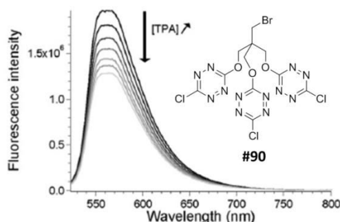
Figure 37. Annihilation de la fluorescence de la tétrazine #90 par ajout de triphénylamine (TPA) de un à six équivalents
