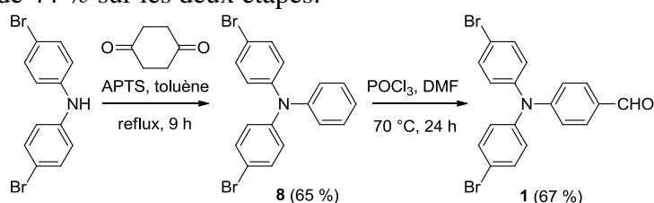
Figure 75. Synthèse de la triphénylamine 1 par la procédure de Kaneko suivie d'une formylation de Vilsmeier-Haack
