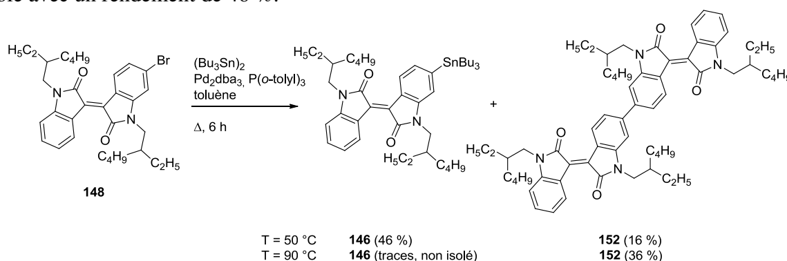
Figure 204. Synthèse de 146
