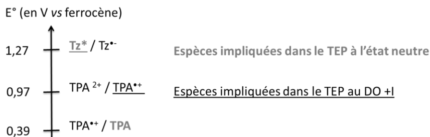
Figure 133. Valeurs des potentiels rédox des couples des espèces impliquées lors de l'oxydation de 39
