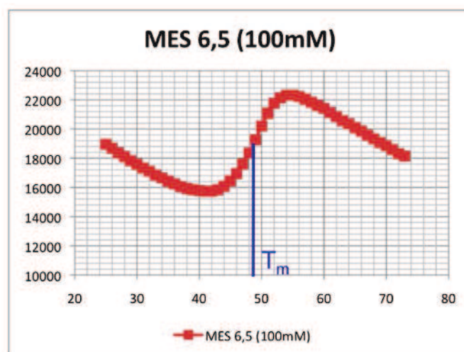
Figure 35 : Représentation graphique d'une mesure en Thermofluor. Le T_m est la valeur de température représentant 50% de la valeur de fluorescence maximale.
