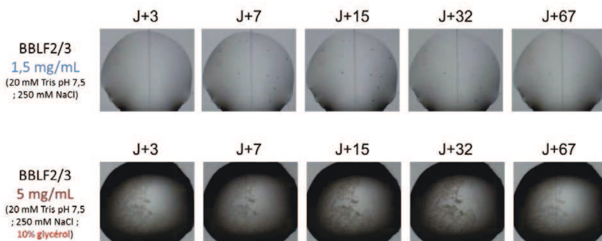
Figure 62 : Clichés des inspections à J+3, J+7, J+15, J+32 et J+67 de BBLF2/3 à 1,5 et 5 mg/mL. Le réservoir contient 100 mM Hépès-Na pH 7,5 ; 100 mM Ammonium Sulfate ; 10 % PEG4000.
