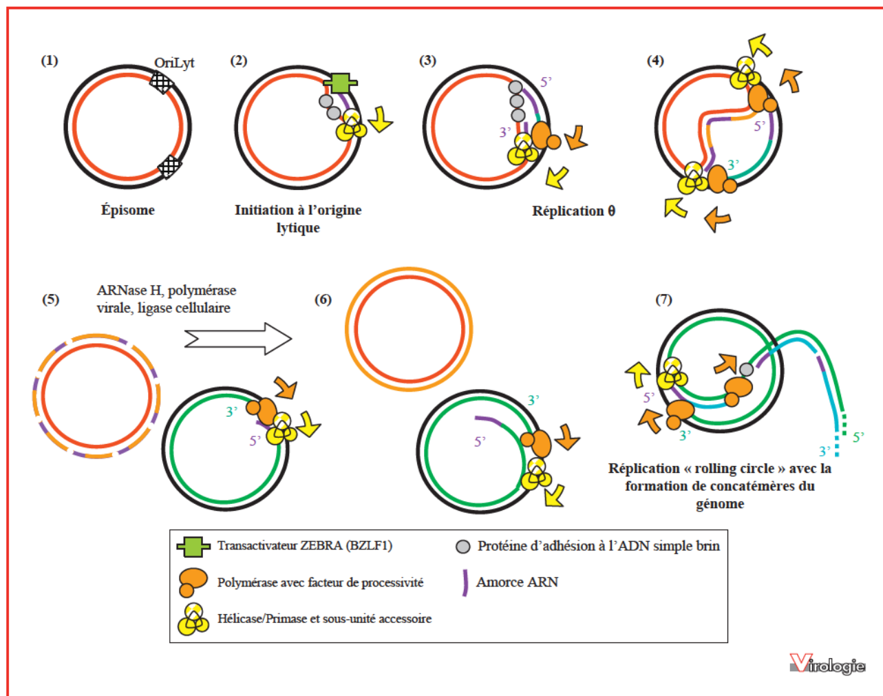
Figure 1. Mécanisme de réplication lytique du virus EBV avec initiation, réplication \theta , et la transition vers la réplication en cercle roulant. Les brins en rouge et noir représentent l'épisode parental, les amorces ARN sont colorées en violet et l'ADN nouvellement synthétisé en orange, vert et bleu. Les flèches colorées indiquent le sens de progression des complexes de l'hélicase-primase et de la polymérase sur l'ADN. (1) Représentation schématisée de l'épisode. (2) Initiation de la réplication au niveau d'OriLyt avec le recrutement du transactivateur ZEBRA, d'un ARNm, de la protéine d'adhésion à l'ADN simple brin et du complexe hélicase-primase. (3) Début de la réplication \theta avec ouverture de la fourche de réplication et début de la synthèse du brin avancé. (4) Progression de la réplication \theta avec synthèse du brin avancé et du brin retardé. (5) Produits à la fin de la réplication \theta : l'épisode répliqué, représenté encore avec les brèches entre les fragments Okazaki du brin retardé ainsi que le brin avancé en transition vers une réplication de type cercle roulant. (6) Finalisation de la réplication de l'épisode par des enzymes cellulaires ARNase H, ligase et la polymérase virale. On retrouve la structure d'ADN double brin circulaire ainsi que le brin avancé qui continue d'être répliqué par le mécanisme du cercle roulant. Un brin retardé complémentaire est synthétisé. (7) Génération de concatémères du génome viral par la réplication de type cercle roulant.
