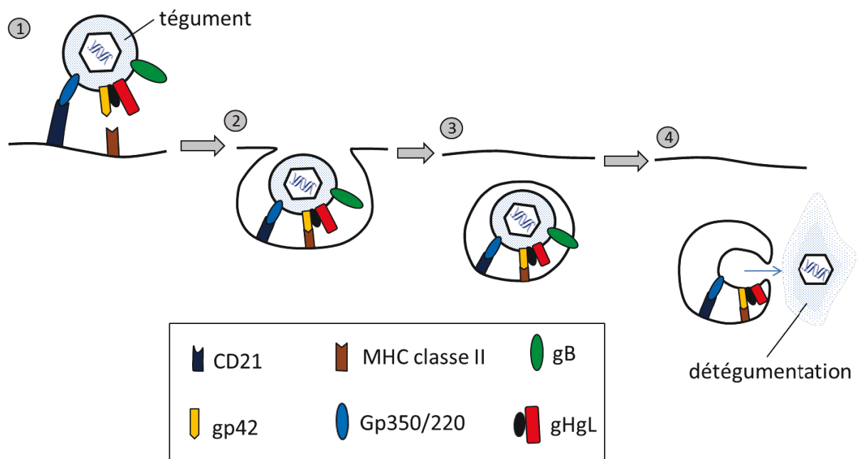
Figure 5 : Mécanismes d'attachement et de fusion au lymphocyte B. Les détails des étapes sont donnés dans le texte. Adapté de Hutt-Fletcher (2007) [17].
