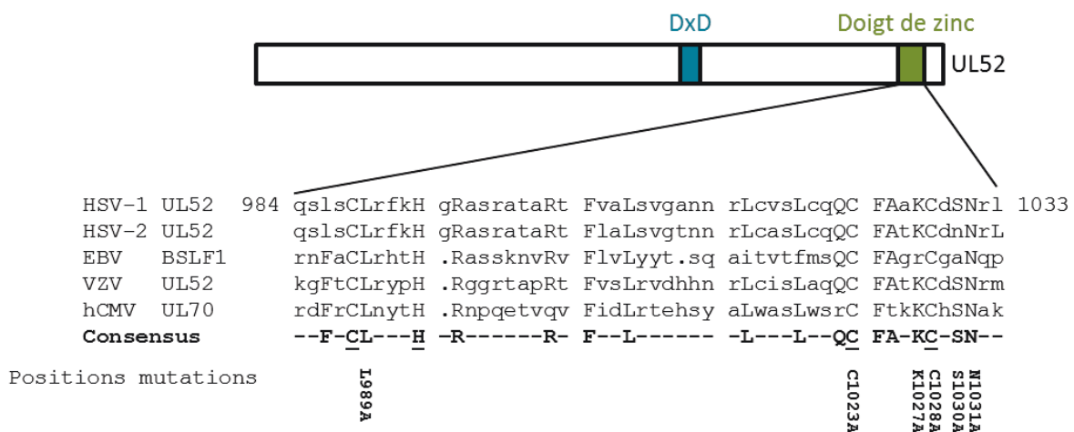
Différents mutants ont été créés pour estimer la contribution du doigt de zinc de la primase sur les activités du complexe H-P. Les mutations des cystéines C1023 et C1028 en alanines (C1023A,C1028A) abolissent la formation du doigt de zinc, les trois autres mutations (L989A, K1027A et la double mutation S1030A,N1031A) impliquent des résidus conservés au sein des herpèsvirus ne contribuant pas directement au maintien de la structure en doigt de zinc (Figure 23). Les tests menés avec les différents mutants ont été réalisés en présence des protéines hélicase (UL5) et sous-unité accessoire (UL8).
