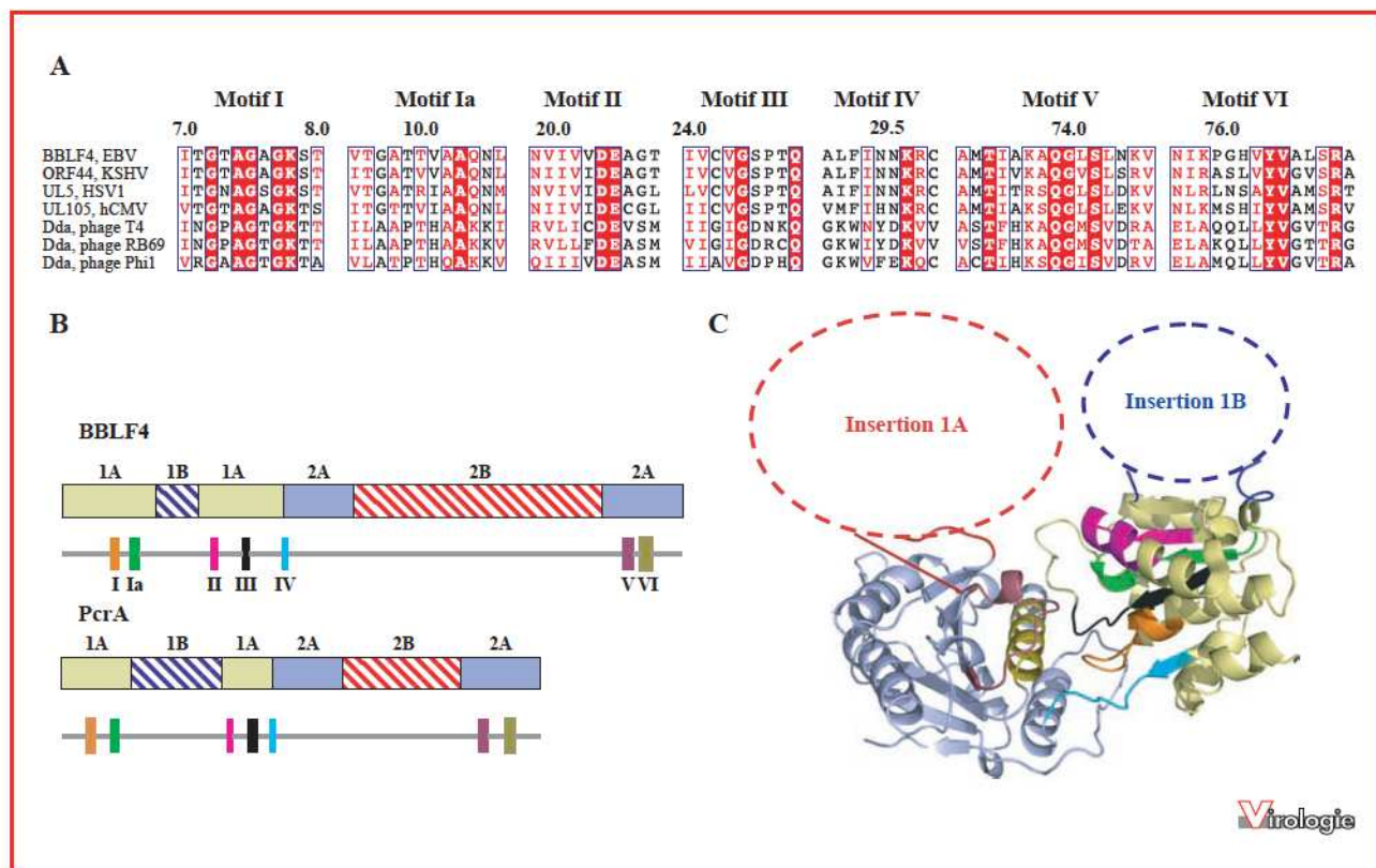
Figure 4. L'hélicase BBLF4. A) Alignement des motifs des hélicases des herpèsvirus avec ceux des hélicases Dda des bactériophages. B) Emplacement des motifs au niveau de la séquence et position des domaines de BBLF4 comparée à celle de PcrA. C) Modèle structural de BBLF4 basé sur PcrA (pdb 1PJR). Motifs et domaines sont colorés comme dans (B).
