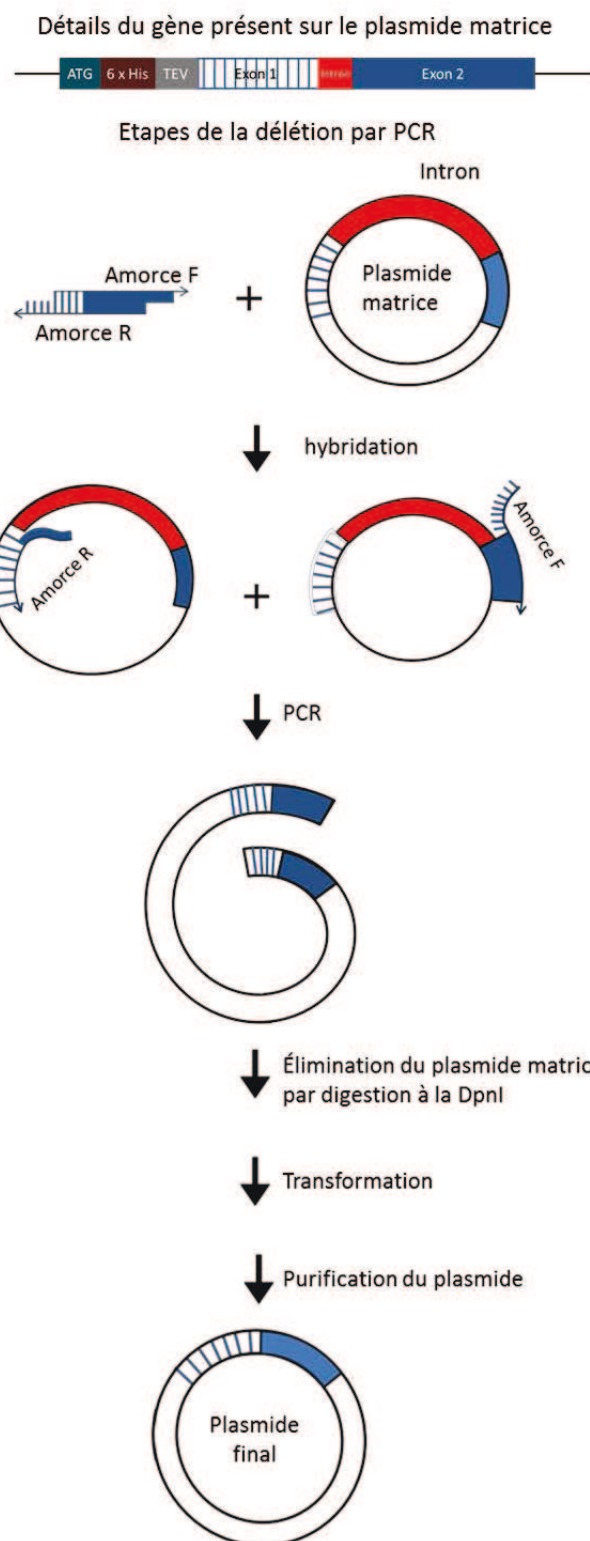
Figure 31 : Principe de la délétion par PCR. Utilisation d'amorce fixant les extrémités des exons 1 et 2, permettant l'amplification complète du plasmide matrice sans l'intron.
