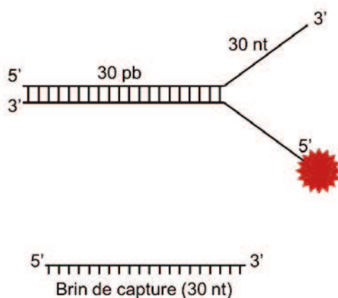
Figure 44 : Substrat de type fourche pour le test hélicase. La cyanine 5 est présente sur le brin 5'. Lors de la séparation de la fourche par l'hélicase, le brin de capture peut se lier au brin non marqué, laissant le brin portant la cyanine 5 sous forme simple brin.
