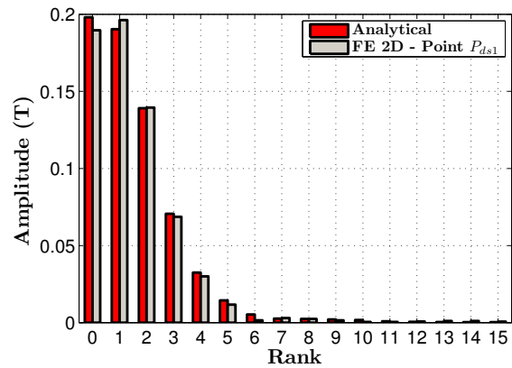
(b) Décomposition harmonique des loci d'induction pour une structure 24-14 plots calculés analytiquement (dent stator) et par EF 2D (point P_{ds1} )
