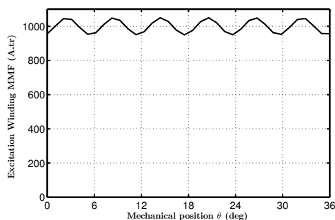
(a) Courant d'excitation avec injection de rang 6
