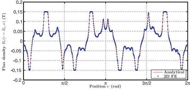
(b) Induction radiale B_r(r = R_e, \nu) calculée analytiquement et par EF 2D : \beta_s = 0.5 et \beta_r = 0.7
