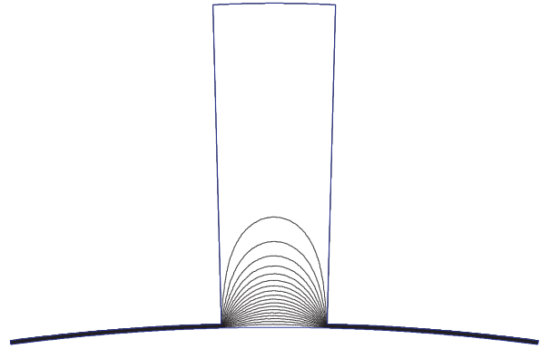
(b) Lignes équipotentielles du potentiel scalaire \psi sous une encoche calculées par EF ( N_s = 24 ) avec \alpha = 0.2
