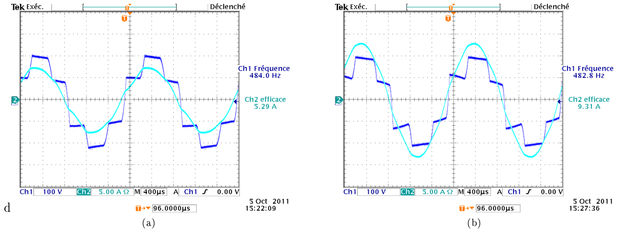
FIGURE 3.27: Forme d'onde pour un point de fonctionnement à 1450\text{tr}/\text{min} : sans capacités (a) et avec capacités de 16\mu\text{F} (b)
