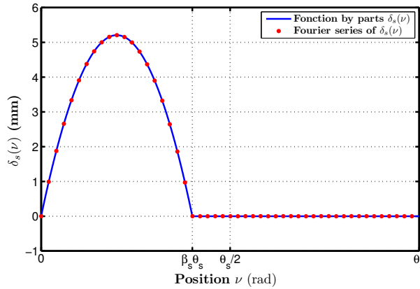
FIGURE 7.6: Evolution de la fonction représentant d'entrefer additionnel \delta_s(\nu) : Fonction réelle (7.12) et son développement en série de Fourier (7.13)
