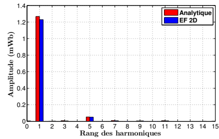
(b) Décompositions harmoniques du flux \varphi_s pour la structure 24-12 plots
