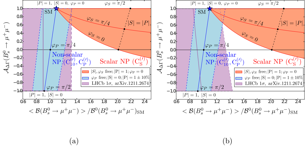
Figure 10: Régions permises dans le plan \mathcal{B}(B_s^0 \rightarrow \mu^+ \mu^-) / \mathcal{B}(B_s^0 \rightarrow \mu^+ \mu^-)_{SM} \times \mathcal{A}_{\Delta\Gamma} si les contributions de la nouvelle physique sont scalaires (rouge) ou non-scalaire (bleue) sur imprimée avec la contrainte expérimentale (violette) avec (b) ou sans (a) la dépendance en \mathcal{A}_{\Delta\Gamma} [17].
