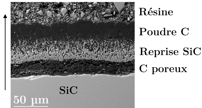
V-F. 31 : Image MEB-BSE illustrant la phase interne riche en C du tube réalisé avec 3 %vol. de C_3H_6 et zone de préchauffage
