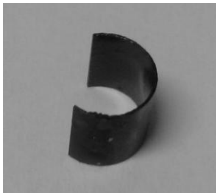
II-F. 22 : éprouvette SiC ( \alpha = 2 , T = 1100 °C, Q_{\text{tot}} = 500 sccm, V_0 = 0 ) en forme de C
