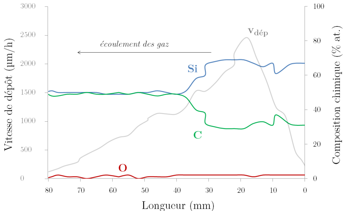
V-F. 1 : Profil longitudinal d'épaisseur et de composition pour le tube élaboré sans déplacement ( \alpha = 2 , T = 1200\text{ °C} , Q_{\text{tot}} = 1000\text{ sccm} )
