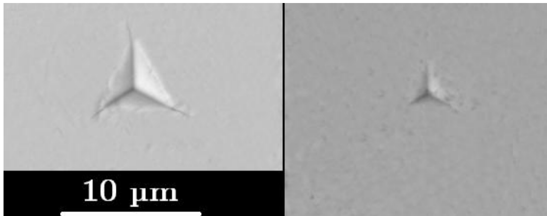
VI-F. 3 : Différence de profondeur de pénétration selon la zone étudiée (gauche : SiC+Si, droite : SiC)
