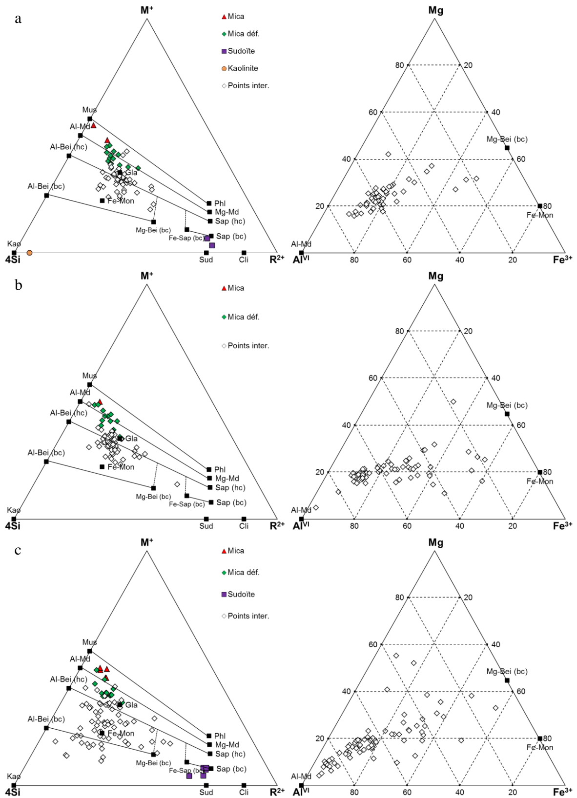
FIGURE III-24. Composition chimique de la fraction < 4 \mu m des échantillons du groupe I avec (a) : BARB ; (b) : STSY et (c) : CARO-G placés dans les diagrammes M^+-4Si-R^{2+} (adaptés d'après Meunier & Velde, 1989). Les points expérimentaux de compositions intermédiaires entre plusieurs phyllosilicates ont aussi été placés dans les diagrammes Mg-Al^{VI}-Fe^{3+} (à droite).
