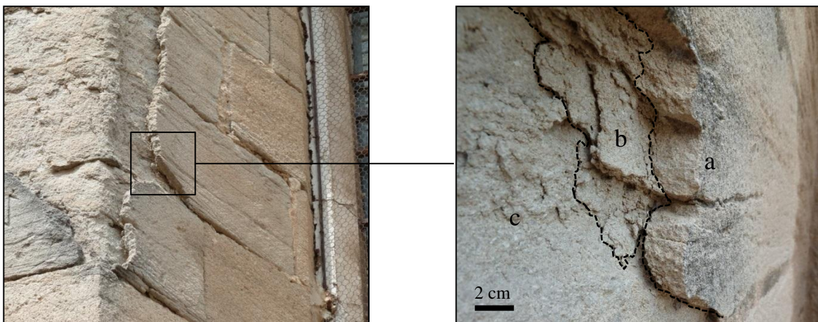
FIGURE I-1. Morphologie de la desquamation en plaques touchant la pierre de Caromb (à gauche) et observable sur la façade Sud de l'église Saint Maurice de Caromb (Vaucluse, France). Détail (à droite) des trois zones distinguables à la surface d'une assise affectée. Les traits pointillés délimitent la plaque en formation (a) de la zone fracturée (b). Une zone non affectée (c) apparaît à la suite de la chute d'une partie de la plaque.
