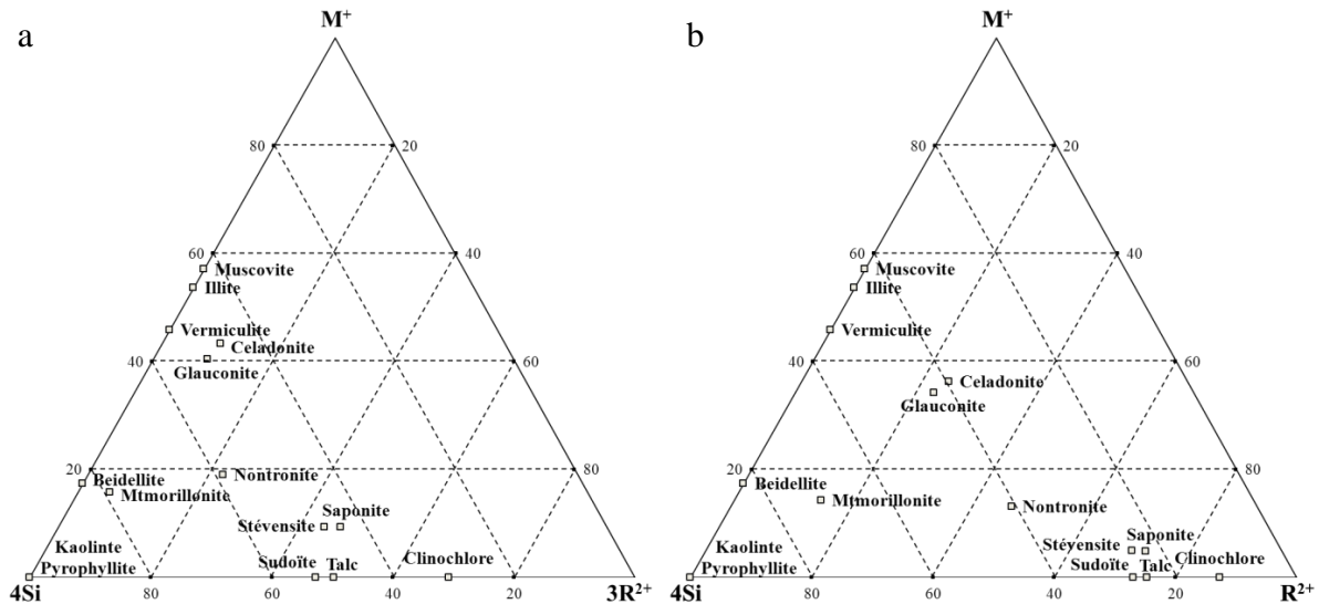
FIGURE I-19. Projections de la composition chimique des principaux phyllosilicates dans les diagrammes ternaires M^+-4Si-3R^{2+} (a) et M^+-4Si-R^{2+} (b) (d'après Meunier & Velde, 1989).
