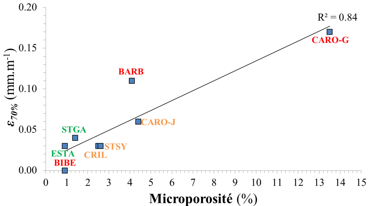
FIGURE V-5. Relation entre la microporosité et le coefficient de dilatation hygrique ( \varepsilon ) mesuré à 70 % d'humidité relative.
