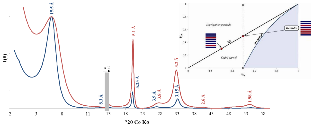
FIGURE III-11. Intensité diffractée calculée pour une structure interstratifiée glauconite / Fe-montmorillonite 2W ( N = 20 ). Cas de l'empilement aléatoire (ou désordre P_{AA} = W_A ) dit R0 avec des proportions relatives variables entre les deux composants (50-50 en rouge et 30-70 en bleu). Position sur le diagramme de probabilité donnée en vignette.
