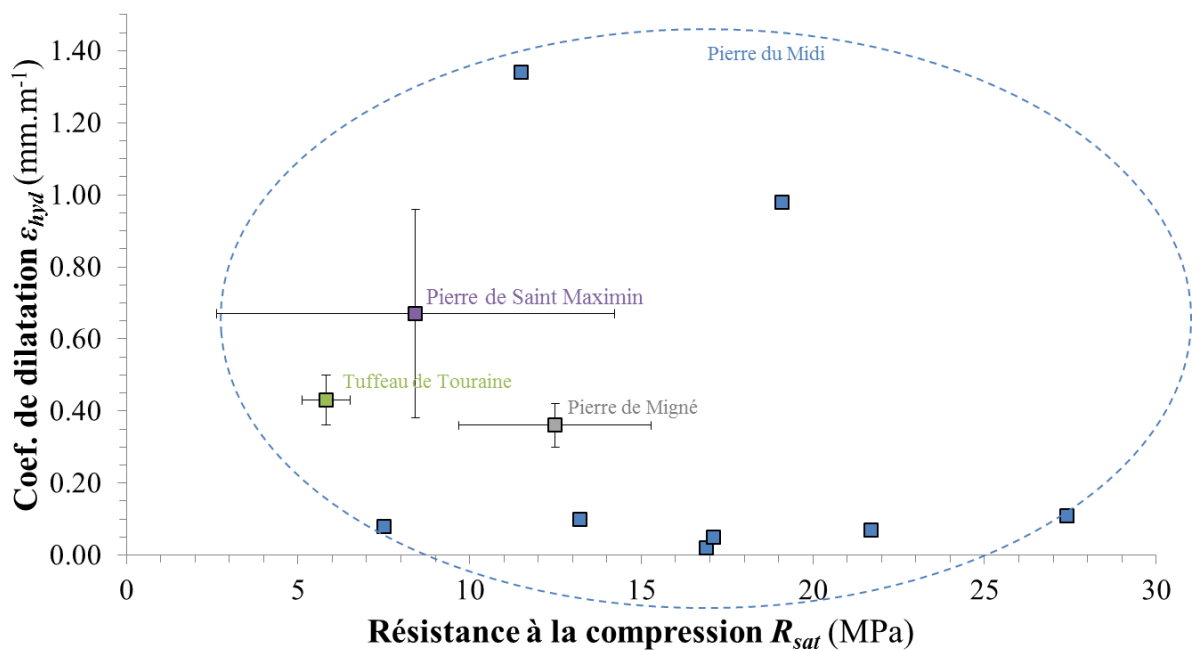
FIGURE IV-27. Relation entre le coefficient de résistance à la compression à l'état saturé en eau ( R_{sat} ) et le coefficient de dilatation hydrique \epsilon_{hyd} des grandes familles de pierres sédimentaires françaises.
