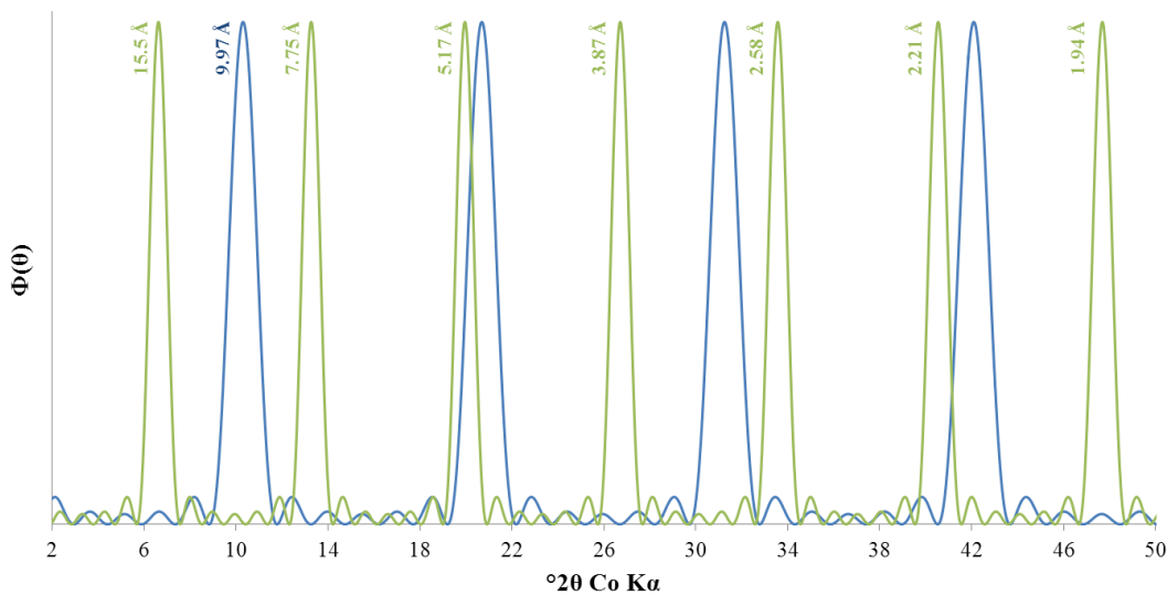
FIGURE III-1. Fonction d'interférence calculée pour des d_{001} de 15,5 Å (en vert) et 9,97 Å (en bleu). Dans chaque cas le nombre de feuillets participant à la diffraction cohérente N est égal à 7.
