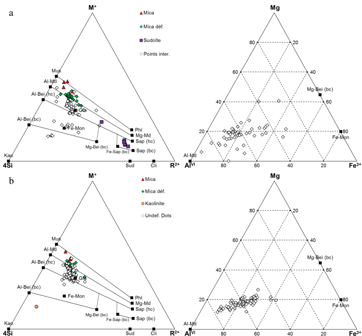
FIGURE III-25. Composition chimique de la fraction < 4 \mu\text{m} des échantillons du groupe II avec (a) : STGA et (b) : VILL-G placés dans les diagrammes \text{M}^+-4\text{Si}-\text{R}^{2+} (adaptés d'après Meunier & Velde, 1989). Les points expérimentaux de compositions intermédiaires entre plusieurs phyllosilicates ont aussi été placés dans les diagrammes \text{Mg}-\text{Al}^{\text{VI}}-\text{Fe}^{3+} (à droite).
