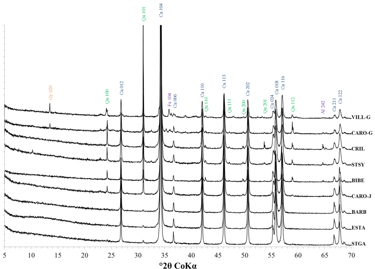
FIGURE II-26. Diffractogrammes de rayons X sur poudre totale des échantillons. Avec, Ca : calcite, Qu : quartz, Gy : gypse et Fe : feldspath alcalin. Les indices de Laue (indices de Miller ( hkl ) x l'ordre de la diffraction) sont indiqués pour chaque pic de diffraction.
