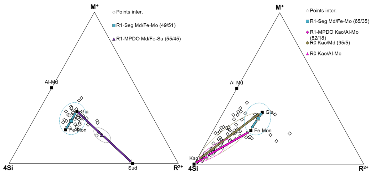
FIGURE III-40. Répartition des phases interstratifiées des échantillons (a) BARB et (b) BIBE dans les diagrammes ternaires M^+ - 4Si - R^{2+} basée sur les résultats de la simulation des raies 00 l de diffraction des rayons X. Les cercles pointillés englobent les points d'analyses appartenant aux phases interstratifiées utilisées pour la simulation des diffractogrammes de rayons X.
