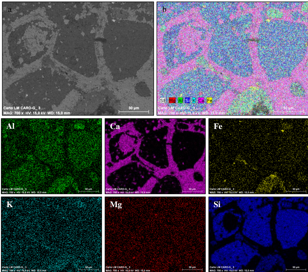
FIGURE III-50. Cartographies élémentaires obtenues en microscopie électronique à balayage (MEB) en mode électrons rétrodiffusés (BSE) sur la zone 2 de l'échantillon CARO-G avec (a) l'image de la zone cartographiée ; (b) l'image recomposée des différents éléments dosés ainsi que les cartographies de ces éléments (Al, Ca, Fe, K, Mg et Si).
