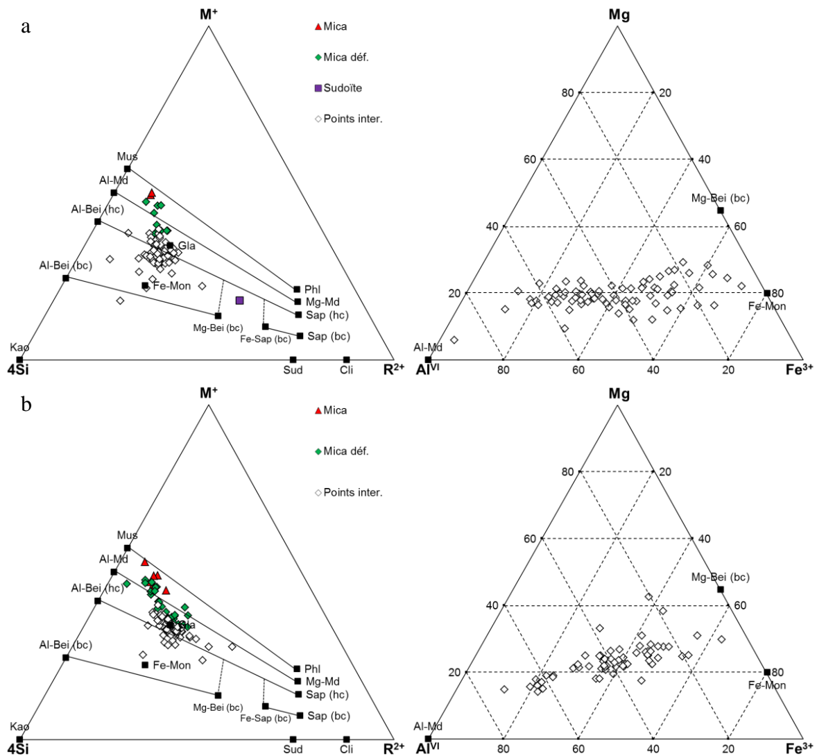
FIGURE III-26. Composition chimique de la fraction < 4 \mu m des échantillons du groupe II avec (a) : CRIL et (b) : CARO-J placés dans les diagrammes M^+ - 4Si - R^{2+} (adaptés d'après Meunier & Velde, 1989). Les points expérimentaux de compositions intermédiaires entre plusieurs phyllosilicates ont aussi été placés dans les diagrammes Mg - Al^{VI} - Fe^{3+} (à droite).
