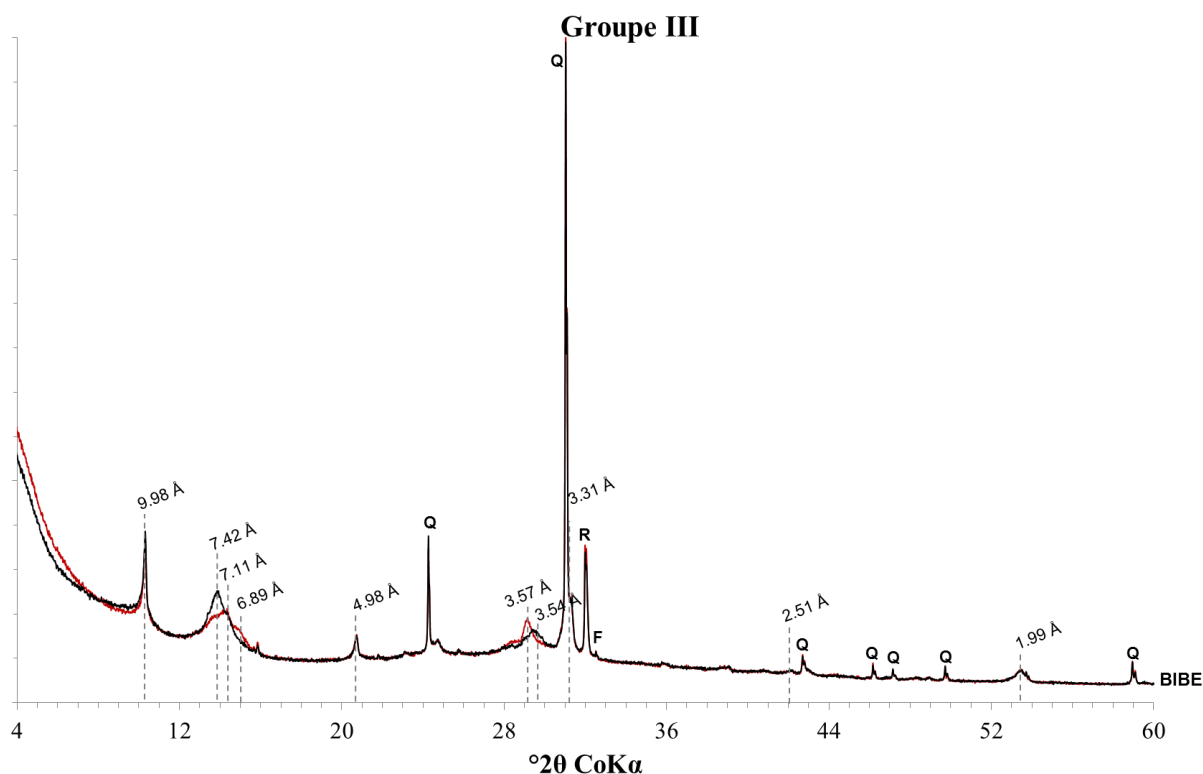
FIGURE III-22. Diffractogrammes expérimentaux des fractions < 4 \mu\text{m} des échantillons appartenant au groupe III (BIBE). Les couleurs et symboles sont les mêmes que ceux utilisés dans la figure III-20.
