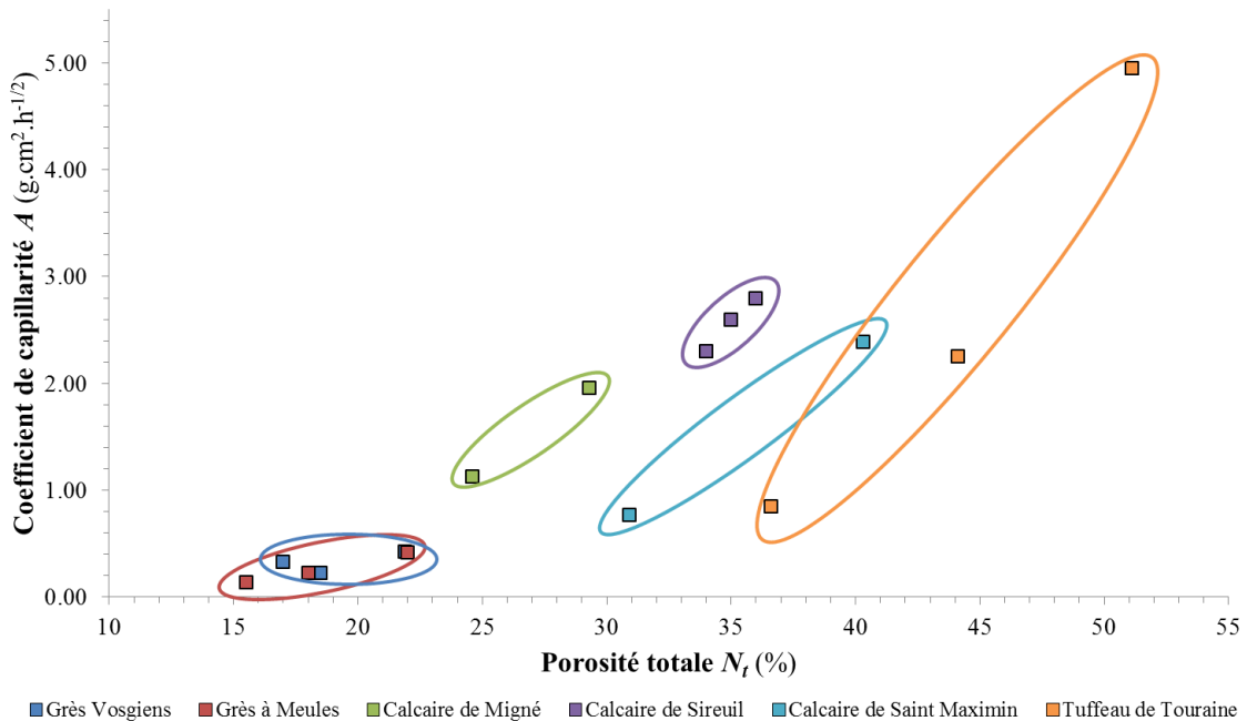
FIGURE I-6. Relation entre la porosité totale ( N_r ) et le coefficient de capillarité (A) de plusieurs pierres de construction (d'après Dessandier, 2000 et Colas, 2011).
