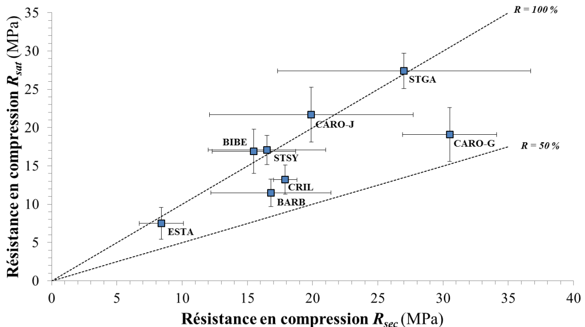
FIGURE IV-17. Comparaison des résistances à la compression uniaxiale à l'état sec ( R_{sec} ) et saturé en eau ( R_{sat} ).
