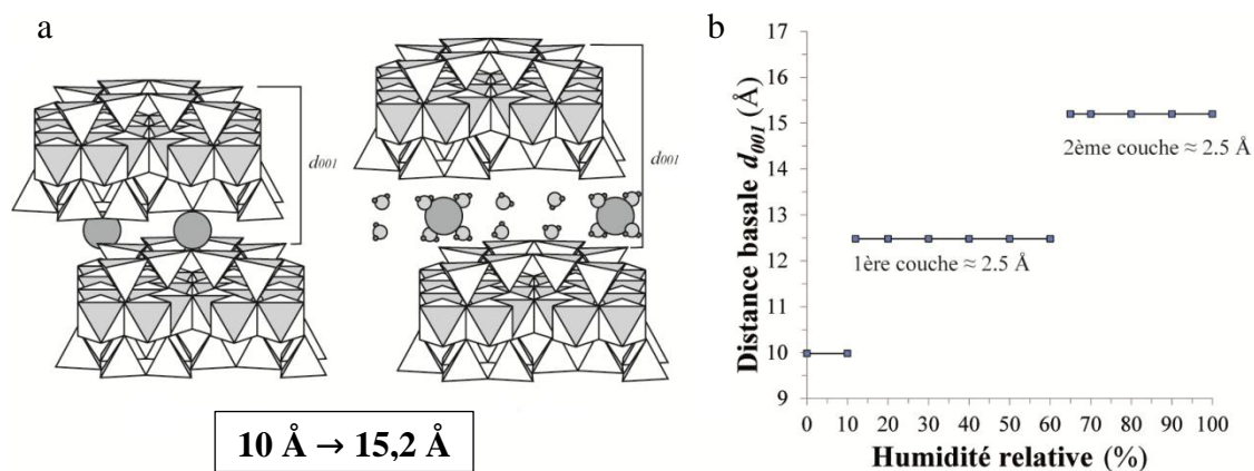
FIGURE I-22. Représentation schématique du gonflement intracristallin des phyllosilicates 2/1 (a) et évolution de la distance basale ( d_{001} ) en fonction de l'humidité relative (b).
