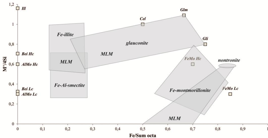
FIGURE V-12. Domaines de composition des phases de phyllosilicates riches en fer dans le diagramme binaire de coordonnées M^+ / 4Si versus Fe / Somme\ octaèdre (d'après Meunier & El Albani, 2006).
