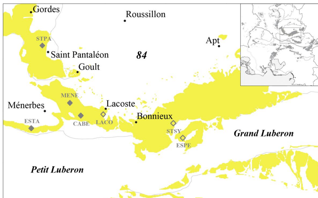
FIGURE II-9. Répartition des principales carrières d'extraction de pierre de taille au sein du sous-bassin d'Apt. Les losanges vides représentent les carrières abandonnées et les losanges pleins représentent les carrières en activité.
