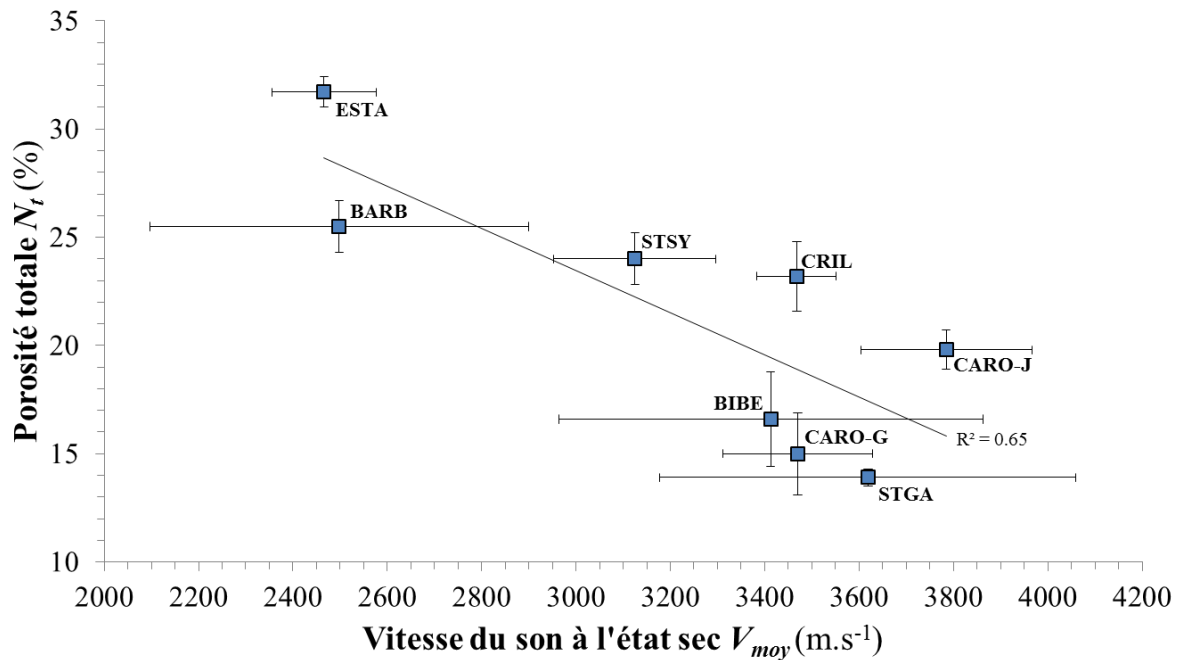
FIGURE IV-16. Relation entre la vitesse de propagation des ondes ultrasoniques V_{moy} mesurée à l'état sec et la porosité totale accessible à l'eau N_t .
