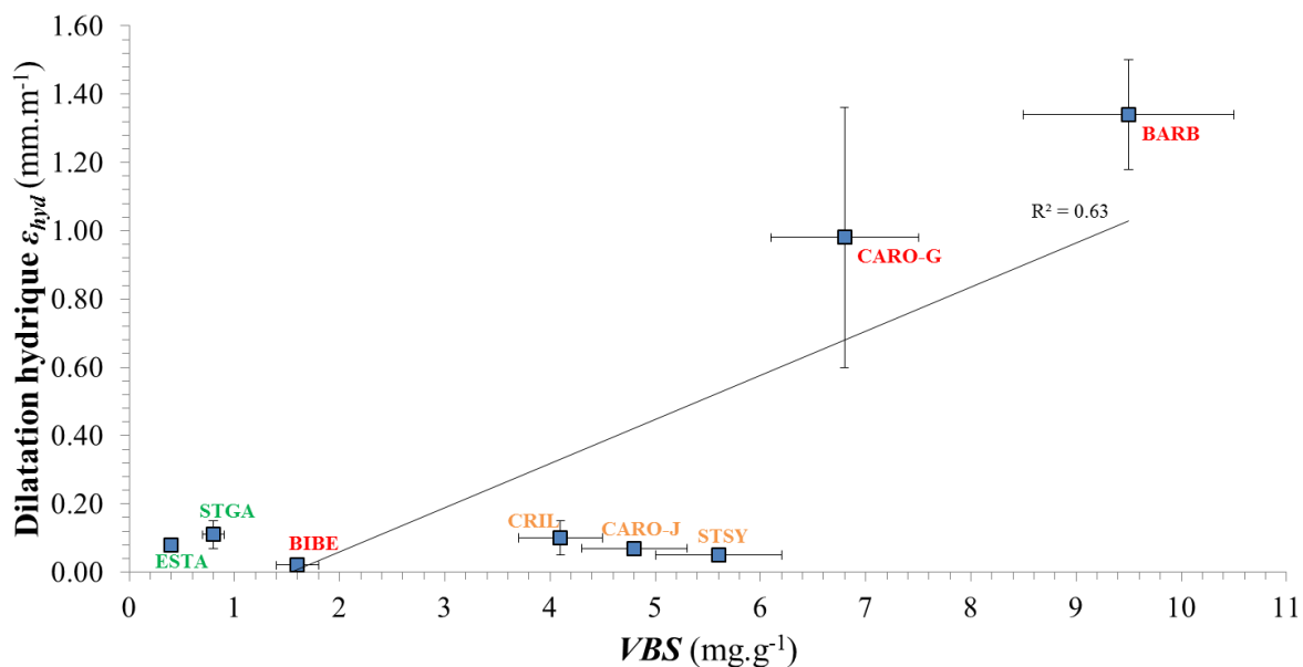
FIGURE V-11. Relation entre la valeur au bleu (VBS) et le coefficient de dilatation hydrique \epsilon_{hyd} .
