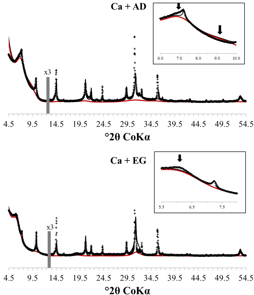
FIGURE III-38. Contribution de la phase interstratifiée R1-ségrégé glauconite/Al-montmorillonite (formule structurale théorique) à l'intensité calculée pour la simulation des diffractogrammes de rayons X de l'échantillon BARB à l'état AD (en haut) et EG (en bas). Les flèches noires indiquent les écarts de simulation causés par la composition et la répartition des cations dans les feuillets de montmorillonite.
