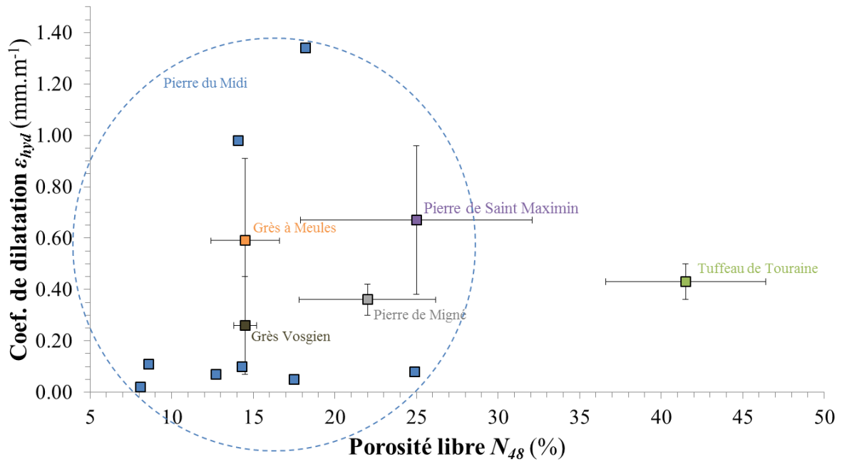
FIGURE IV-26. Relation entre la porosité libre ( N_{48} ) et le coefficient de dilatation hydrique ( \epsilon_{hyd} ) des grandes familles de pierres sédimentaires françaises.
