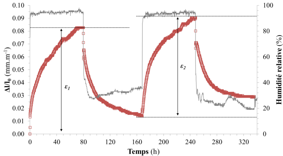
FIGURE IV-6. Exemple de la courbe dilatométrique de l'échantillon CARO-J (carrés rouges) en fonction de la variation de l'humidité relative (trait gris) et définition graphique des paramètres \epsilon_1 et \epsilon_2 utilisés pour le calcul de Z.
