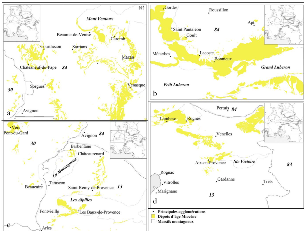
FIGURE II-2. Cartographie des différents sous-bassins étudiés dont, (a) : le sous-bassin d’Avignon-Carpentras ; (b) : le sous-bassin d’Apt ; (c) : le sous-bassin des Alpilles et (d) : le sous-bassin d’Aix-en-Provence.
