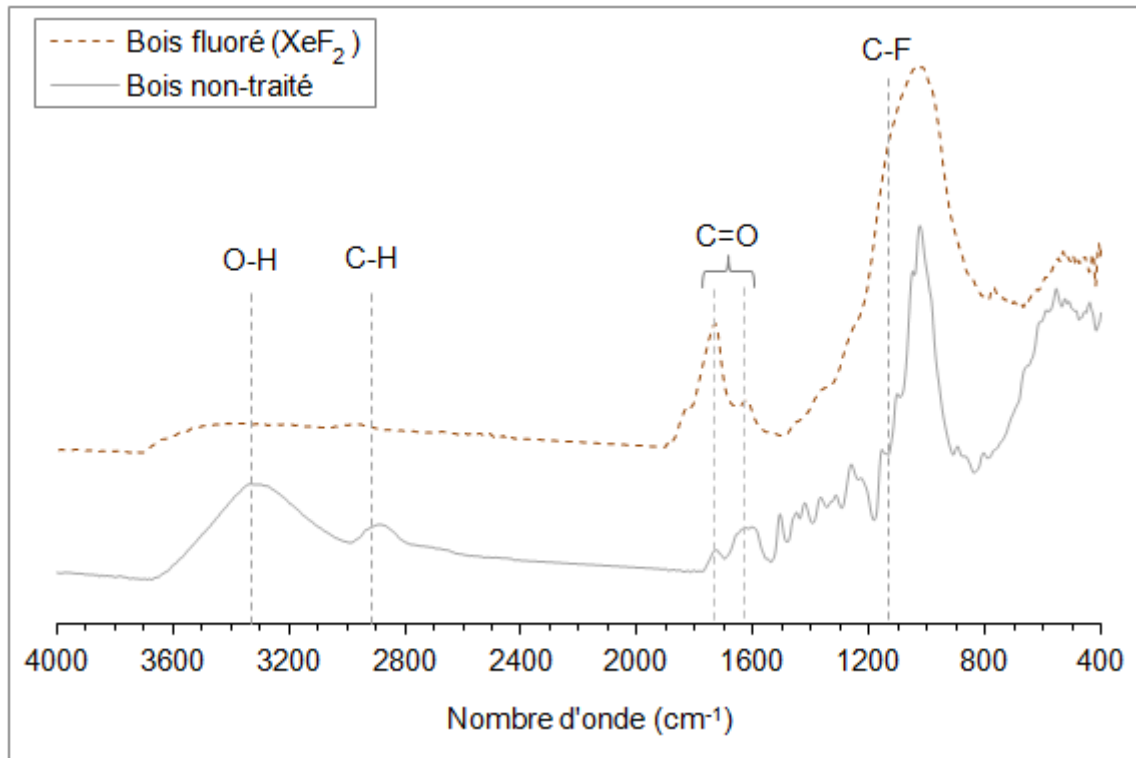
Figure III-7 – Spectres FT-IR normalisés des farines de bois non-traitée et traitée par agent fluorant XeF 2
