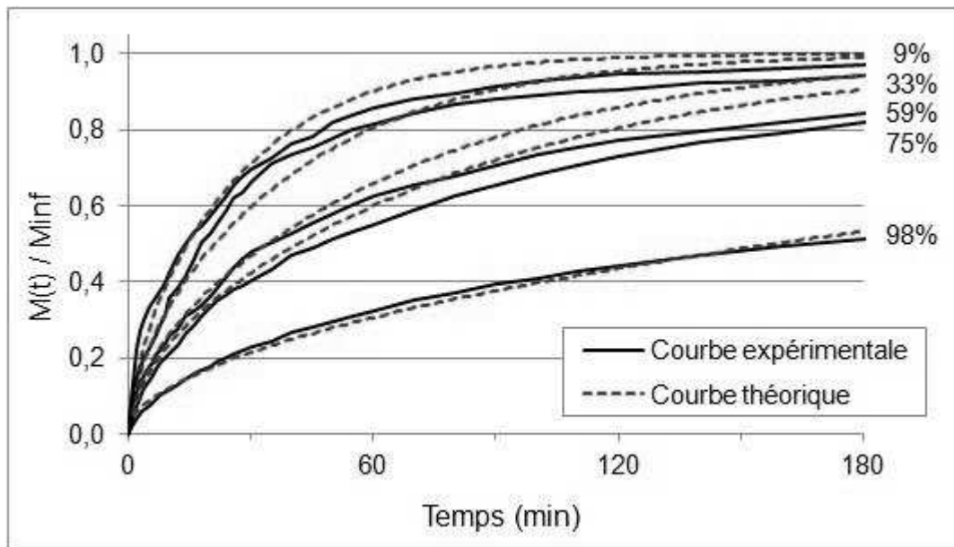
Figure III-26 – Courbe \alpha = M_t/M_\infty en fonction du temps pour le bois non-traité aux diverses humidité relatives
