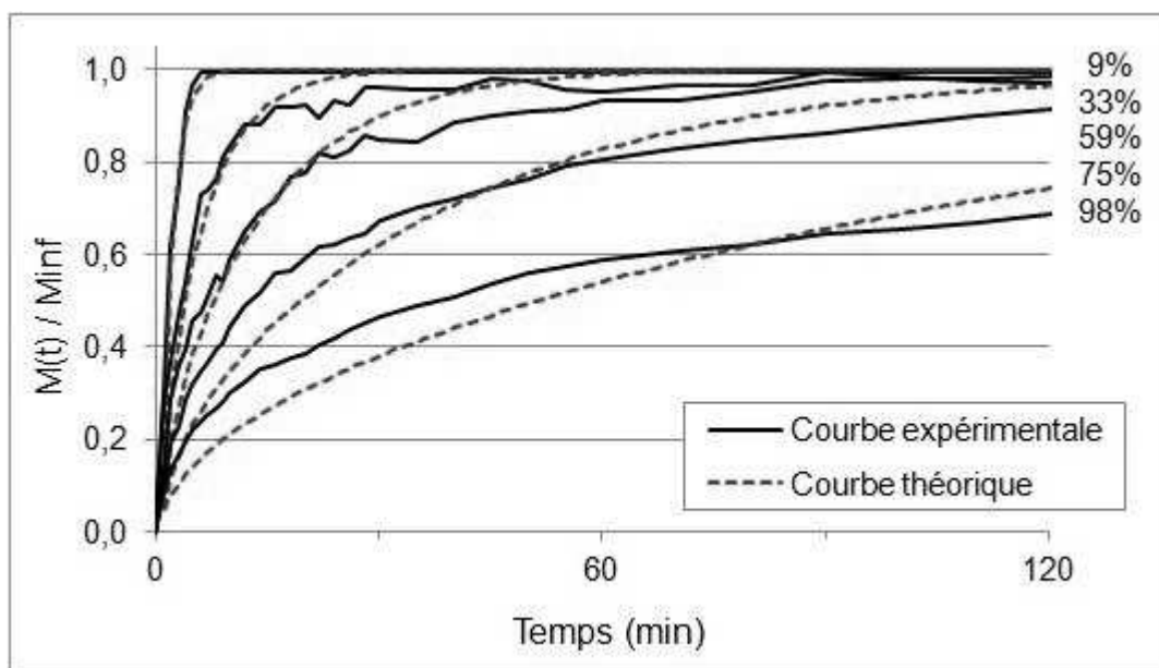
Figure III-27 – Courbe \alpha = M_t/M_\infty en fonction du temps pour le bois fluoré aux diverses humidité relatives
