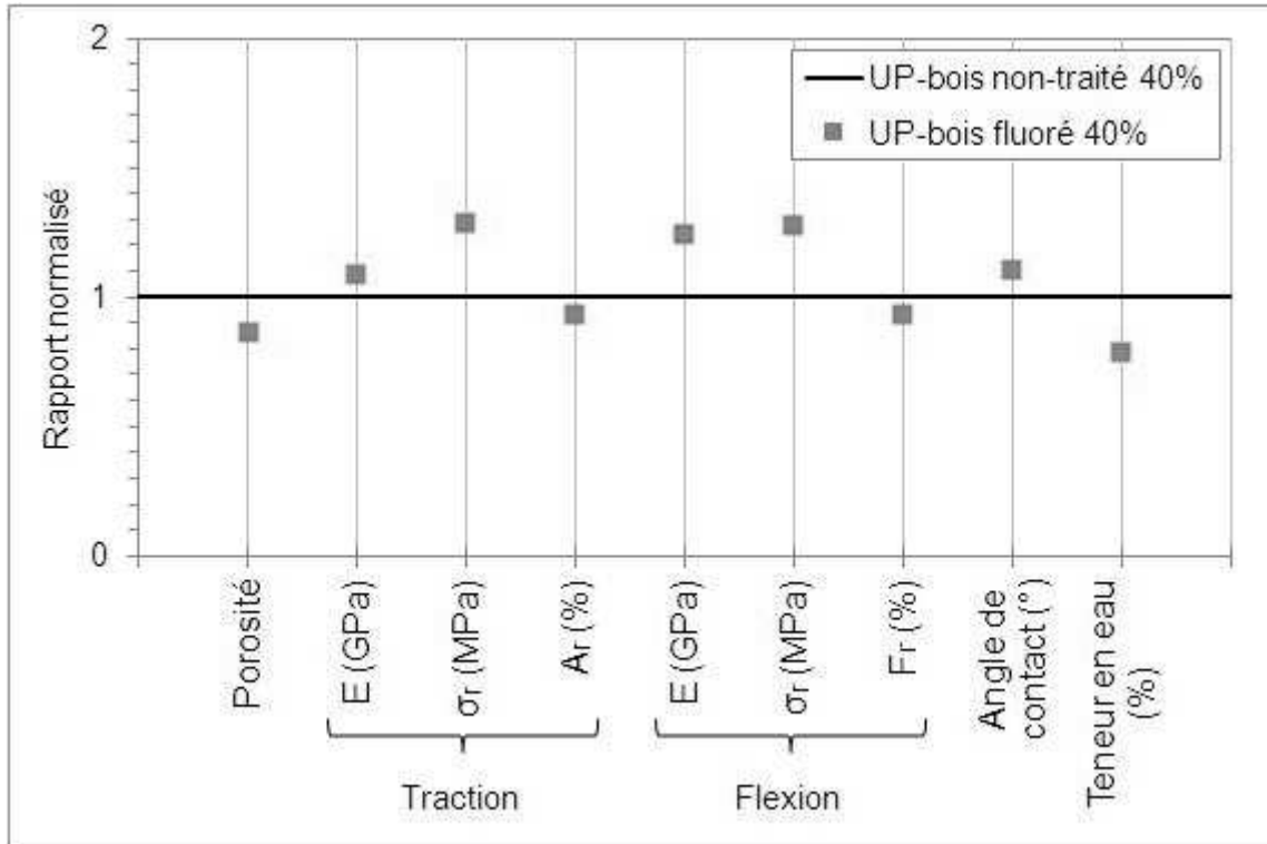
Figure IV-26 – Bilan de l'évolution des propriétés des composites bois-polyester avec la fluoruration des renforts
