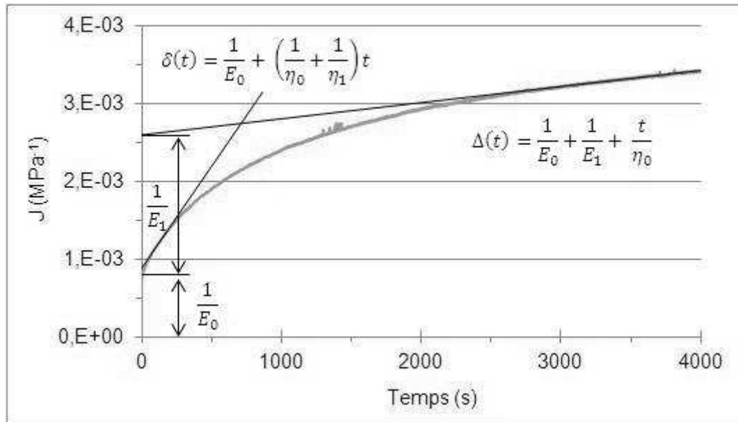
Figure IV-14 – Calcul des caractéristiques du modèle de Burgers et définition des droites \delta(t) et \Delta(t) , exemple du polyester à 45^\circ\text{C}
