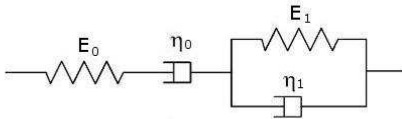
Figure IV-11 – Modèle de fluage de Burgers
