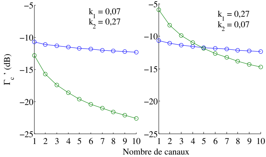
FIGURE 4.9 - Évolution de la limite maximum du GMBO \overline{\Gamma}_c d'un système électroacoustique d'augmentation de couplage selon le nombre de canaux. Condition limite liée à l'instabilité du système ( \circ ); condition limite liée à un facteur de couplage actif supérieur à 1 ( \circ ).
