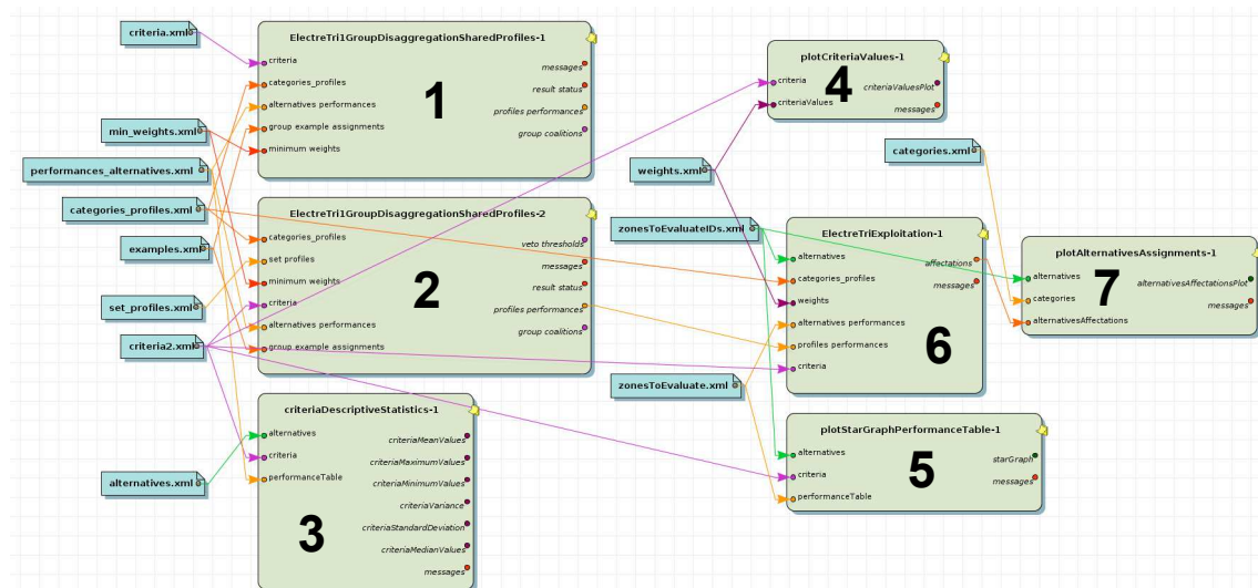
FIGURE 4.2 – Le workflow divisé implémentant le processus de l'exemple illustratif.
