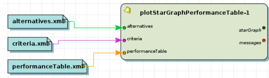
FIGURE 3.17 – La première étape de la construction progressive du workflow diviz supportant le processus d'AMCD.
