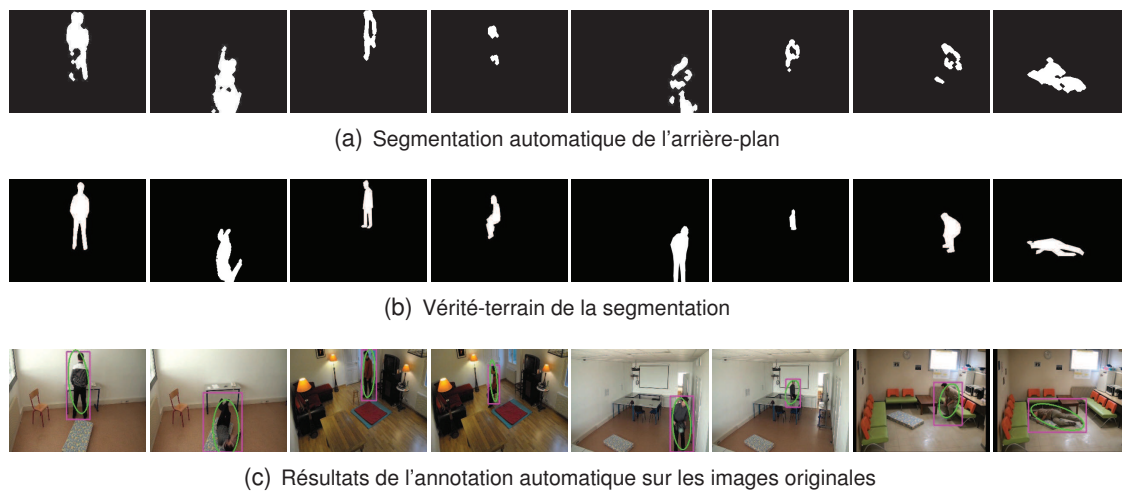
FIGURE 3.5 – Évaluation de l'annotation automatique sur des images de la base DSFD .
