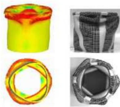
FIGURE 1.5 – Simulations de compression de cylindre réalisées avec Europlexus.
