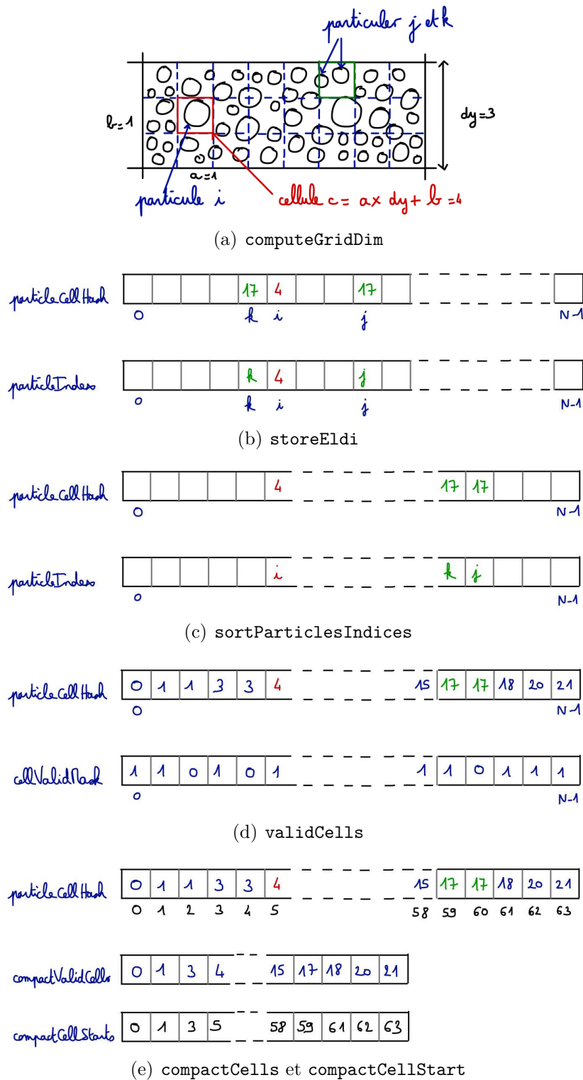
FIGURE 2.10 – Étapes de la détection de collision : calcul des dimensions de la boîte englobante (a), détermination du numéro de cellule de chaque élément (b). Tri des indices et des numéros de cellule dans l'ordre des numéros de cellule (c). Détermination des cellules valides (d). Compactage des cellules et des débuts de cellule valides (e).
