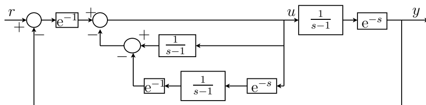
FIGURE 3: Schéma bloc fonctionnel d'un contrôleur stabilisant pour l'Exemple 0.4.
