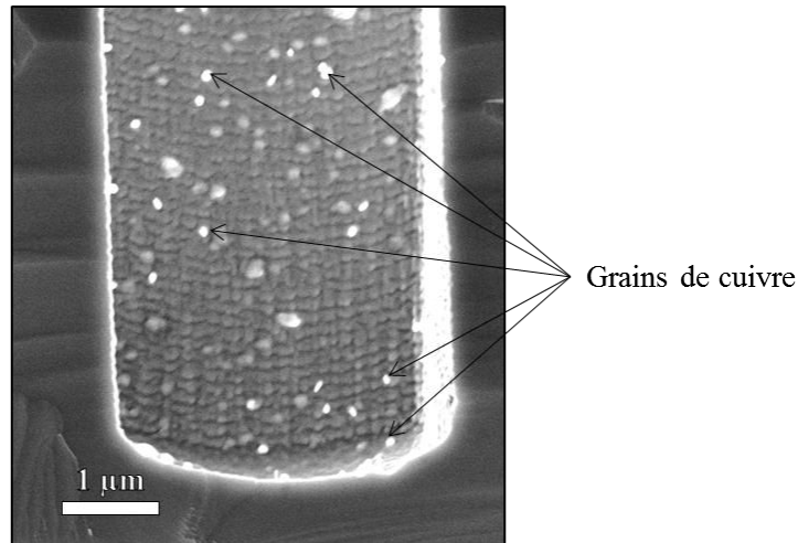
Figure 131 : Dépôt ALD de TaO_xN_y et de cuivre au fond d'un via de 3\ \mu m de large et 20\ \mu m de haut.
