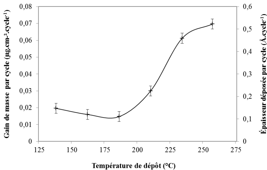
Figure 119 : Gain de masse par cycle mesuré par microgravimétrie lors du dépôt ALD de nitrure tantale à différentes températures.
