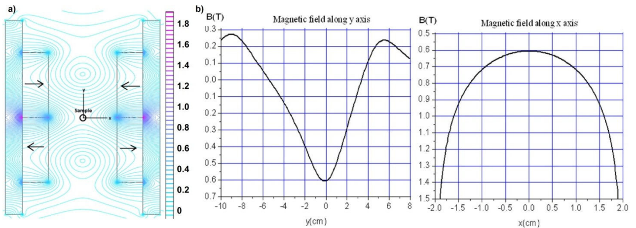
Figure 5.2: Système magnétique: a) isolignes du champ magnétique calculées avec Femm (Meeker 2011); b) distribution du champ magnétique le long de l'axes x et y.
