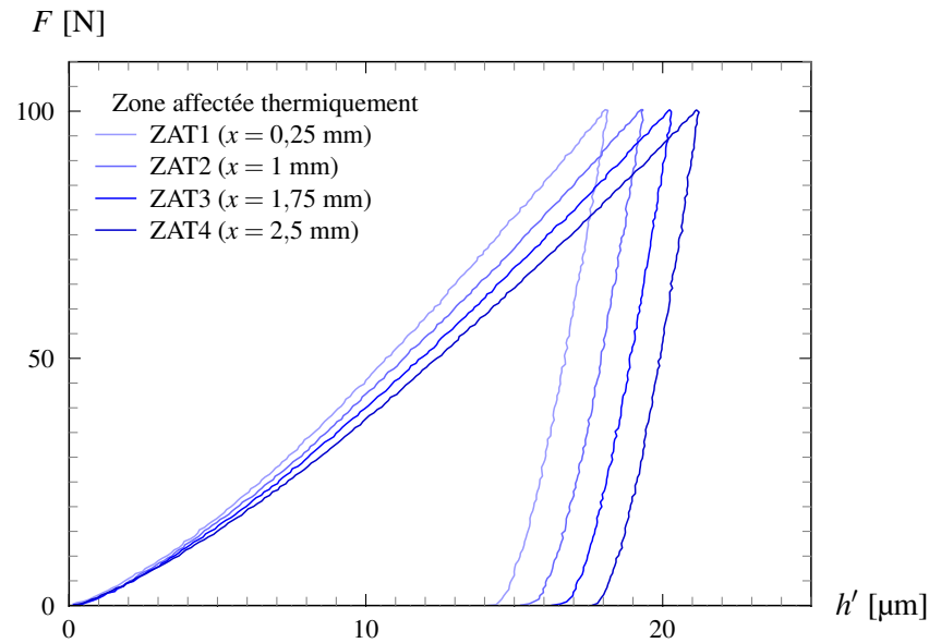
Figure VI.1 : Filiations d'indentations au travers des différentes zones de l'assemblage soudé en croix.
