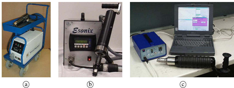
Figure I.26 : Illustrations du Stressonic Needle Peening (a) développé par la Sonats, de l'UIT Esonix (b) de la compagnie Applied Ultrasonics et de l'UltraPeen (c) proposé par Integrity Testing Laboratory.
