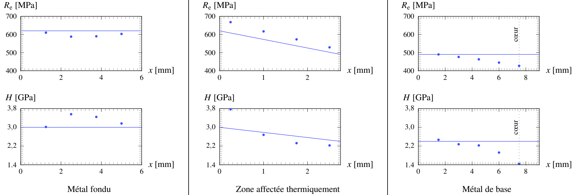
Figure VI.6 : Évolution retenue des caractéristiques mécaniques pour chacune des 3 zones de l'assemblage soudé.
