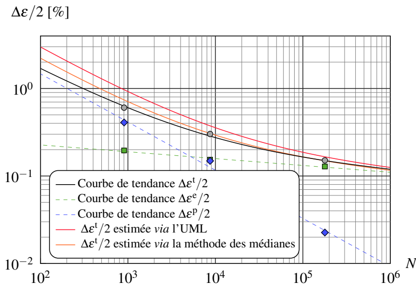
Figure II.8 : Courbes de Manson-Coffin expérimentales et estimées.
