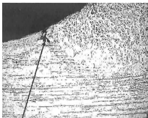
Figure I.49 : Exemple de repli de martelage observé à l'interface entre le métal de base et la zone fondue (Maddox et al. , 2007).
