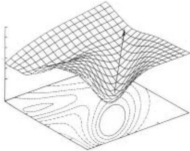
Figure II.6 : Représentation schématique de la surface d'énergie potentielle (PEL).
