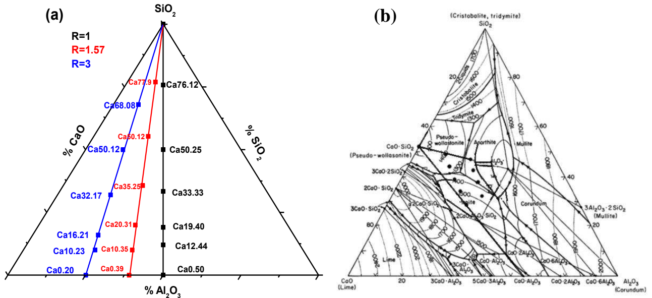
Figure 1.110 : Diagramme de phase expérimental (a), température de fusion T_f (b) pour les aluminosilicates de calcium.
