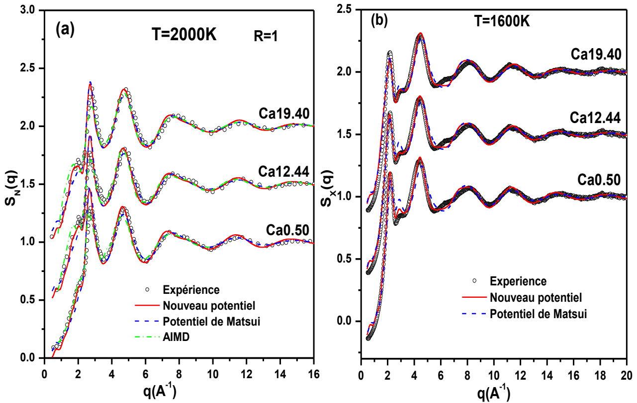
Figure III.3 : Facteur structure total: (a) diffusion de neutrons S_n(q) dans le liquide à T = 2000 \text{ K} , et (b) diffraction de rayons X S_x(q) en surfondu à T = 1600 \text{ K} pour les compositions Ca0.50, Ca12.44 et Ca19.40.
