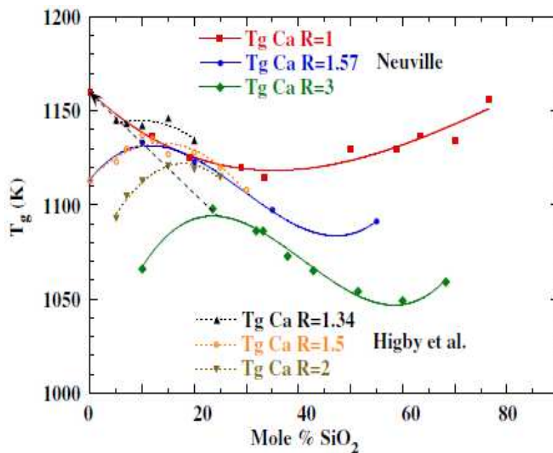
Figure 1.11: Température de transition vitreuse expérimentale T_G des verres CAS [Cormier & al., 2005].
