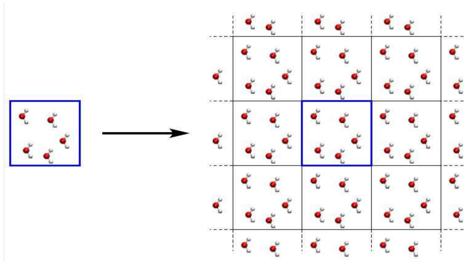
Figure II.1 : Schéma en deux dimensions représentant les conditions aux limites périodiques d'une boîte cubique. La boîte de simulation est encadrée en bleu, elle est entourée de ses images.
