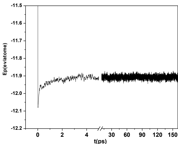
Figure II.3 : la fluctuation de l'énergie potentielle pour la composition Ca_{12.44} à T = 3000 K. L'axe x est interrompu à 5 ps et montre aux temps courts la configuration hors équilibre et à partir de 10 ps la configuration en équilibre : l'énergie potentielle fluctue autour d'une valeur moyenne de -11,903 eV/atome.
