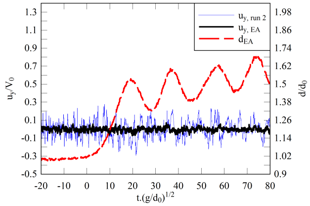
(d) Transversal velocity at z/d_0 = 0.29
