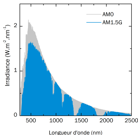
FIGURE 1.1 – Spectres AM0 (extra-terrestre) et AM1.5G (référence terrestre) du rayonnement solaire.
