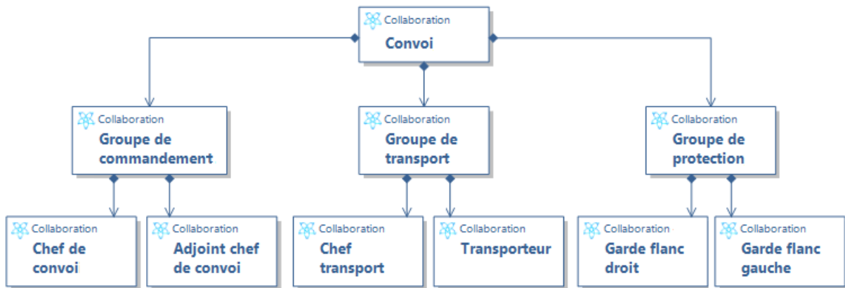
Figure 12 – Application des concepts de la vue "Roles & Collaboration" sur le modèle du convoi (1)
