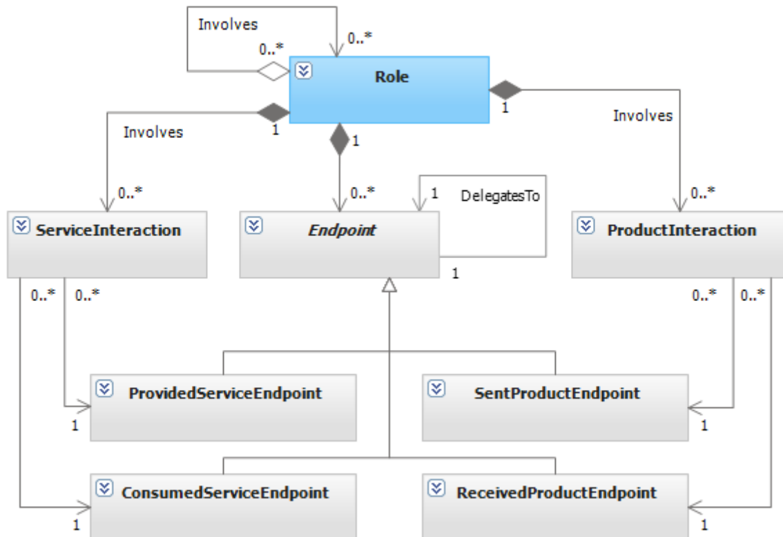
Figure 11 - DSL IDEA : principaux concepts et relations de la vue ROLES & COLLABORATIONS
