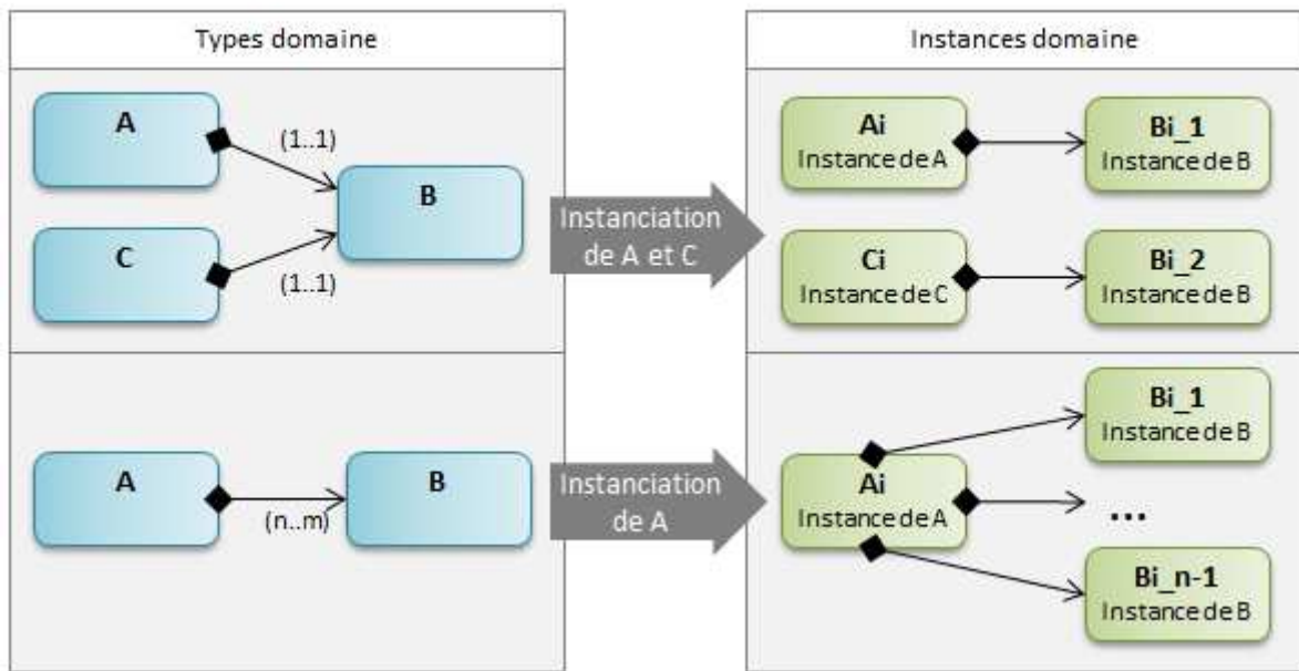
Figure 20 - Principes de l'instanciation des relations hiérarchiques
