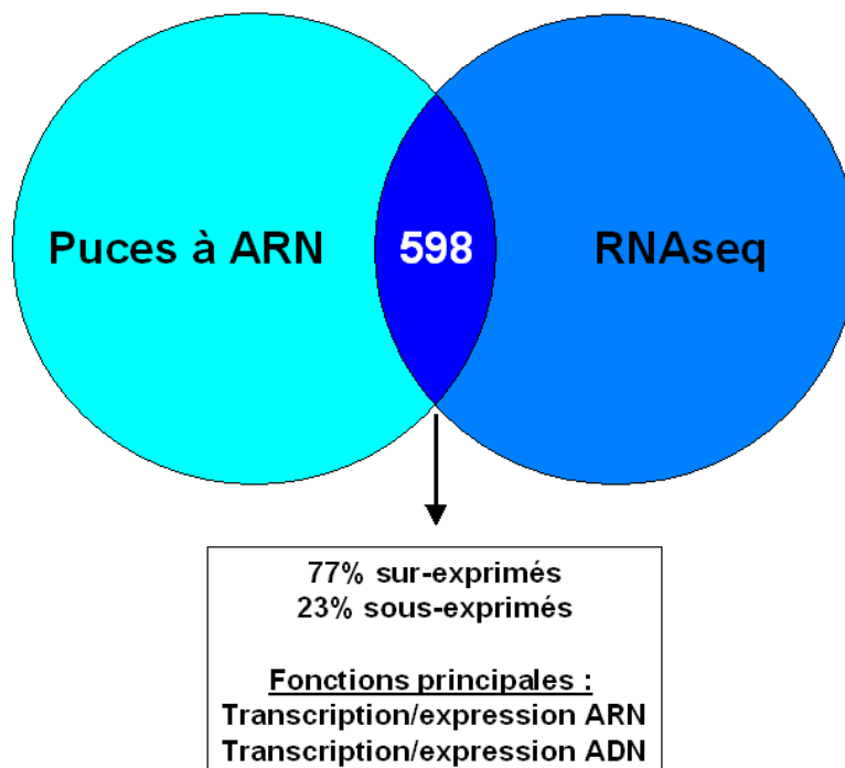
Figure 28 : Recoupement des résultats des analyses sur puces à ARN et de RNAseq et fonctions principales des gènes retrouvés dans les deux analyses.
