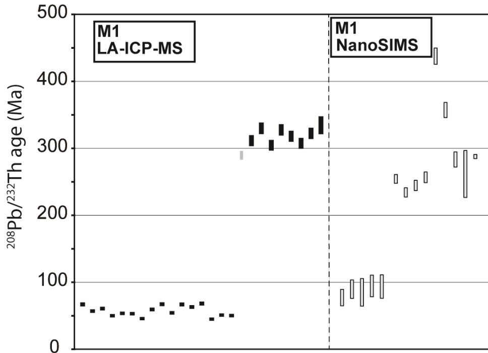
Figure 5-10 : Comparaison entre les âges du domaine M1 mesurés à la NanoSIMS et au LA-ICP-MS. La barre d'erreur correspond à 2\sigma .
