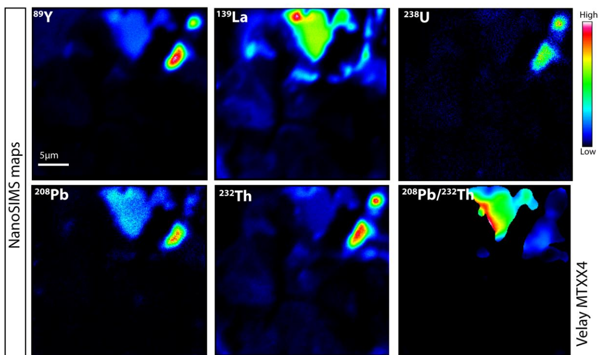
Figure 5-12 : Cartographies réalisées à la NanoSIMS de la monazite MTXX4 du massif du Velay (cf chapitre 3).
