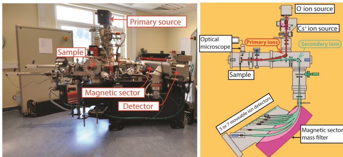
Figure 5-4 : Photographie à gauche et schéma à droite d'une NanoSIMS CAMECA NS50. Le faisceau primaire Cs^+ ou O^- (en rouge) est focalisé sur l'échantillon qu'il bombarde. Les ions secondaires résultants (en vert) sont accélérés dans un champ électrostatique et magnétique, séparés en fonction de leur énergie et rapport masse/charge, puis détectés en multi-collection.
