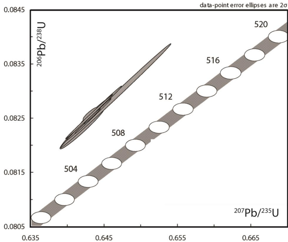
Figure 2-13: Diagramme concordia ^{206}\text{Pb}/^{238}\text{U} vs ^{207}\text{Pb}/^{235}\text{U} dans lequel sont reportées les analyses ID-TIMS de la monazite Moacyr (Gasquet et al., 2010).
