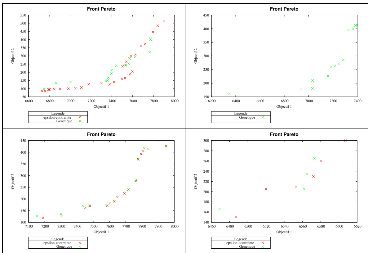
Fig. 5.8 – Représentation du front de Pareto : instance à 15%.
