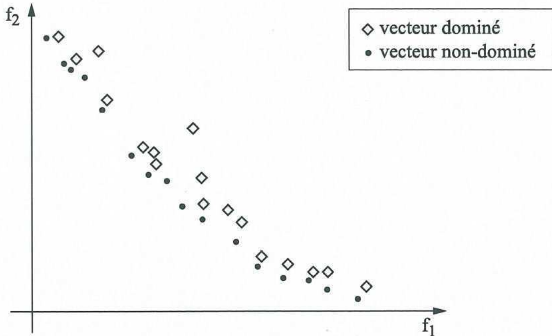
Fig. 4.3 – Représentation de vecteurs dominés et non dominés.
