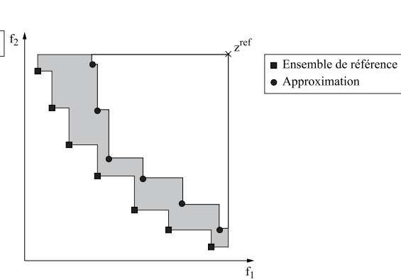
Fig. 4.5 – Indi. d’hypervolume-diff. I_H^- .
