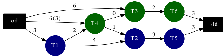
Fig. 2.5 – Exemple de réseau avec des tarifs optimaux négatifs.
