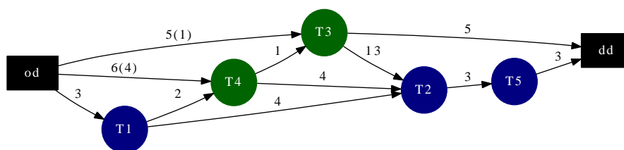
Fig. 2.6 – Réseau illustrant la forme de la fonction objectif du meneur.
