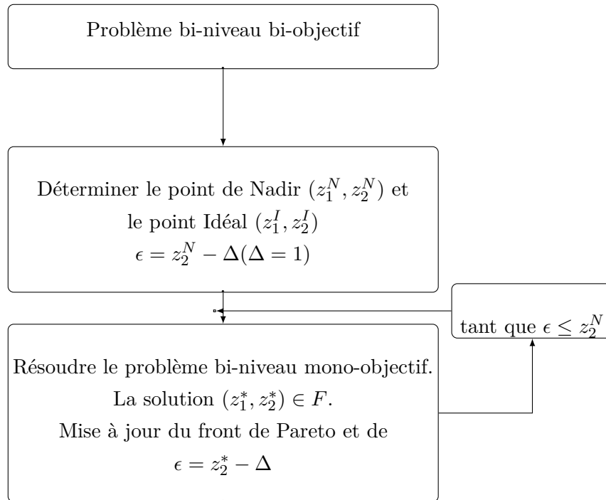
Fig. 5.3 – Méthode du \epsilon -contrainte pour le POBB.
