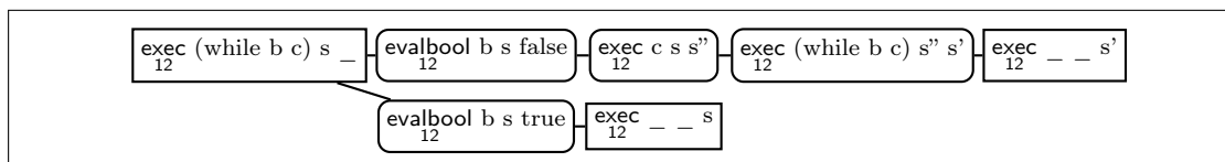
FIGURE 5.9 – Reltree résultant de l'insertion de exec_while1 dans rt_1
