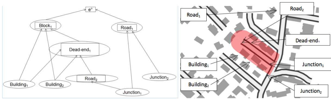
FIGURE 4.5 – Graphe mixte représentant les agents cartographiques et leurs environnements, détectés automatiquement pour une impasse ( dead-end ). L'impasse est placée dans un îlot ( block ) et héberge des bâtiments et une route. Cette route est elle-même en intersection avec la route principale qui borde l'îlot (emprunté à MAUDET et al. [7]).
