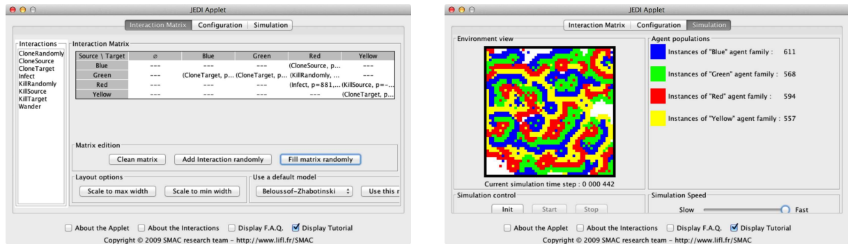
FIGURE 2.9 – L'applet de démonstration de JEDI, dans laquelle on peut interactivement construire une matrice d'interaction à partir des agents et des interactions existantes (à gauche) et en visualiser immédiatement le résultat dans la simulation (à droite).
