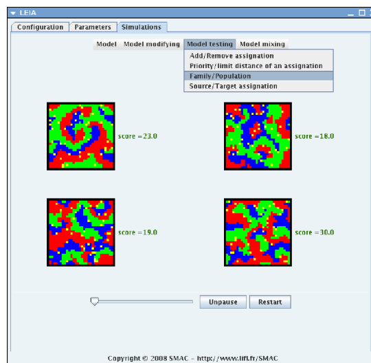
FIGURE 2.10 – Une vue du navigateur LEIA, avec ici quatre simulations lancées en parallèle. L'utilisateur peut choisir un mode de sélection automatique ou interactif, et définir ses propres critères d'évaluation en plus ou à la place des critères intrinsèques prédéfinis.
