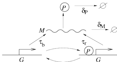
FIGURE 3.2 – Modèle le plus simple : gène réprimé par sa propre protéine. Le gène G à l'état non régulé (à gauche) est transcrit sous forme d'ARN messager ( M ) à un taux supposé constant au cours du temps ( \tau_b ). M est à son tour traduit en protéine ( P ). M et P subissent une dégradation exponentielle au cours du temps (resp. \delta_M et \delta_P ). La protéine P peut se fixer sur un site régulateur de G et réprimer sa transcription (à droite) : G est alors transcrit à un taux \tau_r \ll \tau_b — cf. [30].
