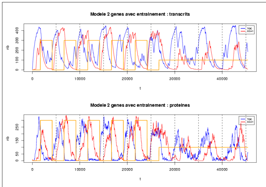
FIGURE 3.6 – Résultats typiques de la simulation à 2 gènes : en haut, courbe des ARNm de TOC et CCA ; en bas, courbe des protéines. La cellule est entraînée d’abord par un signal lumineux carré ( T = 5000 pas) puis on passe en lumière continue. Ici on a \delta_{MA} = \delta_{MB} = 1,5 \cdot 10^{-3} , ce qui équivaut à une demi-vie des ARNm d’un peu plus de 2 h (compatible avec la littérature). À noter : le déphasage progressif en jour continu, le système retournant à sa période libre légèrement supérieure à 24 h.
