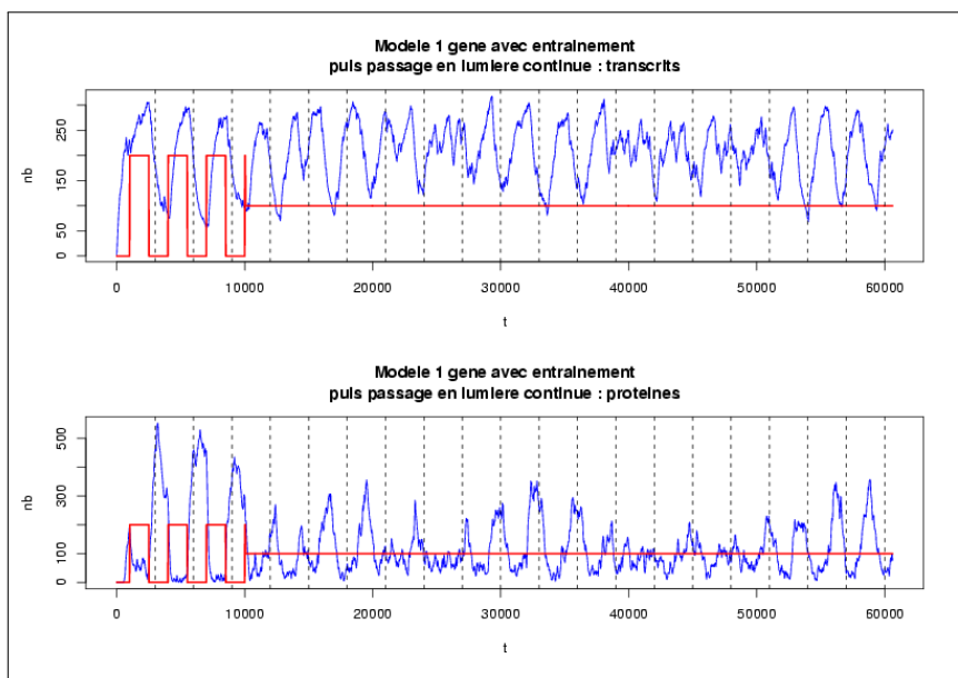
FIGURE 3.5 – Résultats obtenus dans le modèle multi-agents à 1 gène avec l’introduction d’un signal lumineux carré suivi d’un signal lumineux continu. Les pointillés verticaux indiquent la période de forçage.
