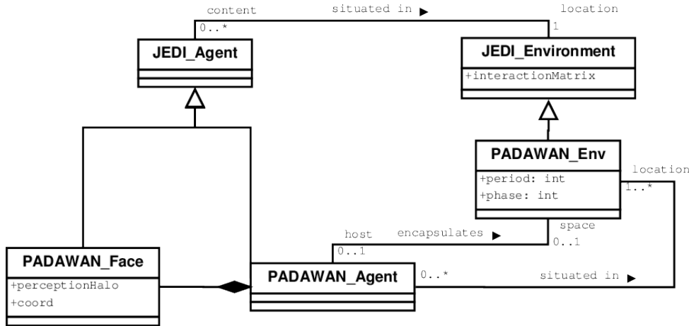
FIGURE 4.2 – Diagramme des classes montrant l’implémentation effective de PADAWAN au sein de la plateforme JEDI. Le modèle conceptuel manipule un agent « monolithique » ( PADAWAN_Agent ) qui est automatiquement décomposé dans la plateforme en un noyau non situé et une collection d’agents faces ( PADAWAN_Face ) situés chacun dans un environnement unique, bénéficiant ainsi du même fonctionnement que des agents JEDI classiques.
