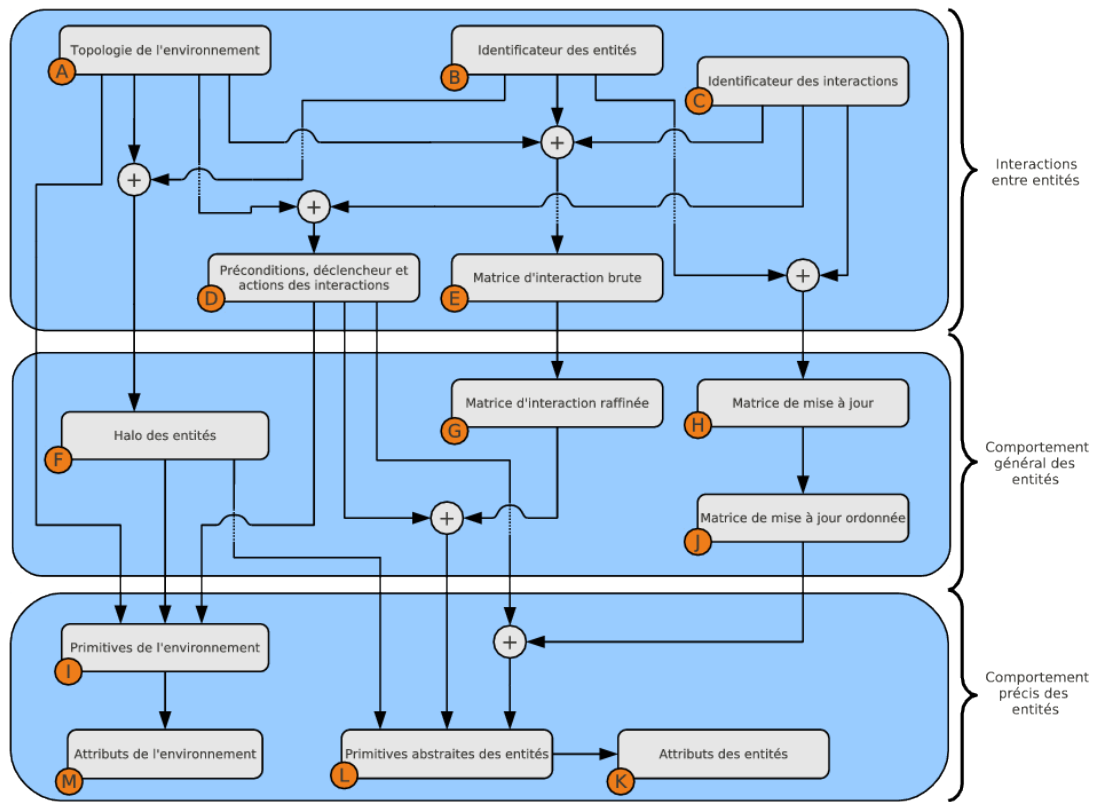
FIGURE 2.4 – Étapes de conception et d'implémentation d'un modèle avec IODA. Une assez grande souplesse est laissée au concepteur dans une approche descendante qui raffine et détaille pas à pas les divers points clefs (emprunté à KUBERA [134]).
