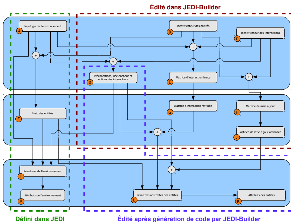
FIGURE 2.8 – Répartition des tâches entre JEDI, JEDI-Builder et le développeur lors de l'utilisation de JEDI-Builder pour l'implémentation d'un modèle IODA (emprunté à KUBERA [134]).
