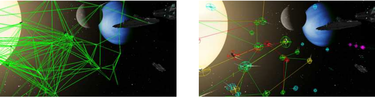
FIGURE 3.12 – Deux vues augmentées de la simulation GALAXIAN : à gauche, les traits représentent les relations de perception entre agents ; à droite, la couleur des sphères autour des agents code l’interaction qu’ils effectuent et le trait les relie à leur cible.
