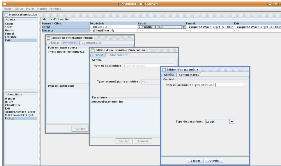
FIGURE 2.7 – Vue de l'IDE JEDI-Builder (emprunté à KUBERA [134]).
