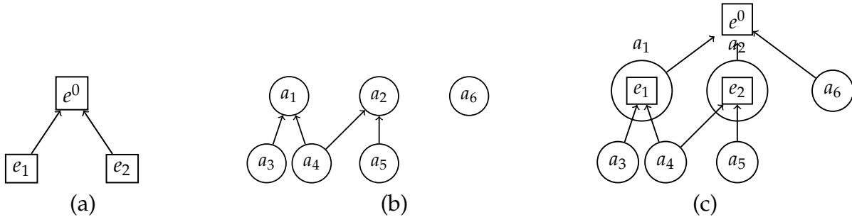
FIGURE 4.1 – (a) Graphes d’inclusion (resp. (b) d’hébergement, et (c) mixte) correspondant à l’exemple décrit dans le texte (p. 76). Par convention les agents sont représentés par des cercles, les environnements par des carrés. La superposition cercle/carré (c) correspond à l’encapsulation d’un environnement par un agent ( \sim ). Les arcs représentent respectivement la relation \subset (a), la relation \sqsubset (b), et la relation \triangleleft (c).
