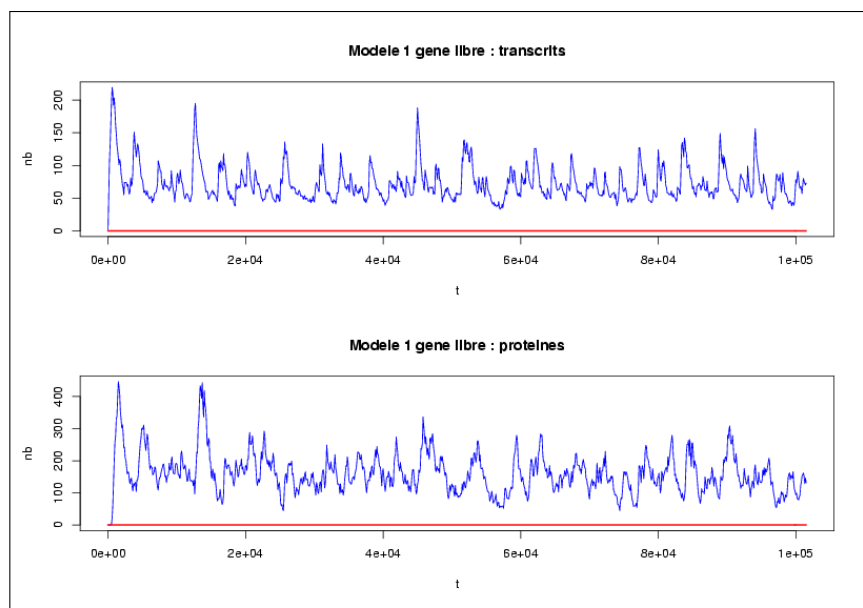
FIGURE 3.4 – Résultats typiques de la simulation à 1 gène du modèle multi-agents, en l’absence de tout signal lumineux : en haut, courbe de l’ARNm ; en bas, celle des protéines. Axe des abscisses : nombre de pas de temps de simulation.
