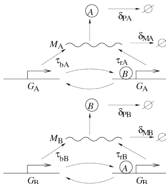
FIGURE 3.3 – Modèle à deux gènes, avec régulation croisée : les protéines A et B , produites respectivement par transcription et traduction des gènes G_A et G_B , régulent la transcription respective de B et A . Il peut s'agir d'une activation ou d'une répression.
