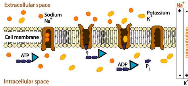
FIGURE 4.3 – Principe de la pompe \text{Na}^+/\text{K}^+ : la pompe est une protéine membranaire. Quand elle est ouverte vers l'intérieur de la cellule, elle peut capter 3 ions sodium \text{Na}^+ . Une molécule d'ATP peut alors phosphoryler la pompe : sa conformation spatiale change et elle libère les ions sodium hors de la cellule. Dès lors, elle peut capter 2 ions potassium \text{K}^+ , ce qui provoque sa déphosphorylation : elle reprend sa première conformation et libère les ions potassium à l'intérieur de la cellule. (Source de l'image : Wikimedia Commons)
