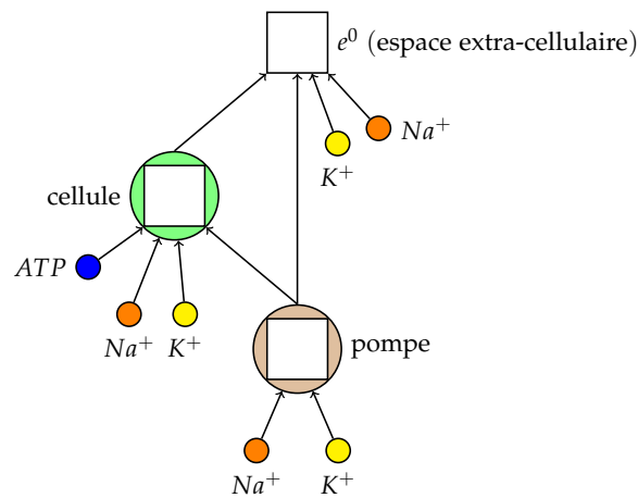
FIGURE 4.4 – Graphe mixte (environnements et agents) correspondant à la modélisation multi-niveaux de la pompe sodium-potassium. Par souci de simplification, un seul agent de chaque famille a été représenté dans chaque environnement (en pratique bien sûr il peut y avoir plusieurs ions sodium dans la cellule, dans la pompe ou à l'extérieur, ou même plusieurs cellules chacune dotée de plusieurs pompes, etc.)
