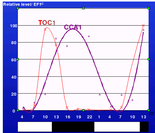
FIGURE 3.1 – Données expérimentales du groupe Horloge circadienne et cycle cellulaire de l'Observatoire océanologique de Banyuls, donnant les niveaux d'expression (quantité normalisée d'ARNm) de deux gènes d' O. tauri (TOC et CCA) en fonction du temps circadien (ZT), mesurés en alternance jour/nuit (bandes blanches et noires).
