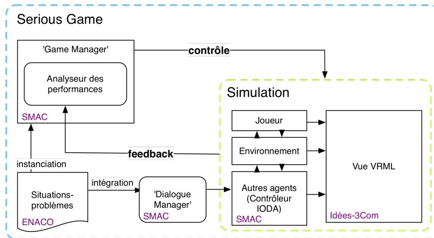
FIGURE 3.8 – L’architecture logicielle de FORMAT-STORE. Pour la partie simulation, l’animation 3D a été assurée par Idées-3Com ; les intervenants de l’équipe SMAC ont géré toute la partie comportementale, ainsi que l’intégration des dialogues correspondant aux situations-problèmes identifiées par les experts, et le contrôle adaptatif de la difficulté du jeu (source : David Panzoli — rapport interne).
