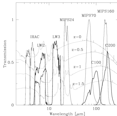
FIGURE 1.10 – Transmissions des filtres chromatiques installés sur les télescope spatiaux Spitzer et ISO . [figure extraite de Fadda et al. (2004)].
