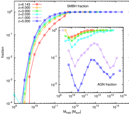
FIGURE 4.28 – Apparition de la population de trou noir super-massif et évolution de la population active. Le cadran principal présente, en fonction de la masse du halo de matière noire et de l'époque (code couleur), la fraction en nombre d'objets, abritant un trou noir super-massif au centre de la galaxie formée en son cœur. Comme attendu, plus la structure est massive, et donc évoluée, et plus la fraction de trou noir super-massif est élevée. Elle tend vers 1 pour les halos de masse M_h > 10^{12} M_\odot . La fenêtre intérieure reporte la fraction en nombre de trous noirs actifs ( L_{bol,AGN} > 0.01L_{Edd} ). Cette fraction très élevée à haut redshift décroît progressivement avec le temps et la masse, signe de l'arrêt de l'accrétion.
