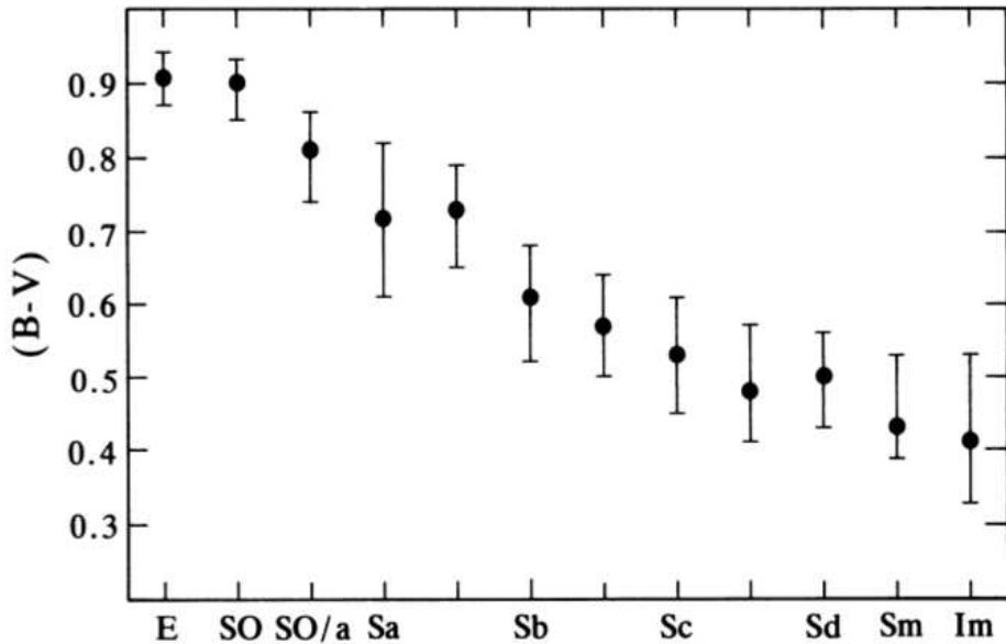
FIGURE 1.24 – Relation entre couleur (b-v) et type morphologique. On constate une nette évolution. Les galaxies de type morphologique elliptique (E) sont caractérisées par une forte couleur rouge ( b - v \simeq 0.9 ). La transition vers les galaxies spirales (S) par l'intermédiaire des galaxies lenticulaires (SO) s'accompagne d'une diminution progressive et constante de la couleur moyenne. Au sein des galaxies dites spirales, la couleur est d'autant plus faible ( (b-v) : 0.7 \rightarrow 0.5 ), la galaxie d'autant plus bleue) que les bras spiraux sont peu nombreux et marqués (Sa \rightarrow Sd). Les galaxies les plus bleues identifiées dans cette étude sont des structures irrégulières ne figurant pas, par définition, dans la célèbre séquence de Hubble. [Figure extraite de Roberts & Haynes (1994)].
