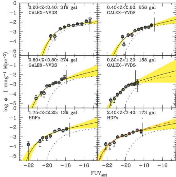
FIGURE 1.33 – Fonction de luminosité rest-frame UV. Construites par Arnouts et al. (2005) à partir de données issues du satellite GALEX , ces distributions sont données pour différents décalages spectraux compris entre 0.2 < z < 3.4 . Les symboles sont issus de mesures directes via l'utilisation de différents estimateurs (e.g. V_{\text{max}} , Ilbert et al. (2004)). La courbe continue noire associée à la zone colorée jaune sont respectivement le meilleur ajustement et la zone d'erreur à 1\sigma . La courbe pointillée noire correspond à une distribution de référence, mesurée localement ( z \simeq 0 ) par Wyder et al. (2005). L'augmentation de la luminosité et l'émergence de galaxies très brillantes pour des redshift z > 0.5 est clairement visible. [Figure extrait de Arnouts et al. (2005)].
