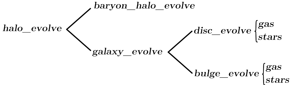
FIGURE 5.1 – Structuration hiérarchique des appels aux procédures élémentaires d'évolution. Chaque procédure s'applique au niveau de structuration caractéristique de la composante à laquelle elle est associée. Alors que les procédures disc_evolve et bulge_evolve permettent de faire progresser l'évolution des contenus, respectivement en gaz et en étoiles du disque et du bulbe, les échanges entre ces deux composantes sont traités par la procédure halo_evolve
