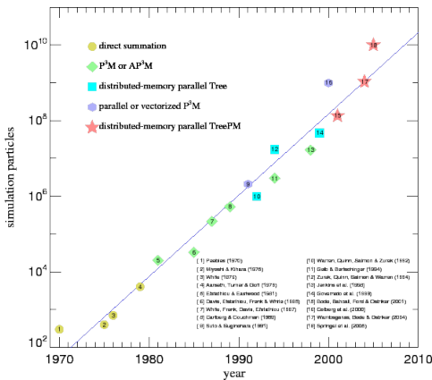
FIGURE 2.8 – Evolution du nombre de particules utilisées dans les simulation N-corps depuis les années 70. Alors que les premières simulations n'utilisaient que quelques centaines de particules, les modélisations actuelles en regroupent plusieurs milliards N_p \simeq 10^{10} . Cette augmentation s'est faite en partie grâce au développement d'algorithmes optimisés (Barnes & Hut, 1986) mais également par l'émergence de machines de calcul dédiées et fortement parallélisées.
