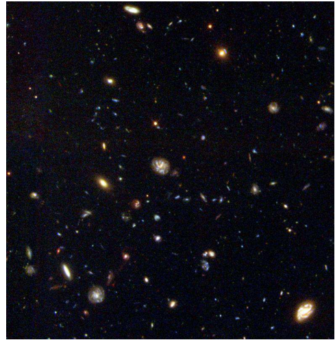
FIGURE 1.7 – Image du Hubble Deep Field South réalisé par le télescope spatial Hubble en septembre et octobre 1998 dans la région du Toucan.
