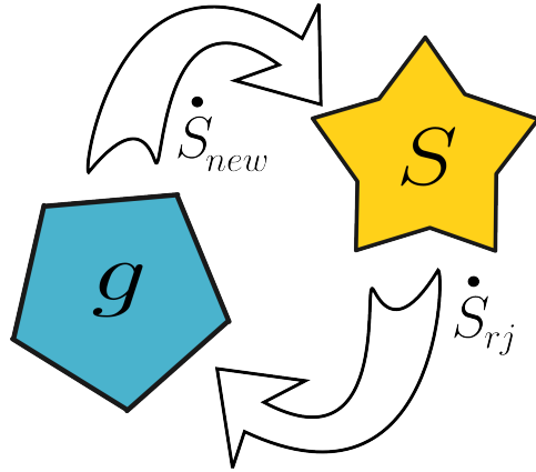
FIGURE 4.22 – Schéma des échanges existants entre une population stellaire \mathcal{S} et le gaz du milieu interstellaire g . Les étoiles sont formées à partir du gaz à un taux \dot{S}_{new} . Les étoiles constituant la population ré-injectent alors progressivement du gaz enrichi en métaux à un rythme \dot{S}_{rj} .
