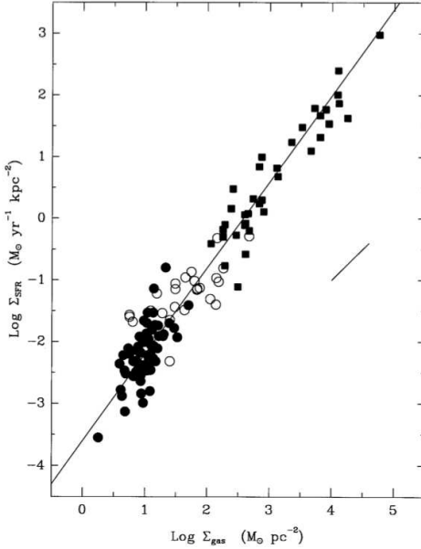
FIGURE 4.21 – Relation de Schimdt-Kennicutt extraite des travaux de Kennicutt (1998b). Les différents points correspondent à différentes mesures effectuées sur un échantillon de galaxies formant des étoiles. Les cercles et carrés pleins indiquent respectivement une galaxie à disque et une galaxie à flambée de formation stellaire. Les symboles vides marquent une mesure effectuée au centre des galaxies à disque. Le meilleur ajustement donné en Eq. 4.47 traduit une relation fonctionnelle, sur plus de trois ordres de grandeur, en densité surfacique de gaz.
