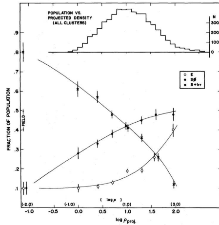
FIGURE 1.27 – Fraction de galaxies en fonction de leur morphologie et de la densité d'objets caractéristique de l'environnement au sein duquel elles évoluent. On constate une forte augmentation de la fraction de galaxies elliptiques dans les environnements denses. A contrario les galaxies spirales dominent les environnements peu denses, elle sont alors qualifiées de galaxies de champs. [figure extraite de Dressler (1980b)].
