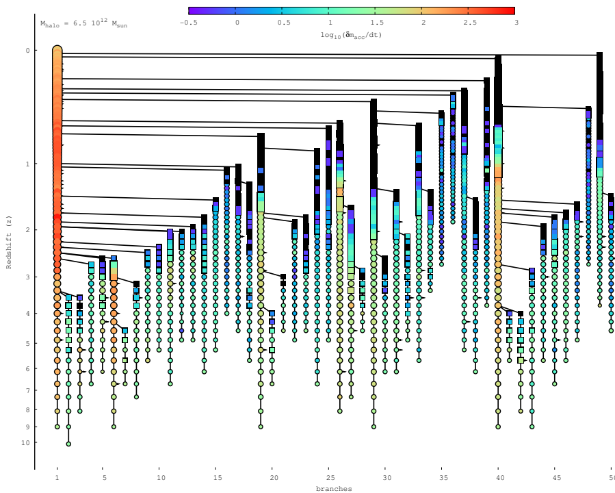
FIGURE 3.4 – Arbre de fusion extrait de la simulation de matière noire. Comme pour la figure 3.1, seules les cinquante branches les plus massives et donc celles contribuant le plus à l’assemblage en masse de la structure principale (branche 1) sont représentées. Les branches portant l’évolution de structures moins massives, devant se connecter à celles représentées, sont indiquées par des embryons (têtes de flèches). De même, les deux types de symboles différencient les halos (ronds) des sous-halos (carrés). La taille du symbole est proportionnelle à la masse du Viriel ( M_{vir} ) de la structure. Le code couleur, référencé par la plage supérieure et restreint aux valeurs extrêmes constatées sur l’ensemble de l’arbre, est dédié ici au taux d’accrétion de matière noire mesuré sur chaque structure. Il est calculé comme étant la masse apportée par l’ensemble des particules identifiées en tant qu’accrétion diffuse, \delta m_{acc} (Eq. 3.13), laquelle est divisée par l’intervalle de temps principal ( dt ) séparant deux instantanés successifs extraits de la simulation N-corps. Une colorisation noire indique une absence d’accrétion diffuse. Deux tendances sont alors identifiables : i) Pour les halos, l’accrétion diffuse est d’autant plus importante que le halo est massif ; ii) Les sous-structures présentent quant à elles un fort déficit en accrétion. Ceci s’explique par le simple fait suivant : ces structures, étant immergées au sein d’une structure plus massive, elles en forment des sur-densités locales, l’accrétion diffuse provenant de l’extérieur est donc naturellement reçue en priorité par la structure principale. On constate également que, lors de phases de survol ( fly-by : branche 18), les sous-halos voient leur accrétion diminuer lors de l’immersion puis ré-augmenter suite à leur sortie.
