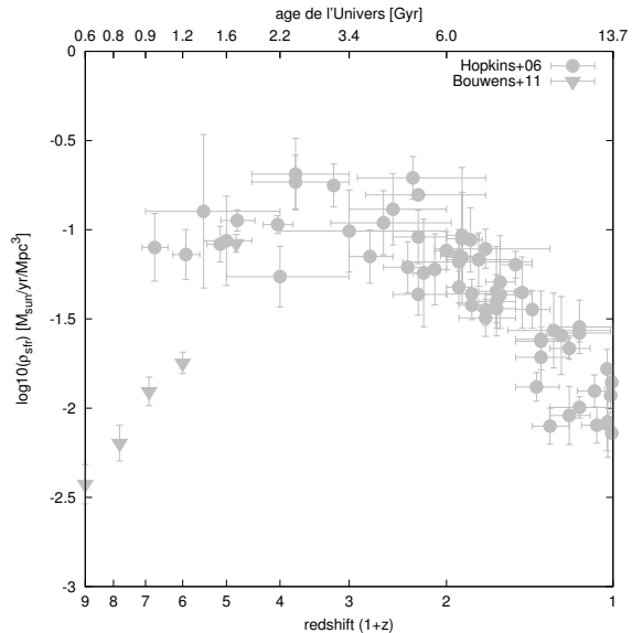
FIGURE 1.31 – Ensemble de mesures, en fonction du temps, normalisé pour un volume comobile d'Univers de 1Mpc^3 , du taux moyen de formation stellaire \rho_{sfr} . Sont reportés, le décalage spectral (redshift : 1+z ) et l'âge de l'Univers en abscisses basse et haute respectivement. Les données représentées ici sont issues des travaux de Hopkins & Beacom (2006), regroupant un grand nombre d'études dédiées à ces mesures. Les points à plus grand décalage spectral, ( z > 6 ), sont extraits de Bouwens et al. (2011). Ces mesures, exprimées dans la convention d'IMF de Chabrier (2003), mettent en avant un pic de formation stellaire entre les redshifts z \in [1 - 3] .
