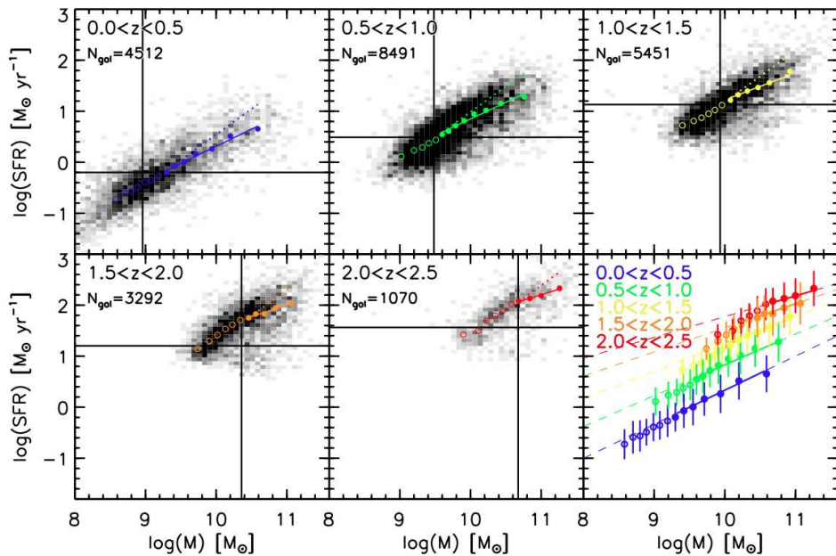
FIGURE 1.36 – Evolution avec le redshift de la relation M_* - SFR . Les trois cadrans supérieur ainsi que les deux cadrans gauches inférieurs, présentent la distribution des 22 816 galaxies observées par le programme NMBS (Whitaker et al., 2011) et sélectionnées dans différents intervalles de redshift ( 0.0 < z < 2.5 ). Les deux droites, verticale et horizontale, marquent les limites en complétude des deux grandeurs indiquées. Dans le cadran inférieur droit sont reportées les relations moyennes ainsi que les déviations standard de chacune d'elles. On constate une nette progression de l'efficacité de la formation stellaire avec le temps, le niveau moyen de la distribution ne faisant que croître avec le redshift. [Figure extraite de Whitaker et al. (2012)].
