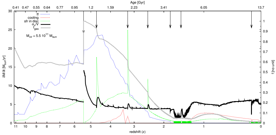
FIGURE 4.15 – Est présentée ici, par la courbe noire, l'évolution du rapport \sigma_V/V pour un disque hébergé par un halo de masse M_{vir} \simeq 5 \times 10^{11} M_\odot à z = 0 . Les flèches verticales indiquent les évènements de fusion. Sont ajoutés : le taux d'accrétion issu de la phase froide (courbe pointillée bleue), le taux de condensation de la phase chaude (courbe pointillée rouge), ainsi que le taux de formation stellaire dans le disque (courbe pointillée verte). Les valeurs correspondantes sont reportées sur l'axe des ordonnées de droite [ M_\odot \cdot \text{an}^{-1} ]. En parallèle, la courbe grise indique la fraction de gaz dans le disque, la valeur étant reportée, comme pour le rapport \sigma_V/V , sur l'axe des ordonnées de gauche. On constate, pour le rapport \sigma_V/V , une évolution continue et stable parsemée de modifications violentes. La première, liée à une fusion majeure, s'explique par la destruction du disque pré-existant. Un nouveau disque, de petite taille, intégralement constitué de gaz ( f_{gas} = 1 ), se forme suite à la forte accrétion de gaz froid. La croissance en masse et taille du disque de gaz s'accompagne d'un retour à de plus faibles valeurs pour le rapport \sigma_V/V . Plusieurs autres variations sont identifiables. Même si elles sont également liées à des fusions, ces dernières étant mineures, le disque est conservé (Sect. 4.4.4). Dans ces disques, et en lien avec les processus de compression du gaz associés aux fusions, des épisodes de flambées de formation d'étoiles sont générés. Les étoiles les plus massives, formées lors de ces épisodes finissent rapidement leur vie en supernovae. Ces dernières redistribuent une partie de leur énergie cinétique dans le milieu interstellaire (Eq. 4.25) faisant ainsi augmenter le rapport \sigma_V/V . Ce dernier décroît et se stabilise par la suite en raison de la dissipation ( f_{disp} \simeq 0.05 ).
