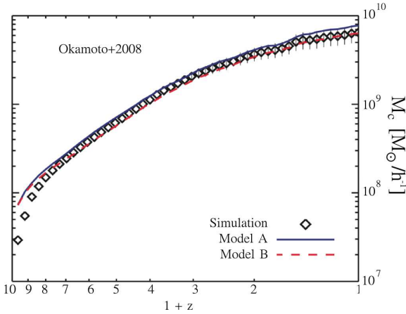
FIGURE 4.4 – Evolution avec le redshift z de la masse de filtrage. Un halo évoluant au redshift z et ayant une masse M_c(z) ne peut maintenir captif qu’une fraction \langle f_b \rangle / 2 des baryons l’environnant. On constate que cette masse croît lorsque le redshift diminue. Cette évolution est due à l’augmentation progressive de la température du milieu intergalactique. De ce fait, les structures pouvant maintenir captif au minimum \langle f_b \rangle / 2 , doivent être, au cours du temps, de plus en plus massives. [Figure extraite de Okamoto et al. (2008)]
