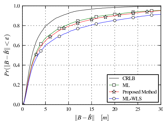
Fig. 7.13: CDF d'erreur de position avec 2 nœuds aidants.
