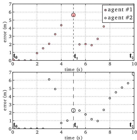
Fig. 7.21: Erreur d'estimation de la position pour les 2 agents en fonction du temps.
