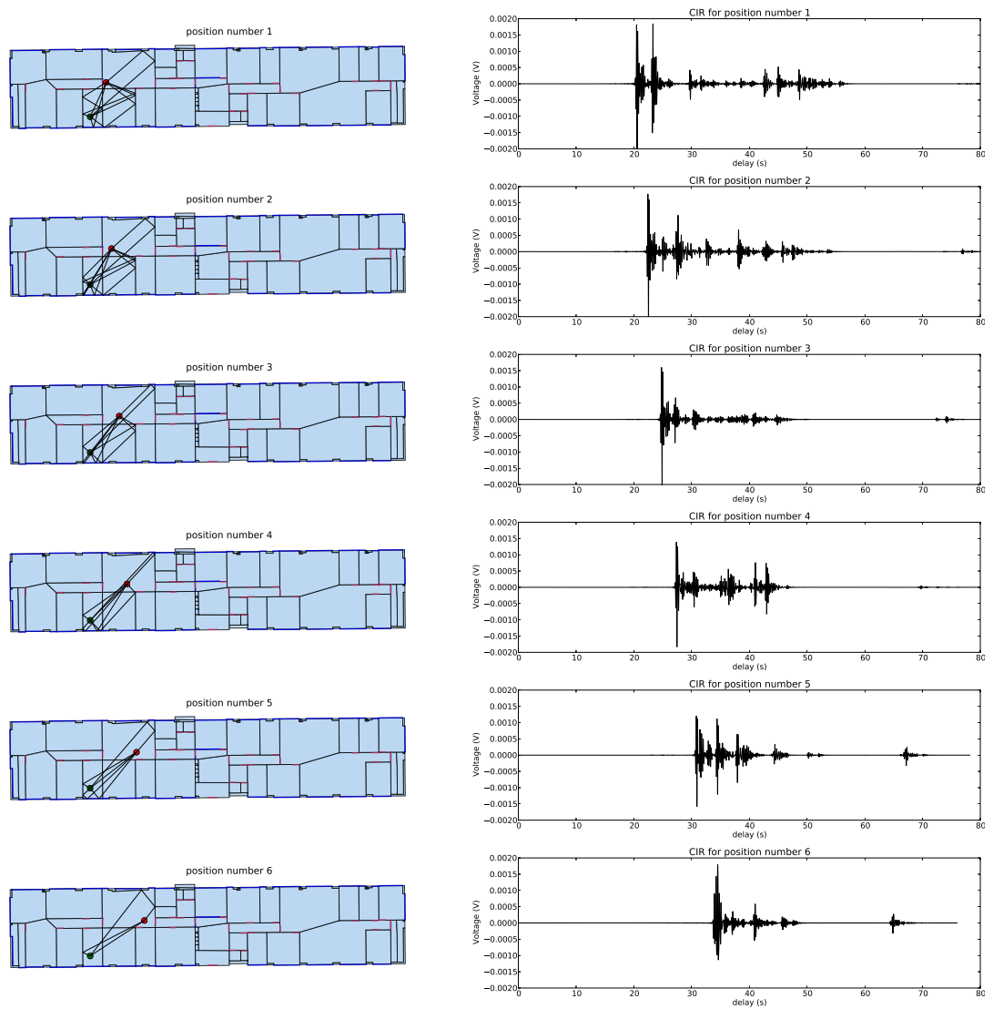
Fig. 7.19: Exemple d'obtention de CIR pour 6 positions d'agent différentes
