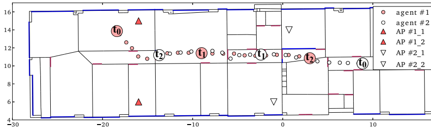
Fig. 7.20: Scenario de simulation pour illustrer l'intérêt de la communication entre agents. L'agent 1 représenté par le rond rouge ne peut se connecter qu'aux ancrées représentées par les triangles rouges. L'agent 2 représenté par le rond noir ne peut se connecter qu'aux ancrées représentées par les triangles verts. Les deux agents peuvent également communiquer entre eux s'ils sont en visibilité
