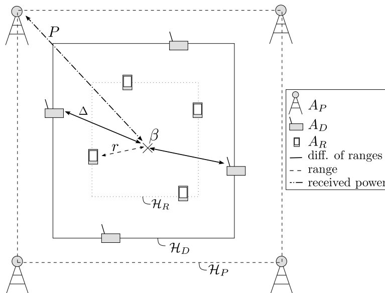
Fig. 7.10: Le nœud à positionner en position \beta a accès: à des observations de distances \{r\} provenant des ancres aux positions \{A_R\} , à des TDoA \{\Delta\} provenant des ancres aux positions \{A_D\} et des RSS \{P\} provenant des ancres aux positions \{A_P\} .
