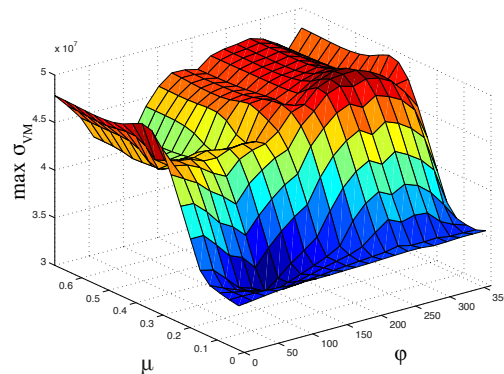
FIGURE 3.27 – Surface de réponse de référence du cas-test de fretage (contrainte de Von Mises maximale dans l'assemblage)
