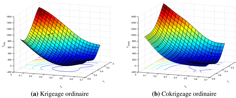
FIGURE 3.24 – Surfaces de réponse des modèles de substitution de type krigeage obtenues à partir de 15 appels au solveur
