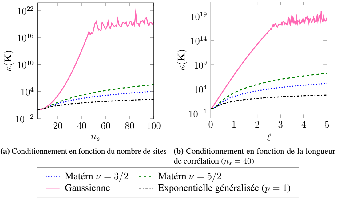
FIGURE 3.7 – Conditionnement de la matrice de corrélation pour 4 fonctions de corrélation (échantillonnages réguliers de l'espace [0, 15] et sans normalisation des sites)
