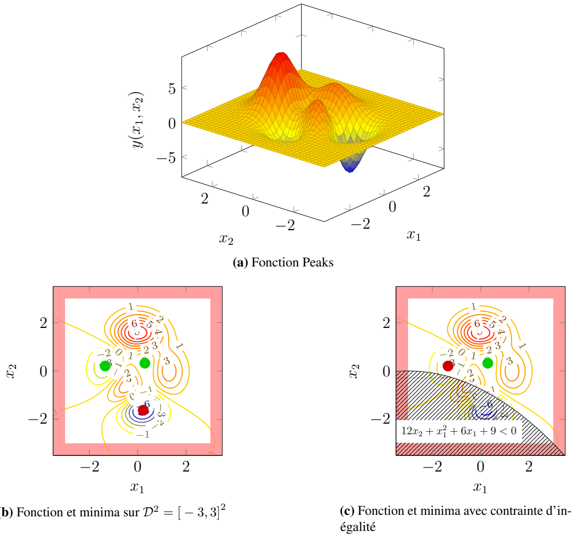
FIGURE 1.4 – Exemple de fonction à 2 variables et minima associés avec et sans contrainte d'inégalité (globaux ● et locaux ●)
