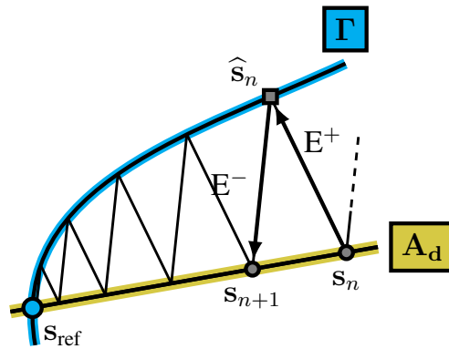
FIGURE 1.15 – Représentation schématique des itérations de l'algorithme LATIN
