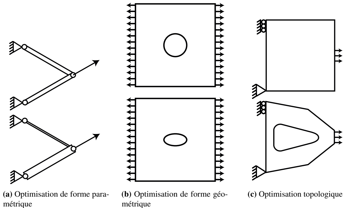
FIGURE 1.2 – Différents types d'optimisation de forme [DUYSINX 1996]
