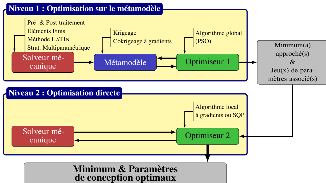
FIGURE 4.1 – Schéma synoptique de l'optimisation à deux niveaux de modèles
