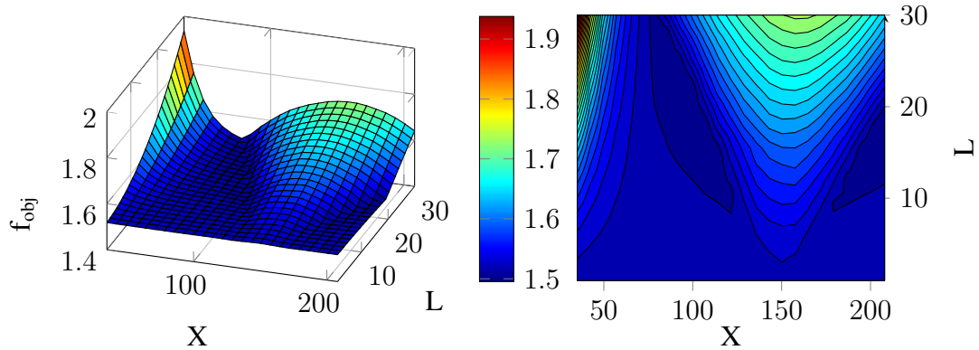
FIGURE 4.13 – Surface de réponse de la fonction objectif considérée obtenue à \eta = 10^{-4}
