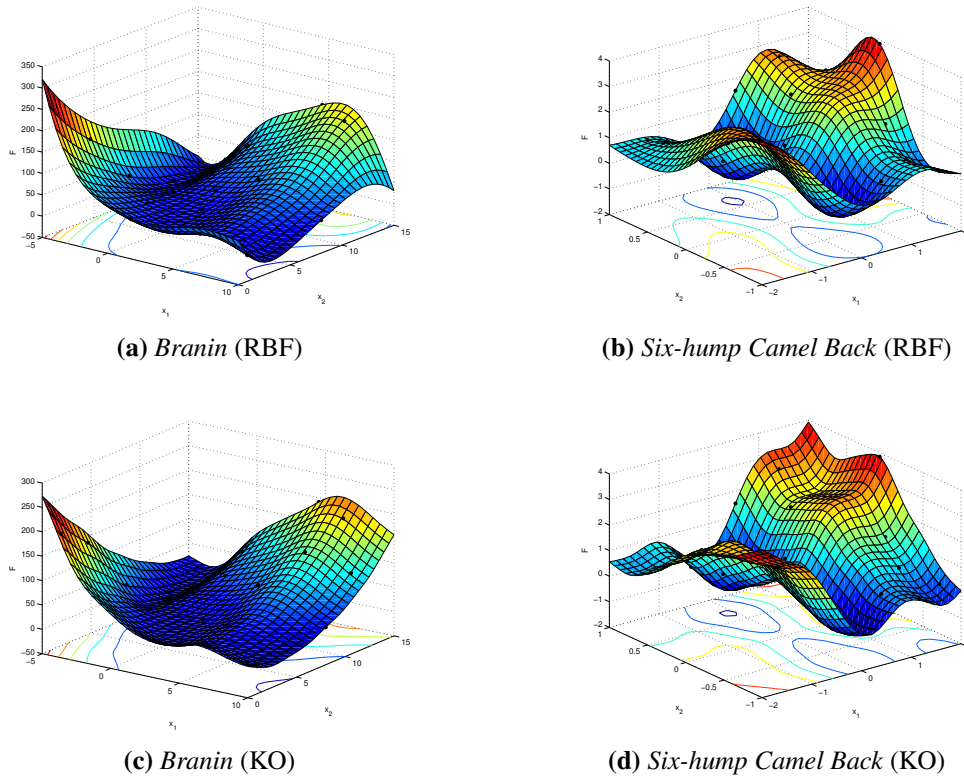
FIGURE 3.15 – Métamodèles isotropes
