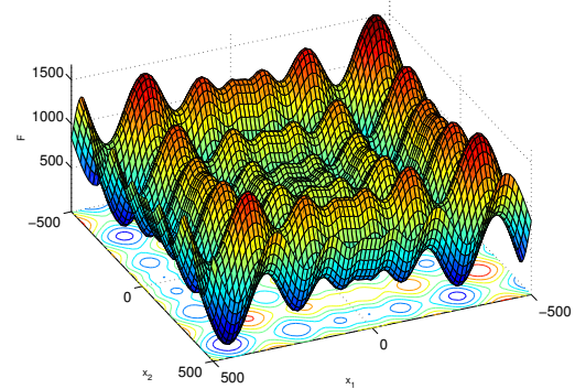
(d) Schwefel
