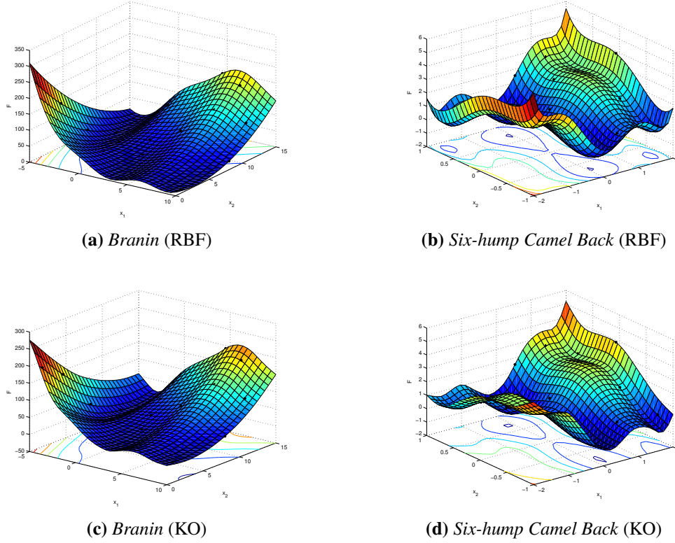
FIGURE 3.16 – Métamodèles anisotropes
