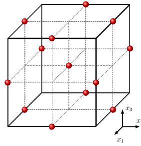
FIGURE 1.23 – Plan de Box-Behnken pour 3 paramètres
