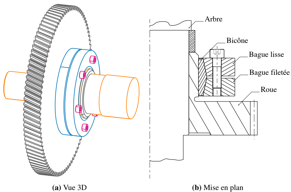
FIGURE 4.14 – Exemple d'assemblage démontable par frette conique
