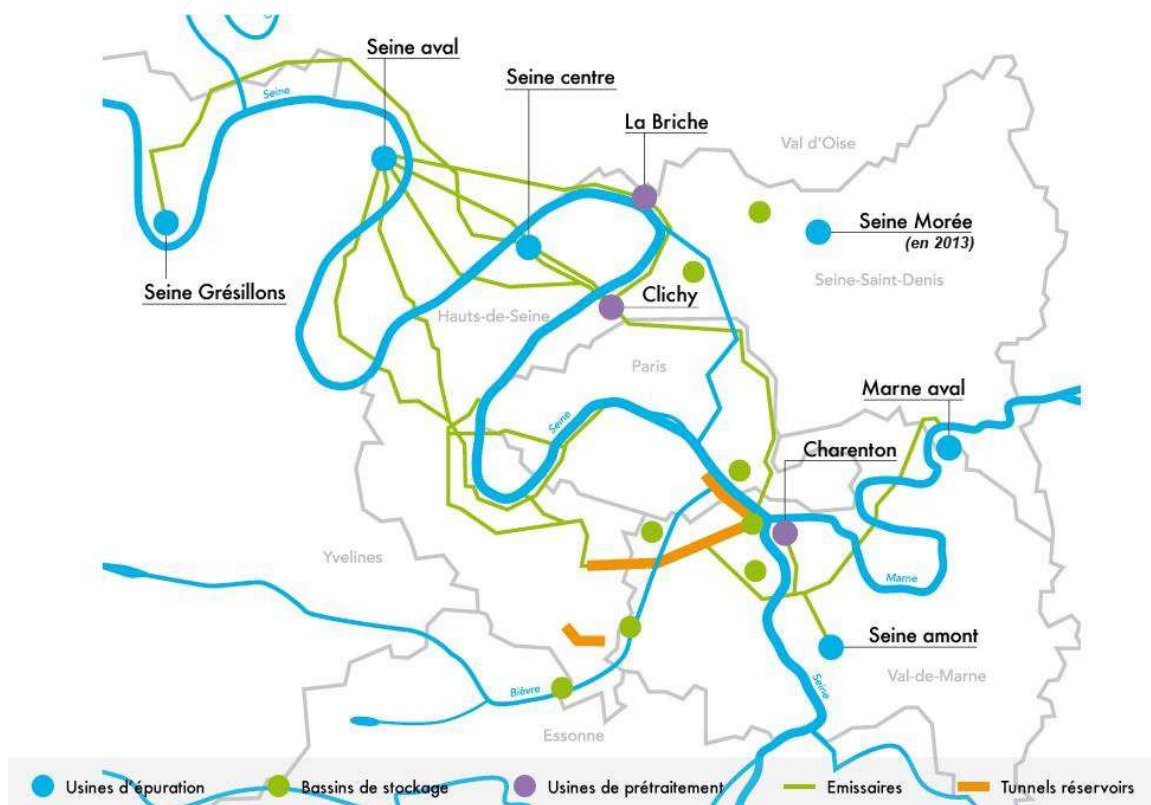
Figure 19 : Réseau de collecte des eaux usées de la région parisienne géré par le Syndicat Interdépartemental d'Assainissement de l'Agglomération Parisienne (SIAAP).
