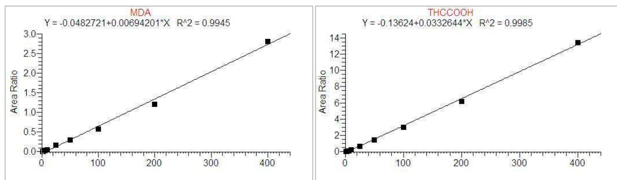
Figure 38 : Droite d'étalonnage aire composé/aire analogue deutéré=f(concentration). Les exemples choisis correspondent aux valeurs extrêmes des coefficients d'ajustement : à gauche, la valeur minimale (MDA) et à droite, la valeur maximale (THC-COOH).
