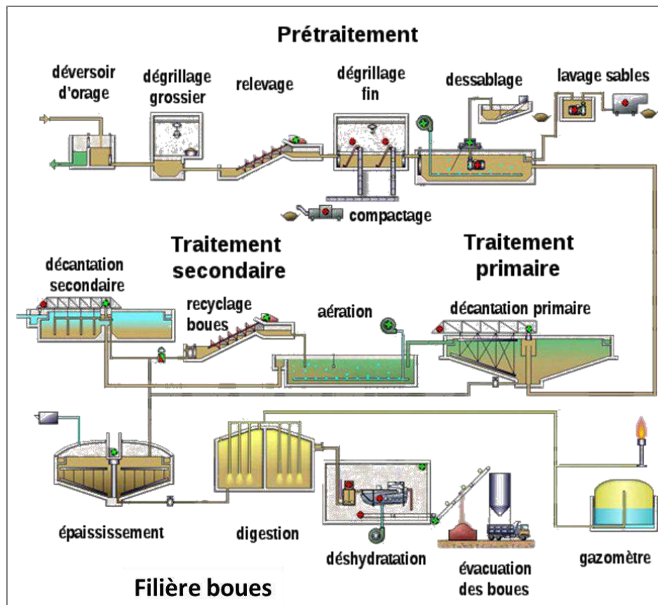
Figure 20 : Schéma du processus de traitement des eaux usées d'une station d'épuration à boues activées.
