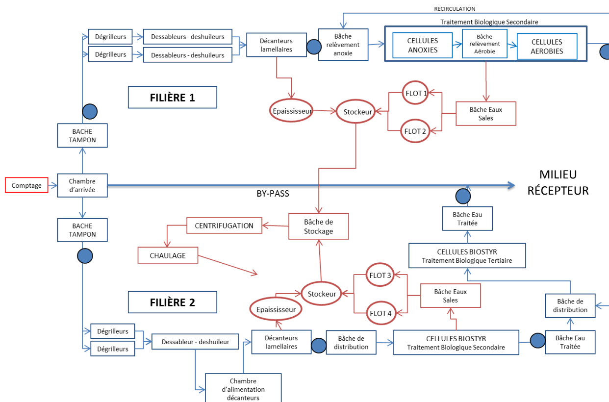
Figure 33 : Schéma de fonctionnement de la STEP SV. Les points bleus représentent les points de prélèvements.
