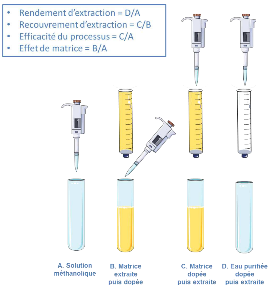
Figure 31 : Schéma du protocole d'expérience destiné à évaluer les performances des méthodes d'extraction sur cartouches SPE.
