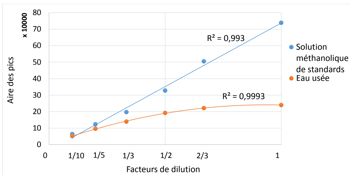
Figure 36 : Relations entre les aires des pics obtenus pour la BZE pour un extrait d'eau usée dopé puis dilué (en orange) et les aires des pics obtenus pour la BZE pour une solution méthanolique diluée dans les mêmes proportions (en bleu).
