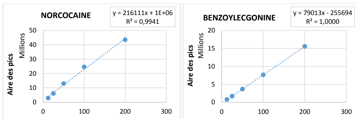
Figure 37 : Fonction de réponse aire=f(concentration). Les exemples choisis correspondent aux molécules pour lesquelles ont été obtenues les valeurs extrêmes des coefficients d'ajustement : à gauche, la valeur minimale (NOR) et à droite, la valeur maximale (BZE).
