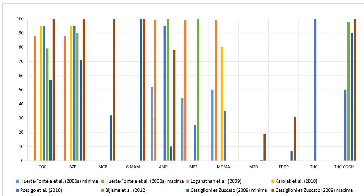
Figure 22 : Synthèse des données de la littérature concernant les pourcentages d'élimination des drogues illicites et des métabolites au sein des STEPs.
