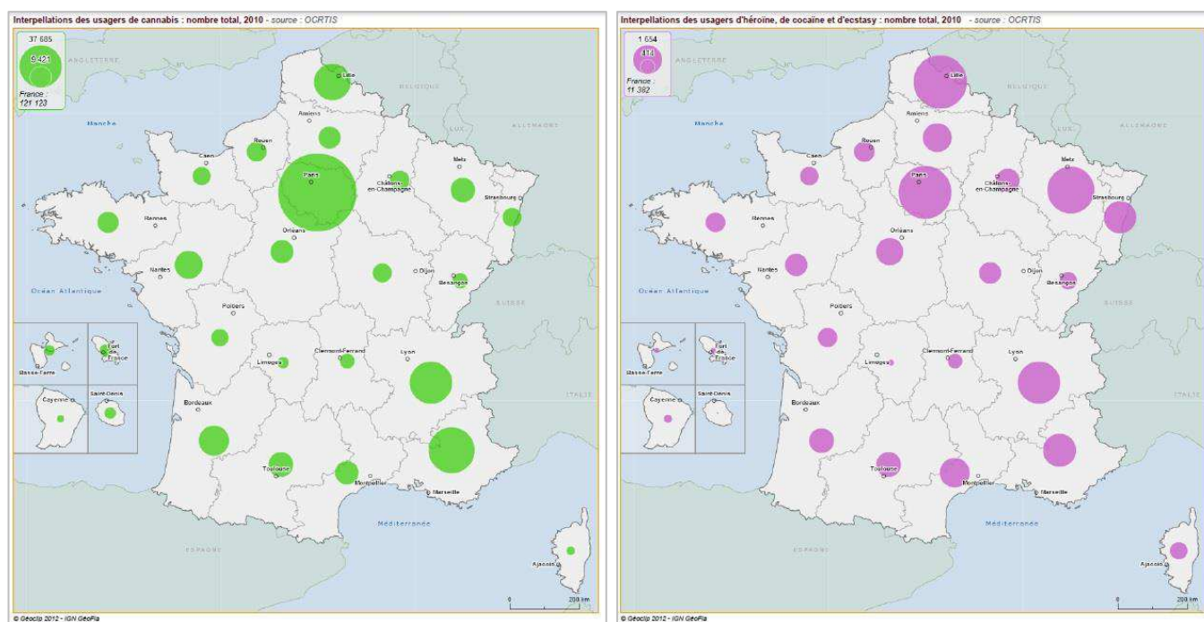
Figure 52 : Cartographies du nombre d'interpellations policières et douanières dans les cas de possession et/ou usage de cannabis (A) ou d'héroïne, de cocaïne et d'ecstasy (B) (OCRTIS, 2010). La taille des cercles est proportionnelle aux nombres d'arrestations.
