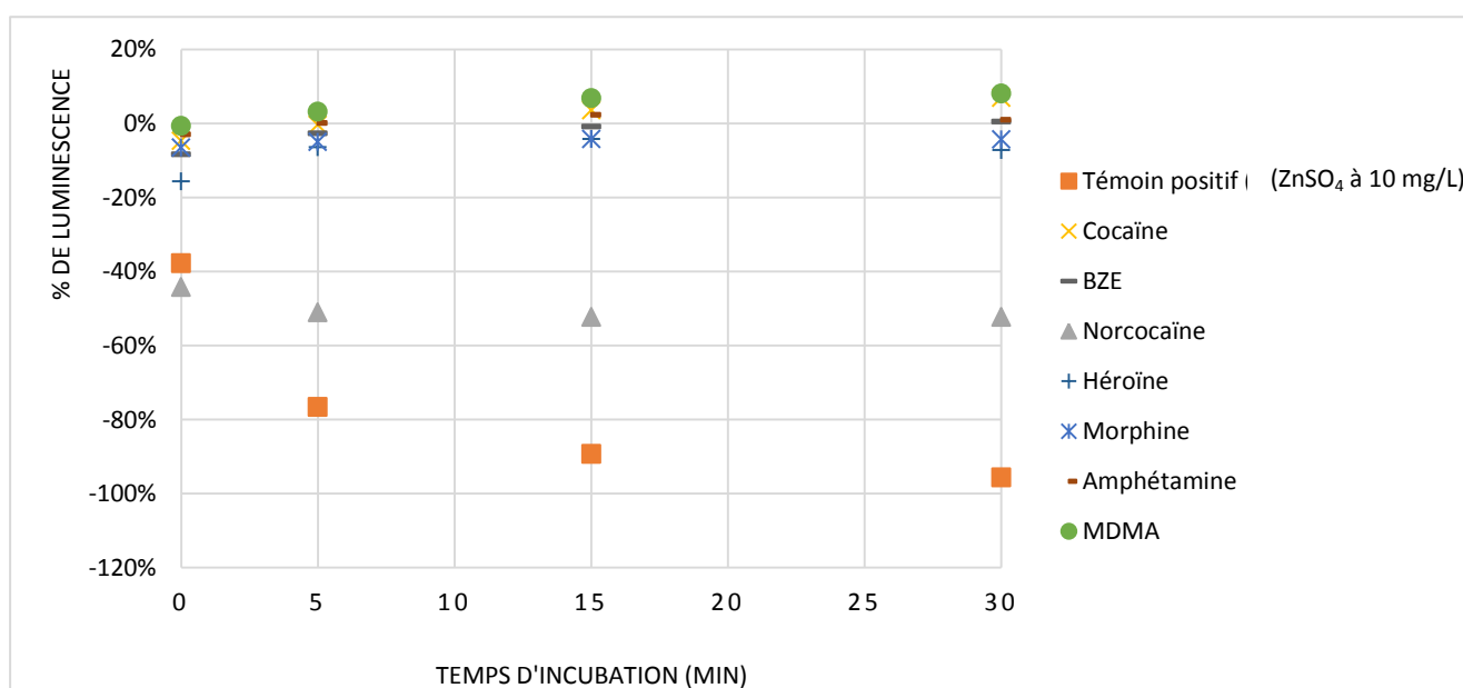
Figure 58 : Pourcentage de variation de la luminescence des bactéries Vibrio fischeri (NRRL B-11177) mesurée après exposition à la drogue (100 mg/L) par rapport à la luminescence mesurée avant exposition.
