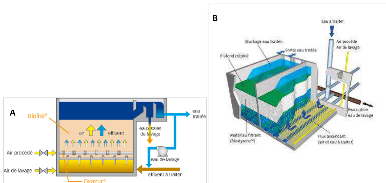
Figure 34 : Schéma des technologies de traitement par biofiltration Biofor® (A) et Biostyr™ (B).
