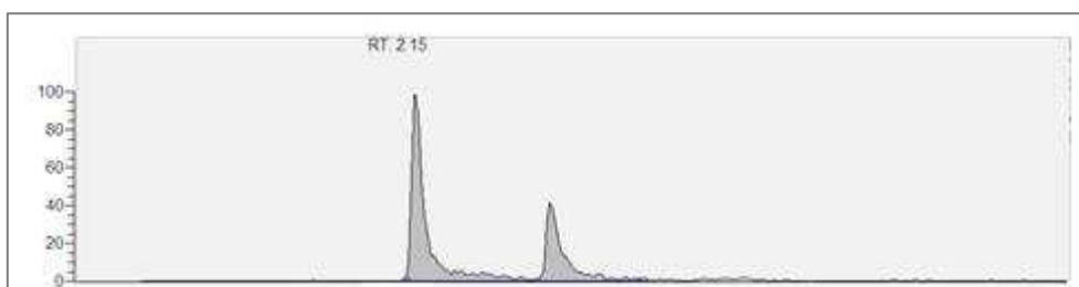
Figure 29 : Chromatogramme de l'EME. Solution méthanolique à la concentration de 100 µg/L. Le temps de rétention est de 2,15 minutes.
