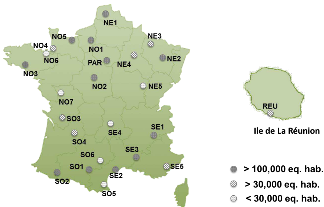
Figure 32 : Localisation et gamme de capacité de traitement des différentes STEPs étudiées.
