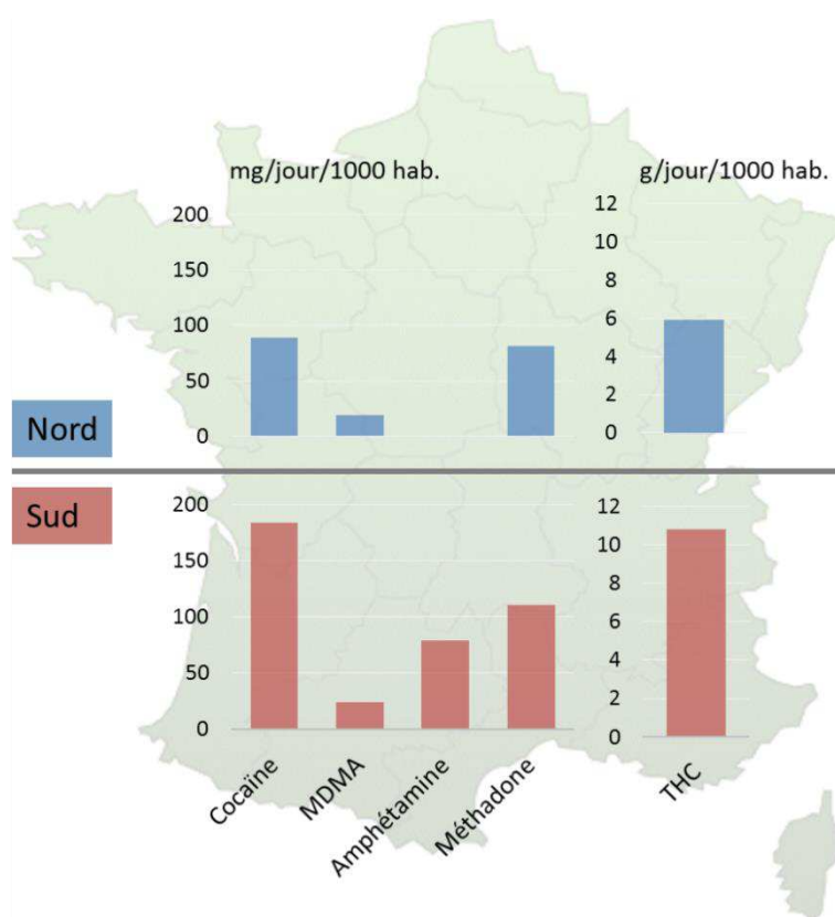
Figure 49 : Médianes des estimations de consommation de drogues (en mg/jour/1 000 hab. et en g/jour/1 000 hab. pour le THC) en fonction de la localisation des sites dans les moitiés Nord ou Sud du territoire métropolitain.
