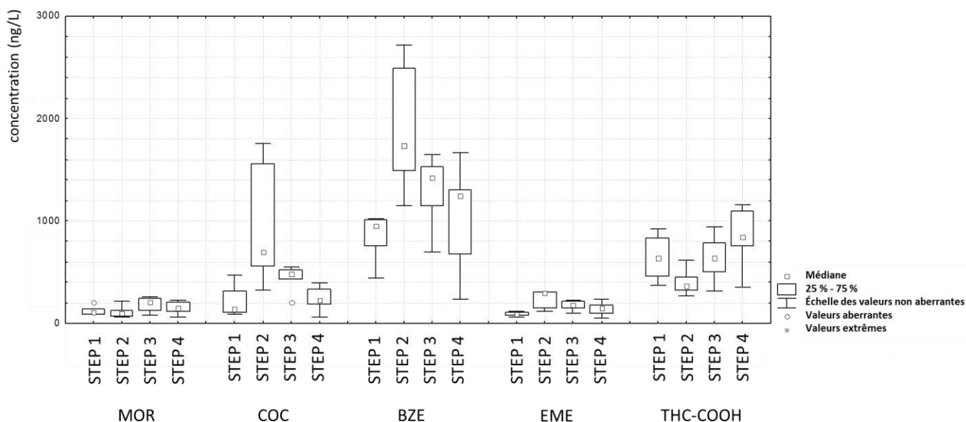
Figure 55 : Box-plot des concentrations mesurées dans les affluents des 4 STEPs analysées. Les valeurs « non détectables » ont été considérées comme des valeurs nulles.
