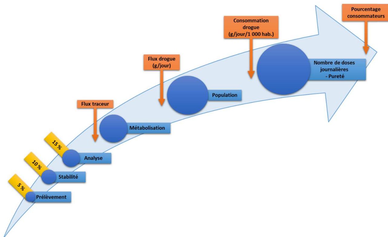
Figure 57 : Schématisation de l'évolution des incertitudes au fur et à mesure de la progression dans la méthode et du mode d'expression du résultat choisi.
