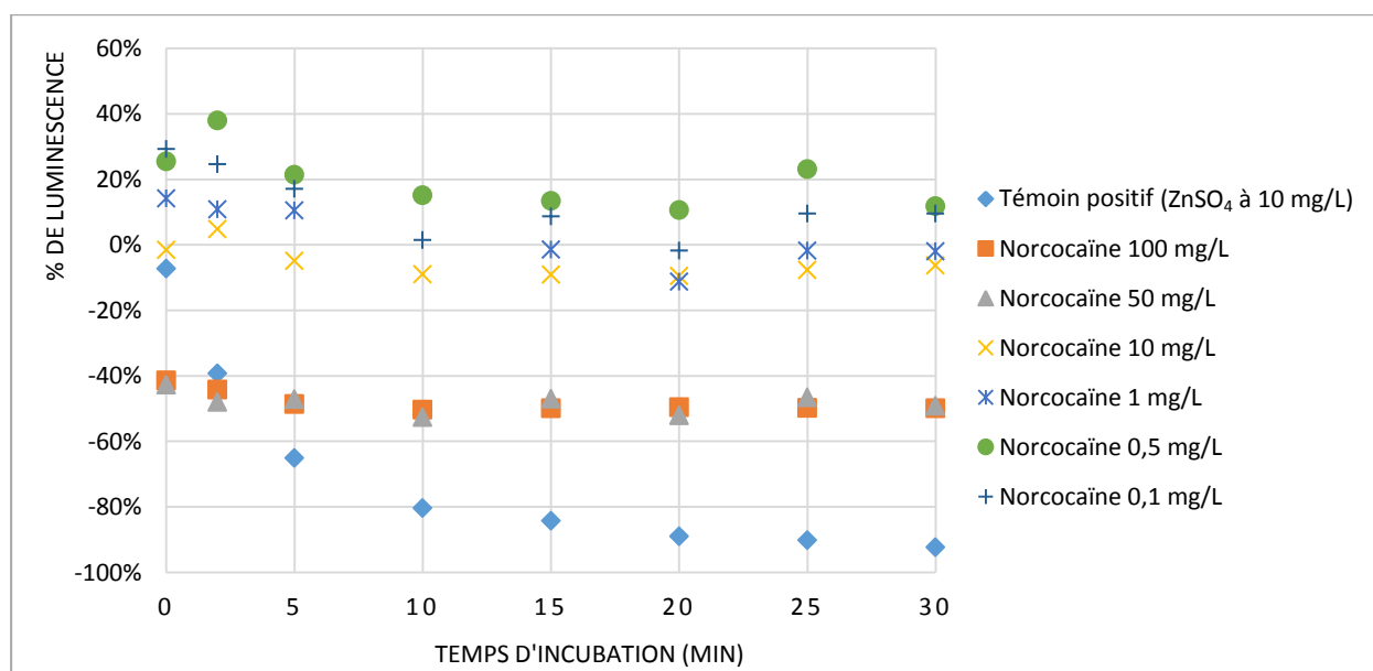
Figure 59 : Pourcentage de luminescence par rapport aux valeurs de luminescence du témoin négatif en fonction du temps et des concentrations de NOR dans le milieu en contact des bactéries Vibrio fischeri NRRL B-11177.
