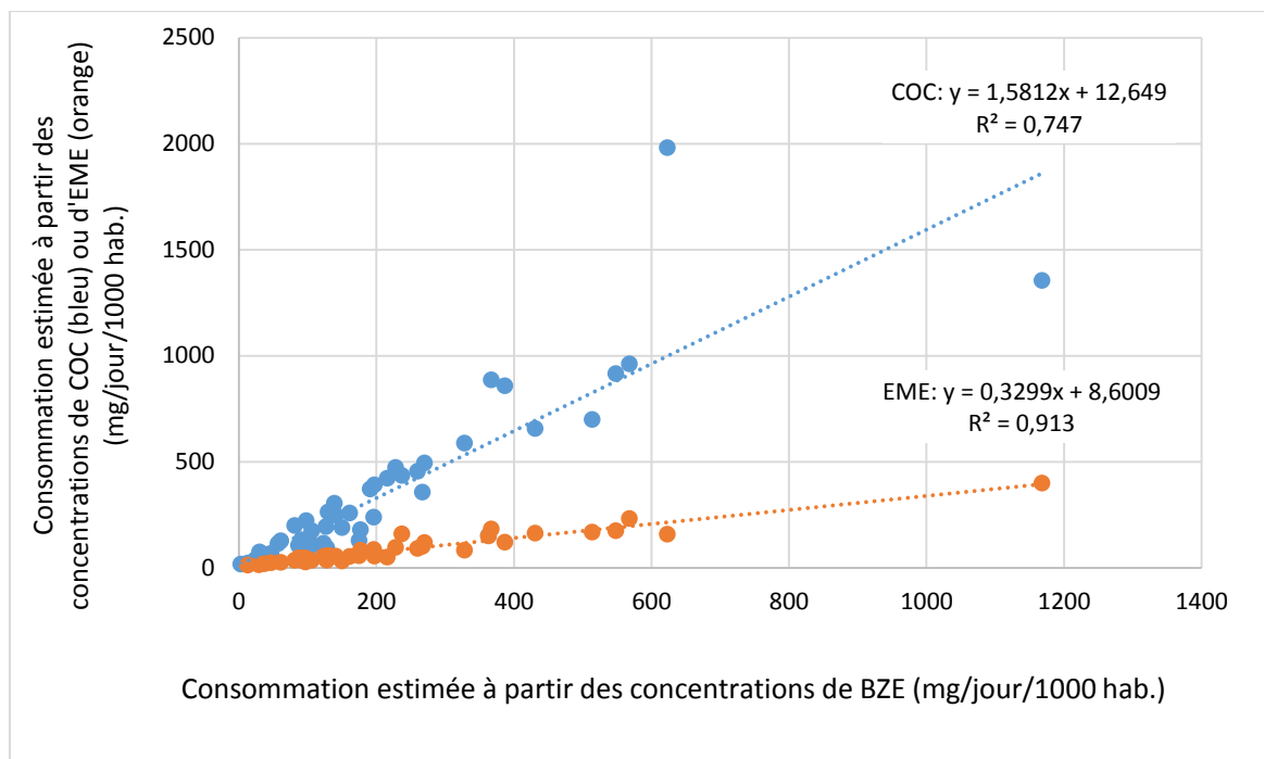
Figure 44 : Corrélation entre les estimations de consommations faites à partir de l'analyse de la COC (bleu) ou de l'EME (orange) et les estimations faites à partir de l'analyse de la BZE.
