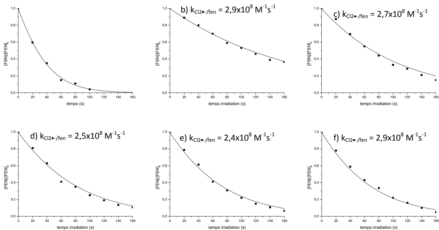
Figure 1 : cinétique de disparition du fénuron sous irradiation à 254 nm d'une solution contenant \{[fénuron] = 1 \times 10^{-6} M, [H_2O_2] = 5 \times 10^{-4} M, a) : [Cl^-] = 0 M, b) : [Cl^-] = 0,0025 M, c) : [Cl^-] = 0,01 M ; ; d) : [Cl^-] = 0,025 M, e) : [Cl^-] = 0,05 M, f) : [Cl^-] = 0,1 M, pH = 2,4 M, 254 nm\} ; ■ points expérimentaux, – modélisation en ajustant au mieux la constante de vitesse k_{Cl_2\bullet-/fen} en fonction des différentes concentrations
