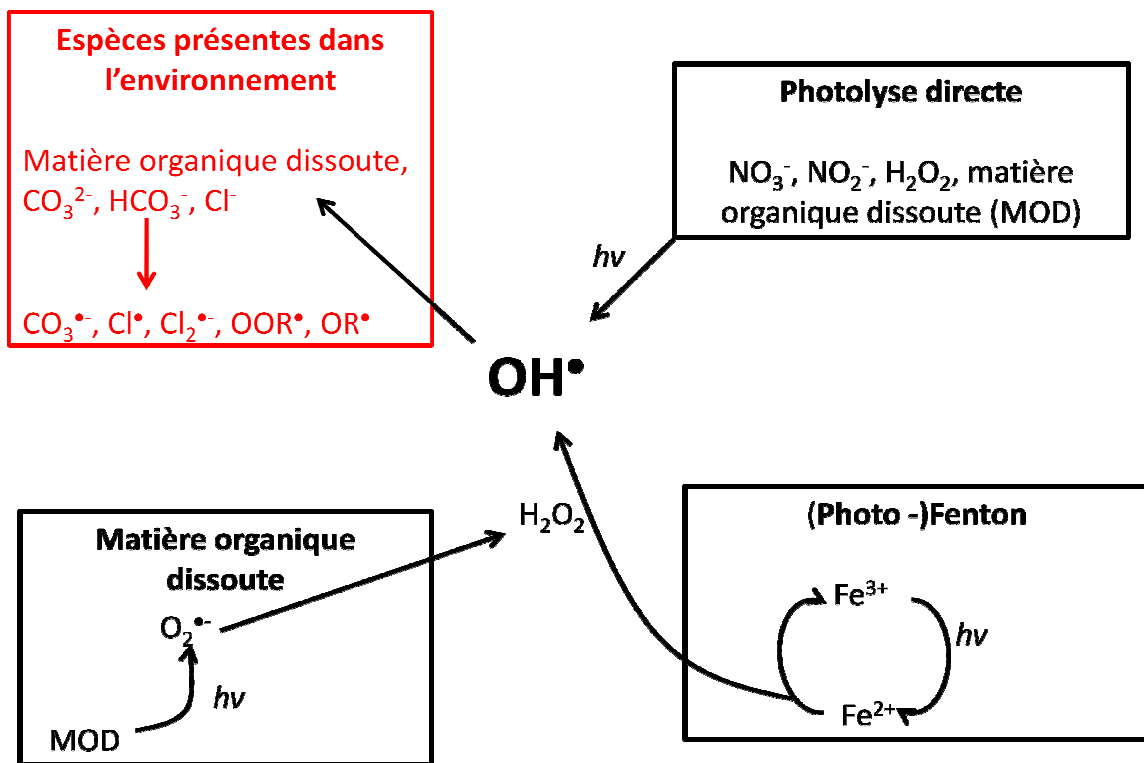
Figure I.3.: Sources de radicaux hydroxyles et production de radicaux \text{CO}_3^{\cdot-} et \text{Cl}^{\cdot}/\text{Cl}_2^{\cdot-} dans les eaux naturelles
