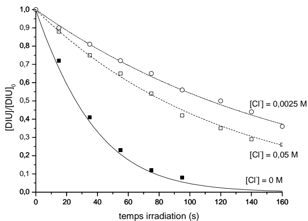
Figure 2 : (a) Disparition du diuron sous irradiation à 254 nm \{ [H_2O_2] = 2 \times 10^{-3} \text{ M} ; [\text{diuron}] = 1,0 \times 10^{-6} \text{ M} ; [\text{Cl}^-] = 0 \text{ à } 0,1 \text{ M} ; \text{pH} = 2,4 ; 254 \text{ nm} \} (b) disparition du diuron avec [\text{Cl}^-] = 0,05 \text{ M} , \text{pH} = 2,4 \text{ M} , 254 \text{ nm} ; \blacksquare points expérimentaux, – modélisation avec k_{\text{diu}/\text{Cl}_2\bullet} = 1,2 \cdot 10^8 \text{ M}^{-1} \text{ s}^{-1} \text{---} modélisation avec k_{\text{diu}/\text{Cl}_2\bullet} = 0 \text{ M}^{-1} \text{ s}^{-1}
