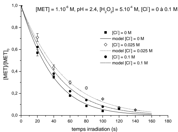
Figure 2 : (a) Disparition du métoxuron sous irradiation à 254 nm \{[H_2O_2] = 5 \times 10^{-4} \text{ M} ; [m\acute{e}toxuron] = 1,0 \times 10^{-6} \text{ M} ; [Cl^-] = 0 \text{ \AA} 0,1 \text{ M} ; pH = 2,4 ; 254 \text{ nm}\} (b) disparition du métoxuron avec [Cl^-] = 0,05 \text{ M} , pH = 2,4 \text{ M} , 254 \text{ nm} ; \blacksquare points expériméنتaux, - modélisation avec k_{pest/Cl_2^{\bullet-}} = 3,9 \cdot 10^8 \text{ M}^{-1}\text{s}^{-1} - - modélisation avec k_{pest/Cl_2^{\bullet-}} = 0 \text{ M}^{-1}\text{s}^{-1} .
