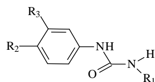
Figure I.8.: Structure d'un composé phénylurée N-déméthylé
