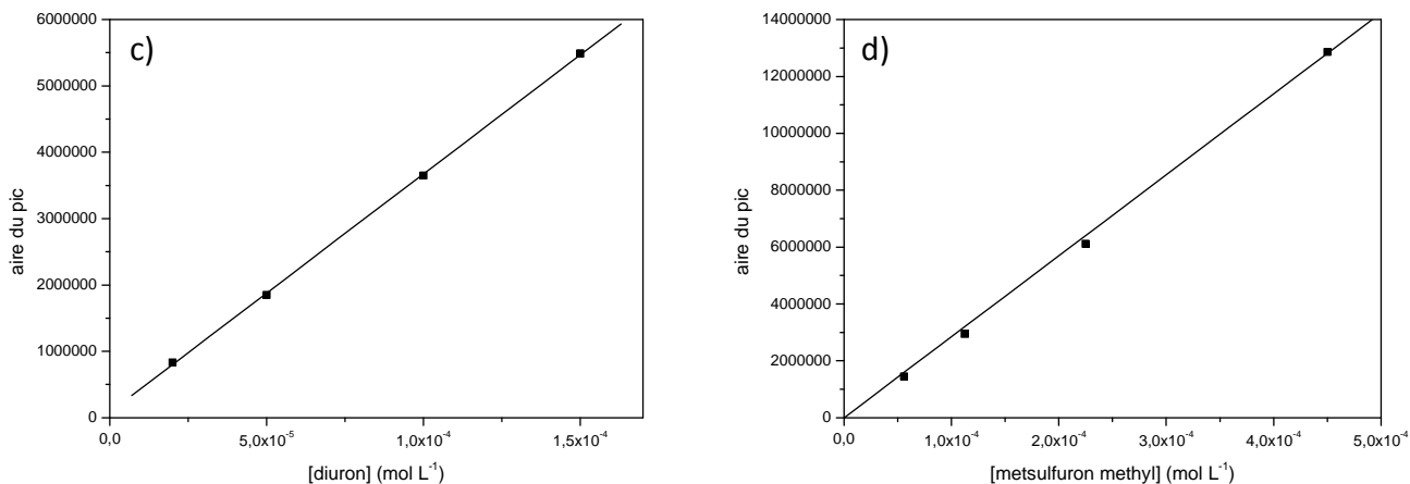
Figure II.10.: Exemples de courbes d'étalonnage CLHP obtenu pour le dosage des différents pesticides étudiés a) isoproturon ; b) fenuron ; c) diuron ; d) metsulfuron methyl
