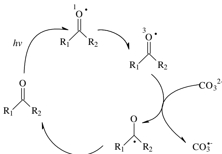
Figure I.5. : Formation du radical carbonaté par la photosensibilisation à l'aide d'une cétone
