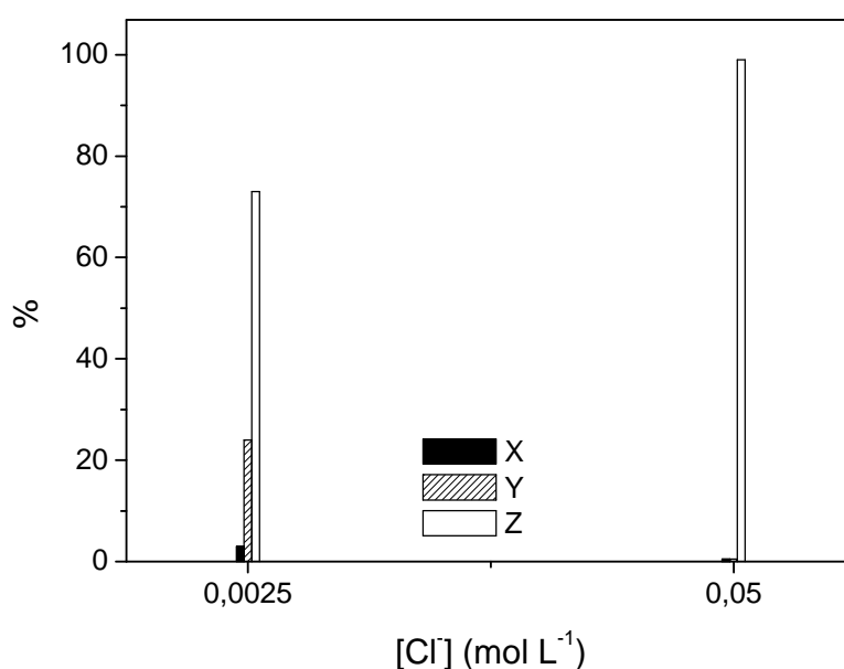
Figure IV.9.: Contribution de la photolyse directe (X), des radicaux OH^{\bullet} (Y), des radicaux Cl_2^{\bullet-}/Cl^{\bullet} (Z) à la dégradation de l'isoproturon ( [isoproturon] = 1 \times 10^{-6} \text{ mol L}^{-1} ; [H_2O_2] = 5 \times 10^{-4} \text{ mol L}^{-1} , pH = 2,4 , [Cl^-] = 0,0025 \text{ mol L}^{-1} et 0,05 \text{ mol L}^{-1} , t = 60 \text{ s} )
