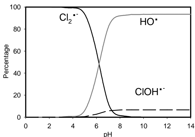
Figure I.6. : Influence du pH sur la répartition des radicaux pour une concentration totale en ions Cl - égale à 0,1 M (De Laat et al. , 2004)
