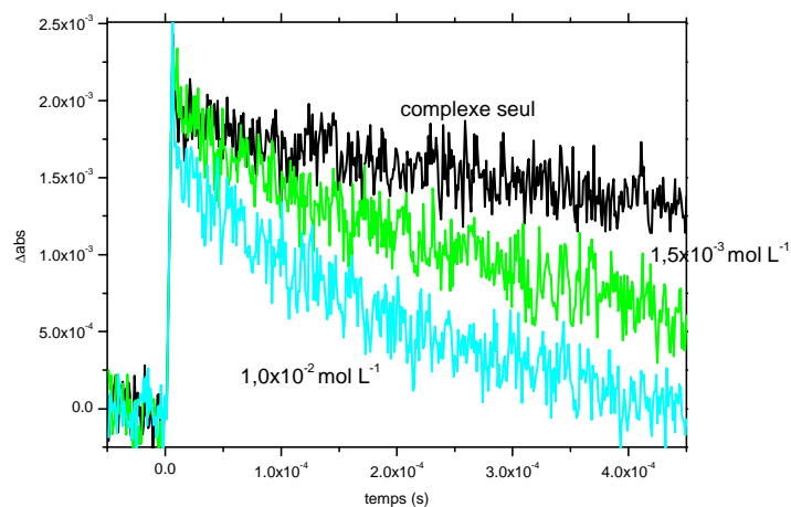
Figure III.16 : Evolution du signal à 600 nm correspondant au radical carbonate en absence et en présence de fénuron. Complexe ( 2,5 \times 10^{-3} \text{ mol L}^{-1} ), pH =6,8, milieu aéré excitation à 355 nm.
