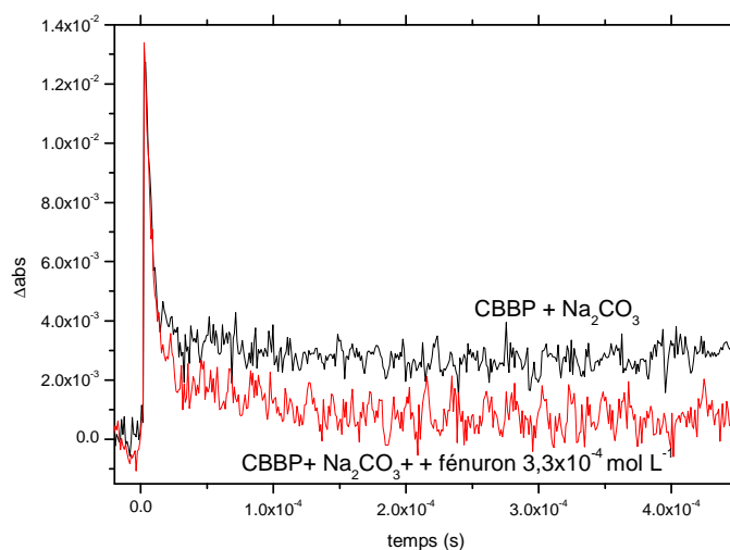
Figure III.19 : Evolution du signal à 600 nm correspondant au radical carbonate en absence et en présence de fénuon ( 3,3 \times 10^{-4} mol L -1 ). CBBP ( 5,0 \times 10^{-5} mol L -1 )/ Na 2 CO 3 (0,6 mol L -1 ), milieu aéré excitation à 355 nm.
