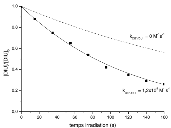
Figure 2 : (a) Disparition du diuron sous irradiation à 254 nm \{ [H_2O_2] = 2 \times 10^{-3} \text{ M} ; [\text{diuron}] = 1,0 \times 10^{-6} \text{ M} ; [\text{Cl}^-] = 0 \text{ à } 0,1 \text{ M} ; \text{pH} = 2,4 ; 254 \text{ nm} \} (b) disparition du diuron avec [\text{Cl}^-] = 0,05 \text{ M} , \text{pH} = 2,4 \text{ M} , 254 \text{ nm} ; \blacksquare points expérimentaux, – modélisation avec k_{\text{diu}/\text{Cl}_2\bullet} = 1,2 \cdot 10^8 \text{ M}^{-1} \text{ s}^{-1} \text{---} modélisation avec k_{\text{diu}/\text{Cl}_2\bullet} = 0 \text{ M}^{-1} \text{ s}^{-1}
