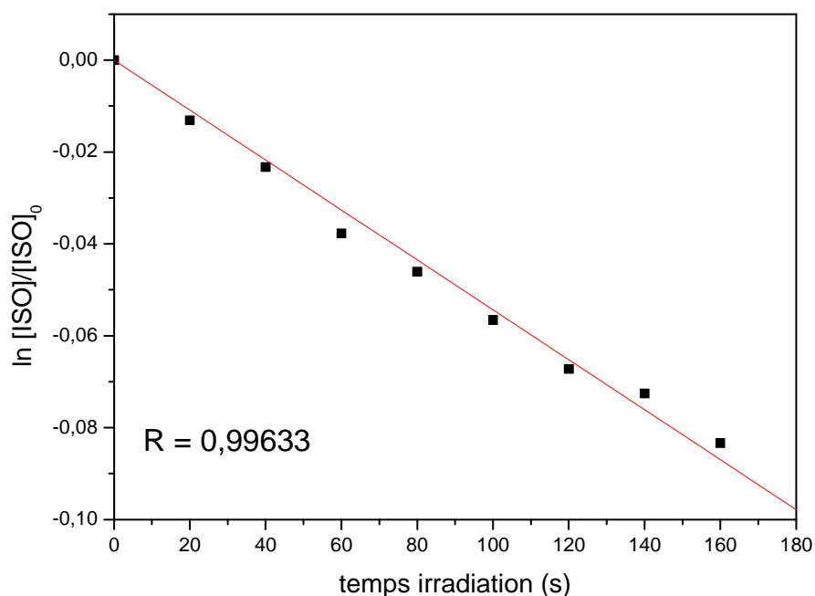
Figure IV.1: Photolyse directe de l'isoproturon ( [isoproturon] = 1,0 \times 10^{-6} \text{ mol L}^{-1} , \text{pH} = 2,4 , 254 \text{ nm} ) : application de l'équation cinétique d'ordre 1 apparent
