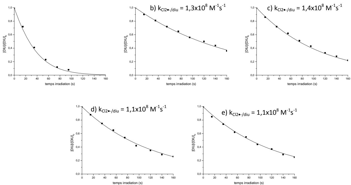
Figure 1 : cinétique de disparition du diuron sous irradiation à 254 nm d'une solution contenant \{[diuron] = 1 \times 10^{-6} \text{ M}, [H_2O_2] = 5 \times 10^{-4} \text{ M}, \text{ a) } : [Cl^-] = 0 \text{ M}, \text{ b) } : [Cl^-] = 0,0025 \text{ M} ; ; \text{ c) } : [Cl^-] = 0,01 \text{ M} ; \text{ d) } : [Cl^-] = 0,05 \text{ M} \text{ et e) } : [Cl^-] = 0,1 \text{ M}, \text{ pH} = 2,4 \text{ M}, 254 \text{ nm}\} ; ■ points expérimentaux, – modélisation en ajustant au mieux la constante de vitesse k_{Cl_2\bullet-/diu} en fonction des différentes concentrations.
