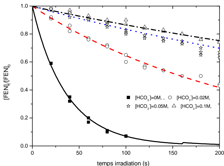
Figure III.27: Evolution de la conversion du fénuon sous excitation du peroxyde d'hydrogène à 254 nm en présence d'hydrogénocarbonate à différentes concentrations. \text{H}_2\text{O}_2 ( 1,0 \times 10^{-3} \text{ mol L}^{-1} ) / Fénuon ( 1,0 \times 10^{-6} \text{ mol L}^{-1} ), pH = 8,4.
