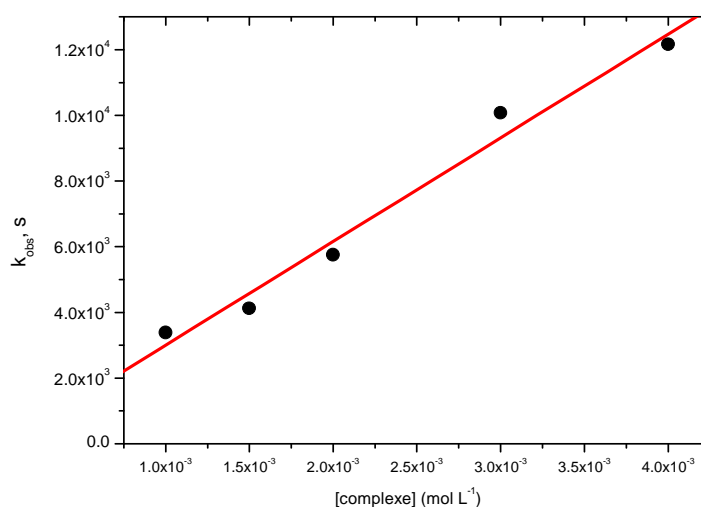
Figure III.4: La constante de vitesse de premier ordre, k_{obs} , de la disparition du radical carbonate en fonction de la concentration initiale de complexe.
