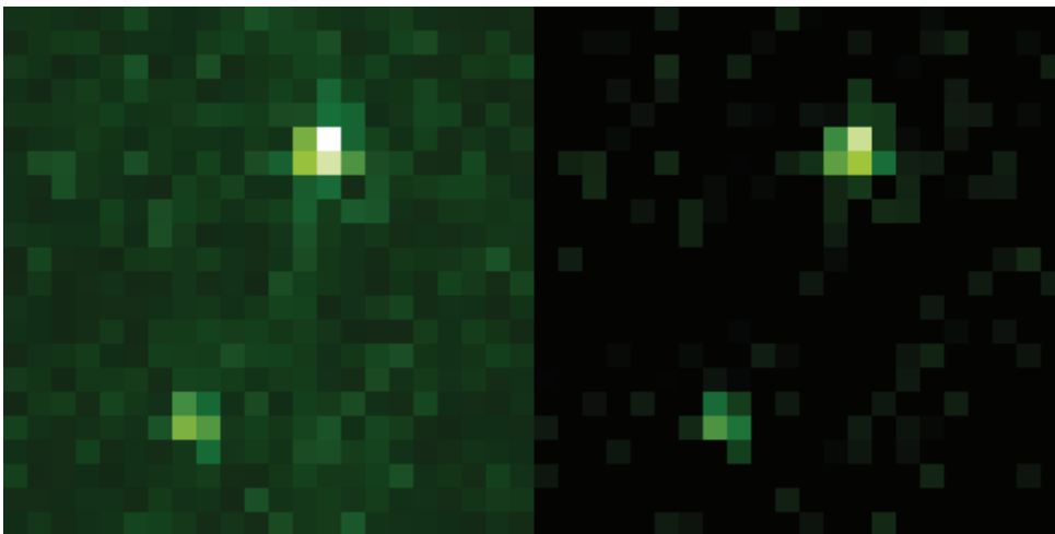
Figure 5.3 – Imagerie SH brute, à gauche et traitée, à droite, de la binaire STF1744, t_{\text{exp}} = 3 ms.
