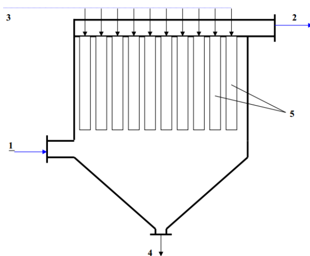
1 – Réseau de canalisation véhiculant l'air empoussiéré jusqu'au filtre, 2 – Ventilateur d'extraction -Air dépoussiéré, 3 – Alimentation en air comprimé pour rinçage inversé, 4 – Côté air empoussiéré + Vanne écluse, 5 – Manches.
