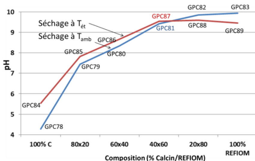
Figure V-6 : Influence du calcin ajouté au REFIOm sur le pH de lixiviat (% massiques).
