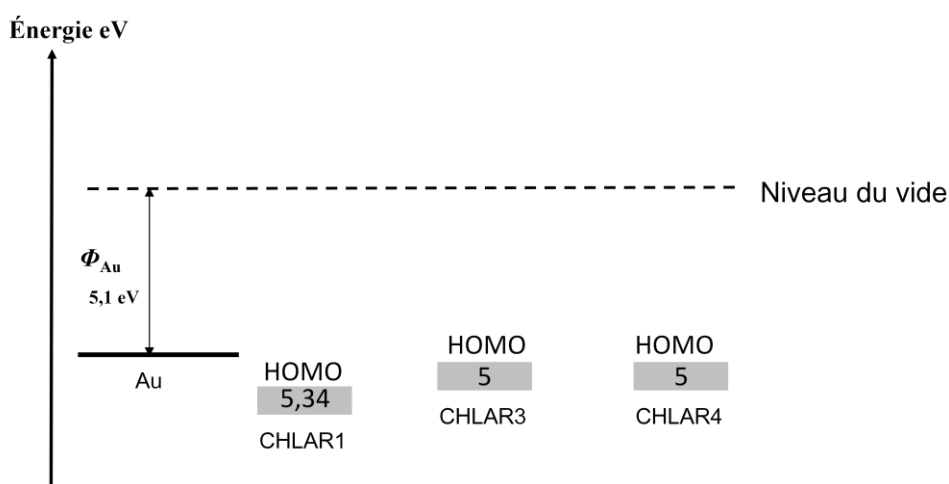
Figure 3.5 : Positionnement des niveaux HOMO des polymères par rapport au travail d'extraction de l'or.
