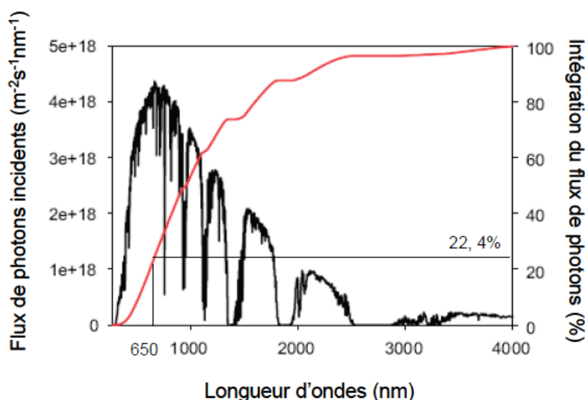
Figure 3.1 : Représentation spectrale normalisée du flux de photons incidents dans les conditions AM 1.5.
