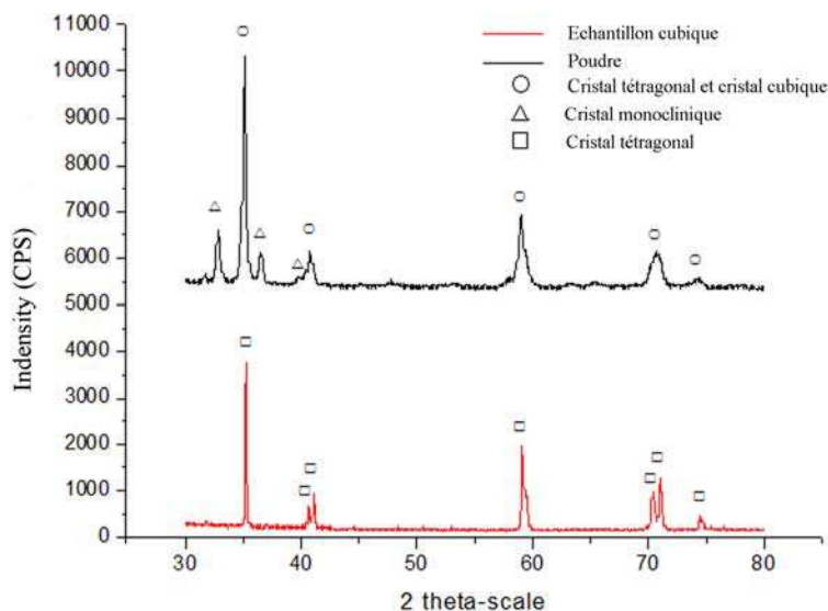
Figure III.33. Diagramme de diffraction de rayons X de la poudre YSZ et de l'échantillon cubique
