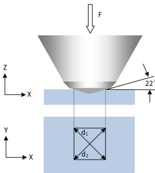
Figure II. 9. Principe de la dureté Vickers
