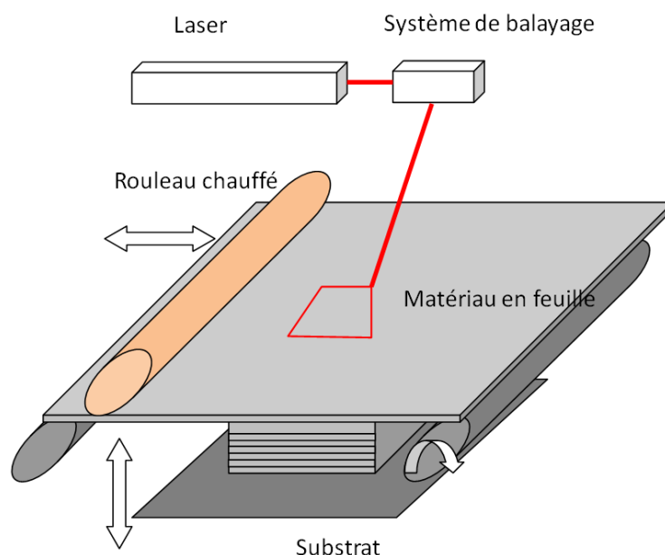
Figure I.10. Principe du procédé de fabrication d'objet par laminage
