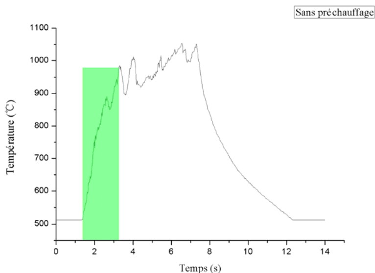
Figure IV.3. Température de la surface de l'échantillon en fonction de temps pendant le processus de numérisation sans préchauffage
