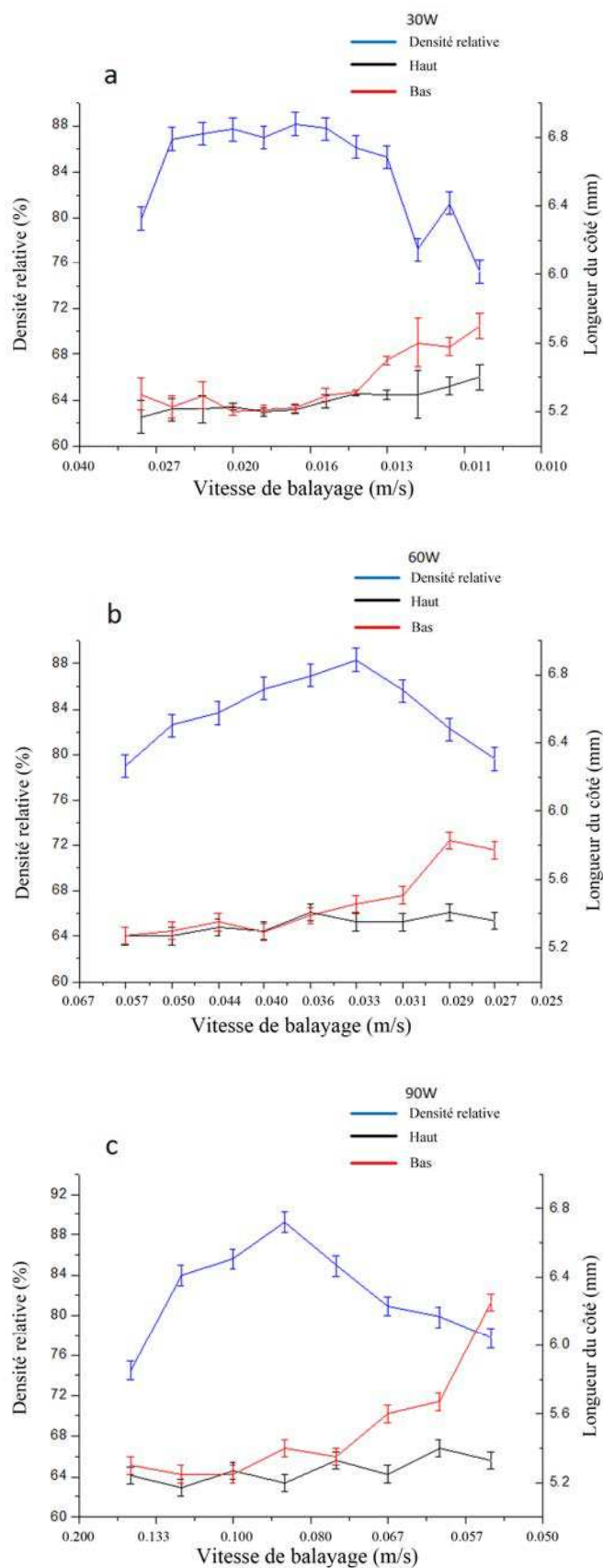
Figure III.31. Influence du temps d'exposition sur la densité relative et la longueur du côté avec préchauffage 250 °C et différentes puissances : (a) 30 W, (b) 60 W, (c) 90 W
