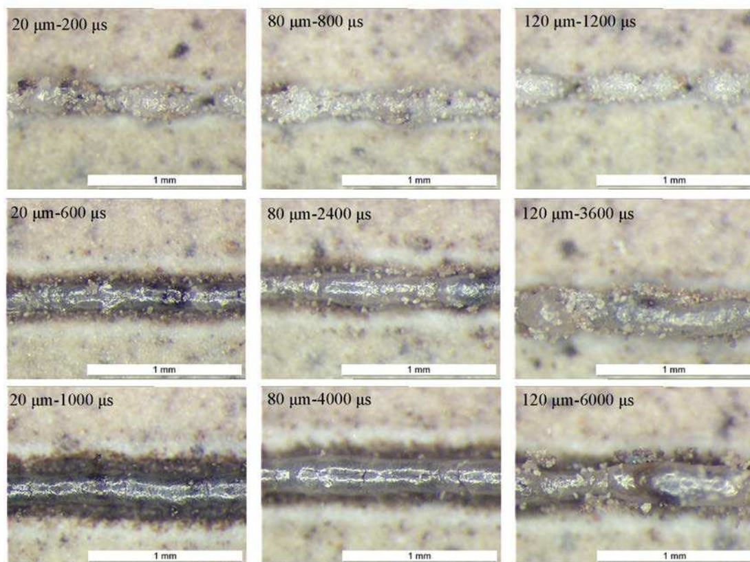
Figure III.39. Microstructure du cordon fabriqué avec des points distances et des temps d'exposition différents (même vitesse de balayage) avec le préchauffage 250 °C
