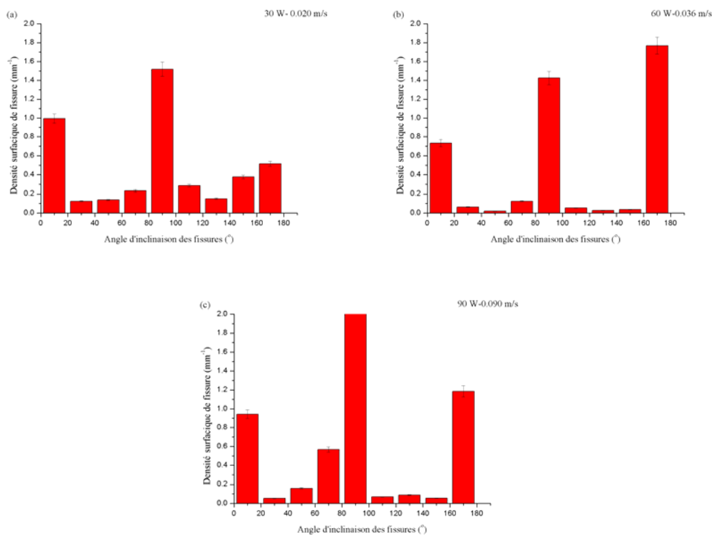
Figure III.29. Distribution de l'angle d'inclinaison des fissures avec les paramètres optimisés, (a) 30 W-0,020 m/s, (b) 60 W-0,036 m/s et (c) 90 W- 0,090 m/s et le préchauffage à 250 °C
