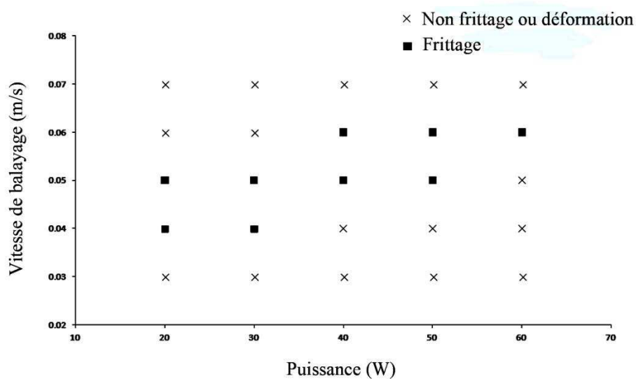
Figure III.4. Distribution des paramètres pour le frittage du mélange de poudre ( \text{Al}_2\text{O}_3 -Al 70-30)
