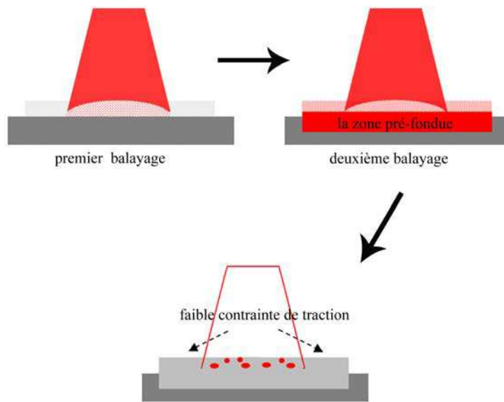
Figure IV.14. Schéma expliquant la cause de la disparition de la fissure
