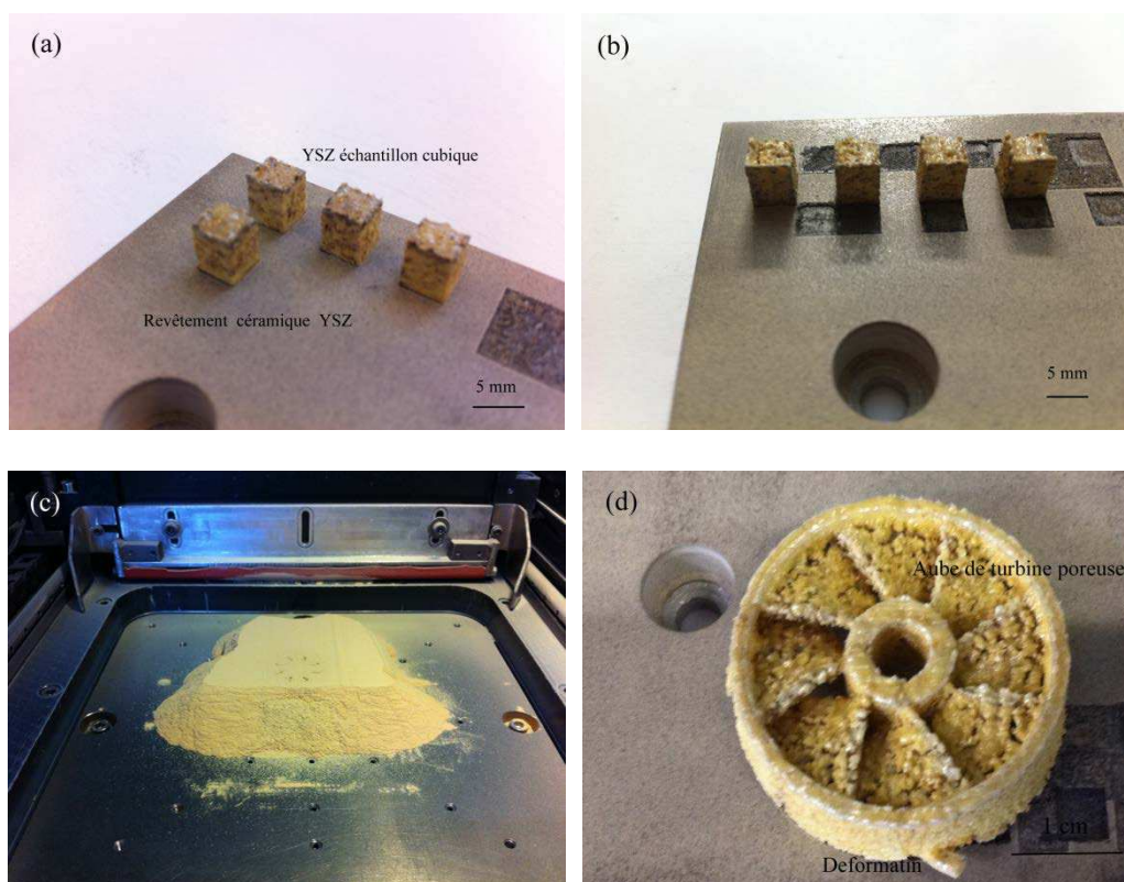
Figure III.23. (a) et (b) Quatre cubes 5 \text{ mm} \times 5 \text{ mm} \times 5 \text{ mm} avec différentes vitesses de balayage, (c) et (d) la turbine, échantillon de diamètre 30 mm
