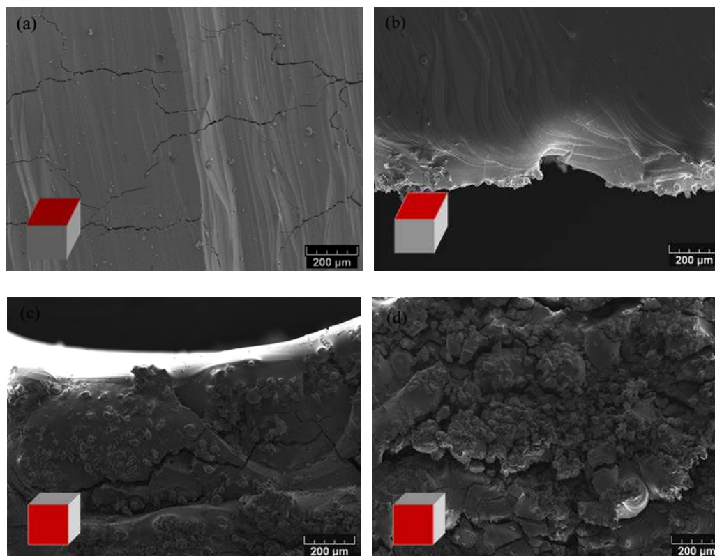
Figure III.27. La surface et le côté de l'échantillon original fabriqué avec la température de préchauffage 250 °C
