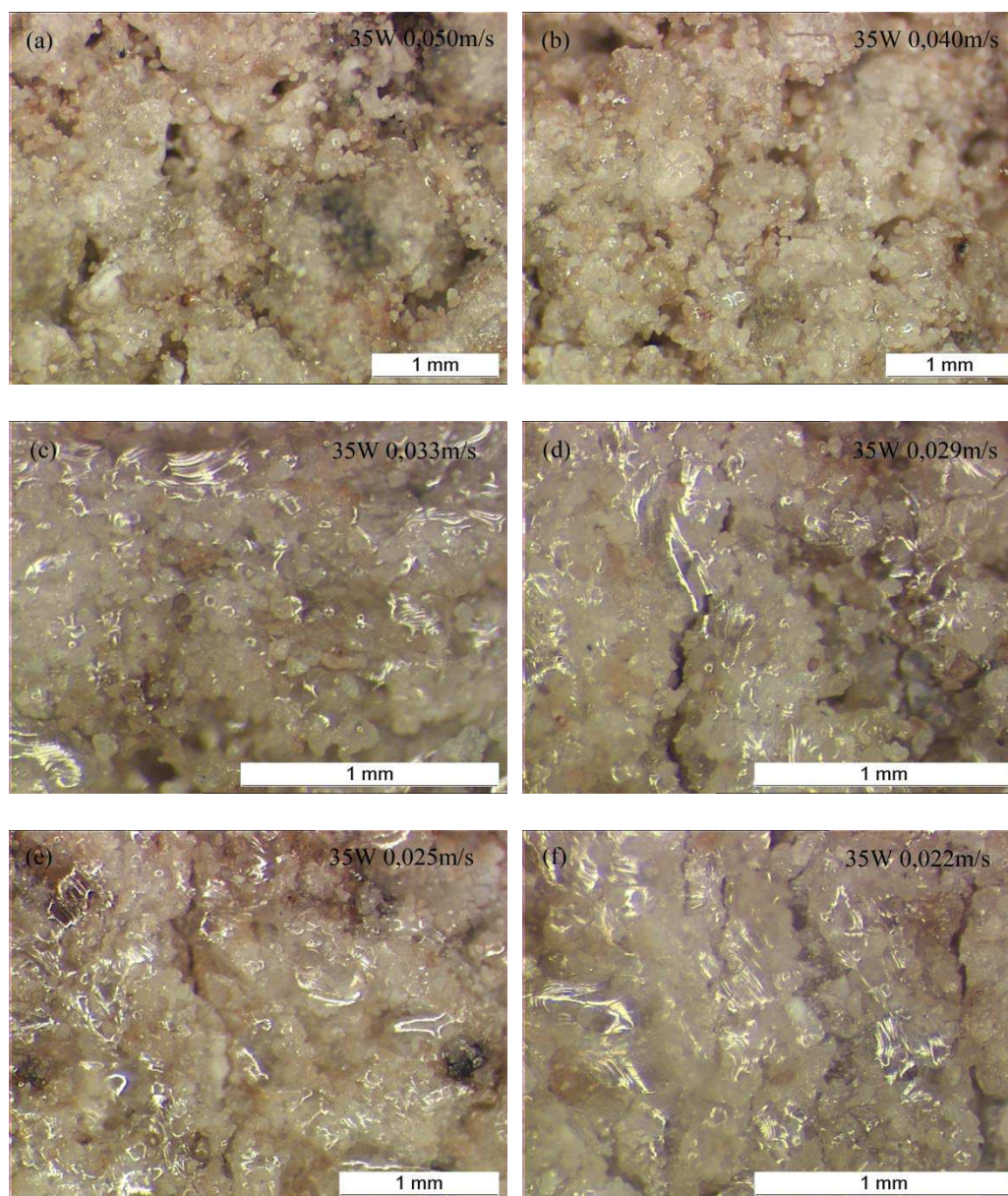
Figure III.9. Microstructure de la surface des échantillons élaborés avec la puissance 35 W et différentes vitesses de balayage: (a) 0,050 m/s, (b) 0,040 m/s, (c) 0,033 m/s, (d) 0,029 m/s, (e) 0,025 m/s, (f) 0,022 m/s
