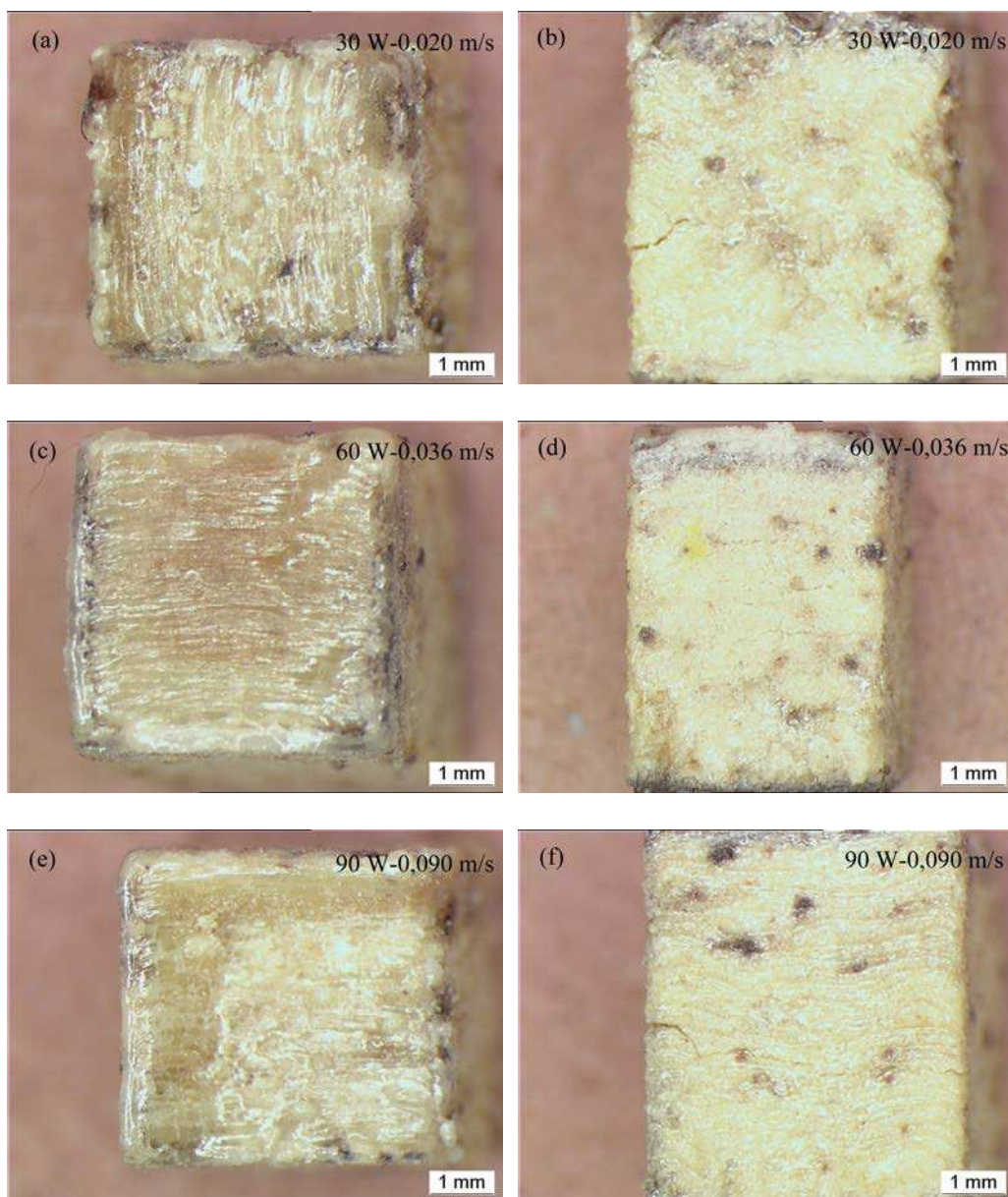
Figure III.24. Surface et face latérale de l'échantillon cubique fabriqué par des puissances différentes de laser avec préchauffage 250 °C, (a), (b) 30 W-0,020 m/s, (c), (d) 60 W-0,036 m/s, (e), (f) 90 W- 0,090 m/s
