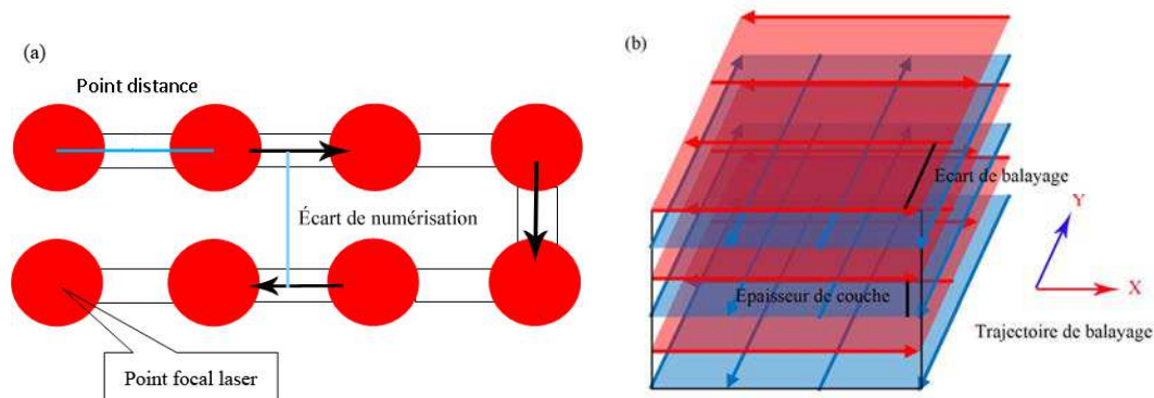
Figure III.2. (a) mode de laser balayage, (b) trajectoire de balayage pendant le procédé SLM
