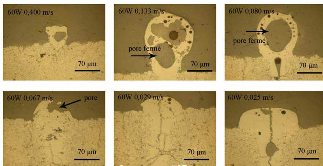
Figure III.41. Microstructure de la section d'un cordon fait à 60 W avec différentes vitesses de balayage
