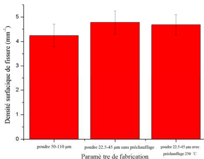
Figure III.30. Comparaison de la densité des fissures des échantillons fabriqués avec les différents paramètres (poudre 55-110 μm, 22,5-45 μm, sans préchauffage, et avec préchauffage à 250 °C)
