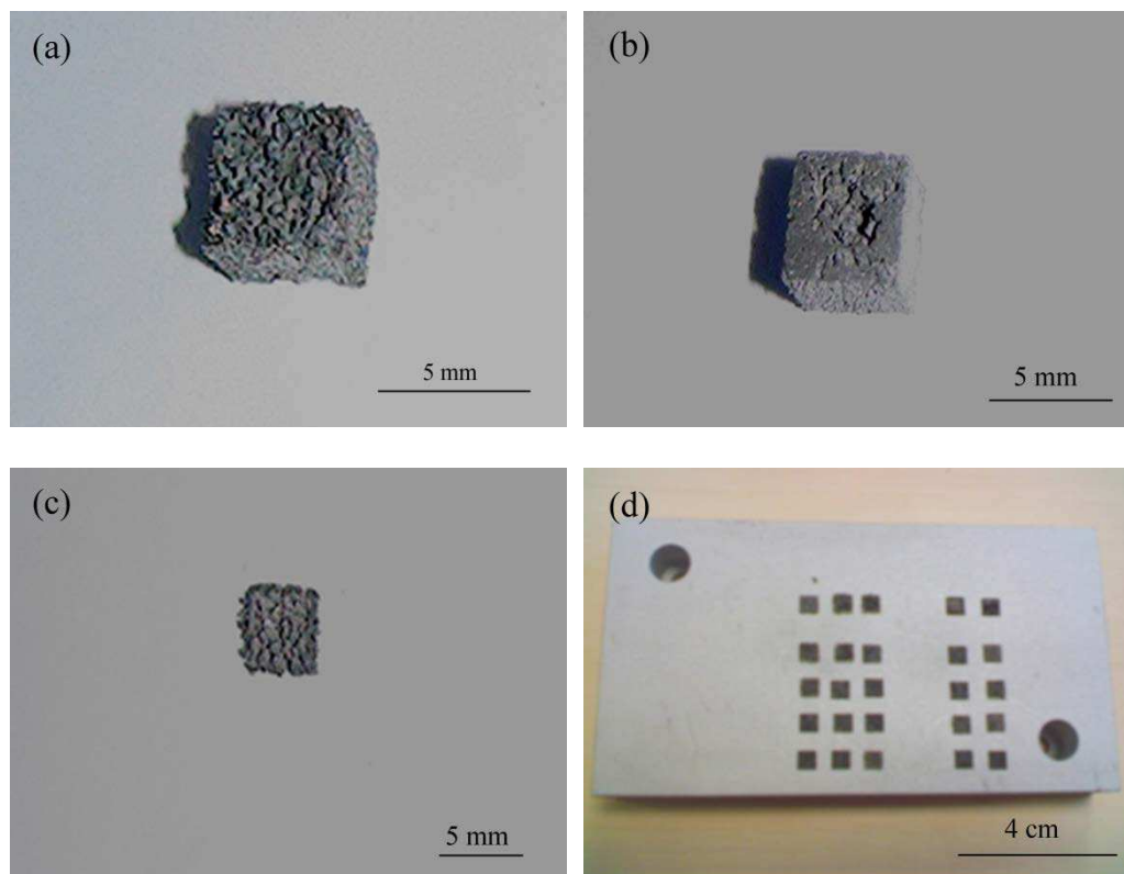
Figure III.5. Etat de frittage du mélange de poudre \text{Al}_2\text{O}_3\text{-Al 70-30} , (a) haut d'échantillon, (b) bas d'échantillon, (c) couche de poudre frittée (d) support métallique
