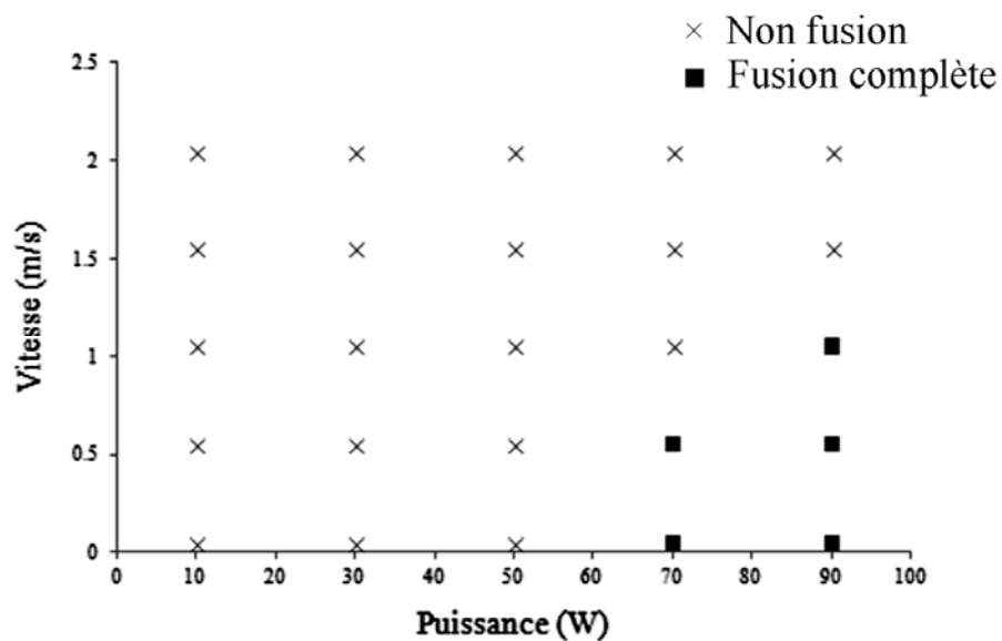
Figure III.3. Fusion sélective par laser initial d'un matériau céramique YSZ avec des puissances et des vitesses de balayage différentes
