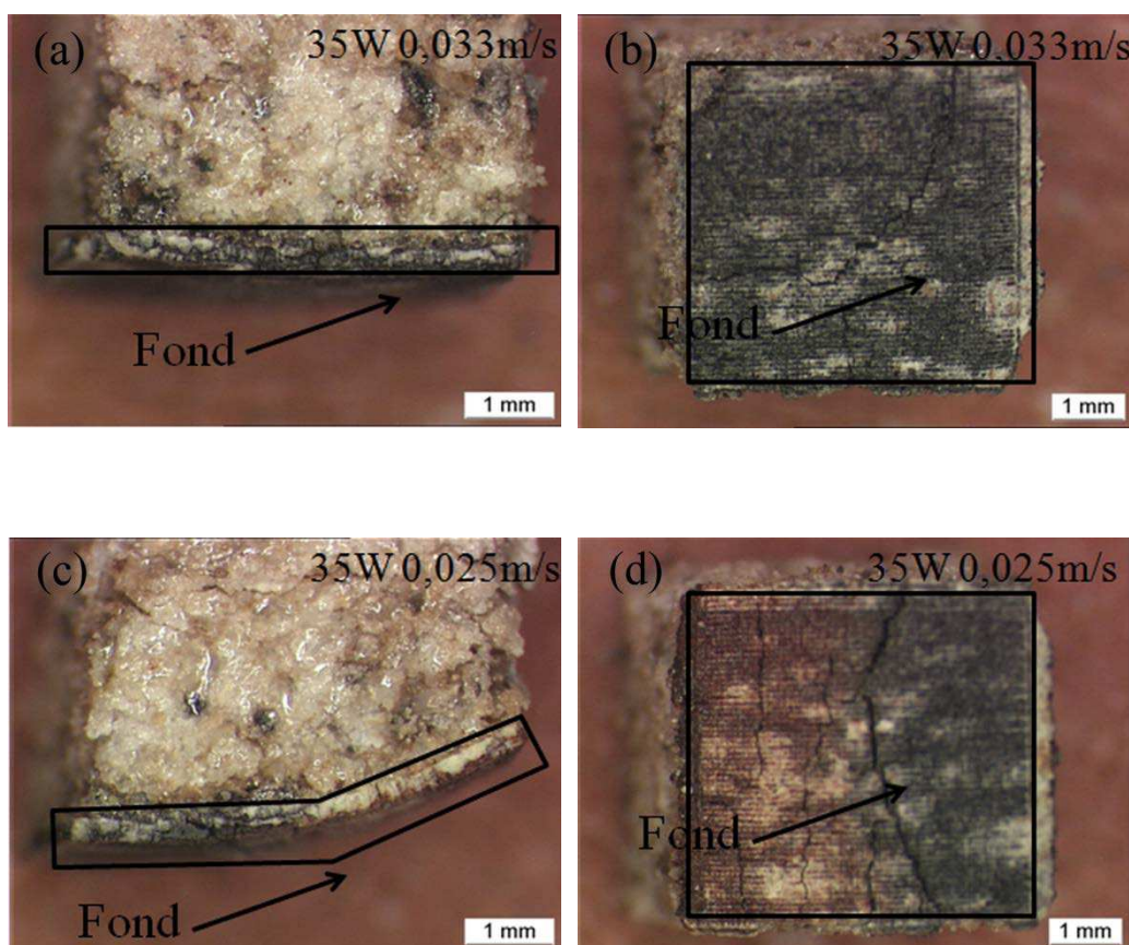
Figure III.11. Déformation du fond d'échantillon YSZ 55-110 \mu\text{m} , (a), (b) 35 W-0,033 m/s, (c), (d) 35 W-0,025 m/s
