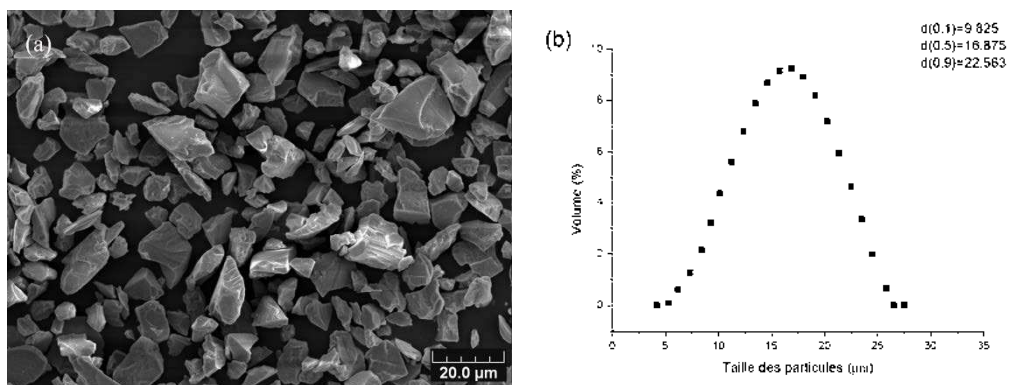
Figure II.1. (a) Image MEB de la poudre YSZ 9-22,5 \mu\text{m} ; (b) Distribution granulométrique de cette même poudre
