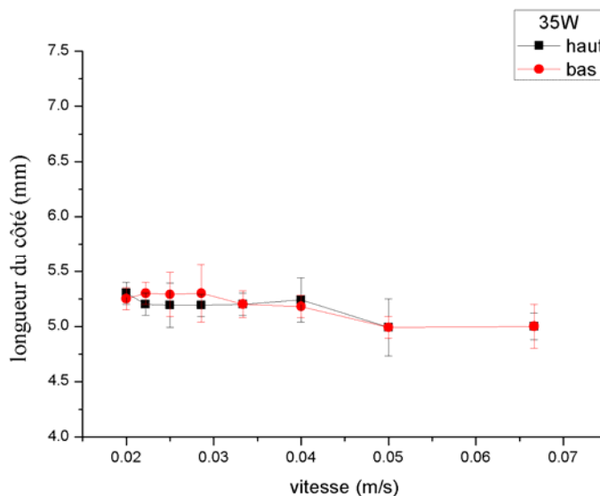
Figure III.16. Relation entre vitesse et longueur du côté à la puissance 35 W ; la longueur du côté en bas : la ligne rouge, la longueur du côté en haut : la ligne noire
