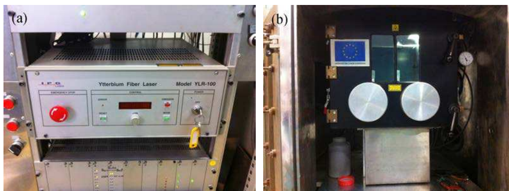
Figure II.4. (a) Equipement de Nd : YAG laser ; (b) cellule de fabrication dans la machine SLM 250
