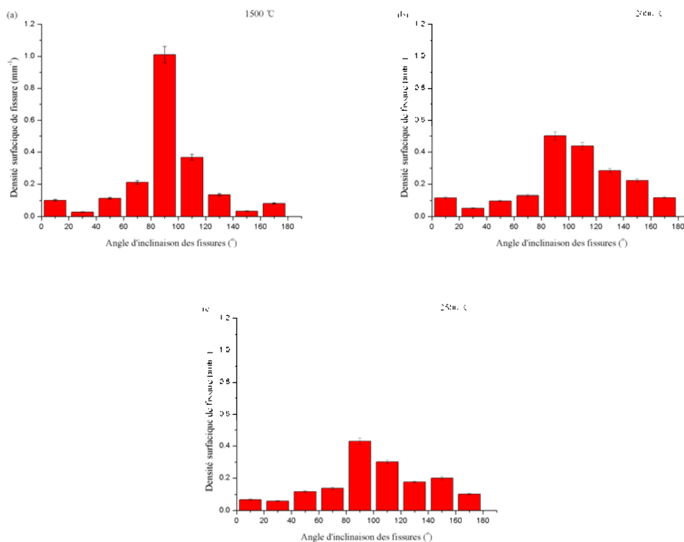
Figure IV.12. Distribution des fissures dans la section verticale d'échantillon avec préchauffage à différentes températures: (a) 1500 °C, (b) 2000 °C et (c) 2500 °C
