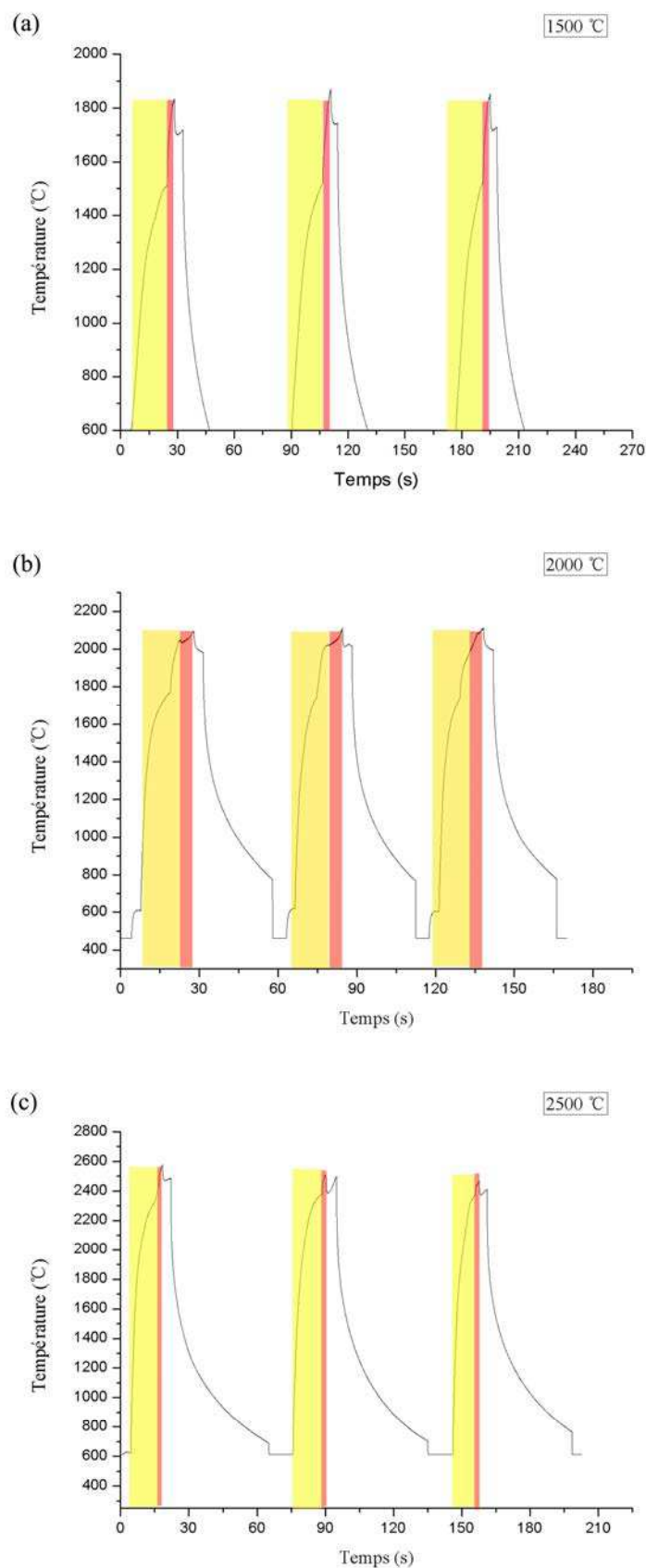
Figure IV.5. Température de surface de l'échantillon en fonction du temps avec différentes températures de préchauffage (a) 1500 °C (b) 2000 °C et (c) 2500 °C
