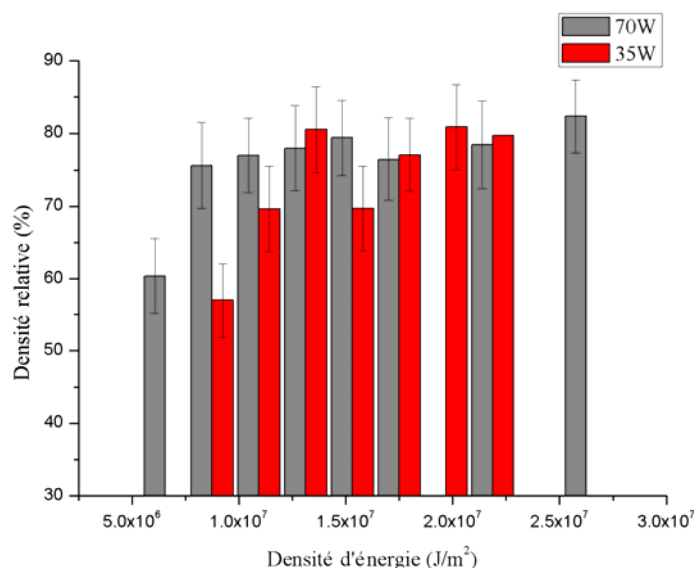
Figure III.15. Relation entre la densité d'énergie et la densité relative aux différentes puissances de laser ; barres noires 70 W et rouges 35 W
