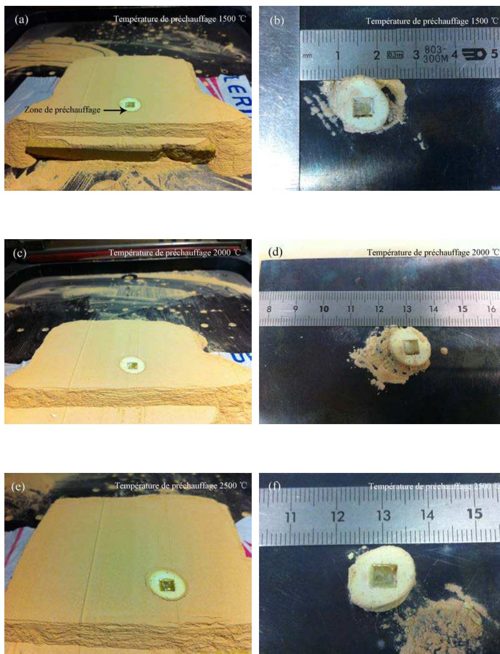
Figure IV.6. Photos des échantillons faits à 60 W avec les différentes températures de préchauffage : (a) (b) 1500 °C, (c) (d) 2000 °C et (e) (f) 2500 °C
