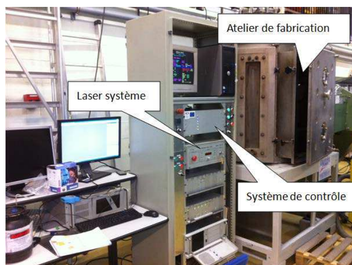
Figure I.15. La première génération de machines MCP ReaLizer SLM 250
