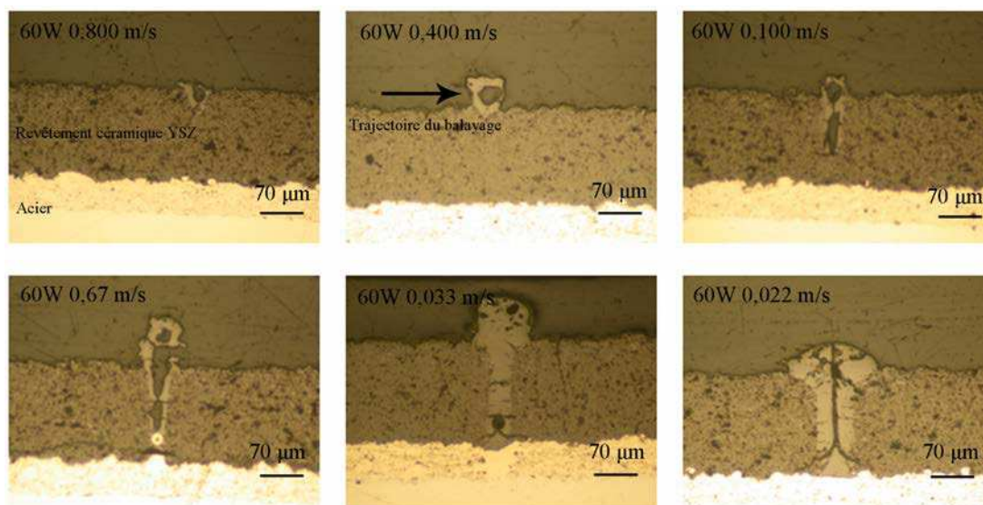
Figure III.40. Section du cordon fait à 60 W avec différentes vitesses de balayage
