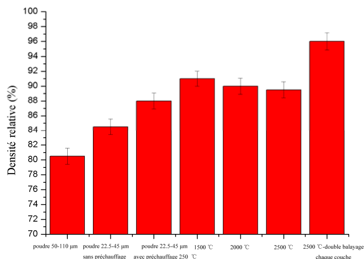
Figure IV.17 Comparaison de densité relative en fonction des paramètres de fabrication
