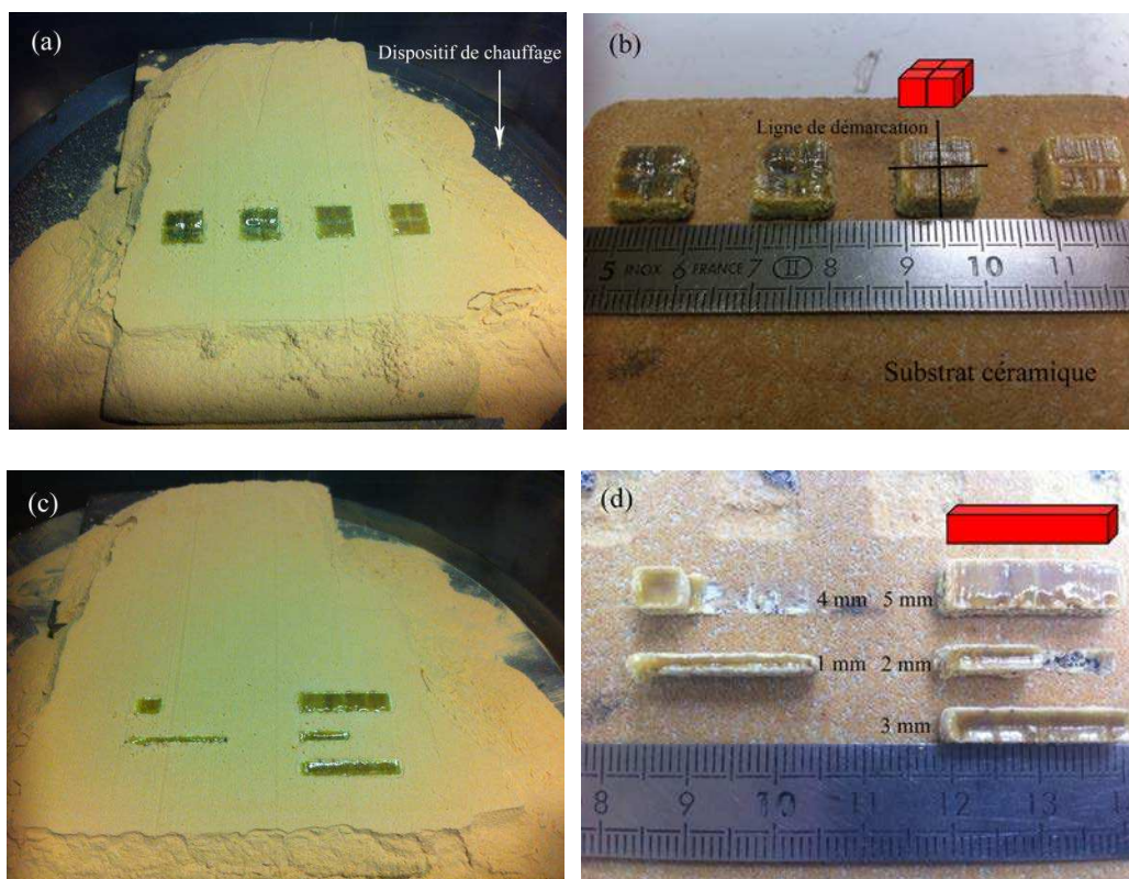
Figure III.34. Photos d'échantillons grandes tailles, (a), (b) modèle d'échantillon 10 mm × 10 mm × 5 mm, (c), (d) modèles d'échantillons 1 mm × 20 mm × 5 mm, 2 mm × 20 mm × 5 mm, 3 mm × 20 mm × 5 mm, 4 mm × 20 mm × 5 mm, 5 mm × 20 mm × 5 mm
