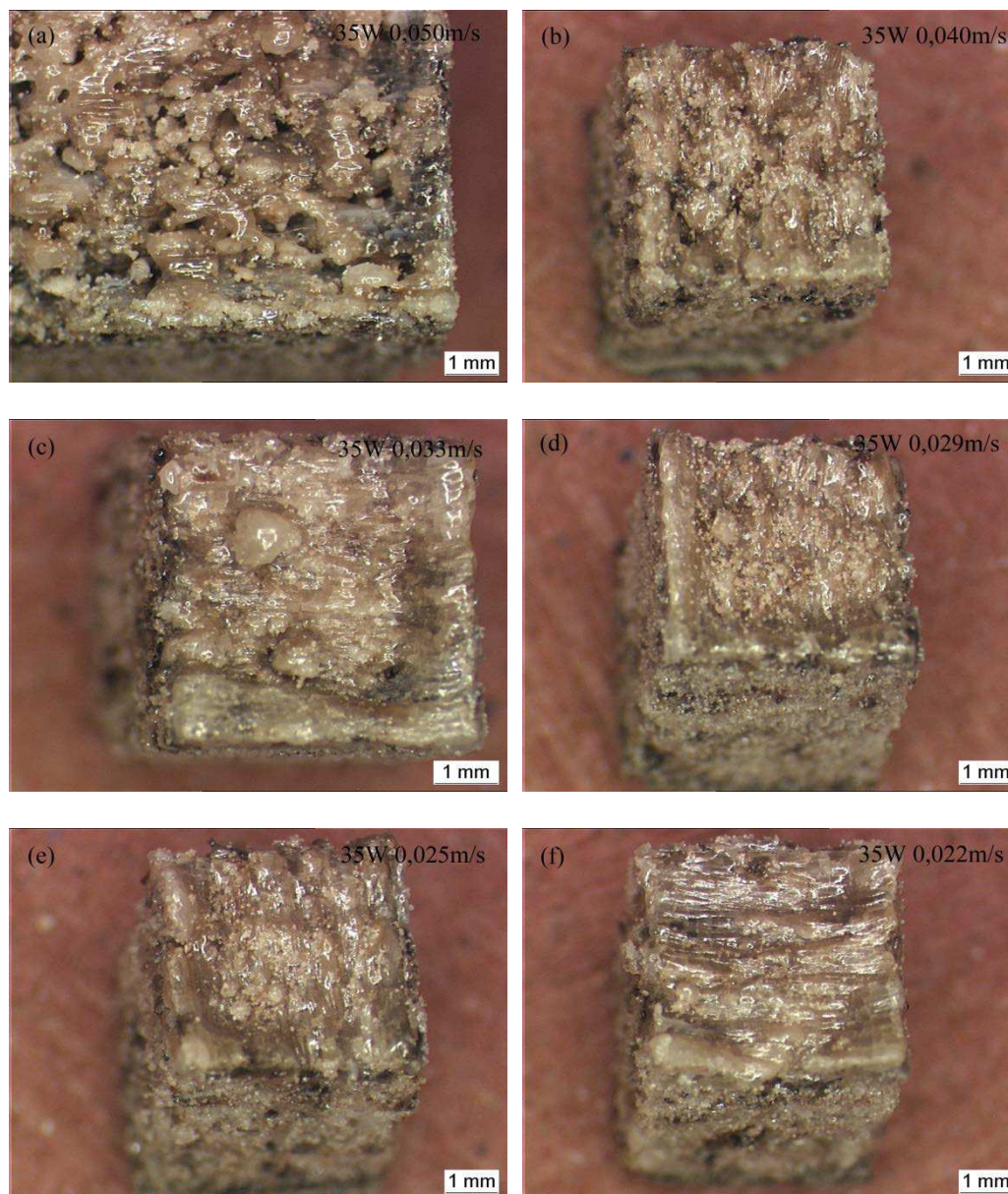
Figure III.8. Photos des échantillons fabriqués par laser puissance 35 W avec différentes vitesses de balayage: (a) 0,050 m/s, (b) 0,040 m/s, (c) 0,033 m/s, (d) 0,029 m/s, (e) 0,025 m/s, (f) 0,022 m/s
