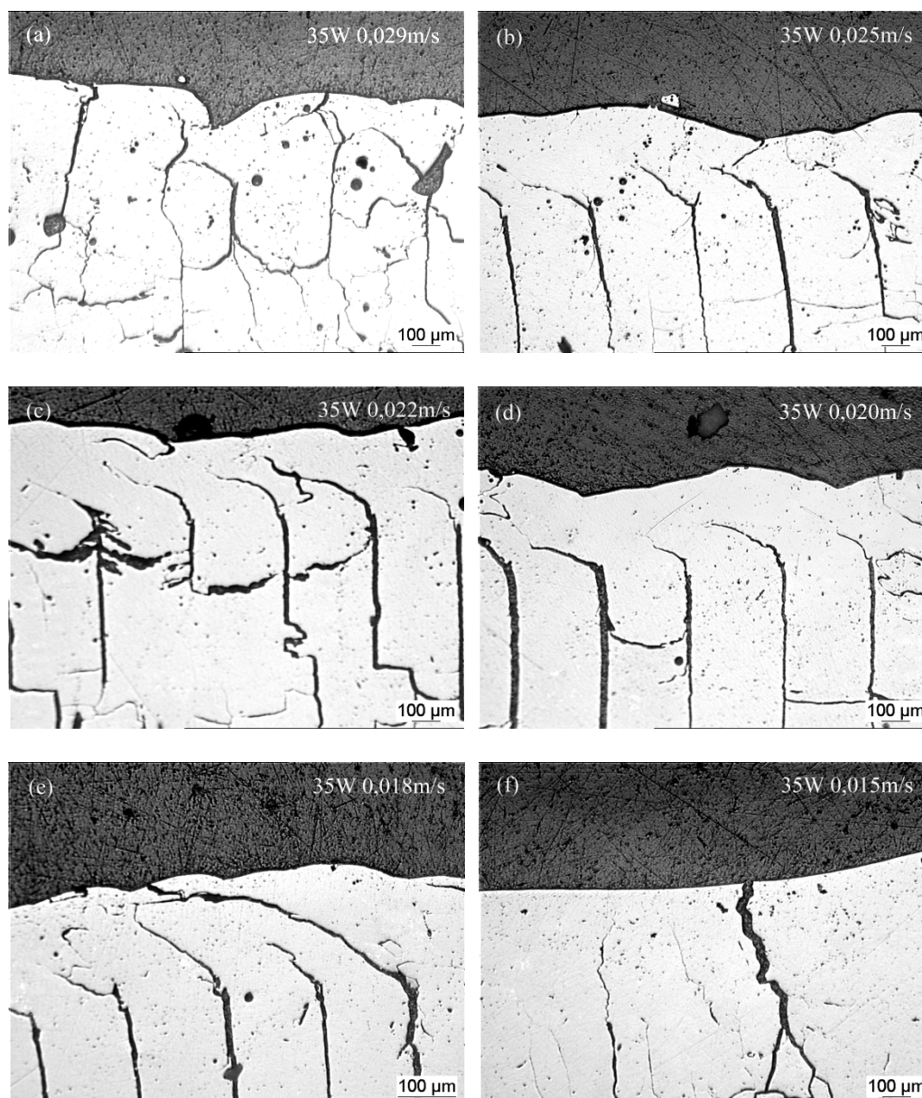
Figure III.18. Microstructure d'échantillon fabriqué par de la poudre fine 22,5-45 μm, (a) 35 W-0,029 m/s, (b) 35 W-0,025 m/s, (c) 35 W-0,022 m/s, (d) 35 W-0,020 m/s, (e) 35 W-0,018 m/s, (f) 35 W-0,015 m/s
