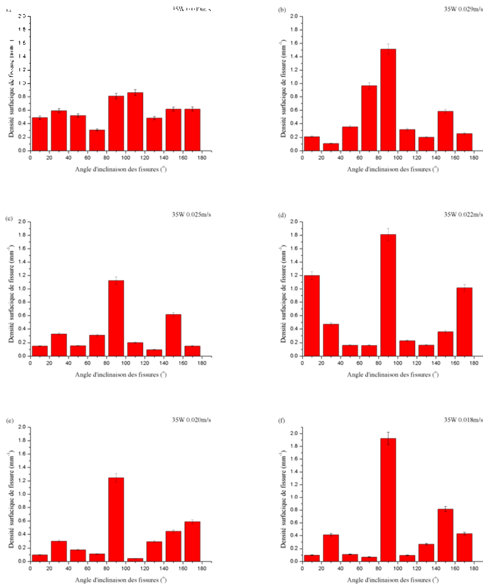
Figure III.19. Distribution des fissures dans la section verticale des échantillons fabriqués avec de la poudre fine 22,5-45 \mu\text{m} , (a) 35 W-0,040 m/s (b) 35 W-0,029 m/s, (c) 35 W-0,025 m/s, (d) 35 W-0,022 m/s, (e) 35 W-0,020 m/s, (f) 35 W-0,018 m/s
