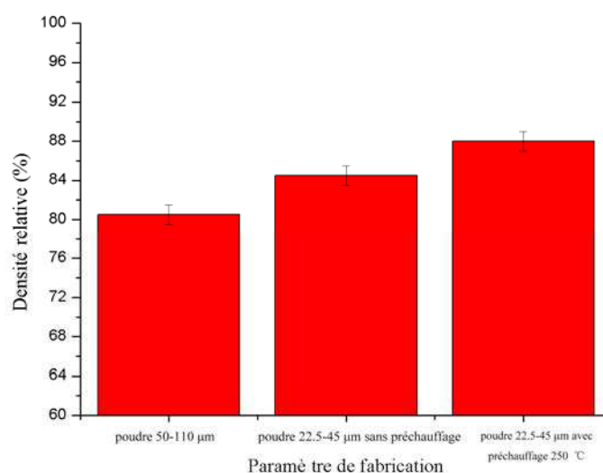
Figure III.32. Comparaison de la densité relative de l'échantillon fabriqué avec des paramètres différents (poudre 55-110 \mu\text{m} , 22,5-45 \mu\text{m} , sans préchauffage et avec préchauffage 250 ^{\circ}\text{C} )
