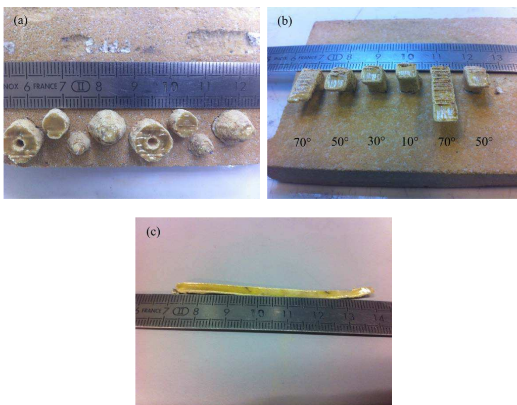
Figure III.35. Photos des échantillons spéciaux : (a) modèle de cône et modèle de colonne, (b) modèles à angles différents 70°, 50°, 60°, 10°, (c) modèle d'échantillon 5 mm × 70 mm × 1 mm
