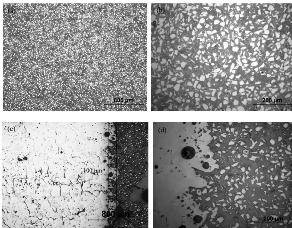
Figure IV.9. (a) (b) microstructure de la poudre préchauffée à 2000 ^{\circ}\text{C} , (c) (d) frontière de l'échantillon
