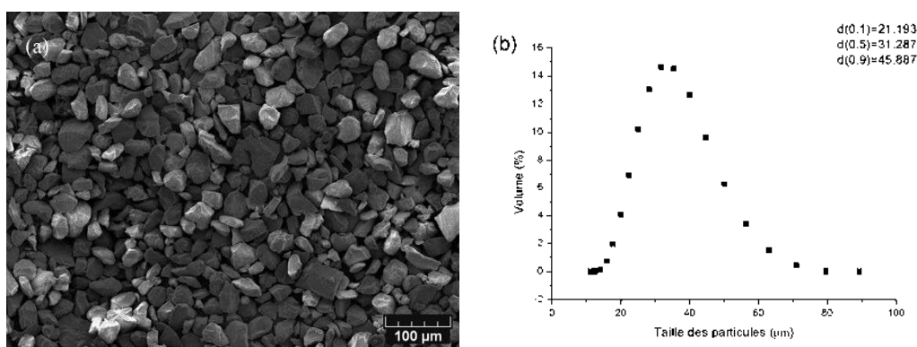
Figure II.2. (a) Image MEB de la poudre YSZ 22,5-45 \mu\text{m} ; (b) Distribution granulométrique de cette même poudre
