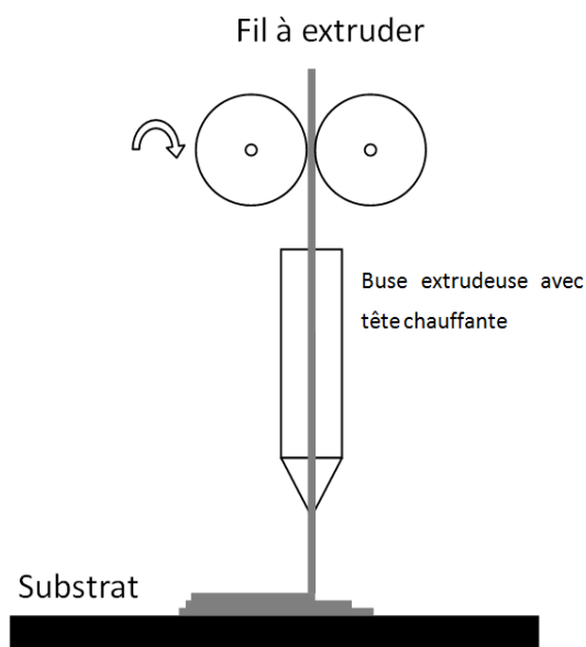
Figure I.9. Procédé de dépôt de filament extrudé
