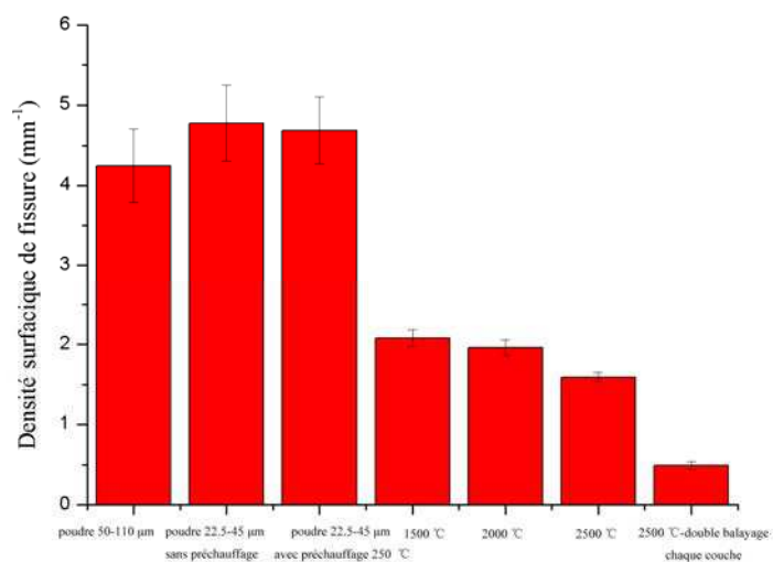
Figure IV.13. Comparaison de la densité surfacique de la fissure en fonction des paramètres de fabrication
