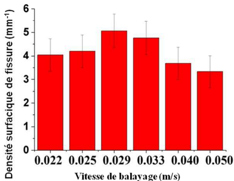
Figure III.13. Relation entre la densité surfacique des fissures et la vitesse de balayage
