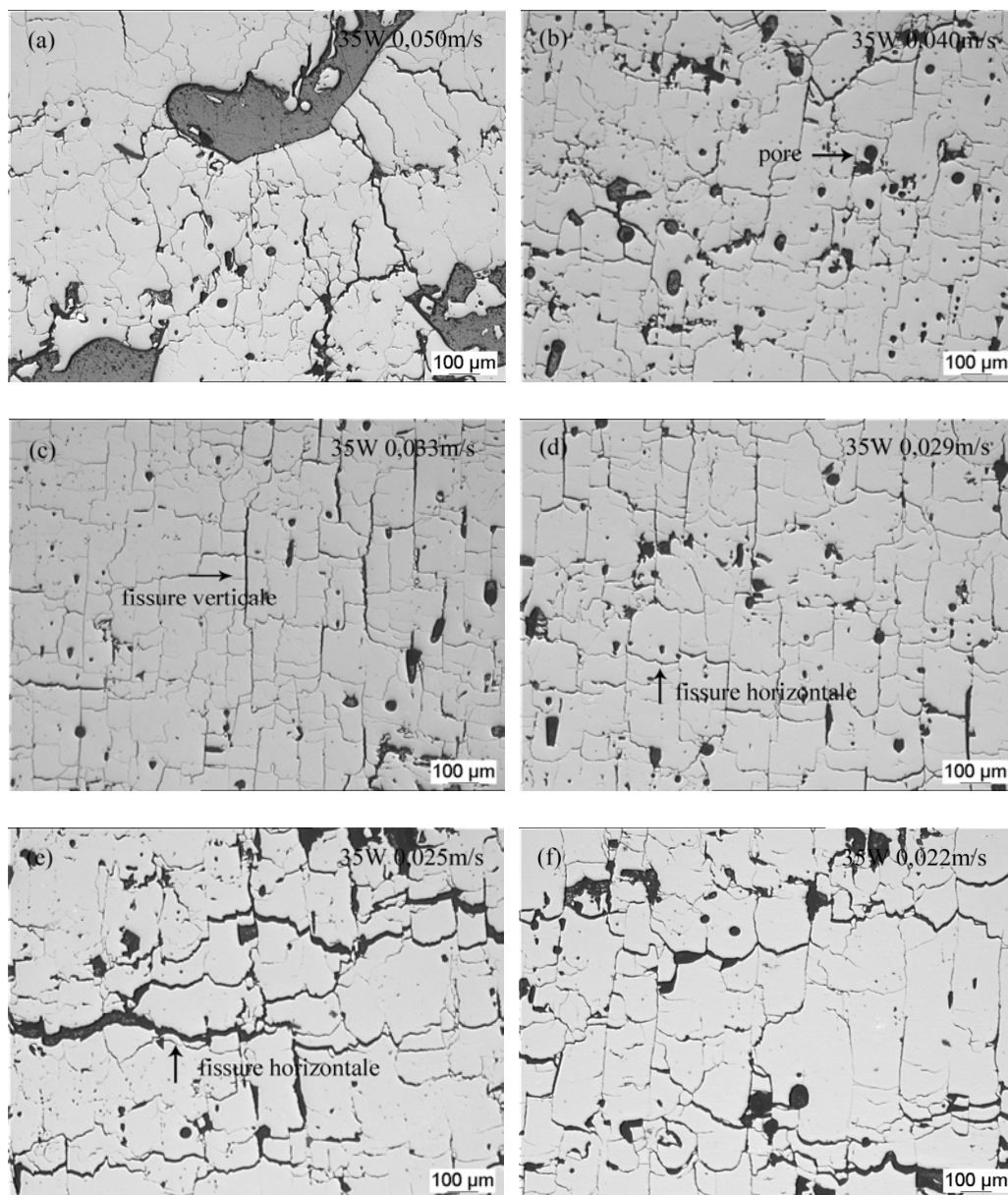
Figure III.10. Microstructures des sections verticales à puissance 35 W avec différentes vitesses de balayage : (a) 0,050 m/s, (b) 0,040 m/s, (c) 0,033 m/s, (d) 0,029 m/s, (e) 0,025 m/s, (f) 0,022 m/s
