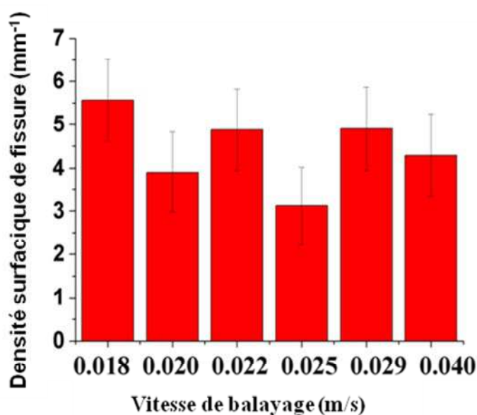
Figure III.20. Relation entre la densité surfacique des fissures et la vitesse de balayage
