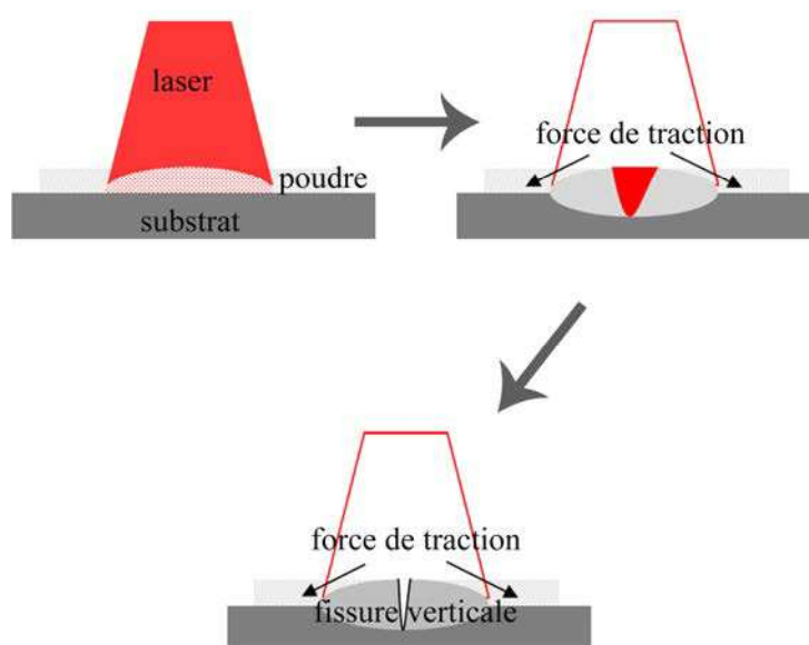
Figure III.42. Schéma de la génération de fissure pendant le refroidissement
