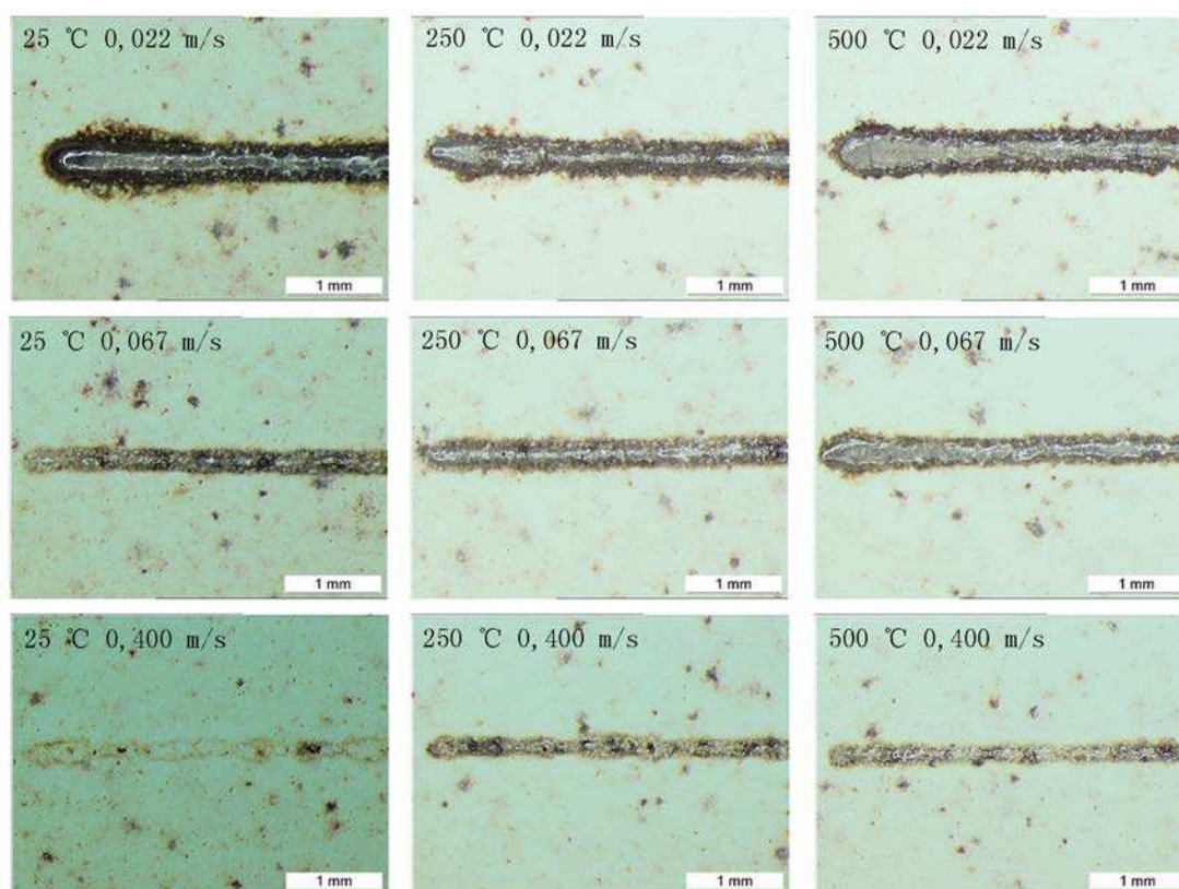
Figure III.36. Cordons fabriqués avec le préchauffage des différentes températures (25 °C, 250 °C et 500 °C) et vitesses de balayage (0,022 m/s, 0,067m/s et 0,400 m/s)
