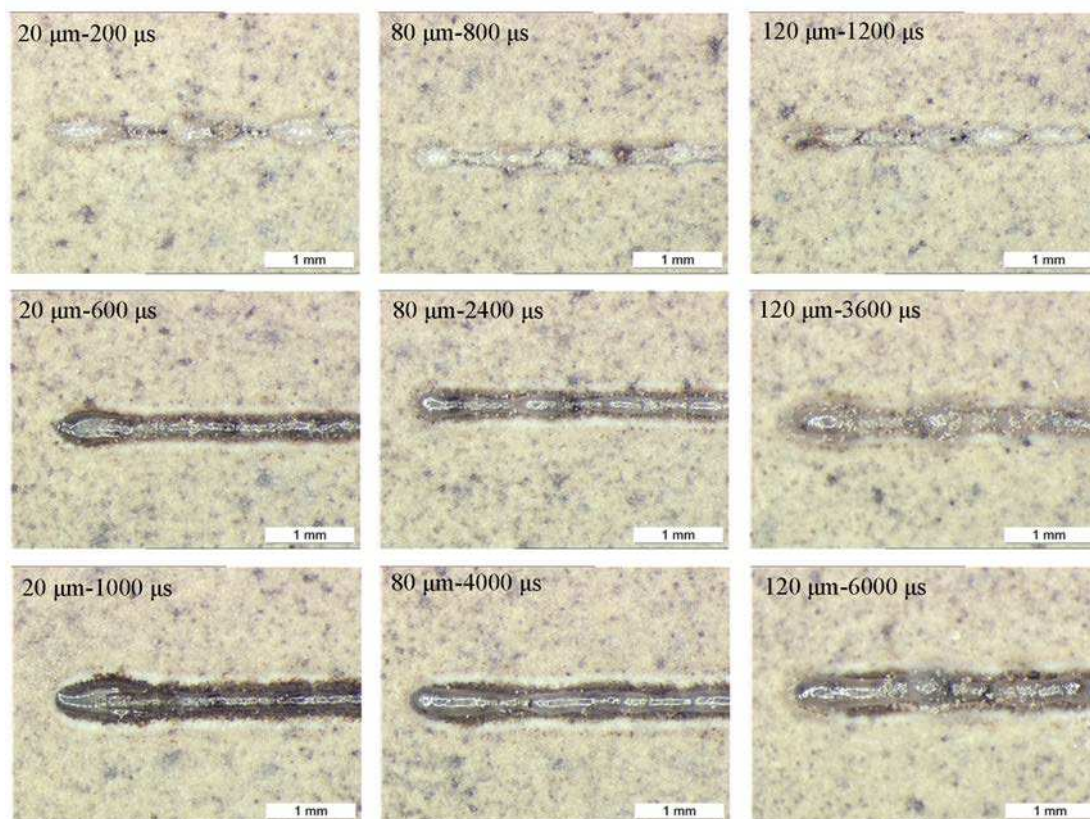
Figure III.38. Cordon fabriqué avec différents points distances et temps d'exposition (même vitesse de balayage) avec le préchauffage 250 °C
