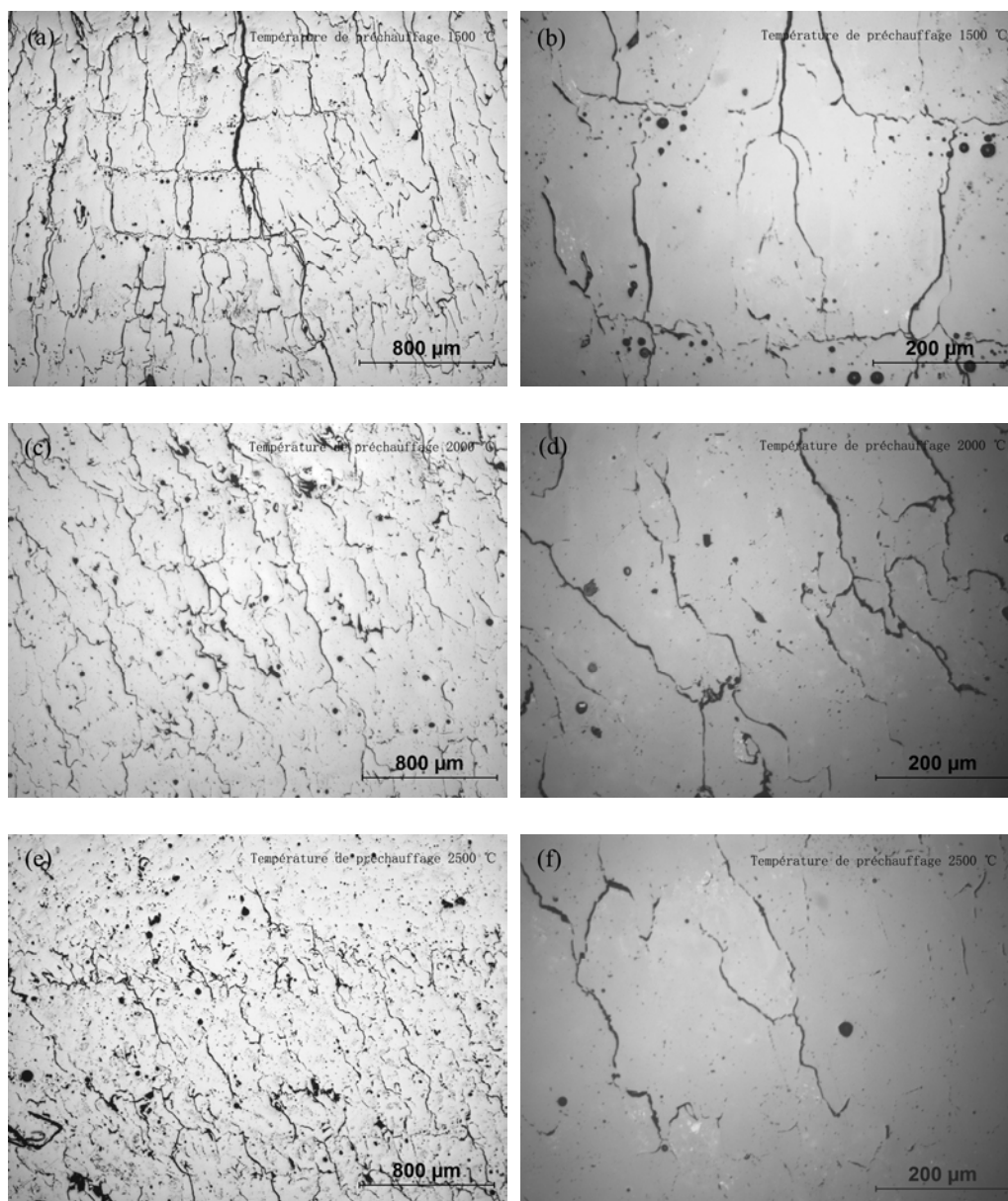
Figure IV.8. Microstructure d'échantillon fait à 60 W avec le préchauffage des différentes températures, (a) (b) 1500 °C, (c) (d) 2000 °C, (e) (f) 2500 °C
