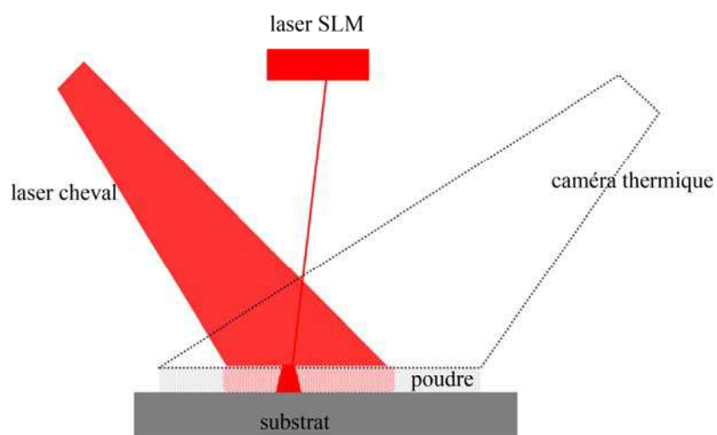
Figure IV. 1. Schéma du préchauffage par laser CHEVAL
