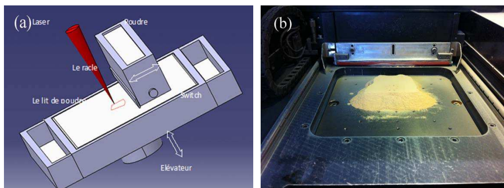
Figure III.1. (a) principe de la machine de fusion sélective par laser MCP REALIZER SLM 250, (b) plate-forme de fabrication
