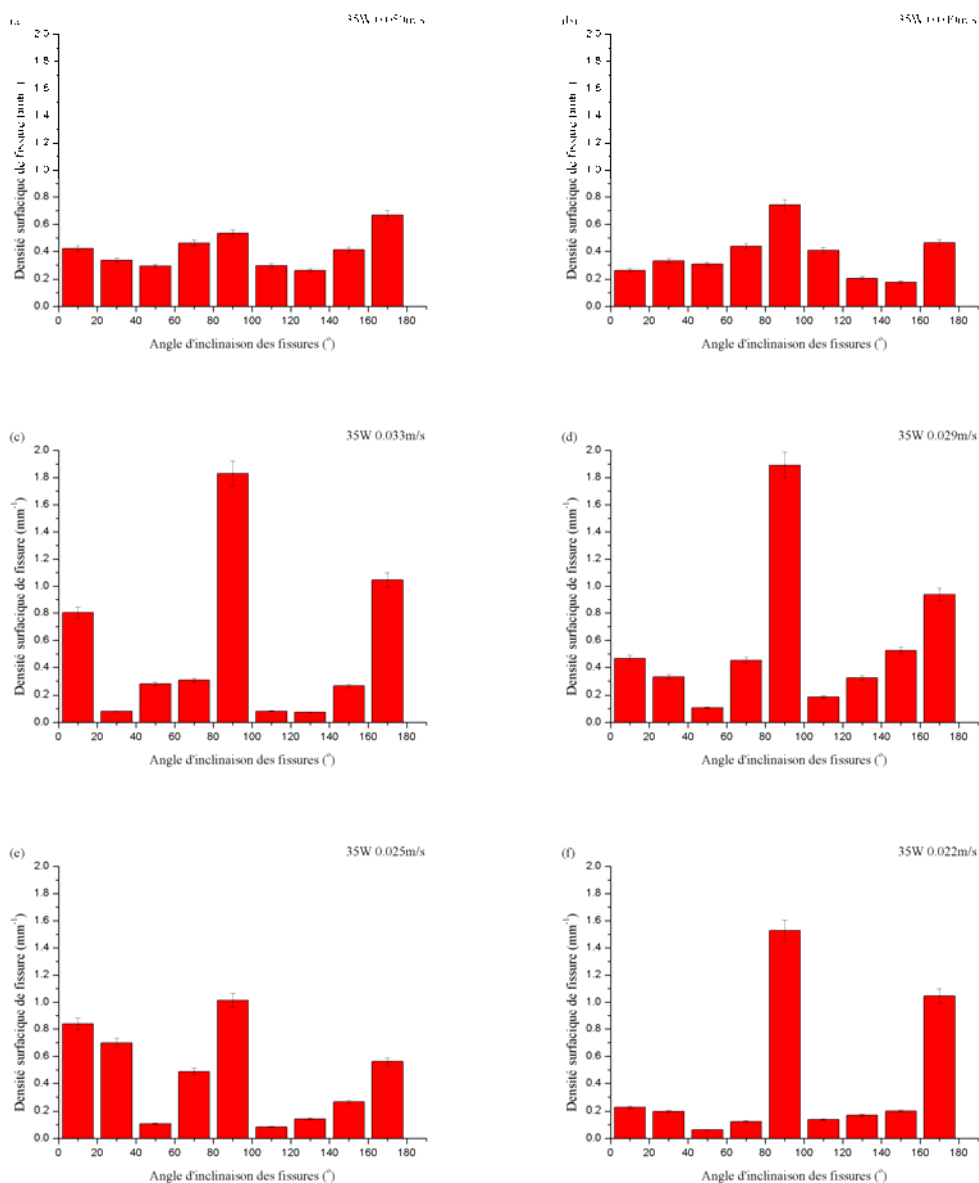
Figure III.12. Distribution des fissures dans la section verticale d'échantillons faits à une puissance de 35 W avec différentes vitesses de balayage : (a) 0,050 m/s, (b) 0,040 m/s, (c) 0,033 m/s, (d) 0,029 m/s, (e) 0,025 m/s, (f) 0,022 m/s
