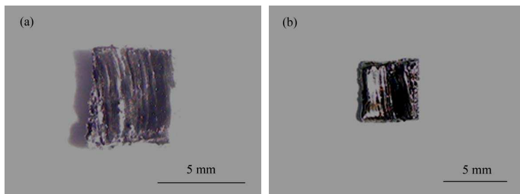
Figure III. 7. Fabrication initiale de la céramique de YSZ, (a) 70 W, (b) 90 W
