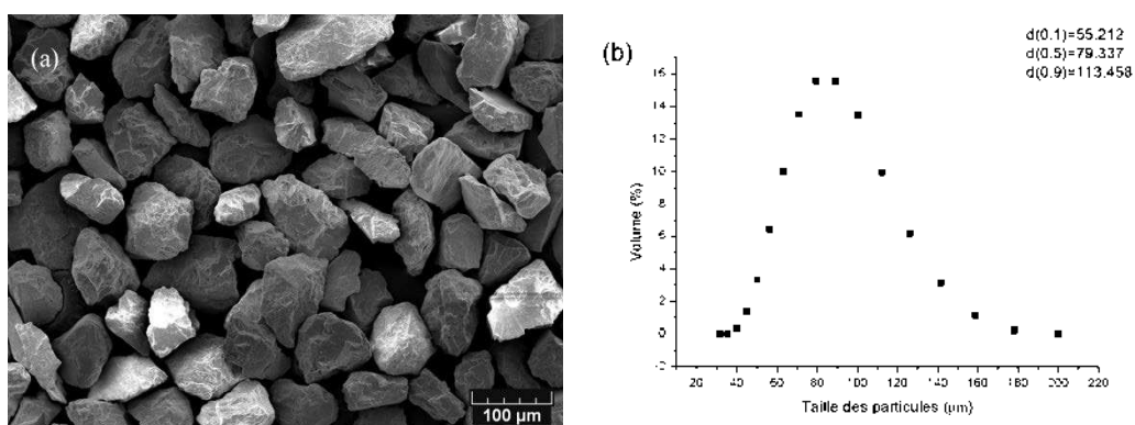
Figure II.3. (a) Image MEB de la poudre YSZ 55-110 \mu\text{m} ; (b) Distribution granulométrique de cette même poudre
