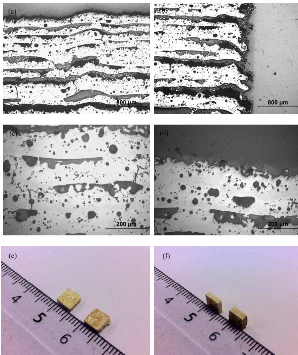
Figure IV.10. (a) (b) (c) (d) : microstructures sectionnelles d'échantillon fabriqué par laser de densité d'énergie faible (puissance 30 W et vitesse de balayage 4 m/s) avec préchauffage à 2500 °C, (e) (f) : photo de la surface et du côté de l'échantillon fait à 30 W et la vitesse de balayage 4 m/s, avec préchauffage à 2500 °C
