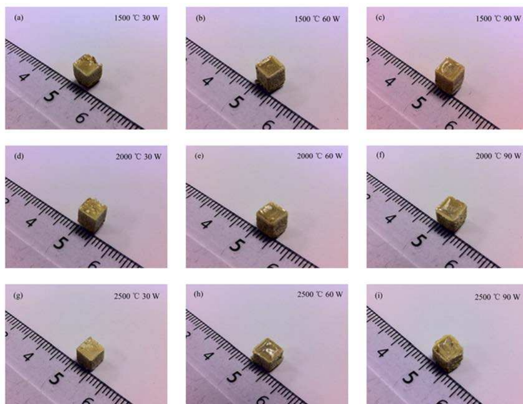
Figure IV.7. Echantillon cubique avec différentes températures de préchauffage (1500 °C, 2000 °C et 2500 °C) et puissance de laser (30 W, 60 W et 90 W)
