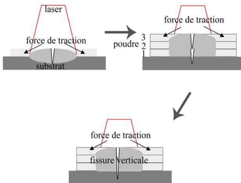
Figure III.43. Schéma de la génération de fissure traversante
