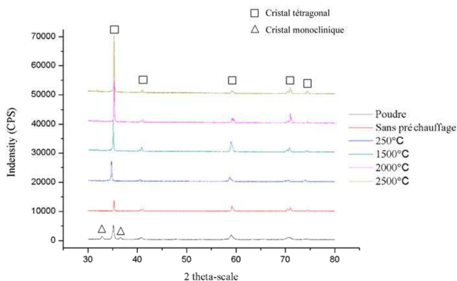
Figure IV.18. Diagramme de diffraction de rayons X de la poudre YSZ et des échantillons faits à différentes température de préchauffage : 250 °C, 1500 °C, 2000 °C et 2500 °C
