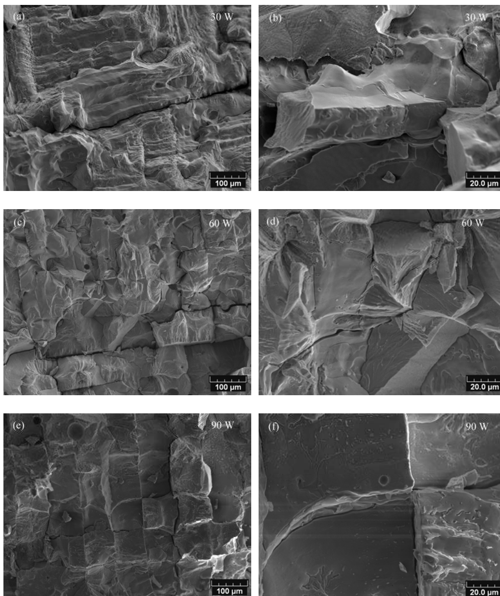
Figure III.28. Morphologie de la surface de fracture des échantillons faits avec différentes puissances : 30 W, 60 W, et 90 W
