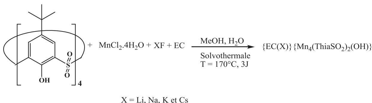
Figure II.28: Synthèses des composés (6), (7), (8) et (9).
