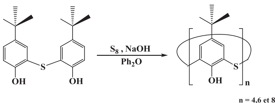
Figure I.2: Synthèse du p-tert -butylthiacalix[n]arène.
