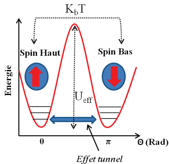
Figure I.26: Puits de potentiel représentant les différents états d'énergie ms. représentation des deux chemins pour le retournement des spins.
