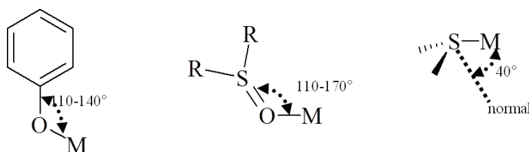
Figure I.17: Orientations typiques de la liaison métal-ligand (ligand : phénolate, sulfoxyde et thioéther) [64].
