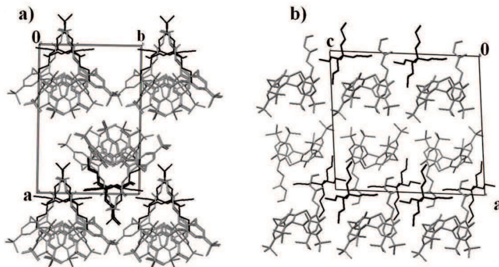
Figure IV.5: Empilement du composé ( T7B ). a) selon l'axe c , b) selon l'axe b . Le tétrabutylammonium est représenté en trait noir.
