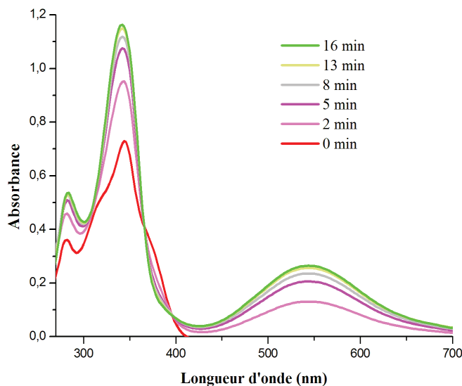
Figure III.18: Evolution du spectre d'absorption UV-visible d'une solution de ThiaSO 2 [ 4,5 \cdot 10^{-5} M ] et de Mn(NO 3 ) 2 [ 4,2 \cdot 10^{-5} M ] dans la DMF en fonction du temps d'illumination à 400 nm.
