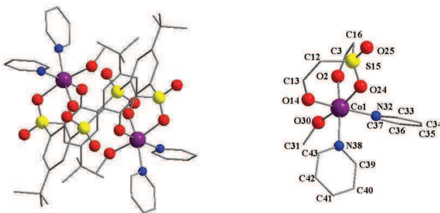
Figure V.24: Structure moléculaire de (16) et représentation de l'environnement de l'ion cobalt.
