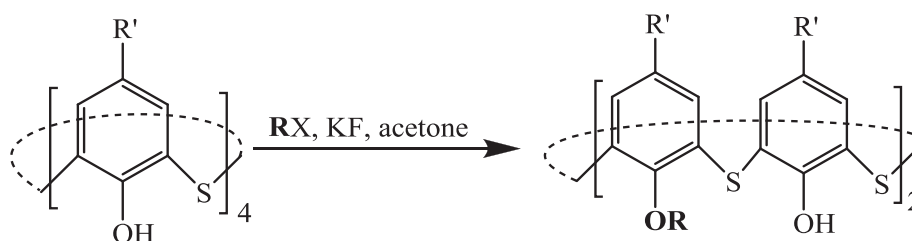
Figure IV.1: Synthèse des thiacalixarène di-substitué (T1-T6).
