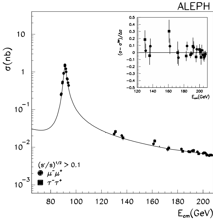
FIG. 4.6 – Sections efficaces inclusives pour les événements di-muons (points) et di-taus (carrés) en fonction de l'énergie dans le centre de masse [67]. Les courbes donnent les prédictions obtenues par ZFITTER [67]. L'encart présente la différence entre les mesures et les prédictions du Modèle Standard normalisées aux sections efficaces prédites. Pour les points en-dessous de 189 GeV, les résultats sont présentés dans la référence [69].
