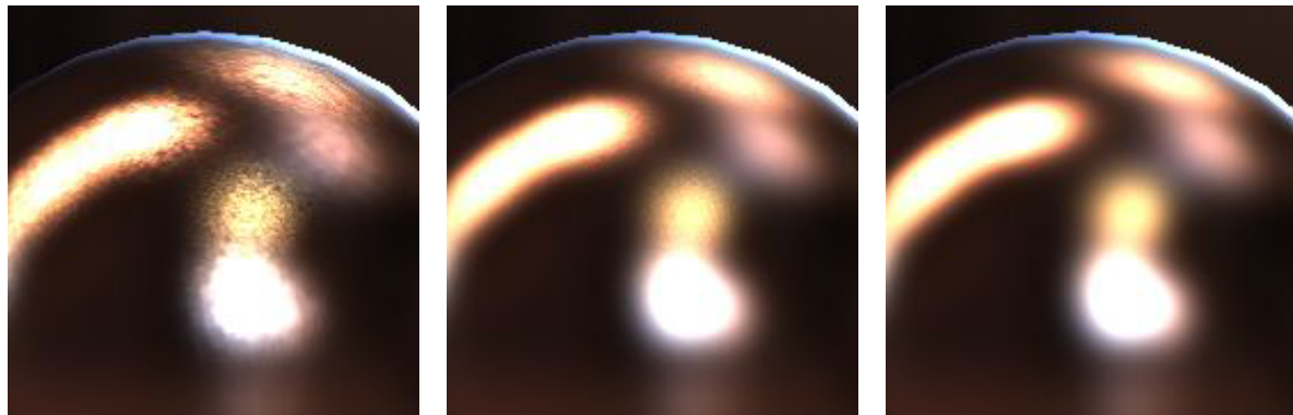
Mersenne twister
