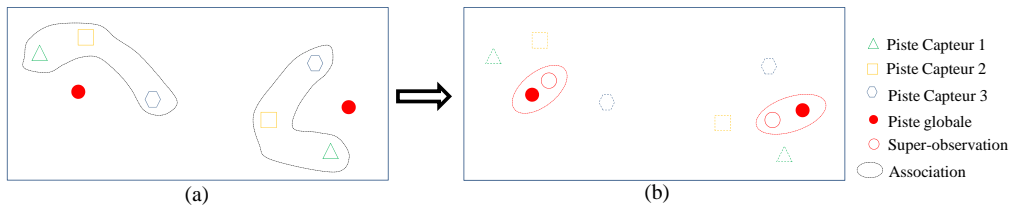
Figure 3.8: Les pistes locales des capteurs sont d'abord associées entre elles (a) pour former des super-observations qui sont ensuite associées avec les pistes globales du système (b)
