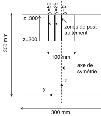
Figure 11.20 – Zones de posttraitement dans le béton, à l'interface
