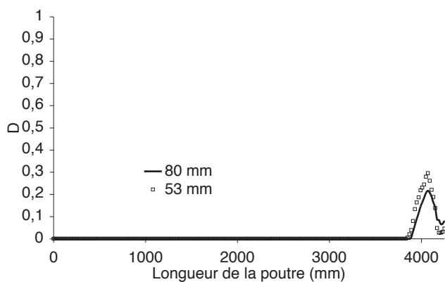
(b) Distribution de l'endommagement ( D ) à 478 KN en fonction de la longueur caractéristique.
