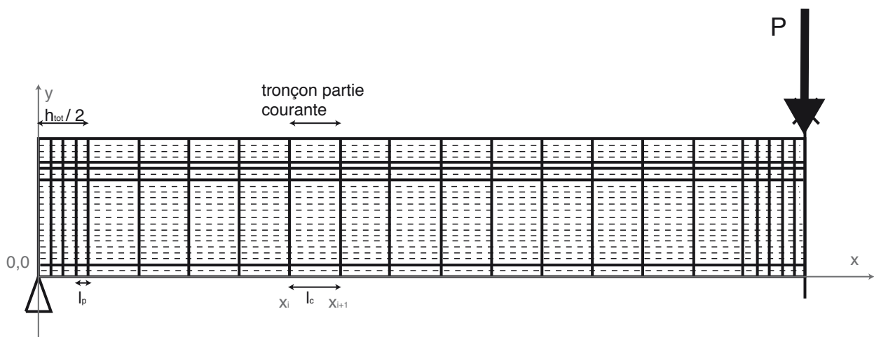
Figure 15.3 – Maillage de la poutre : discrétisation longitudinale
