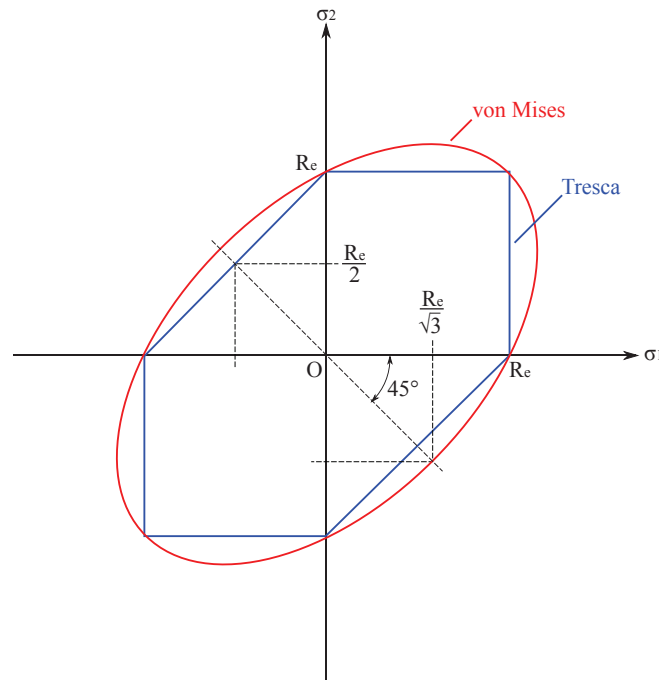
Figure 5.5 – Tracé du critère de Tresca et de Von Mises dans le plan des contraintes principales \sigma_1 \sigma_2
