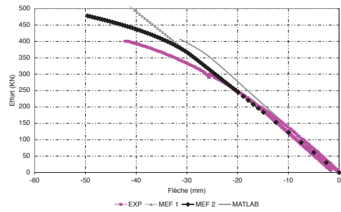
(d) AB4 Section Centrale
