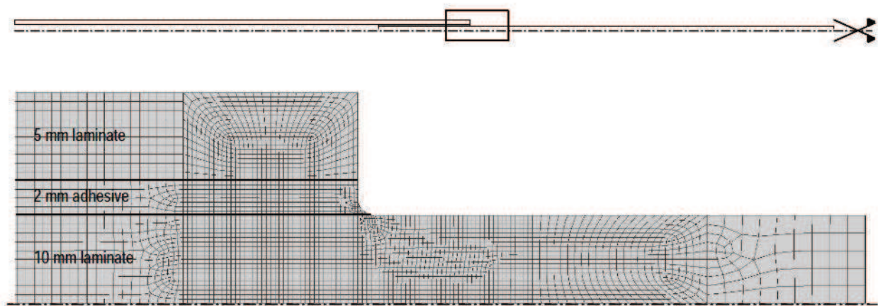
Figure 10.1 – Maillage joint à double recouvrement en 2D (De Castro San Roman, 2005)
