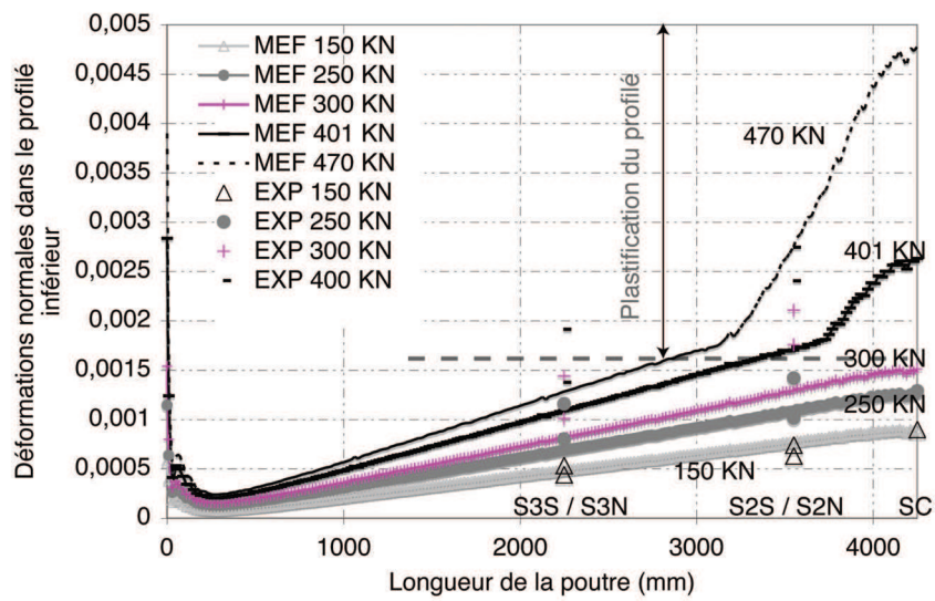
(c) Evolution le long de la poutre des déformations dans le profilé : semelle inférieure
