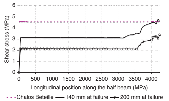
(d) AB4 à 400 kN
