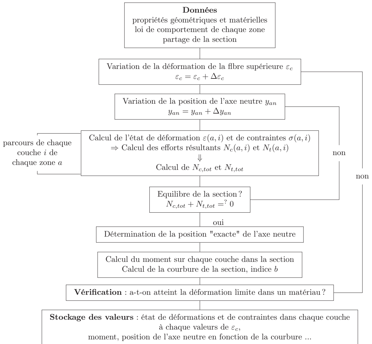
Figure 15.7 – Organigramme 1 : détermination de la loi moment courbure d’une section multicouche
