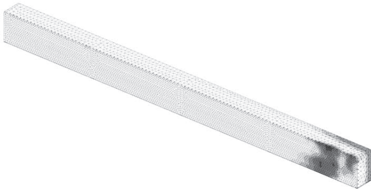
(b) 95 % F_u et D_{max} = 0,71
