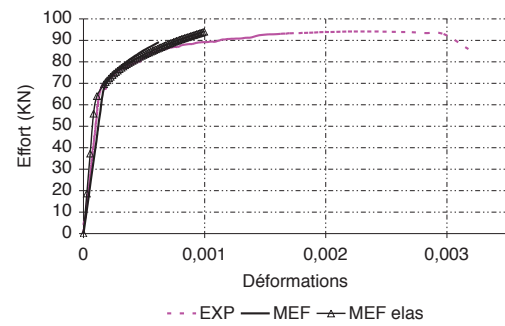
(b) Béton : dalle inférieure
