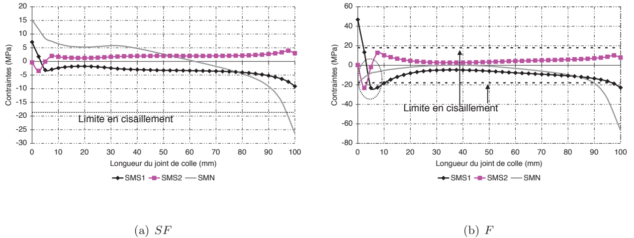
Figure 11.53 – Distribution des contraintes tangentielles dans le joint de colle aux charges de ruine numériques dans le cas avec ou sans frottement
