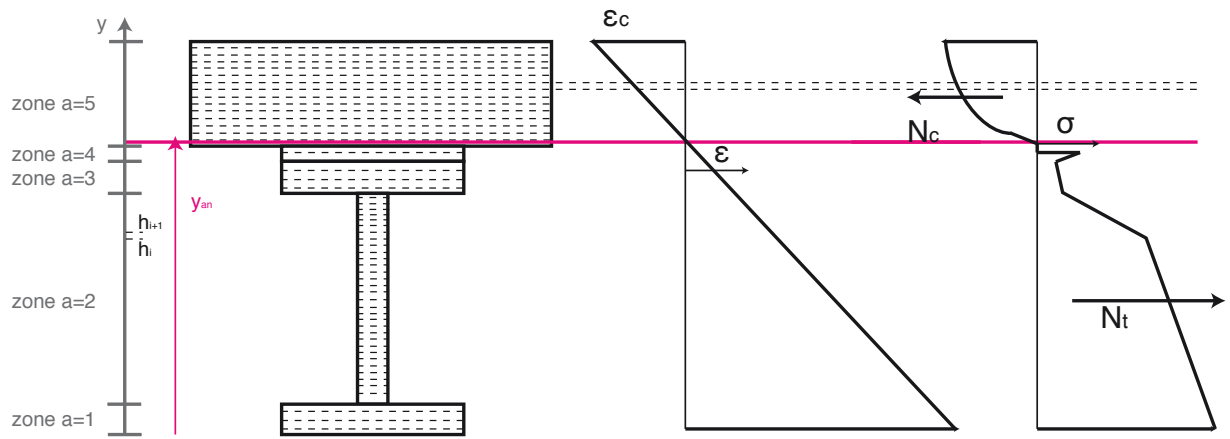
Figure 15.5 – Comportement d'une section multicouche
