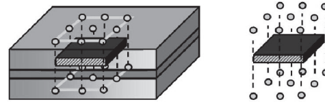
Figure 10.3 – Element fini 3D de l'adhésif (Dillard et al., 2001)
