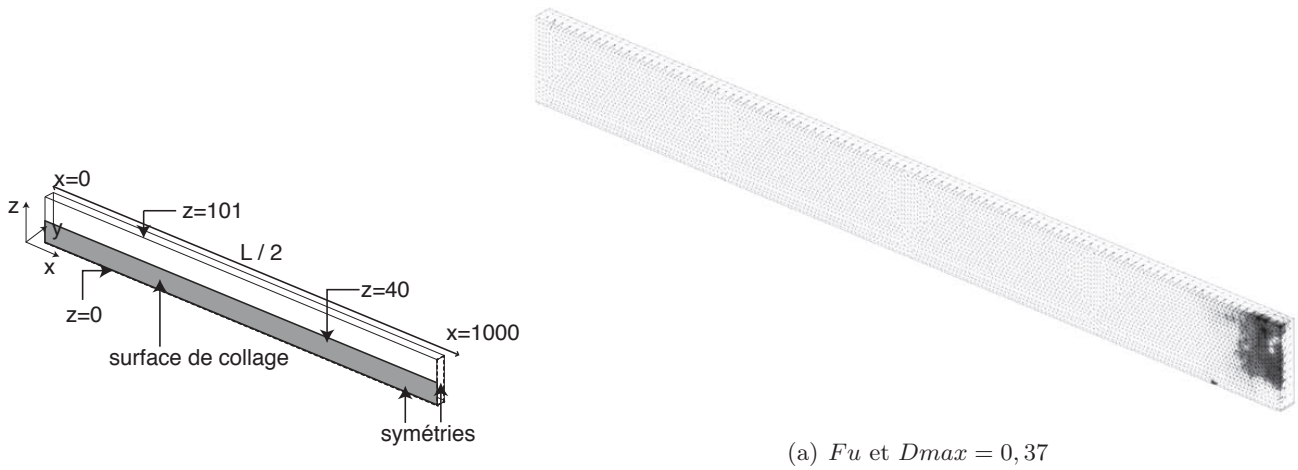
Figure 16.25 – Distribution de l'endommagement pour la poutre AB3
