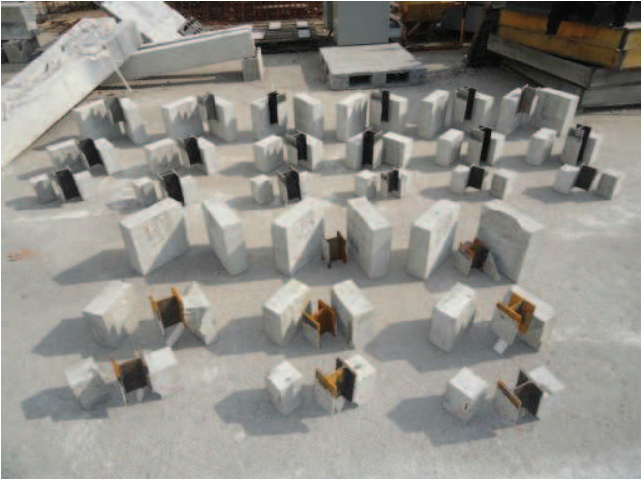
Figure 9.8 – Eprouvettes PO1 , PO2 et PO3 cassées.
