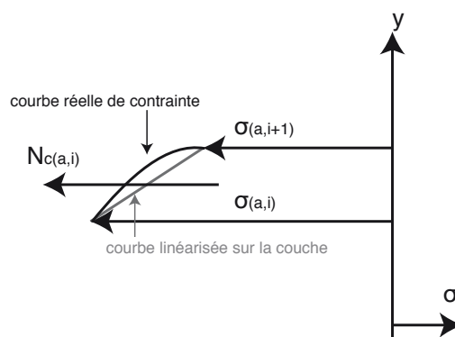
Figure 15.6 – Etat de contrainte sur une couche i . ( \sigma correspond aux contraintes normales, N_c(a, i) aux efforts normaux de compression ici)
