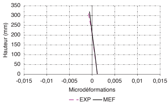
(a) AB1 , section sud, à F_u
