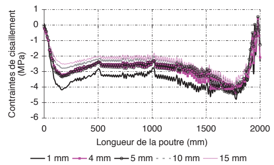
(b) Distribution des contraintes de cisaillement à l'interface
