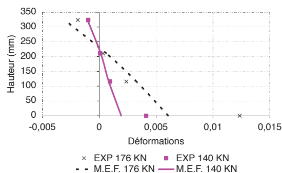
(d) AB2 , section centrale
