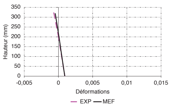
(c) AB2 , section sud à 140 KN
