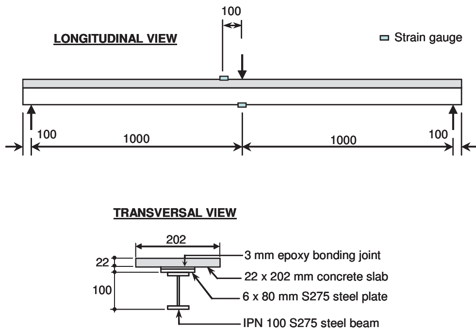
Figure 14.4 – Géométrie de la poutre testée par (Jurkiewicz et al., 2008) et notée AB3
