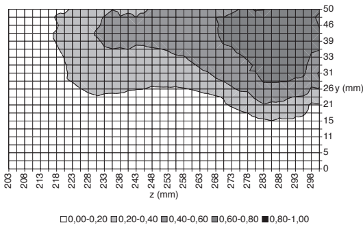
(c) Modèle d'endommagement plastique, modèle NON LOCAL, à 113 kN
