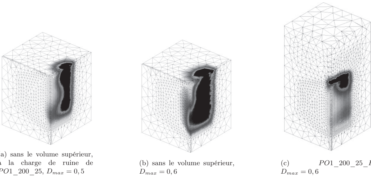
Figure 11.52 – Endommagement à la ruine pour PO1\_200\_25 avec frottement : 2 cas sont comparés : avec ou sans le volume supérieur de béton permettant d’avoir une hauteur de 200\text{ mm} comme pour PO1\_200 , les zones noires correspondent aux zones les plus endommagées
