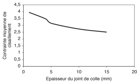
(c) Influence de l'épaisseur de la connexion sur la contrainte moyenne de cisaillement dans le joint de colle
