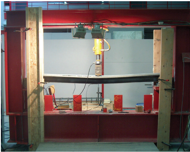
(a) Rupture par rotule plastique
