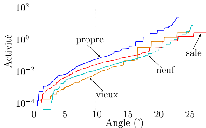
FIGURE 5.3 – Dynamique des réarrangements pour des empilements de billes de taille 30 \times 19 \times 3 \text{ cm}^3 avec différents états de surface : vieux, neuf, propre, et sale.
