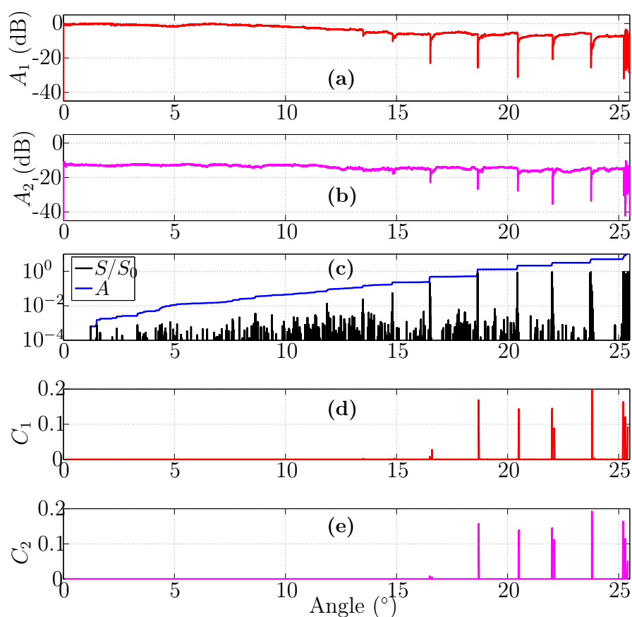
FIGURE 4.5 – Sondage acoustique non linéaire. (a-b) Amplitudes de la composante fondamentale démodulée ( A_1 ) et de sa seconde harmonique ( A_2 ) au cours de l'inclinaison. (c) Dynamique des réarrangements à la surface. (d-e) Coefficients de corrélation entre les amplitudes acoustiques et optiques pour les deux composantes démodulées ( C_1 et C_2 ).
