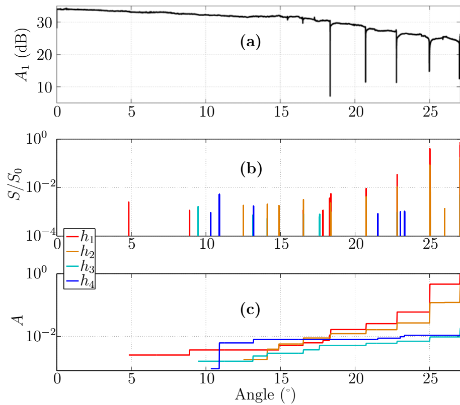
FIGURE C.2 – Détection des réarrangements lors de l’inclinaison d’un empilement de billes de 2 mm de diamètre jusqu’à avalanche. (a) Sondage du volume par méthode acoustique non linéaire en suivant la composante démodulée A_1 . (b) Fraction de surface réarrangée S/S_0 et (c) activité A mesurées sur une des faces latérales à l’arrière d’un transducteur pour 4 zones h suivant la profondeur définies dans la figure C.1.
