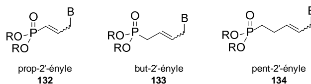
Figure 28. ANPs oléfiniques préalablement étudiés au laboratoire.
