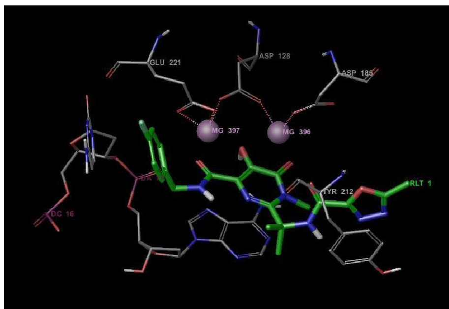
Figure 69. Interaction Raltégravir/Intégrase/ADN Chélation avec Mg396 et Mg397 avec comme partenaires de la protéine : Asp185, Asp128 et Glu221. \pi stacking entre le cycle oxo diazole et la Tyr212, \pi stacking entre le p -fluorobenzyl et DC16 \pi stacking entre le cycle central et DA17
