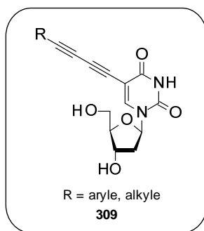
Figure 53. Structure cible portant un motif C 5 -(1,3-diyne).
