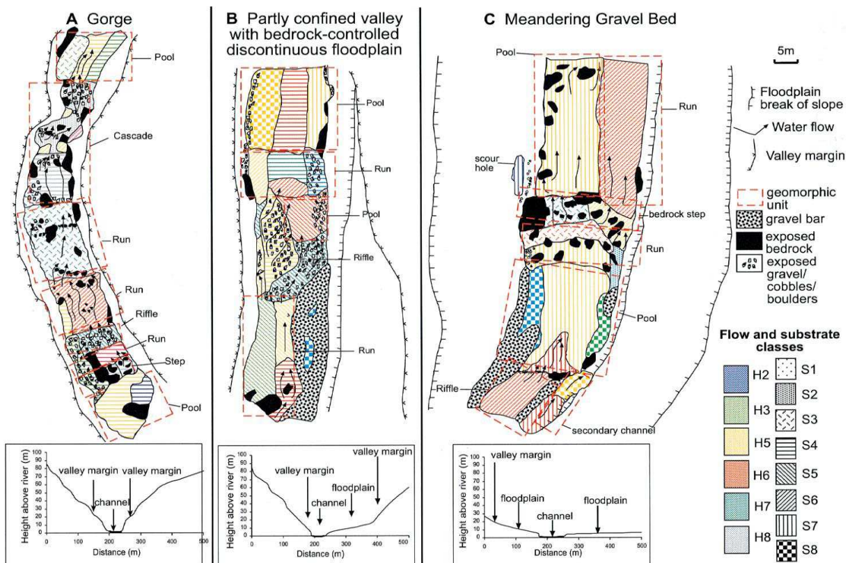
Figure I.4 Cartographie des unités géomorphiques et hydrauliques pour les tronçons représentatifs de trois types de rivières. Le type de rivière de gorge est illustré par un tronçon de la rivière Kerripit ( 31^{\circ}59'55''\text{S} , 151^{\circ}40'15''\text{E} ), située dans une vallée confinée (A). (B) Un exemple du type de rivière de vallée en partie confinée avec zone inondable discontinue contrôlée par la roche mère provenant de la rivière Gloucester ( 32^{\circ}03'10''\text{S} , 151^{\circ}41'20''\text{E} ). Un exemple de type de rivière à lit méandrique graveleux provenant de la rivière Cobark ( 31^{\circ}57'\text{S} , 151^{\circ}42'30''\text{E} ) est présenté en (C). Classes de substrat : S1=100 % de roche mère ; S2=>80 % de roche mère ; S3=30–60 % de roche mère, mélangé avec des galets et des cailloux ; S4=principalement des rochers et des galets ; S5=>60 % de galets ; S6=surtout mélange de galets et de cailloux ; S7=même mélange de galets, cailloux et graviers ; S8=cailloux, de gravier et de sable. Notez les classes de substrat utilisées ici sont tirées des données recueillies dans le bassin versant Manning, et ne sont pas conçues comme des classes génériques. Classes de types d'écoulement de surface : H2=courant à peine perceptible ; H3=faible courant de surface ; H5=ondulations ; H6=ondes stationnaires ininterrompues ; H7=ondes stationnaires interrompues ; H8=cascades. (d'après Thomson et al. , 2001)
