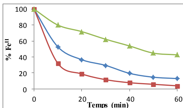
Figure III.48 : Autoxydation de \text{Fe}^{2+} (concentration initiale = 100 \mu\text{M} ) en absence ou en présence de rutine (1 équiv.) et de SAB (1 équiv.) dans le tampon acétate (pH 6, 5 mM phosphate, 25^\circ\text{C} ). ■ \text{Fe}^{\text{II}} - SAB, ◆ \text{Fe}^{\text{II}} - rutine, ▲ \text{Fe}^{\text{II}}
