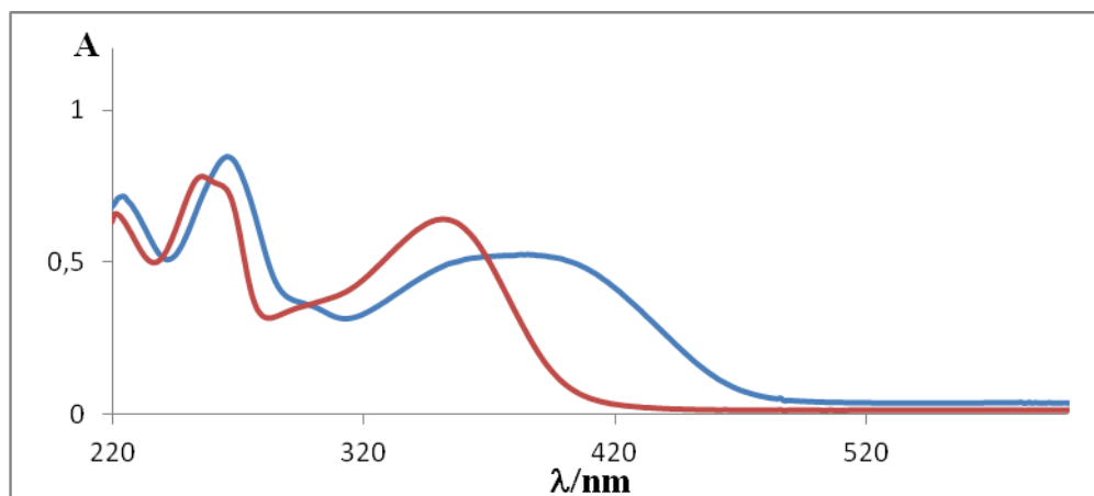
Figure III.8: Complexation de la rutine (50 μM) par Al III (5 équiv.) dans le tampon acétate (0.1M, pH 5, 25°C). — Rutine, — Rutine-Al 3+
