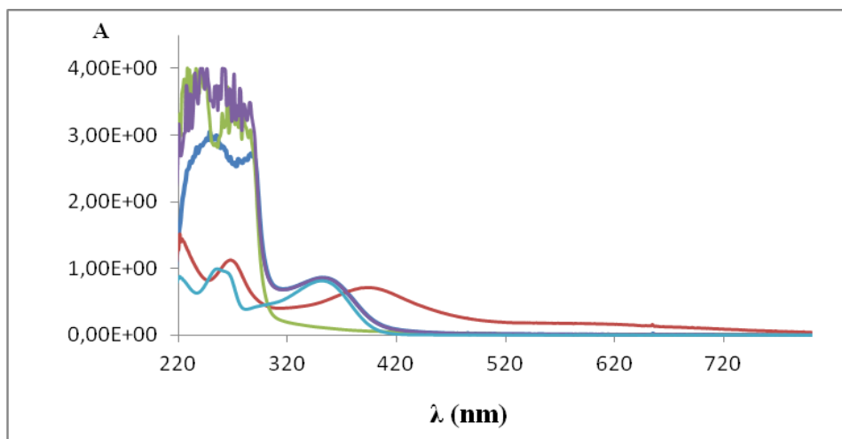
Figure III.19: Interaction de la rutine (50 µM) avec Fe 3+ (1 equiv.) en présence et en absence de la protéine SAB (3 equiv.) dans le tampon acétate (pH 5, 25°C). — Rutine, — SAB (250 µM), — Rutine - Fe 3+ , — Rutine - SAB - Fe 3+
