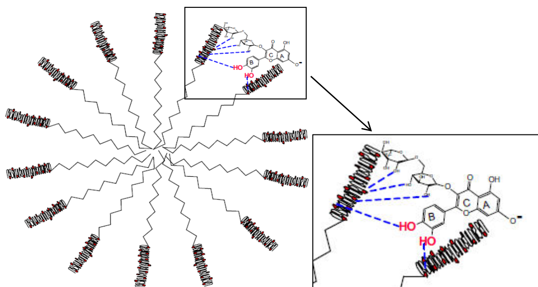
Figure II.12: Positionnement du DPPH• dans une micelle de Brij 35
