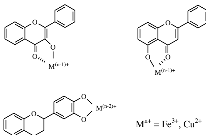
Figure 21: Sites de chélation des ions métalliques par les flavonoïdes [92]
