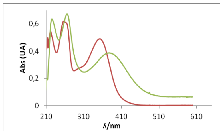
Figure III.20: Interaction de la rutine (50 µM) avec Fe 2+ (1 equiv.) dans le tampon acétate (pH 5, 25°C) après 3h. — Rutine, — Rutine - Fe 2+
