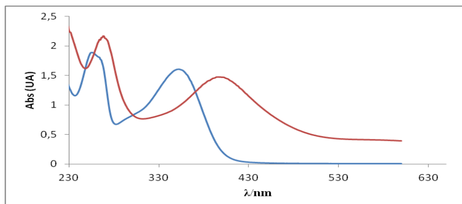
Figure III.12: Complexation de la rutine (50 \mu\text{M} ) par 1 equiv. de \text{Fe}^{3+} dans le tampon acétate (pH 5, 25°C). — Rutine, — Rutine - \text{Fe}^{3+}
