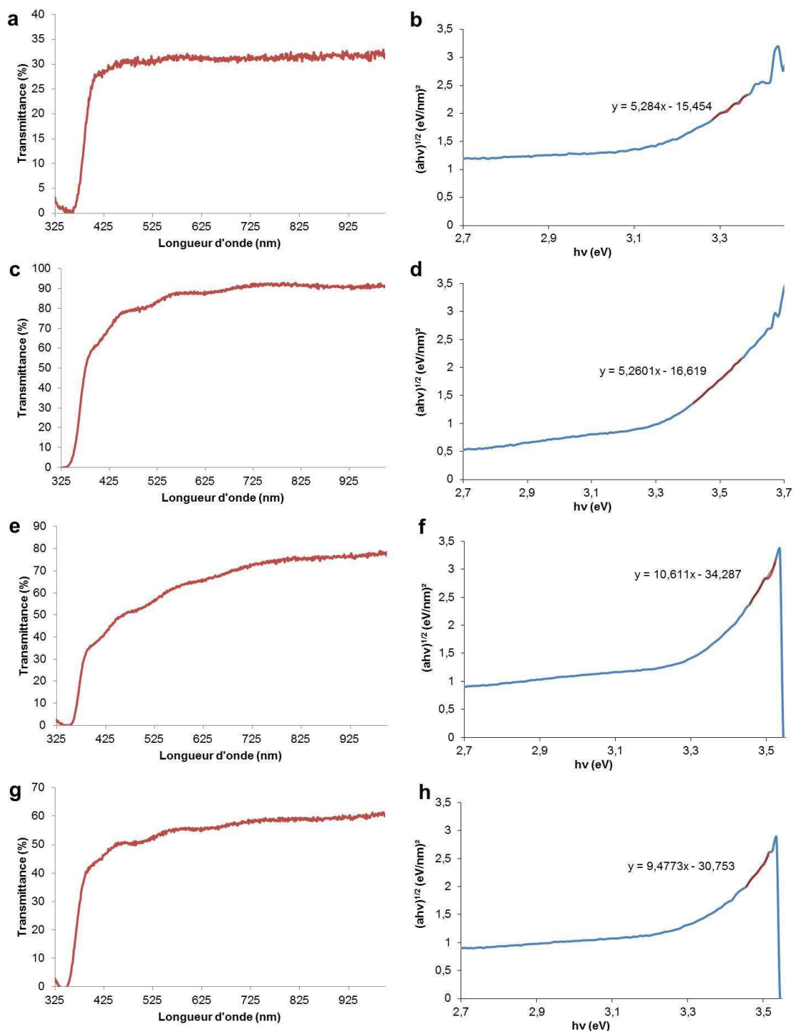
Figure III-25: Spectres de transmission optique et détermination de l'énergie de la bande interdite de films de \text{TiO}_2 formés à partir des poudres A (hydrolyse de \text{TiOSO}_4 à 0,05 M par \text{H}_2\text{O}_2 à température ambiante et traitement thermique à 500 °C) (a et b), poudres B (voie hydrothermale à 200 °C à partir de \text{TiCl}_4 à 1 M) (c et d), poudres C (voie hydrothermale à 200 °C à partir de \text{TiOSO}_4 à 2,5 M (e et f) et poudres D (voie hydrothermale à 200 °C à partir de \text{TiOSO}_4 à 0,4 M) (g et h).
