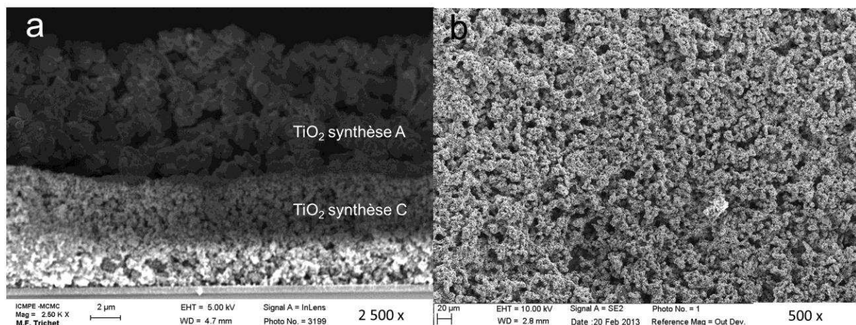
Figure III-7: Clichés MEB de la section (a) et de la surface (b) d'un dépôt de deux couches de \text{TiO}_2 issu de la synthèse A et de la synthèse C de granulométrie différente.
