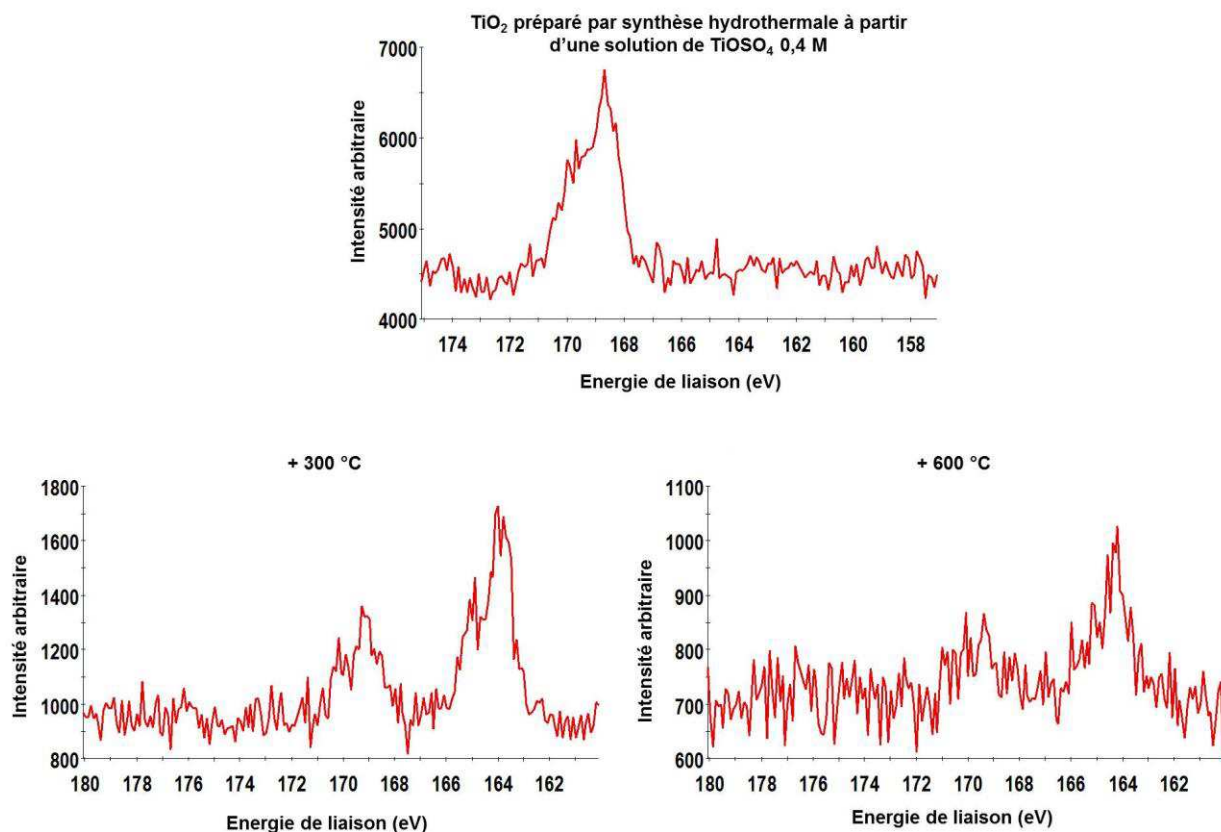
Figure II-24: Diagrammes de spectrométrie photoélectronique X de \text{TiO}_2 sulfaté (synthèse D avant et après traitement thermique à 300 °C et 600 °C).
