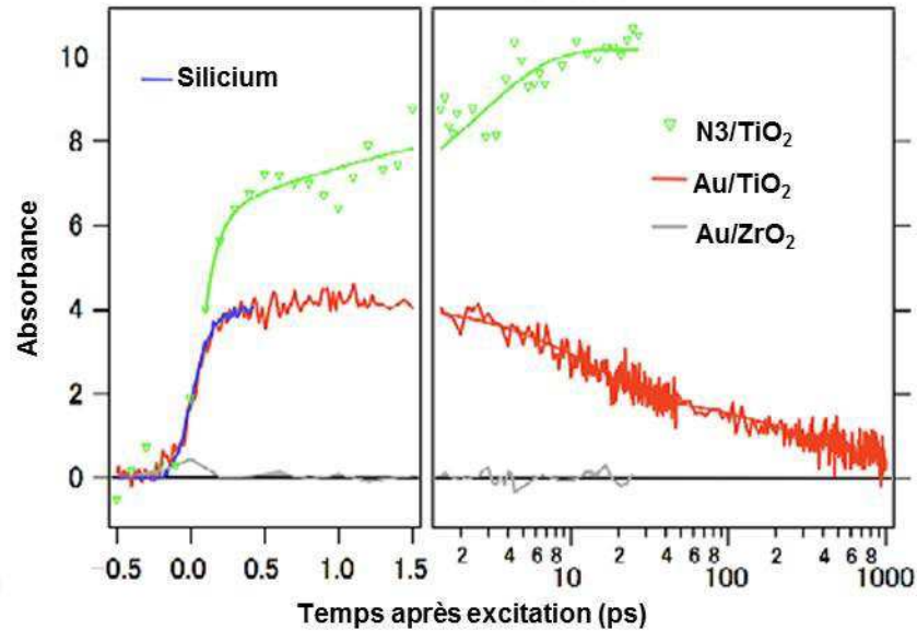
Figure I-29: Absorptions à 3440 nm correspondant à la présence d'électrons libres dans la bande de conduction du semi-conducteur après irradiation d'échantillons de TiO_2 sensibilisé par colorant, de composite Au (10nm)/ ZrO_2 et de composite Au (10nm) TiO_2 (20 nm P25 Degussa) [355].
