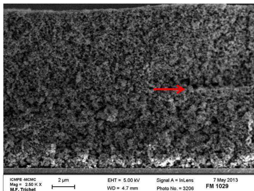
Figure III-6: Cliché MEB de la section d'un dépôt de deux couches homogènes de \text{TiO}_2 issu de la synthèse C.
