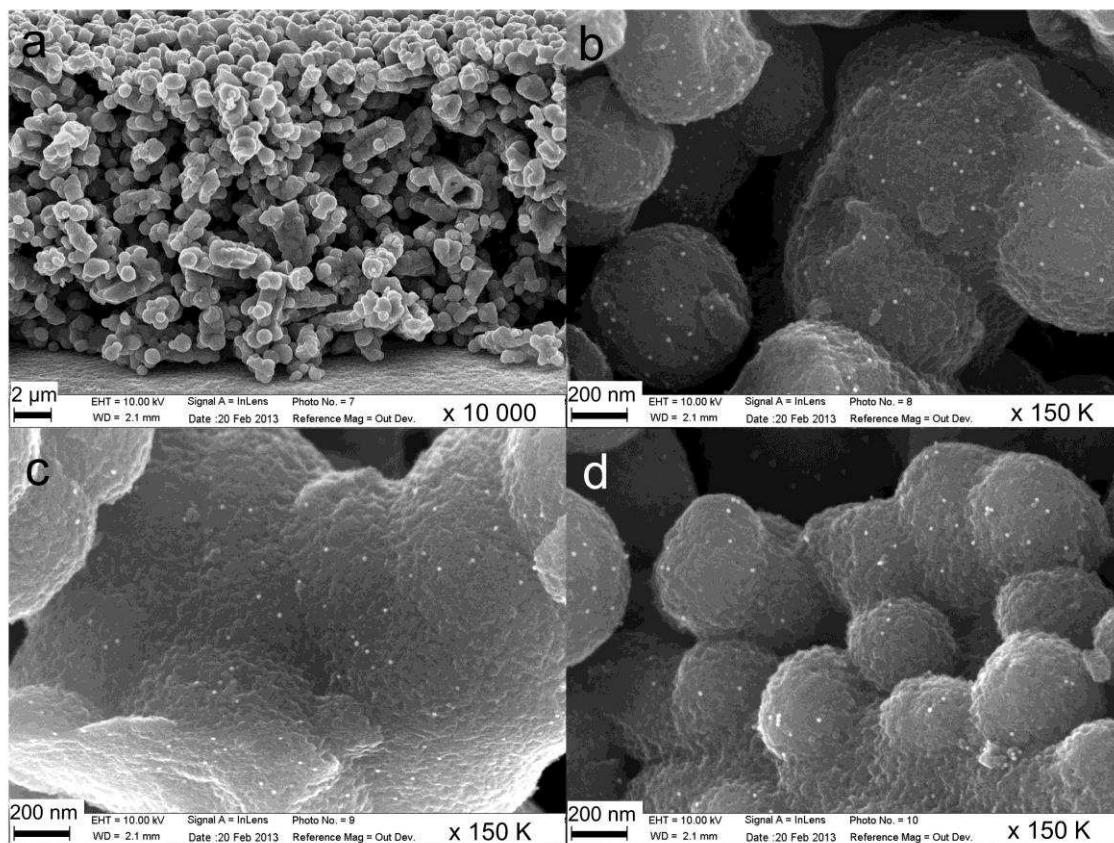
Figure III-20: Clichés MEB de la section d'un film de Au/TiO 2 formé à partir de poudre TiO 2 issue de la synthèse A et de nanoparticules d'or, agrégées en solution aqueuse (a). Zooms sur les couches supérieures (b), médianes (c) et inférieure (d) du film.
