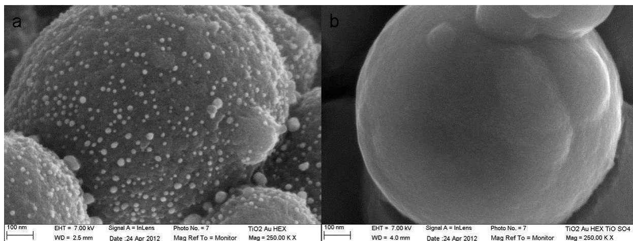
Figure IV-5: Clichés MEB de particules de \text{TiO}_2 décorées de nanoparticules d'or avant (a) et après (b) dépôt d'une couche protectrice de \text{TiO}_2 par voie électrochimique.
