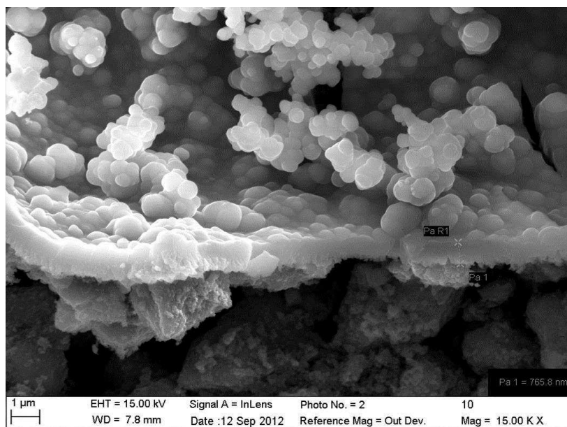
Figure IV-7: Cliché MEB d'une couche de \text{TiO}_2 (766 nm d'épaisseur) électrodéposée en 30 min.
