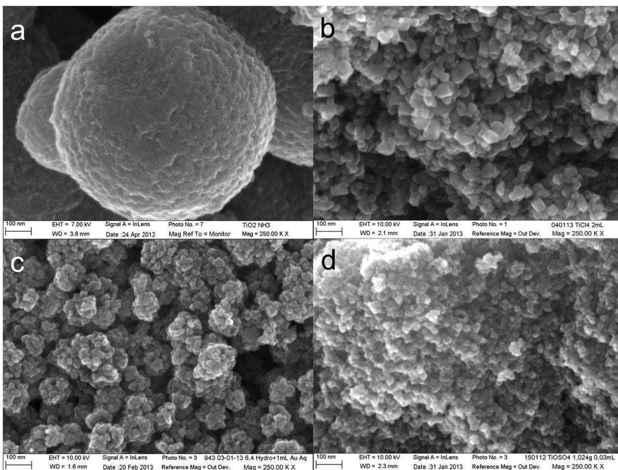
Figure II-26: Clichés MEB des poudres de \text{TiO}_2 issues des synthèses A (a), B (b), C (c) et D (d).
