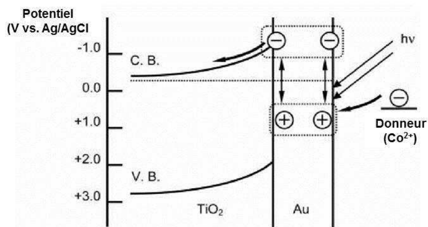
Figure I-25: proposition de mécanisme pour le fonctionnement de cellule solaires plasmoniques sans colorant [346].
