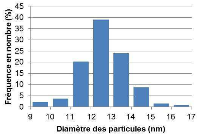
Figure II-28: Distribution en taille des nanoparticules d'or synthétisées en solution aqueuse par la méthode de Jana et col..
