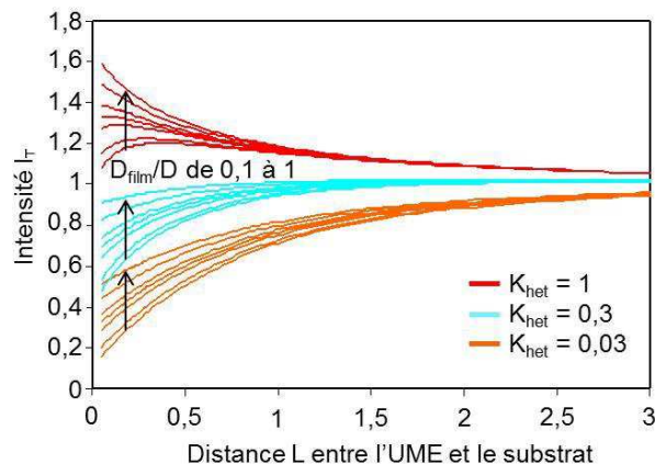
Figure III-34: Influence du transport poreux sur les courbes d'approche d'un film poreux réactif d'épaisseur E = 0,5 . Les valeurs de la vitesse de transfert de charge adimensionnelle K_{het} sont 1 (rouge), 0,3 (turquoise), et 0,03 (orange). Les valeurs de D_{film}/D sont de bas en haut 0,1 0,2 0,4 0,5 0,6 0,8 et 1.
