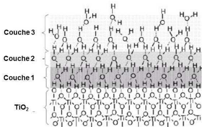
Figure I-9 : Structure hypothétique des couches d'eau sur une surface idéale de \text{TiO}_2 déduite des observations en RMN du proton d'après [40].
