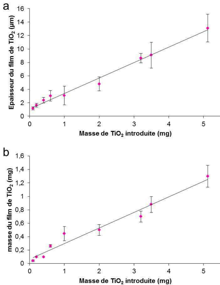
Figure III-2: Evolution de l'épaisseur (a) et de la masse (b) des films de \text{TiO}_2 déposé en fonction de la masse de poudre issue de la synthèse A introduite.
