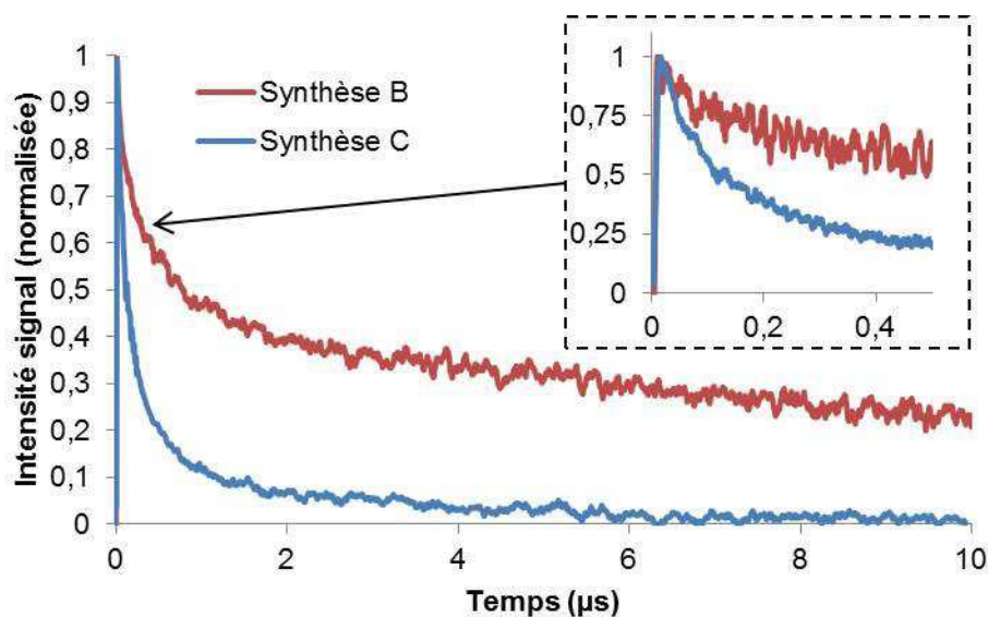
Figure IV-16: Signaux de TRMC de films de \text{TiO}_2 synthétisés par les synthèses B et C.
