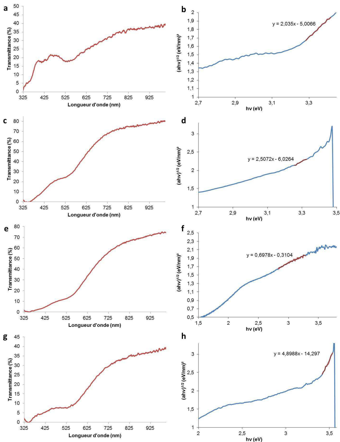
Figure III-26: Spectres de transmission optique et détermination de l'énergie de la bande interdite de films constitués de 3% mass. de nanoparticules d'or de 6nm et de TiO 2 synthétisés par les synthèses A (a et b), B (c et d), C (e et f) et D (g et h).
