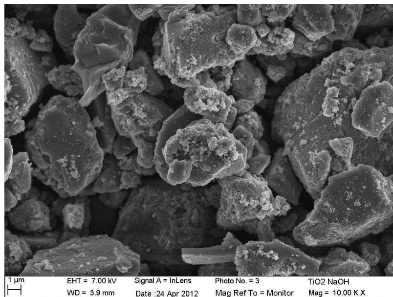
Figure II-6 : Cliché MEB de la poudre de \text{TiO}_2 synthétisée à 85 °C avec ajout de NaOH.
