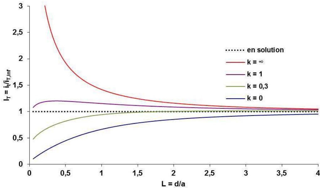
Figure 4: Courbes d'approches représentant le courant mesuré à l'ultramicroélectrode pour différentes réactivités de surfaces.
