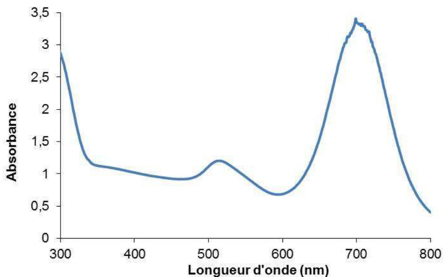
Figure II-31: Spectre d'absorption d'une solution de nanobâtonnets d'or préparée par la méthode de Sau et col..
