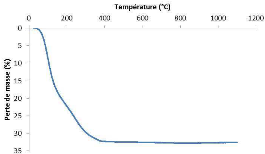
Figure II-2: ATG de \text{TiO}(\text{OH})_2, 1,5\text{H}_2\text{O} obtenu par synthèse A.
