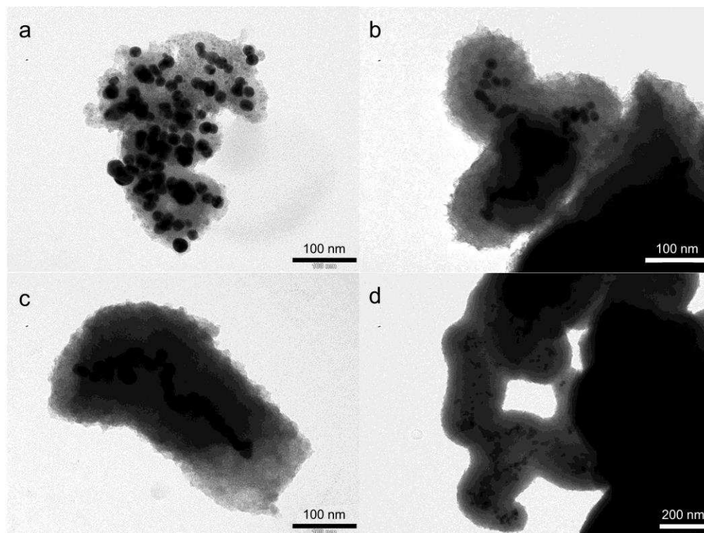
Figure IV-9 : Clichés MET de nanoparticules d'or entourées d'une couche de TiO 2 obtenues par hydrolyse à température ambiante de TiOSO 4 au sein d'une solution de particules d'or en solution aqueuse à 1 mg.l -1 . Les concentrations en TiOSO 4 sont de 2 mM (a), 10 mM (b), 20 mM (c) et 27 mM (d).
