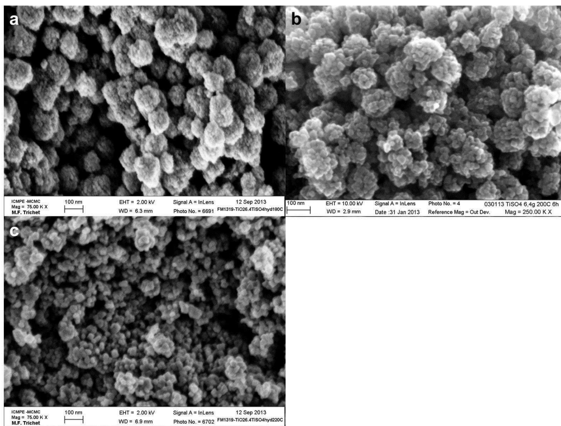
Figure II-17: Clichés MEB des poudres TiO 2 synthétisées par voie hydrothermales à partir de TiOSO 4 (2,5 M) à 180 °C (a), 200 °C (synthèse C) (b) et 220 °C (c).
