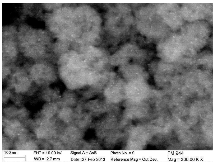
Figure III-37: Cliché de microscopie électronique à balayage d'un film de TiO 2 issu de la synthèse C chargé de 5,4 % massique de nanoparticules d'or de 6 nm.
