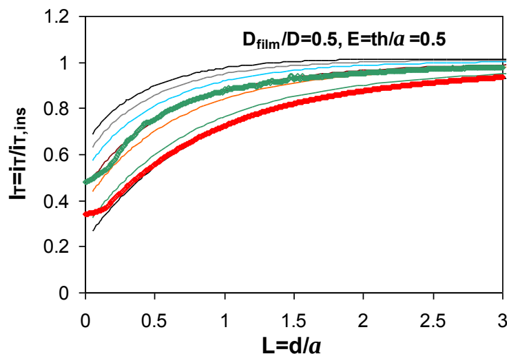
Figure III-35: Courbes d'approche de films poreux de TiO_2 issu de la synthèse C d'épaisseur 6 \mu m avec (vert) et sans (rouge) incorporation de 4,2 % mass. de nanoparticules d'or. Comparaison avec des courbes simulées pour une diffusion dans le film de D_{film}/D = 0,5 et un transfert d'électron hétérogène \kappa_{het}=0 0,03 0,1 0,14 (fit) 0,2 0,25 et 0,3.
