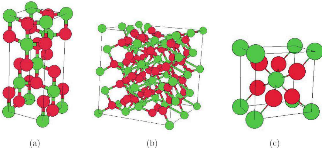
Figure I-7 : Structures cristallographiques de \text{TiO}_2 : (a) anatase, (b) brookite, (c) rutile. En vert \text{Ti}^{4+} et en rouge \text{O}^{2-} .
