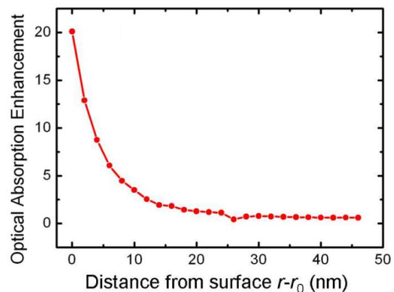
Figure I-27: Facteur d'amélioration d'absorption des colorants par la présence du champs électrique en fonction de la distance du chromophore par rapport à la surface de la particule enrobée [175].
