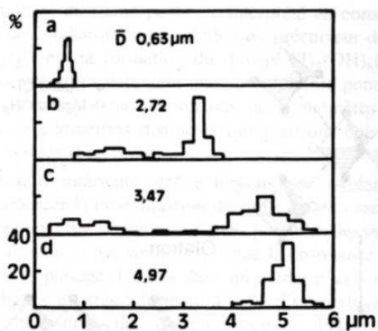
Figure I-4 : Distribution de taille des particules de rutile en fonction du temps de chauffage d'une solution aqueuse d'oxyhydroxyde de titane à 95 °C. Durée (a) 0 h ; (b) 1 h ; (c) 3 h ; (d) 6 h. (HCl : 2,13 mol/l et Ti : 0,22 mol/l) [2].
