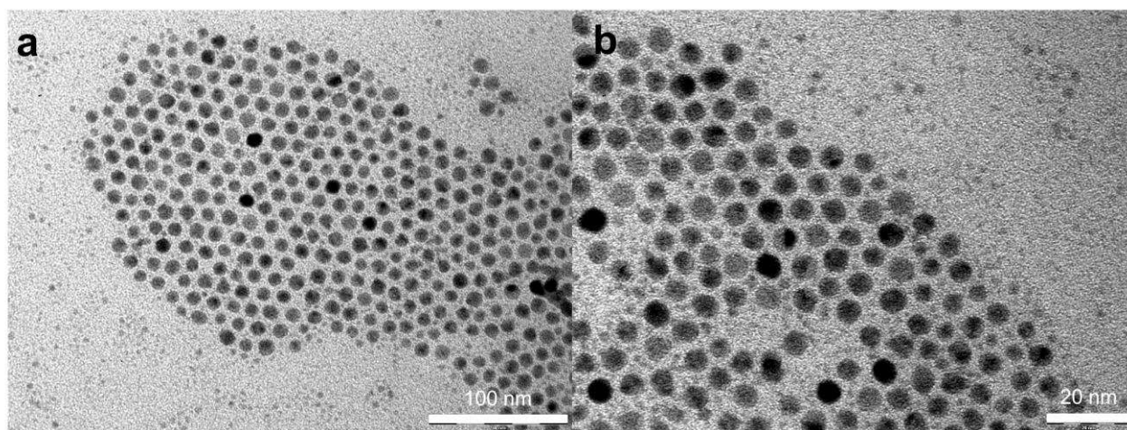
Figure II-33: Clichés MET de nanoparticules d'or de 6 nm synthétisées à partir de \text{ClAuPPh}_3 dans \text{C}_6\text{H}_6 .
