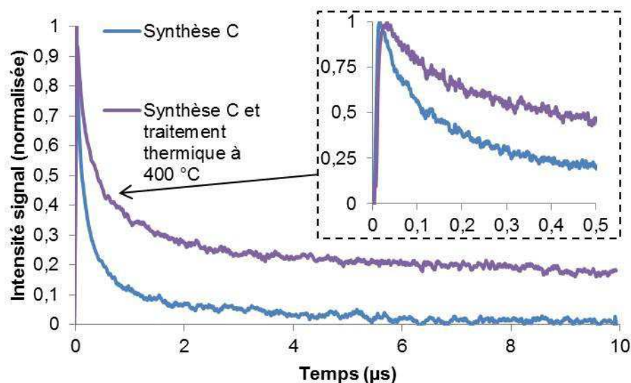
Figure IV-18: Signaux de TRMC de films de \text{TiO}_2 synthétisés par la synthèse C, avant et après traitement thermique à 400 °C.
