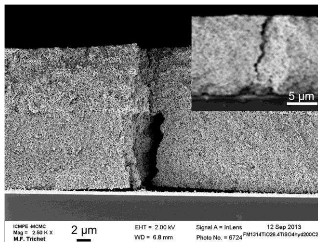
Figure III-11: Cliché MEB de la section de deux films de \text{TiO}_2 issu de la synthèse C montrant une délamination partielle (film formé par 2 dépôts successifs) consécutive à la fissuration et une fissuration partielle sans délamination (encart).
