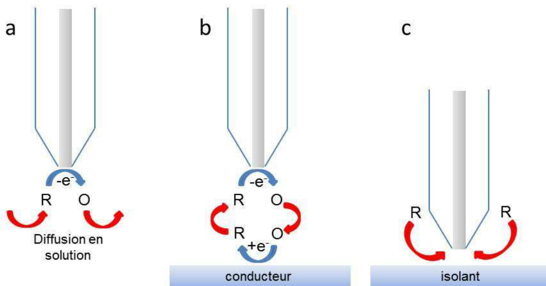
Figure 3: Schémas des processus intervenant pendant l'analyse SECM lorsque l'ultramicroélectrode est éloignée de tout substrat (a), proche d'une surface conductrice (b) et proche d'une surface isolante (c).
