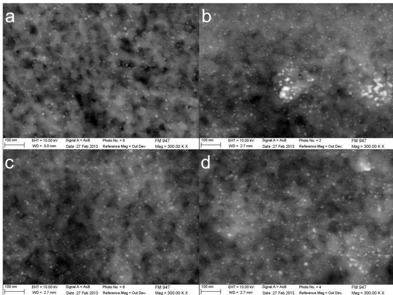
Figure III-18: Clichés MEB par électrons rétrodiffusés de différentes zones (en surface (a) ou au sein du film (sections), dans la partie supérieure (b), médiane (c) ou inférieure (d)) d'un même film de \text{TiO}_2 issu de la synthèse C imprégné par une dispersion d'or en milieu organique.
