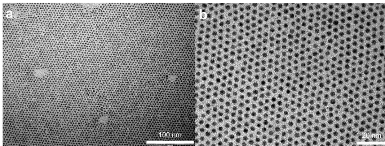
Figure II-32: Clichés MET de nanoparticules d'or de 2 nm synthétisées à partir de \text{ClAuPPh}_3 dans \text{CHCl}_3 .
