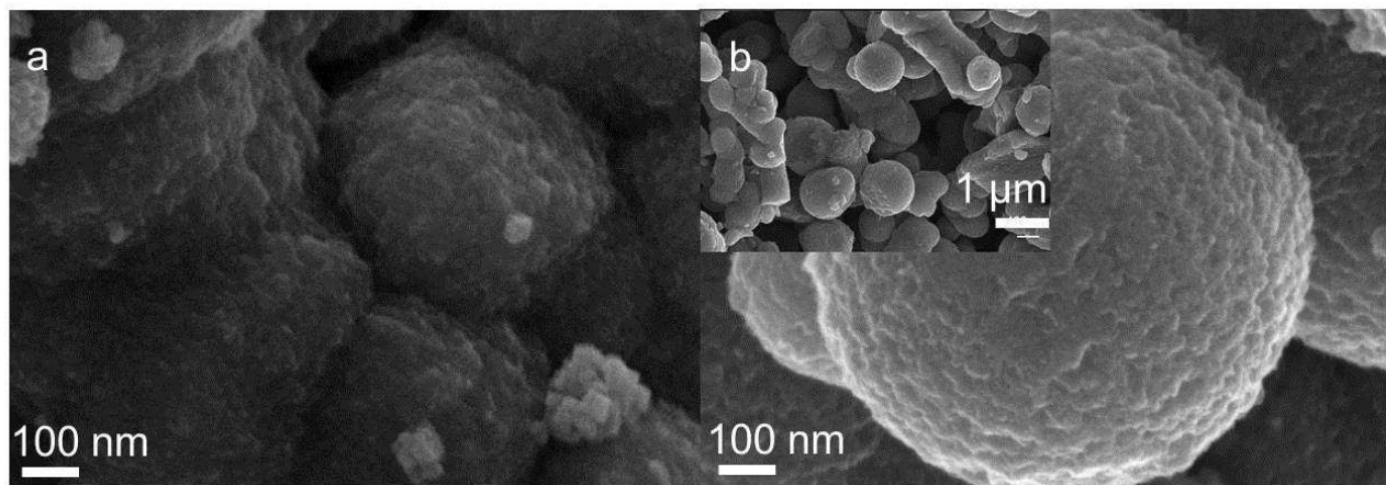
Figure II-4: Clichés MEB de la poudre obtenue à l'issue de l'hydrolyse à température ambiante avant (a) et après (b) calcination à 500 °C.
