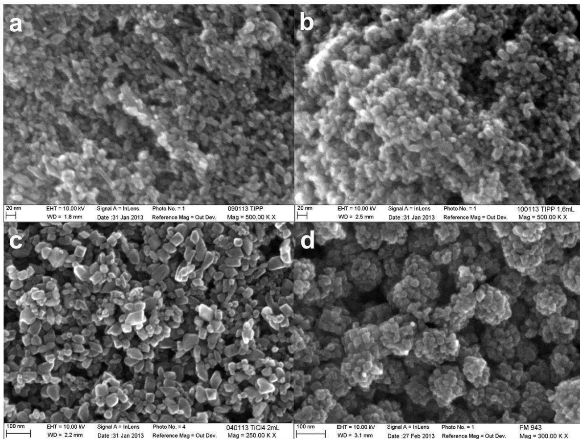
Figure II-12: Clichés MEB des poudres \text{TiO}_2 synthétisées à partir de différents précurseurs : TiPP par les méthodes de Ito et col. (a) et Barbe et col. (b), \text{TiCl}_4 (synthèse B) (c) et \text{TiOSO}_4 à 200^\circ\text{C} et 2,5 M (synthèse C) (d).
