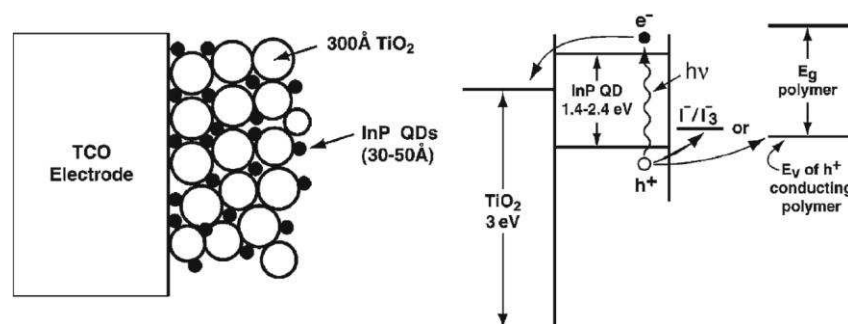
Figure I-20: Représentation schématique d'une cellule solaire à quantum dots [314].
