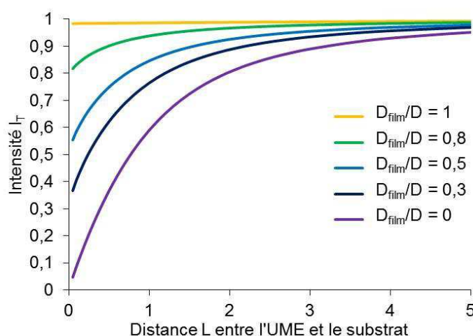
Figure III-28: Evolution de l'intensité adimensionnelle I_T en fonction de L pour des films d'épaisseur E = 5 ayant différentes valeurs de D_{film}/D .
