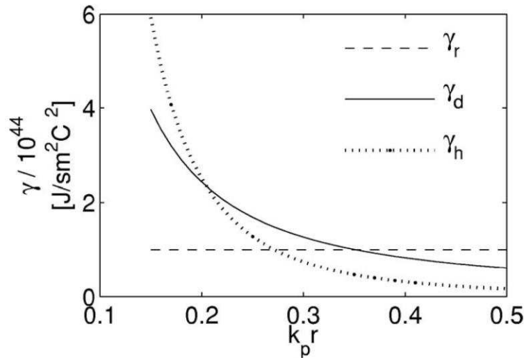
Figure I-26 : Les trois mécanismes d'amortissement \gamma en fonction de k_p r pour \Delta E / \hbar \omega = 0,15 [80].
