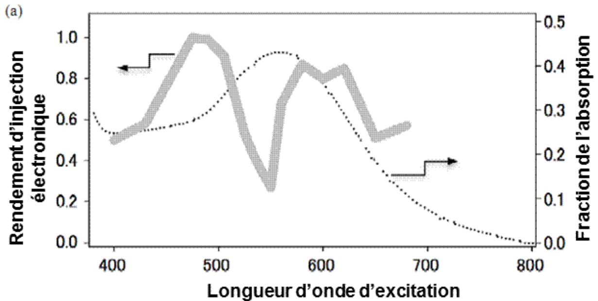
Figure I-24: Taux d'injection de nanoparticules d'or (10 nm) vers des nanoparticules de TiO 2 (30 nm) en fonction de la longueur d'onde de l'excitation laser (courbe grise). Comparaison avec le spectre d'absorption du même film (pointillés) [355].
