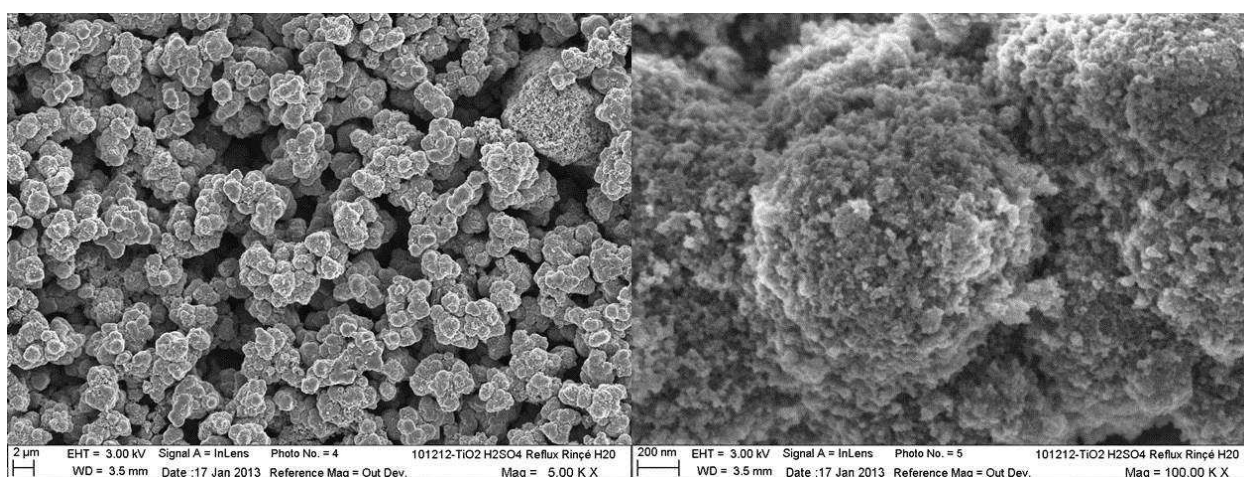
Figure II-7 : Clichés MEB de la poudre synthétisée à partir de \text{TiOSO}_4 \text{H}_2\text{SO}_4 \text{H}_2\text{O} .
