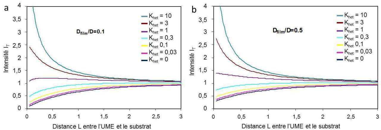
Figure III-33: Evolution de l'intensité I_T en fonction de L pour des films ayant différentes vitesses de transfert de charge K_{het} (comprise entre 0 et 10) sur les courbes d'approche de films poreux d'épaisseur E = 0,5 et D_{film}/D = 0,1 (a) ou 0,5 (b).
