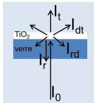
Figure III-24: Schéma du fractionnement de l'intensité lumineuse incidente I_0 sur un film de \text{TiO}_2 déposé sur un substrat de verre. I_r est la fraction réfléchi, I_t la fraction transmise, I_{dt} la fraction diffusée transmise et I_{rd} la fraction rétrodiffusée.
