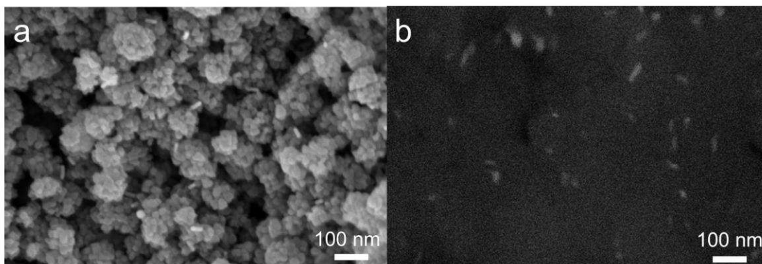
Figure III-21: Clichés MEB par électrons secondaires (a) et rétrodiffusés (b) de la section d'un film de Au/TiO 2 formé à partir de poudre TiO 2 issue de la synthèse C et de nano-bâtonnets d'or, agrégés en solution aqueuse.
