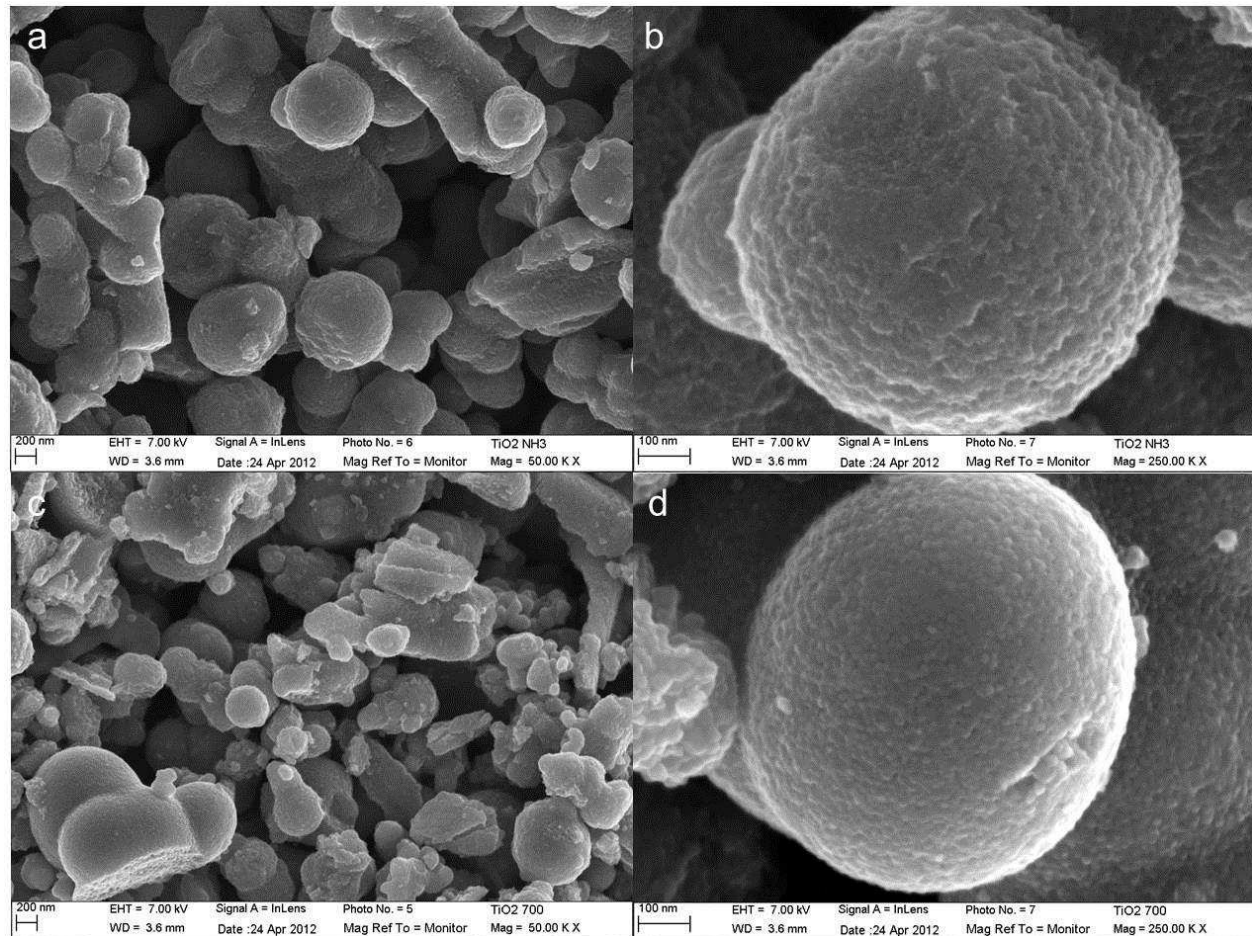
Figure II-20: Clichés MEB de la poudre de TiO 2 issue de la synthèse A avec une température de calcination de 500 °C (a et b) et 700 °C (c et d).
