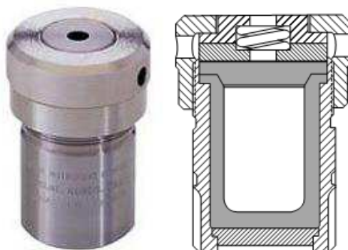
Figure II-9: Photographie et schéma du réacteur utilisé pour les synthèses hydrothermales [10].
