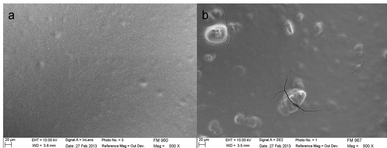
Figure III-5: Clichés MEB de la surface de films déposés à partir d'une dispersion de \text{TiO}_2 issu de la synthèse C décantée (a) ou non décantée (b).
