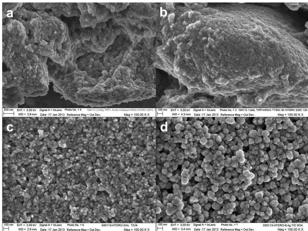
Figure II-13 : Clichés MEB des structures d'agglomération des poudres \text{TiO}_2 synthétisées à partir de différents précurseurs : TiPP par les méthodes de Ito et col. (a) et Barbe et col. (b), \text{TiCl}_4 (synthèse B) (c) et \text{TiOSO}_4 à 200 °C et 2,5 M (synthèse C) (d).
