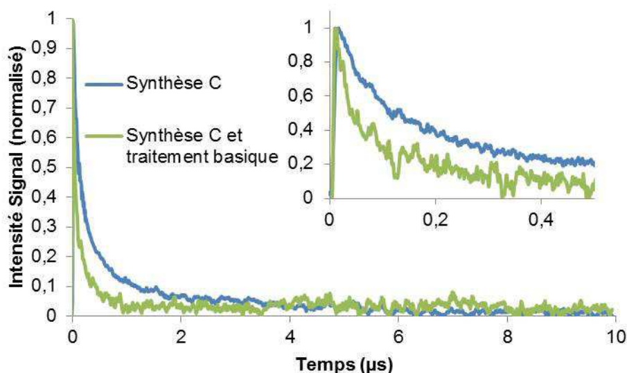
Figure IV-17: Signaux de TRMC de films de \text{TiO}_2 synthétisés par la synthèse C, avec et sans traitement basique visant à retirer les ligands sulfates.
