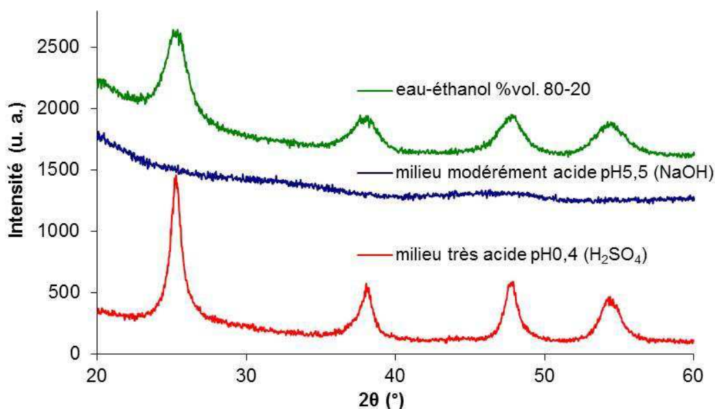
Figure II-5 : Diffractogrammes RX des poudres de \text{TiO}_2 synthétisées par hydrolyse à 85 °C.
