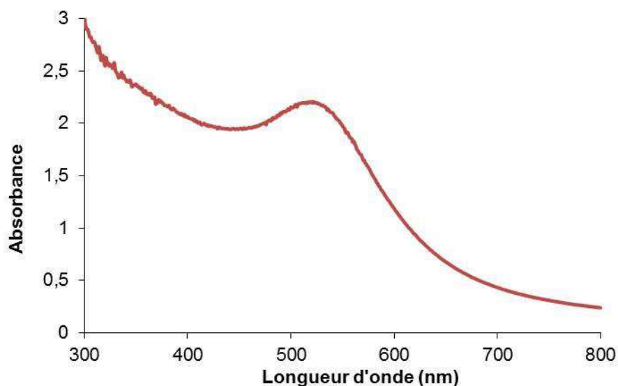
Figure II-35: Spectre d'absorption d'une solution de nanoparticules d'or de 6 nm.
