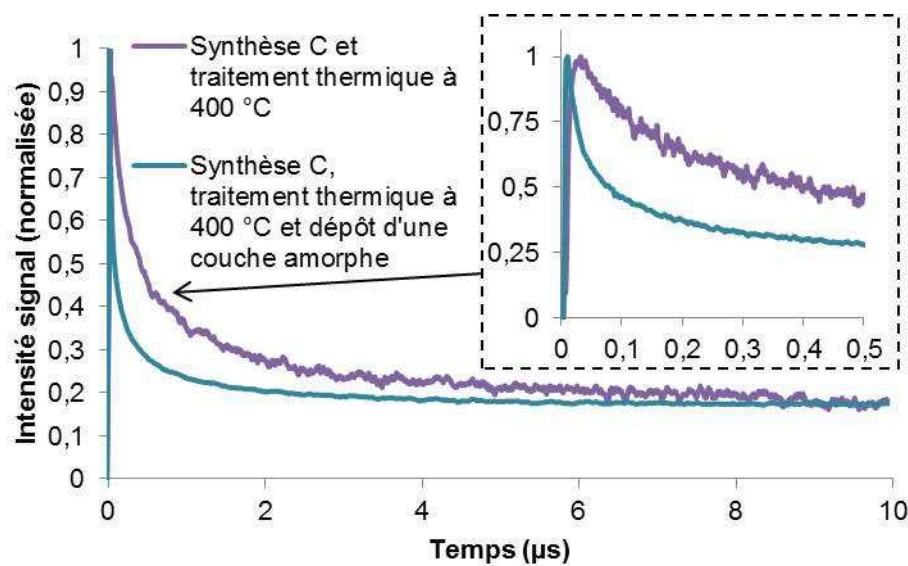
Figure IV-20: Signaux de TRMC de films de \text{TiO}_2 synthétisés par la synthèse C puis traités thermiquement, avec et sans couche amorphe
