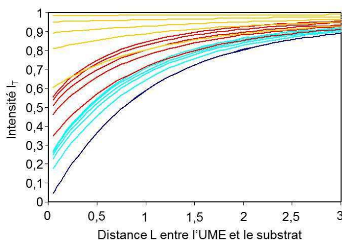
Figure III-29: Evolution de l'intensité I_T en fonction de L pour des films de différentes épaisseurs ( E = 1-10 ) et différentes valeurs de D_{film}/D (0 ; 0,2 ; 0,5 ; 1).
