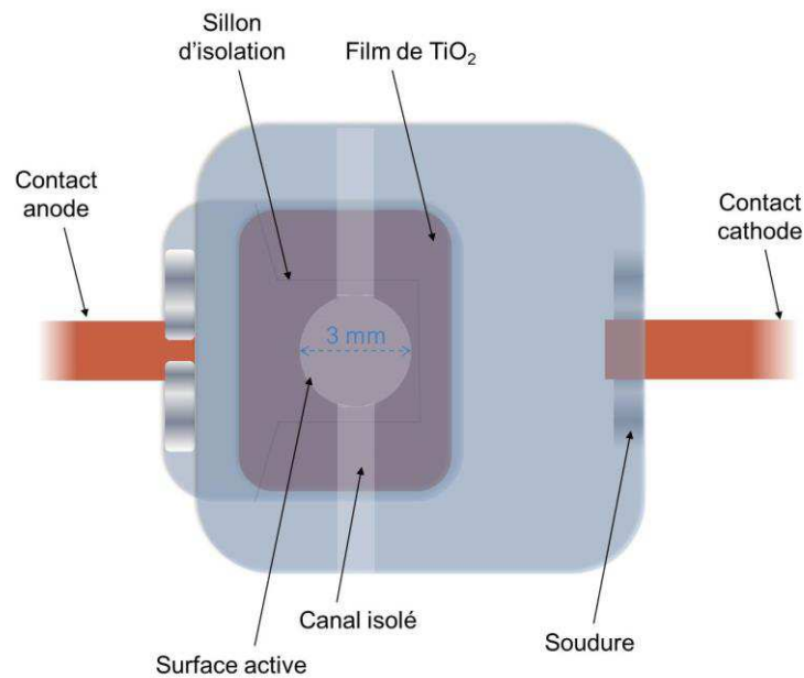
Figure IV-3: Schéma d'une cellule solaire à colorant avec anode \text{TiO}_2 .
