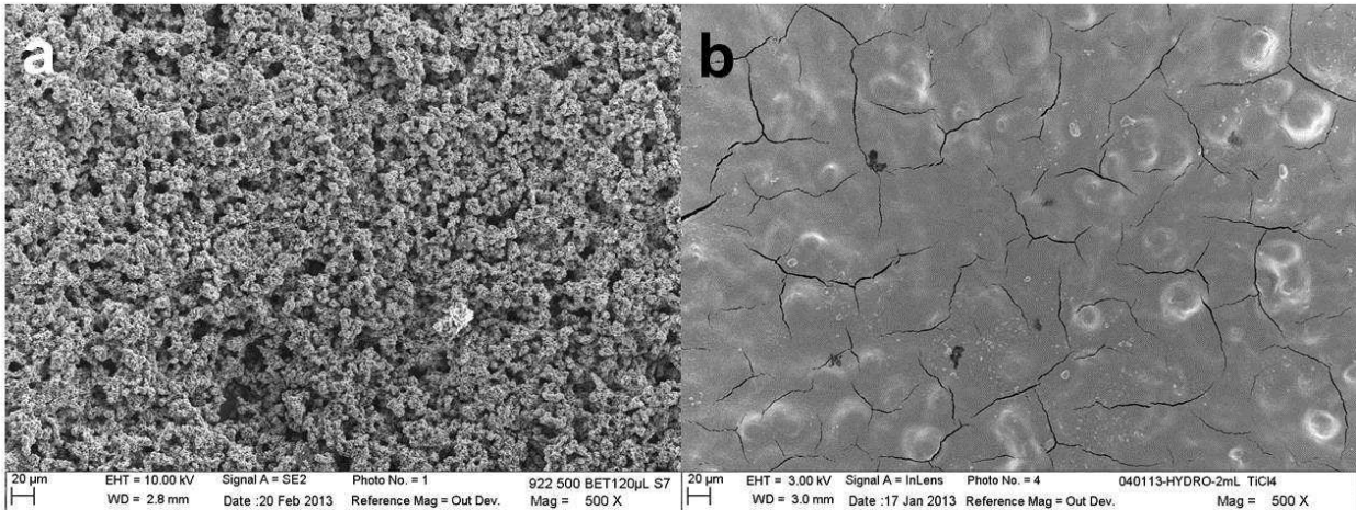
Figure III-12: Clichés MEB des surfaces de films de \text{TiO}_2 issus des synthèses A (a) et B (b) avec des épaisseurs respectives de 30 \mu\text{m} et 10 \mu\text{m} .
