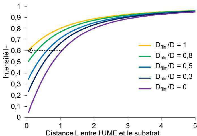
Figure III-27: Evolution de l'intensité adimensionnelle I_T en fonction de L pour des films d'épaisseur E = 1 ayant différentes valeurs de D_{film}/D .
