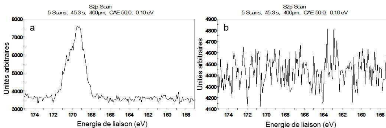
Figure II-25: Diagrammes de spectrométrie photoélectronique X de \text{TiO}_2 issu de la synthèse C sulfaté avant (a) et après (b) traitement basique.
