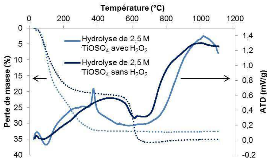
Figure II-23: ATG (pointillés) et ATD (traits pleins) de TiO(OH) 2 , 1,5H 2 O obtenu par synthèse A (bleu clair) et du produit de l'hydrolyse partielle de TiOSO 4(aq) 2,5 M à température ambiante pendant 2 jours (bleu foncé).
