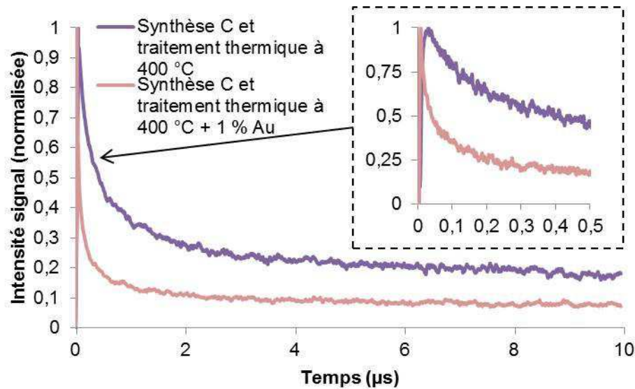
Figure IV-19: Signaux de TRMC de films de \text{TiO}_2 synthétisés par la synthèse C puis traité thermiquement, avec et sans or
