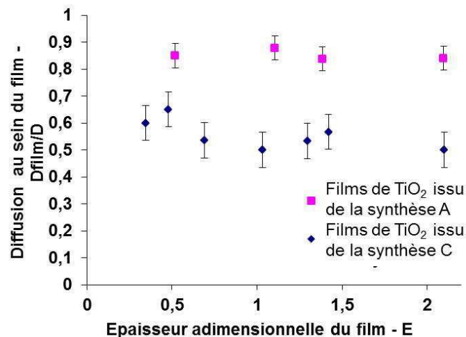
Figure III-31: Transport estimé par SECM pour les films de TiO_2 d'épaisseurs micrométriques issus des synthèses A et C.
