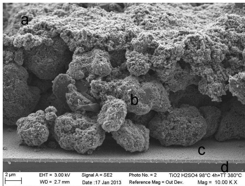
Figure III-4: Cliché MEB de la section d'une couche granulaire de \text{TiO}_2 comprenant des agglomérats nanométriques (a) et micrométriques (b) sur une couche conductrice principalement composée de \text{SnO}_2 (c) déposée sur du verre (d).
