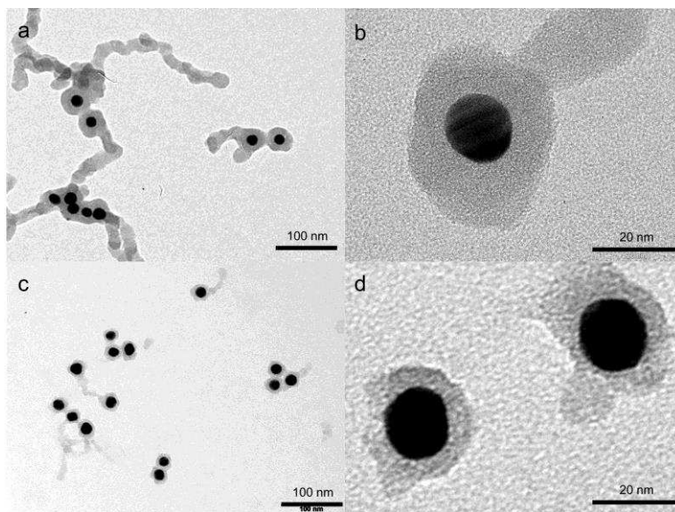
Figure IV-8: Clichés TEM de nanoparticules cœur-écorce Au@SiO 2 formées en solution aqueuse par l'ajout de 16 \mu l (a et b) et 8 \mu l (c et d) de TEOS.
