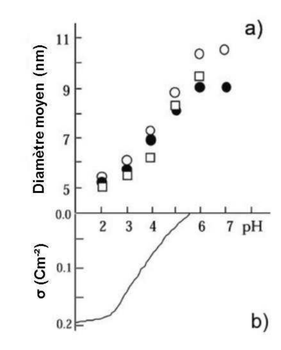
Figure I-6 : (a) Taille moyenne des particules d'anatase formées à 60 °C à différents pH et forces ioniques. Taille moyenne après 24h (cercles pleins) et une semaine (cercles vides) ([NaCl] = 0,5 mol.L -1 ) et taille moyenne après une semaine avec une ([NaCl] = 3 mol.L -1 ) (carrés vides). (b) Variation de la densité de charges de surfaces de particules d'anatase formées à un pH = 3 après 3 jours à 60 °C. Les mesures ont été effectuées à 25 °C et une force ionique ajustée à 0,01 mol.L -1 par addition de NaNO 3 [18].
