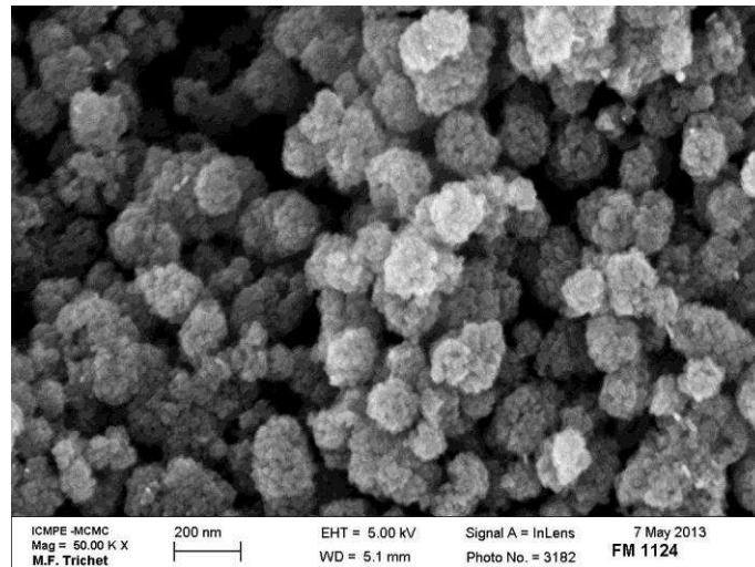
Figure III-32: Cliché MEB de la poudre de \text{TiO}_2 issue de la synthèse C.
