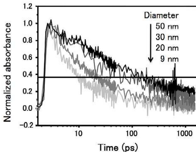
Figure I-30: Effet de la taille des nanoparticules de TiO_2 sur la cinétique de recombinaison des électrons injectés [355].
