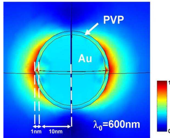
Figure I-14: Intensité normalisée du champ électrique créé par une nanoparticule d'or enrobée de PVP en présence d'une onde plane incidente de longueur d'onde 600 nm [175].
