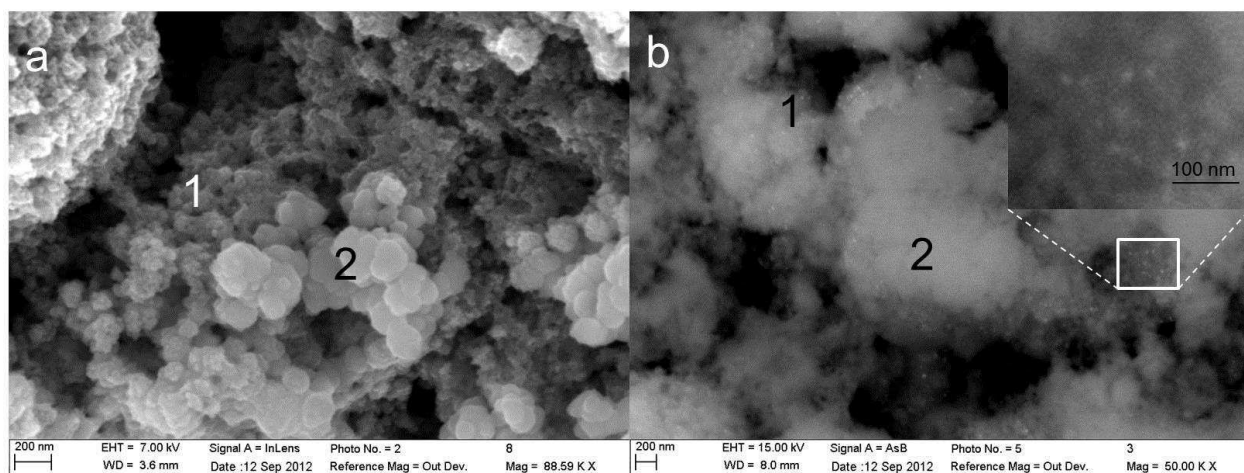
Figure IV-6: Clichés MEB en modes électrons secondaires (a) et électrons rétrodiffusés (b) d'un électrodépôt de 10 secondes de \text{TiO}_2 sur une couche mésoporeuse d'anatase.
