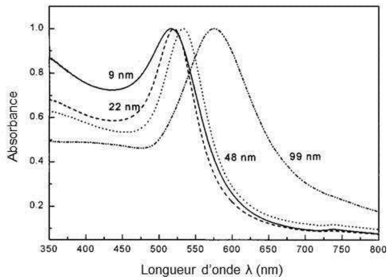
Figure I-15: Spectres d'absorption de nanoparticules d'or de 9 nm, 22 nm, 48 nm et 99 nm de diamètre dispersées dans l'eau. Les intensités ont été normalisées par les maximums d'absorption situés respectivement à 517 nm, 521 nm, 533 nm et 575 nm [183].
