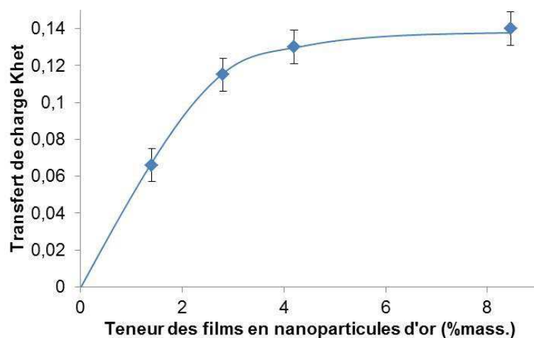
Figure III-36: Influence de la quantité de nanoparticules d'or sur la constante de transfert de charge apparente des films Au/TiO 2 .
