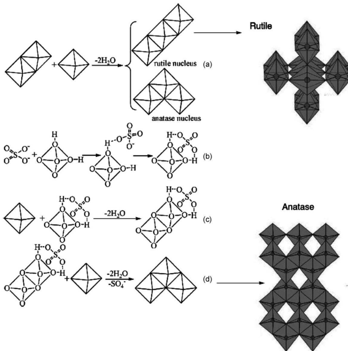
Figure I-3 : Proposition de mécanisme de formation de rutile et d'anatase. L'orientation du troisième octaèdre détermine quelle maille est formée (a). Les interactions entre \text{SO}_4^{2-} et \text{TiO}_6^{2-} (b) entraînent le partage des arêtes (c) et la formation d'anatase (d). [5]
