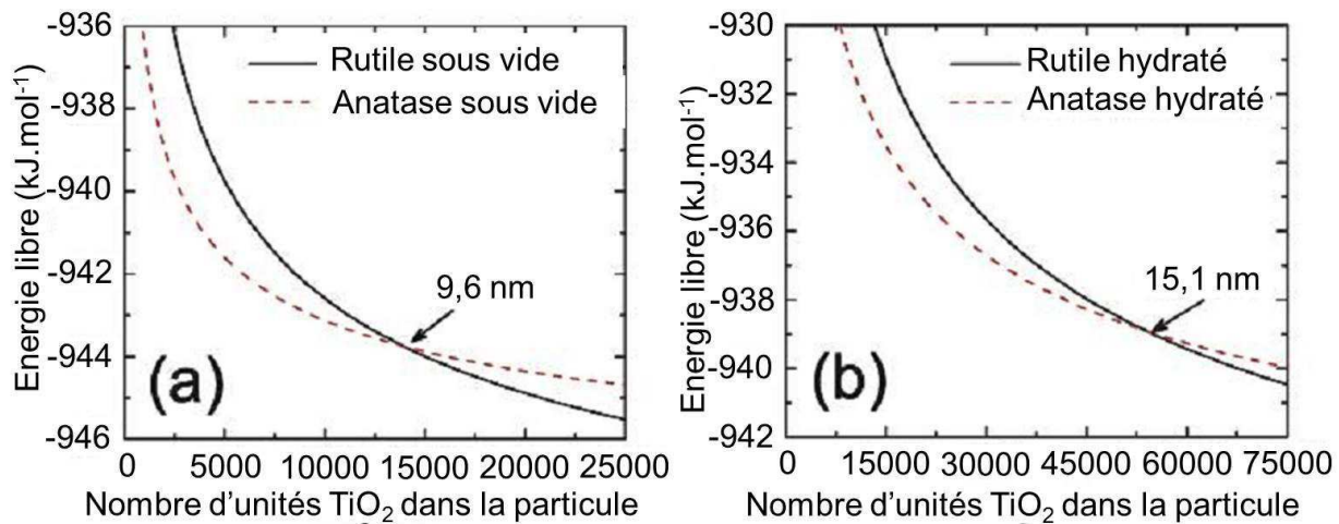
Figure I-5 : Stabilité thermodynamique des phases \text{TiO}_2 anatase et rutile obtenue par modélisation d'après Barnard et col. [13]: (a) pour une surface propre et (b) pour une surface hydratée.
