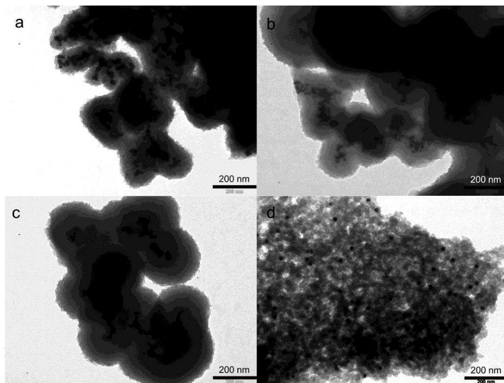
Figure IV-10: Clichés MET de nanoparticules d'or entourées d'une couche de \text{TiO}_2 obtenues par hydrolyse à température ambiante de \text{TiOSO}_4 au sein d'une solution de particules d'or en solution aqueuse de 67 \text{ mg.l}^{-1} (a), 15,4 \text{ mg.l}^{-1} (b), 10,5 \text{ mg.l}^{-1} (c) et 1 \text{ mg.l}^{-1} (d) avec un rapport molaire n_{\text{Ti}}/n_{\text{Au}} constant et égal à 40 (eg. 2 \cdot 10^{-5} mol de \text{TiOSO}_4 et 5 \cdot 10^{-7} mol de Au).
