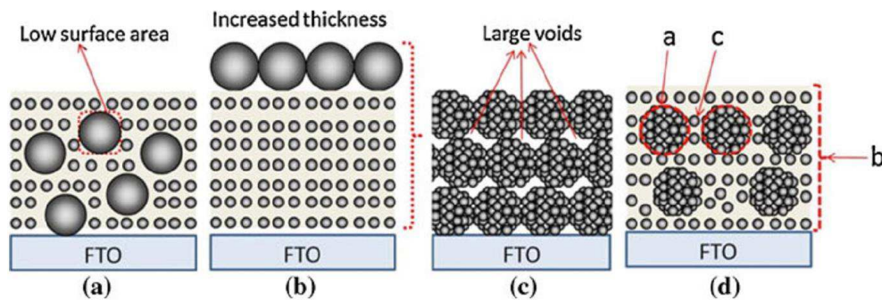
Figure I-21: Schémas de différentes techniques pour augmenter la diffusion du rayonnement visible au sein de la couche de semi-conducteur [316].
