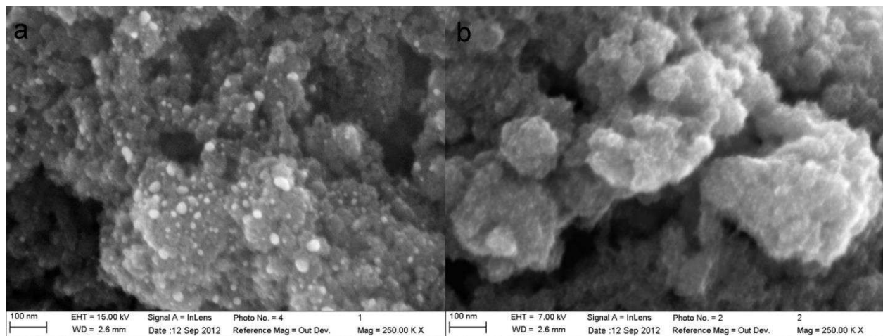
Figure IV-4: Clichés MEB d'une couche de \text{TiO}_2 anatase et nanoparticules d'or avant (a) et après (b) dépôt d'une couche protectrice de \text{TiO}_2 amorphe via trempage dans une solution de \text{TiCl}_4 .
