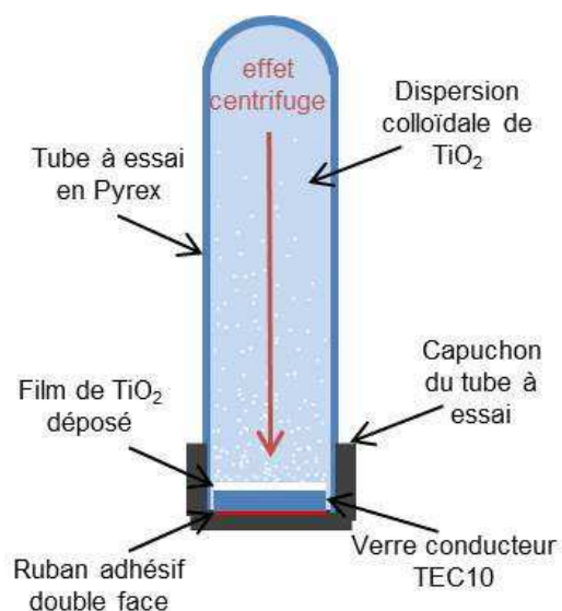
Figure III-1 : Schéma du dispositif expérimental du dépôt de \text{TiO}_2 par centrifugation.
