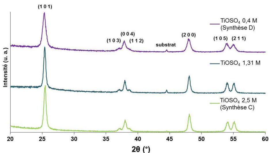
Figure II-14: Diffractogrammes RX des poudres \text{TiO}_2 préparées par voie hydrothermale à 200 °C à partir de différentes concentrations de \text{TiOSO}_4 : 0,4 M (synthèse D), 1,3 M et 2,5 M (synthèse C).
