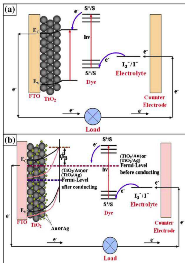
Figure I-28 : Comparaison entre le schéma de fonctionnement d'une cellule solaire à colorant classique (a) et celui d'une cellule solaire à colorant avec des particules composites Au (ou Ag) - \text{TiO}_2 (b) [387].
