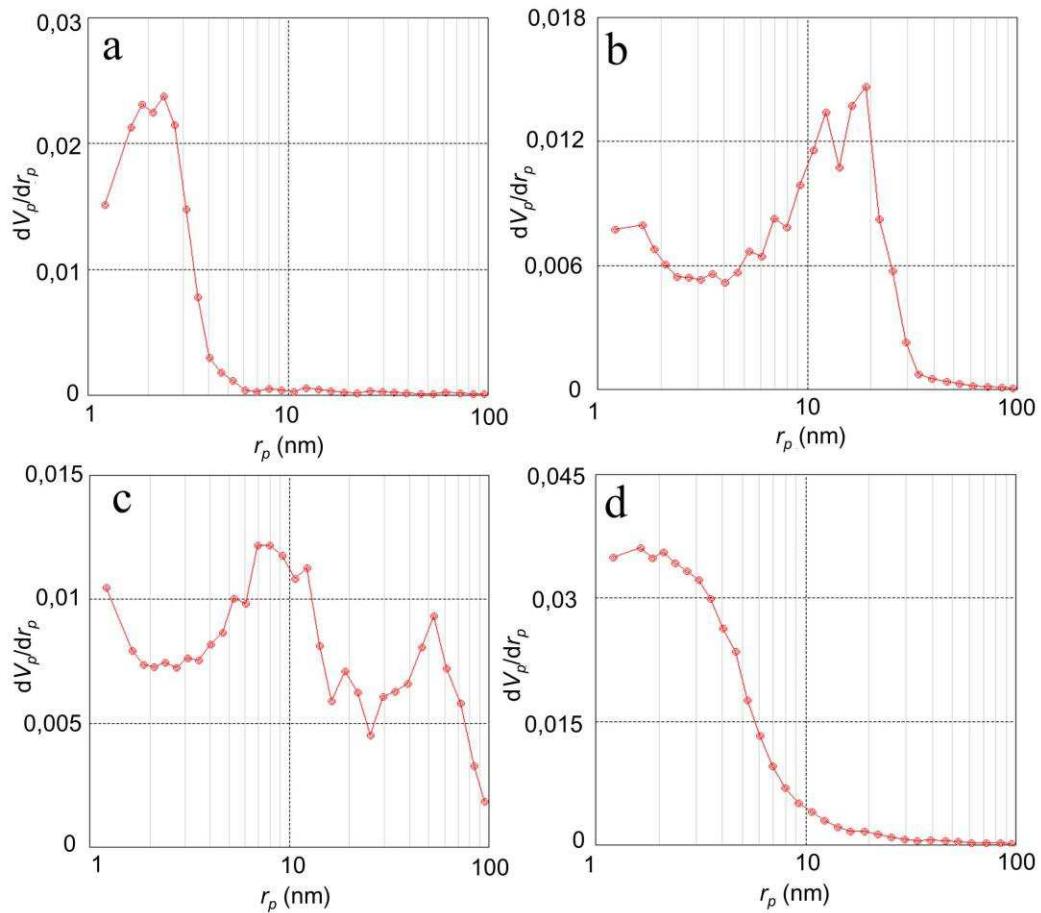
Figure II-22: Analyse BJH de mesure d'adsorption de gaz ( N_2 à 77 K) sur des poudres de TiO_2 issues des synthèses A (a), B (b), C (c), et D (d). Les courbes présentent le volume poreux ( V_p ) en fonction du diamètre des pores considérés comme sphériques ( r_p ).
