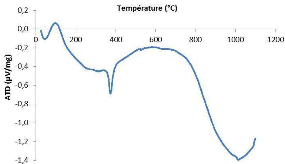
Figure II-3: ATD de \text{TiO}(\text{OH})_2, 1,5\text{H}_2\text{O} obtenu par synthèse A.
