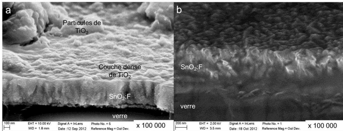
Figure III-8: Clichés MEB (section) d'une couche nanométrique de \text{TiO}_2 recouvrant un substrat TEC10 et quelques particules d'anatase (a) et du substrat de TEC10 seul (b).
