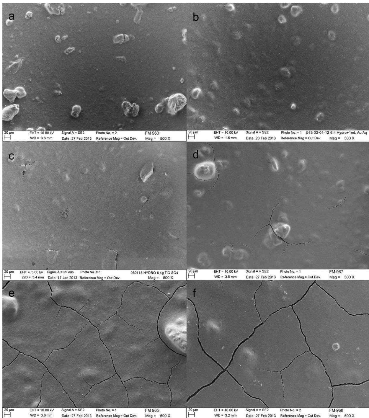
Figure III-13: Clichés MEB de la surface de films de \text{TiO}_2 de différentes épaisseurs formés à partir de poudres issues de la synthèse C). Les épaisseurs moyennes des films sont de 2 \mu\text{m} (a), 8 \mu\text{m} (b), 12 \mu\text{m} (c), 14 \mu\text{m} (d), 16 \mu\text{m} (e) et 20 \mu\text{m} (f).
