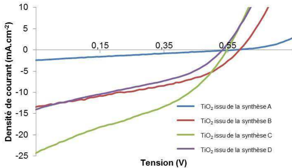
Figure IV-14: Evolution de la densité de courant en fonction de la tension aux bornes de la cellule pour des cellules fabriquées à partir des TiO 2 issus des synthèses A, B, C et D.
