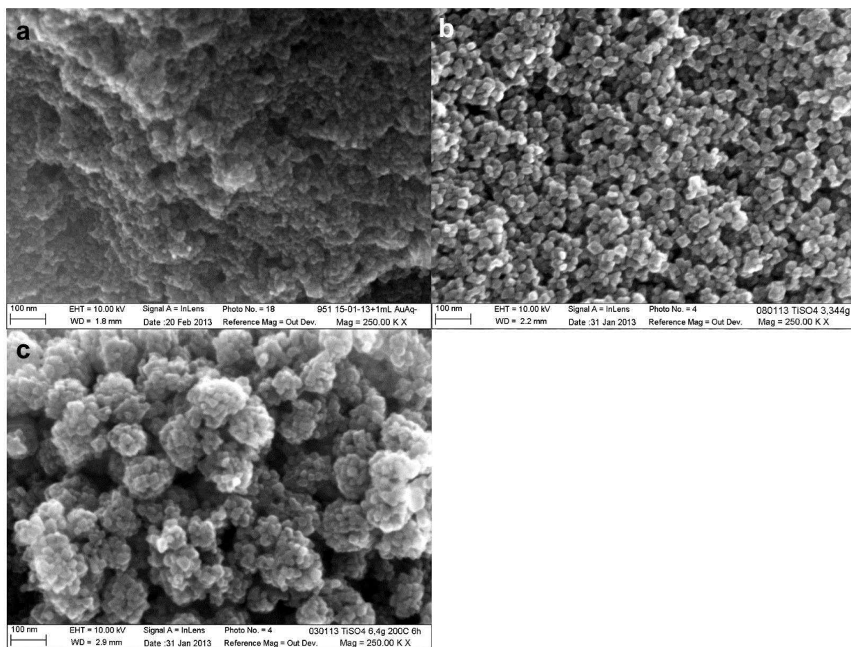
Figure II-15 : Clichés MEB des poudres \text{TiO}_2 synthétisées par voie hydrothermales à partir de \text{TiOSO}_4 à 200 °C aux concentrations de 0,4 M (synthèse D) (a), 1,3 M (b) et 2,5 M (synthèse C) (c).
