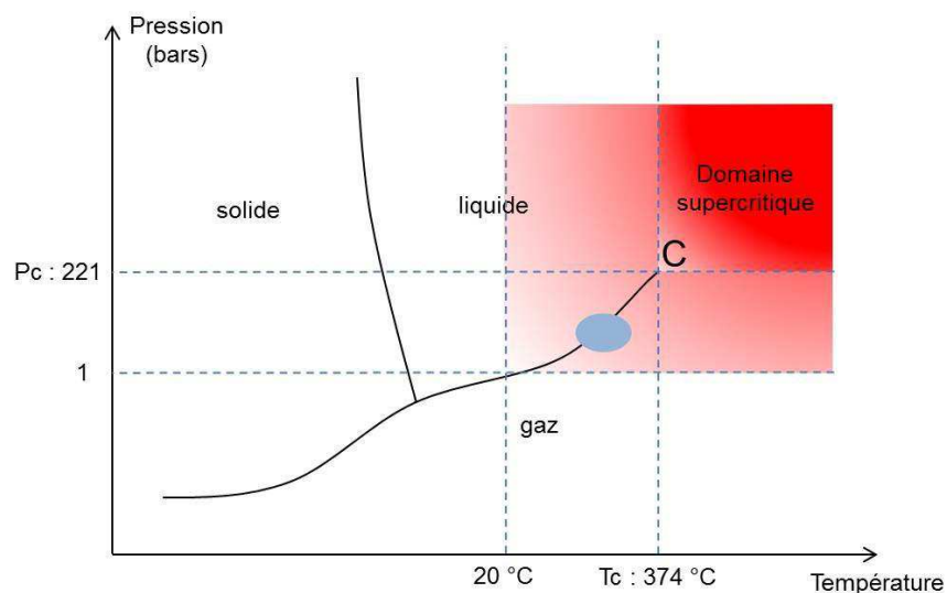
Figure II-10 : Diagramme schématisique Pression-Température de l'eau. C est le point critique et l'ovale bleu situe les conditions expérimentales utilisées.
