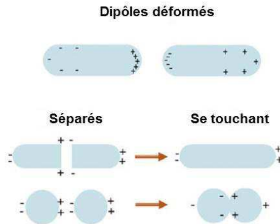
Figure I-16 : Distorsion de la distribution des charges surfaciques lorsque deux nanoparticules métalliques sont jointes par une surface plane ou par un contact ponctuel [190].
