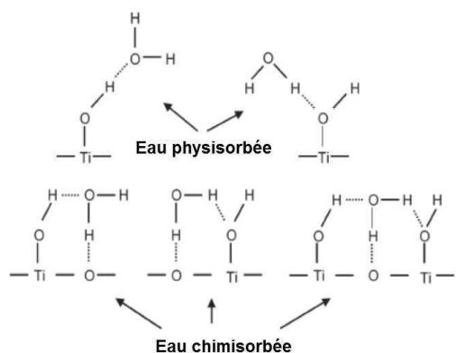
Figure I-8 : Structure de l'eau sur la surface de \text{TiO}_2 [39].
