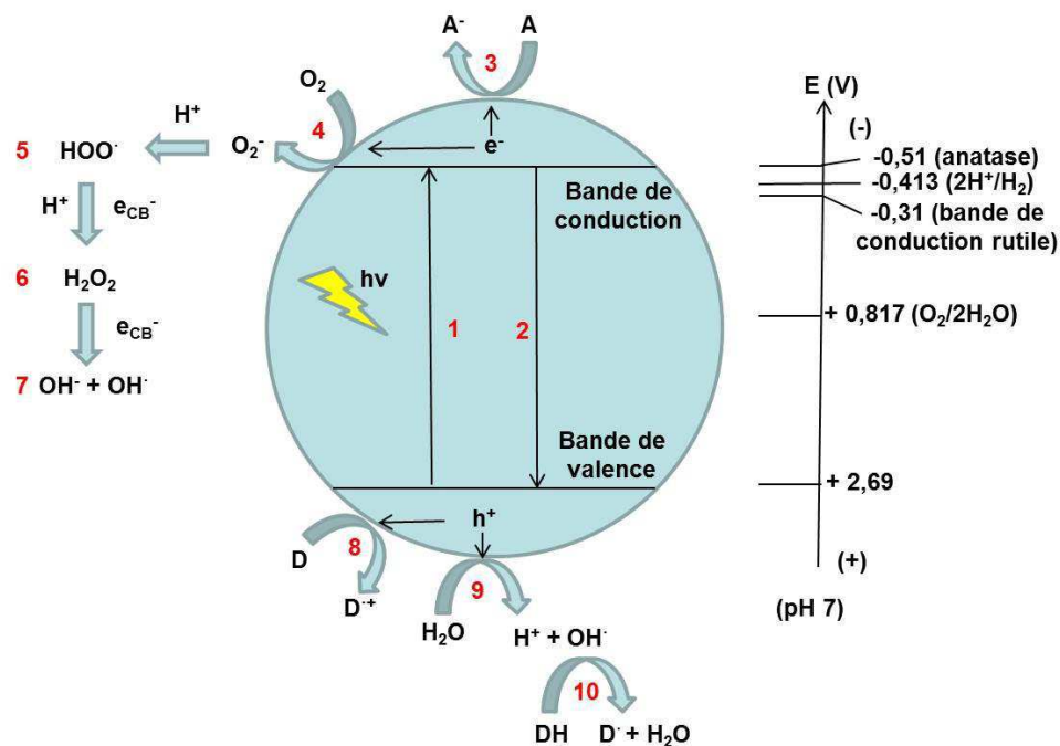
Figure I-10: illustration schématique des mécanismes catalytiques du \text{TiO}_2 :
