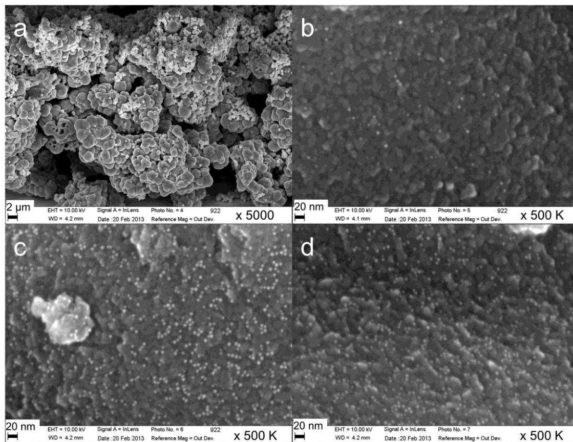
Figure III-19: Clichés MEB de la section d'un film de TiO 2 (synthèse A) imprégné d'or déposé au goutte à goutte à partir d'une dispersion dans l'hexane (a). Zooms sur les couches supérieures (b), médianes (c) et inférieure (d) du film.
