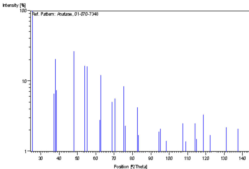
Figure 1: Fiche ICSD n° 01-070-7348 pour \text{TiO}_2 anatase.
