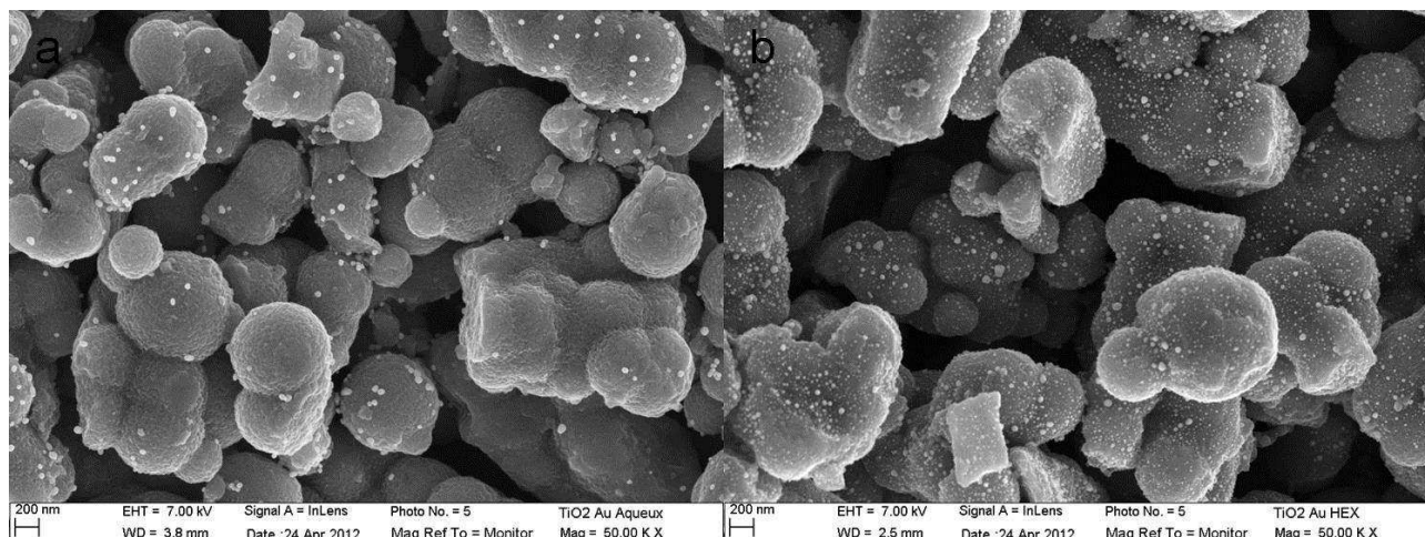
Figure III-15 : Clichés MEB de sections de films de \text{TiO}_2 issus de la synthèse A imprégnés d'or par dépôt goutte à goutte de solutions d'or synthétisées par voie aqueuse (a) et organique (b).
