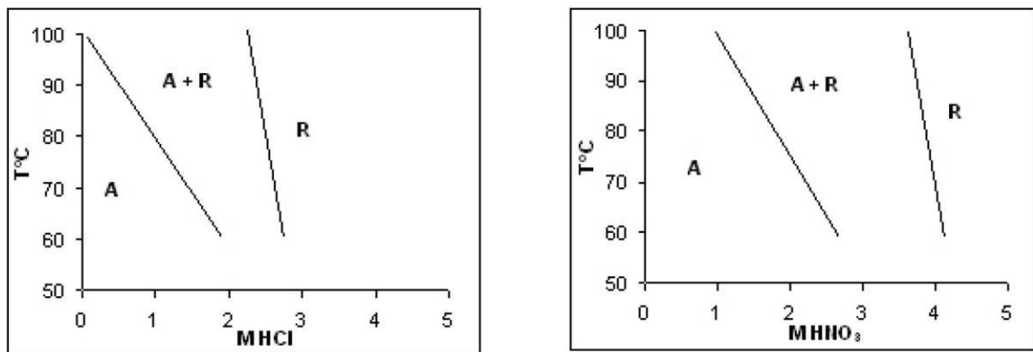
Figure I-2 : Domaine de précipitation du rutile (R) et de l'anatase (A) en fonction de la molarité en HCl ou HNO_3 et de la température des solutions aqueuses [2].
