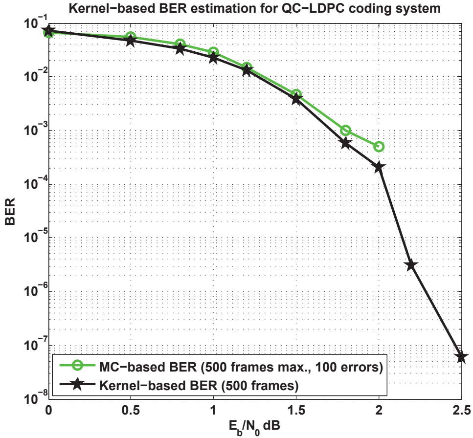
Figure 4 — L'estimation du BER par la méthode du noyau (LDPC codes, canal AWGN, N = 317\ 500 )
